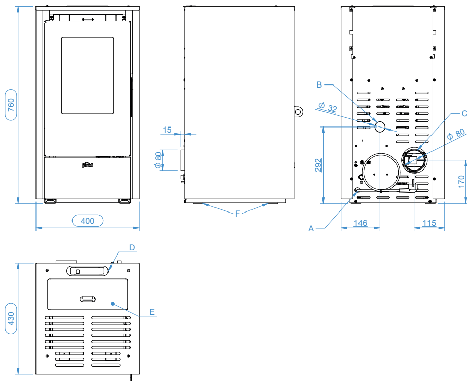
Disposição LIRA SLIM PLUS
