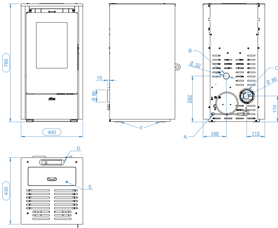
Layout LIRA SLIM PLUS
