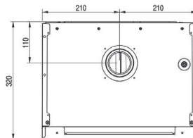
Vista superior
