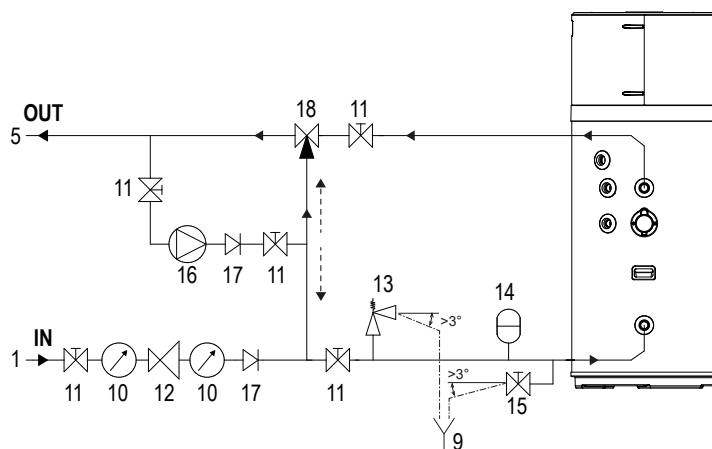
fig. 58 - Ejemplo de sistema de agua CON válvula mezcladora termostática (recirculación en la conexión de entrada de agua fría de la unidad)
