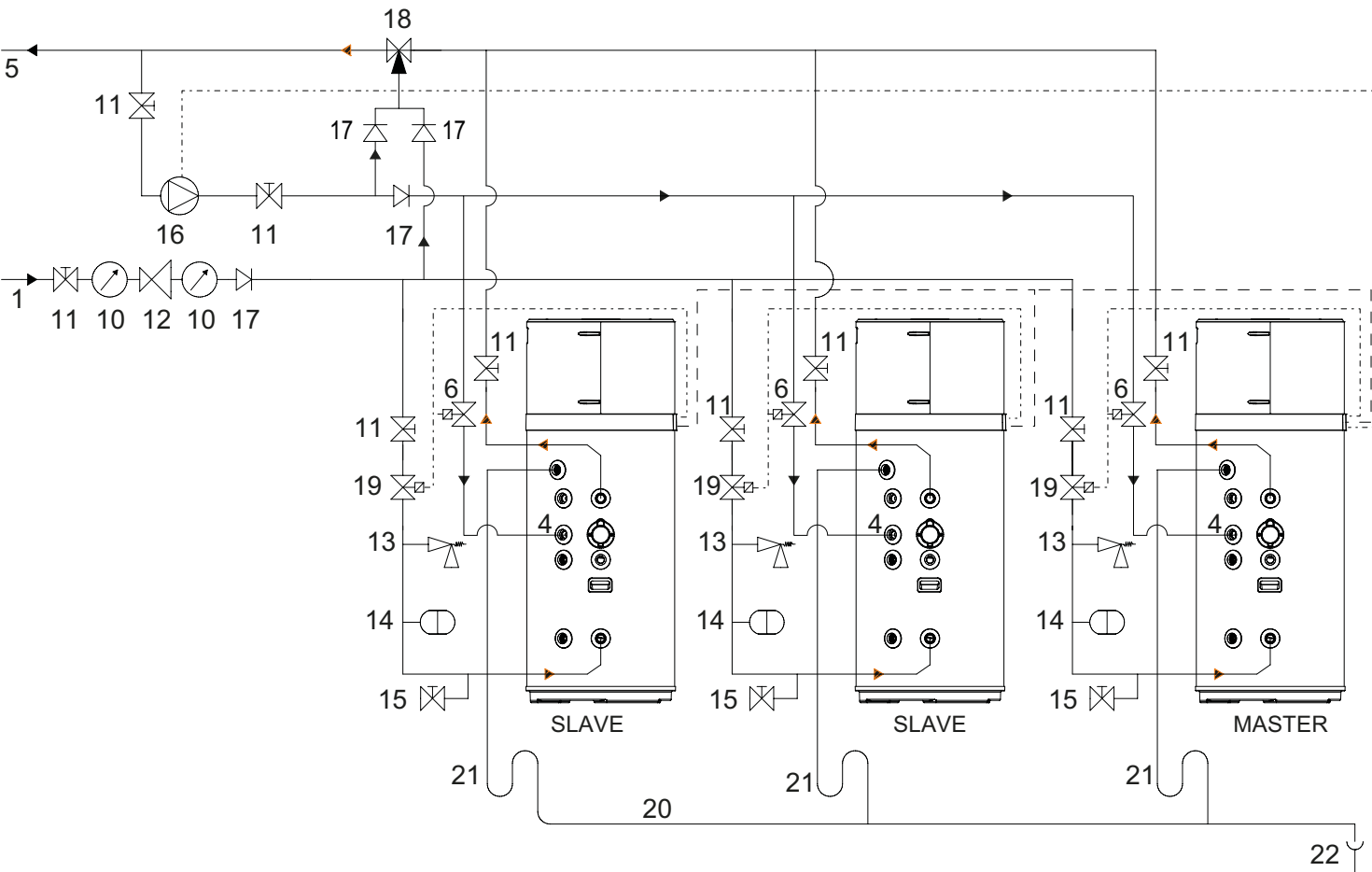
fig. 62 - Ejemplo de sistema de agua CON válvula mezcladora termostática (recirculación en conexión de recirculación de agua de la unidad)
