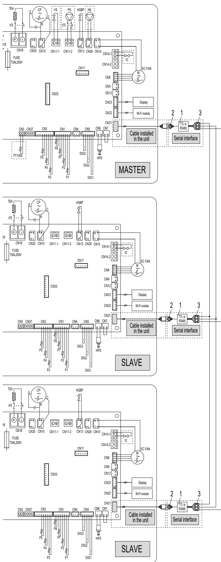
fig. 70 - Diagrama de cableado en cascada
