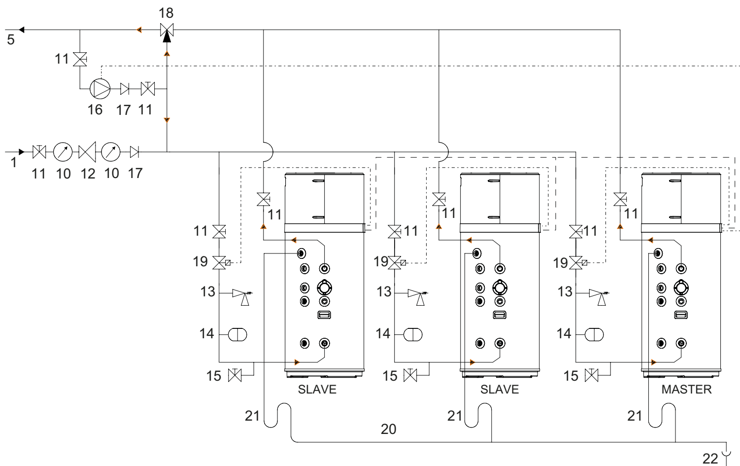
fig. 61 - Ejemplo de sistema de agua CON válvula mezcladora termostática (recirculación en la conexión de entrada de agua fría de la unidad)
