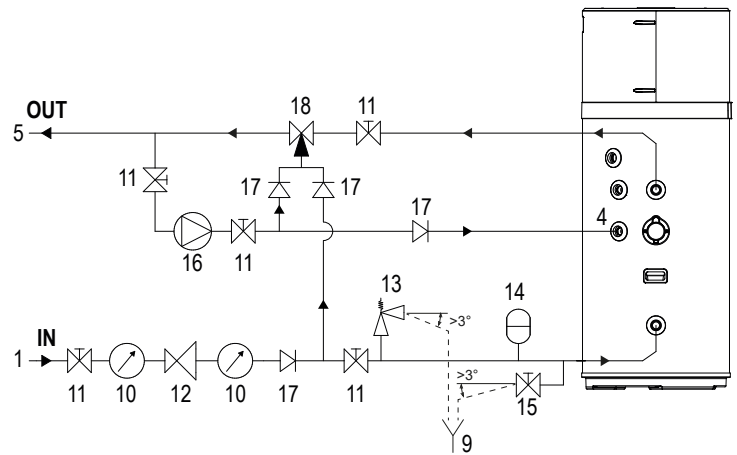
fig. 59 - Ejemplo de sistema de agua CON válvula mezcladora termostática (recirculación en la conexión de recirculación de agua de la unidad)
