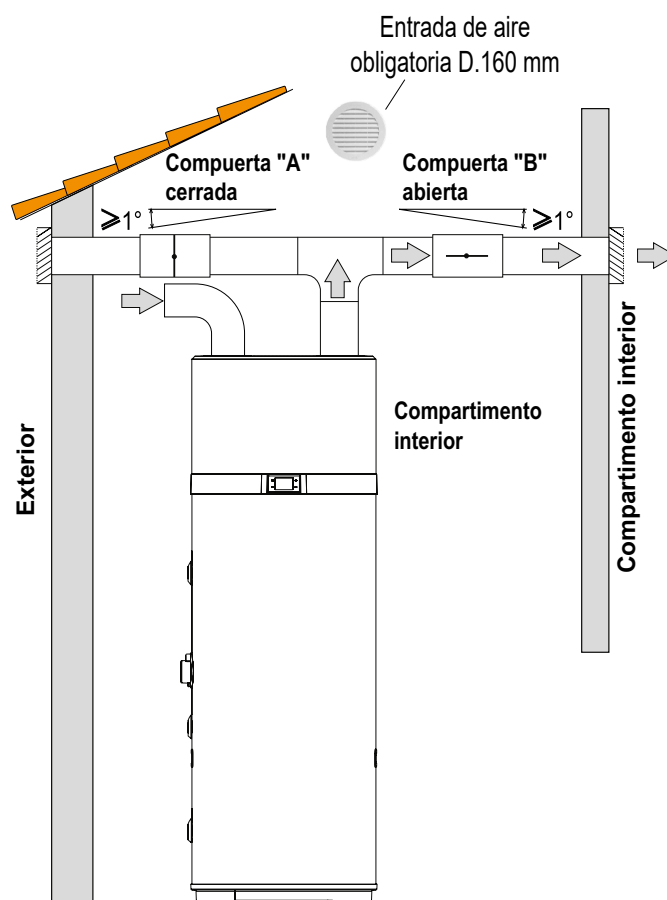
fig. 54- Ejemplo de instalación para la temporada estival
