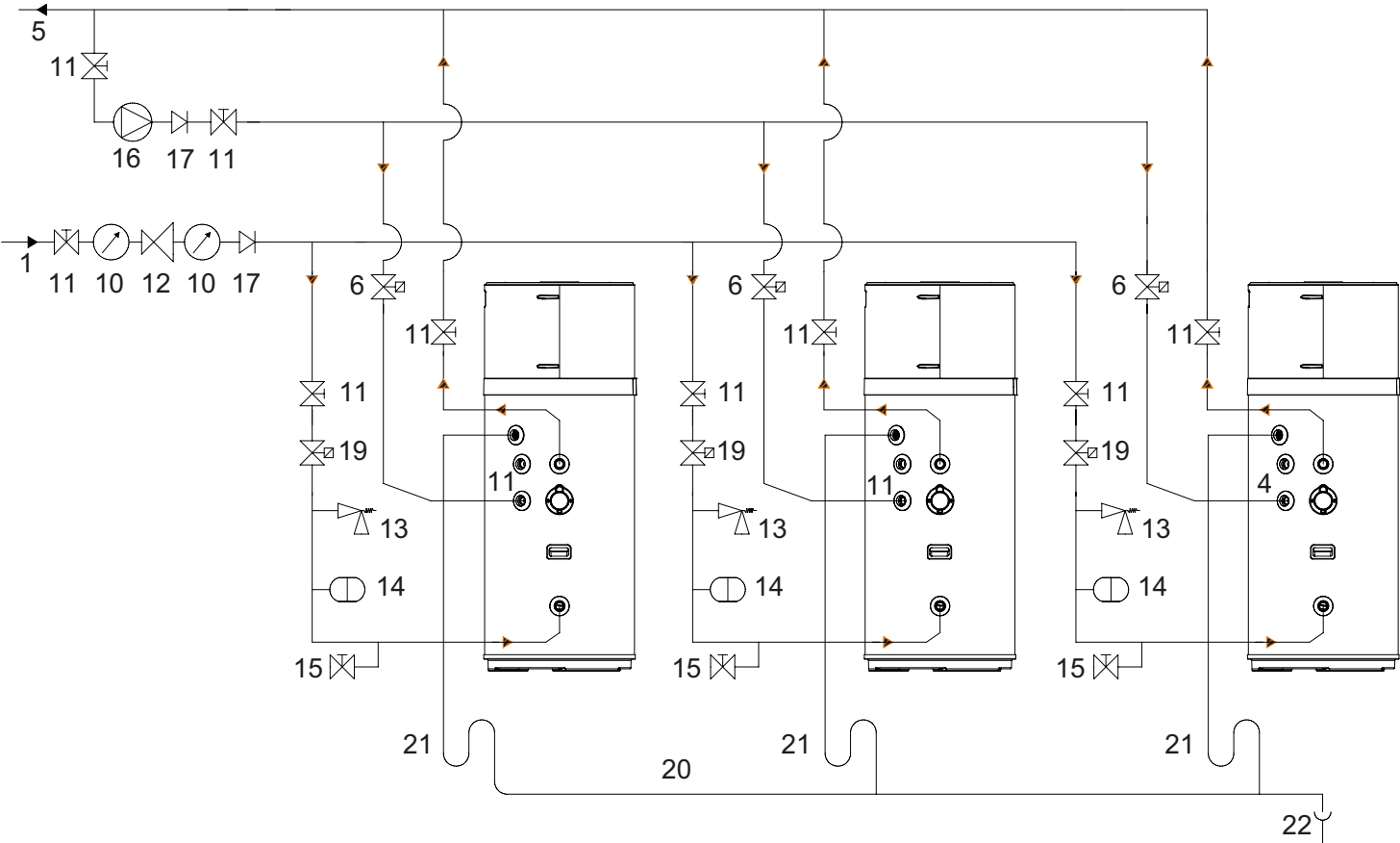
fig. 60 - Ejemplo de sistema de agua SIN válvula mezcladora termostática
