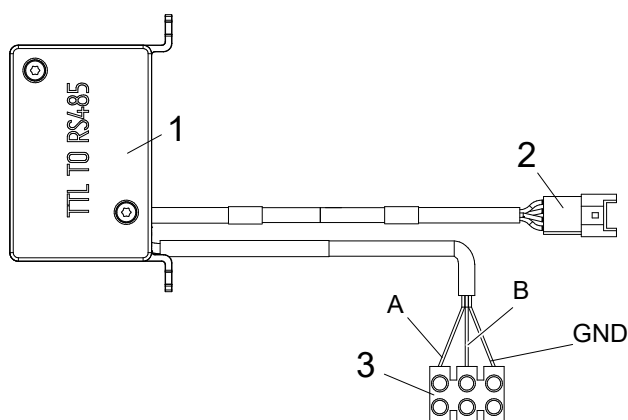
fig. 69 - Kit de interfaz serie TTL-RS485
