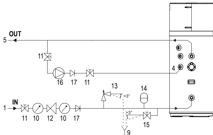
fig. 57 - Ejemplo de sistema de agua SIN válvula mezcladora termostática
