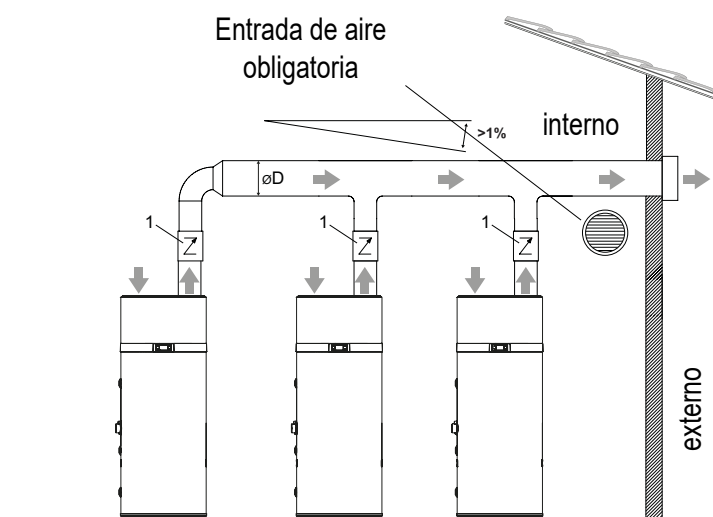
fig. 53 - Ejemplo de conexión de descarga de aire
