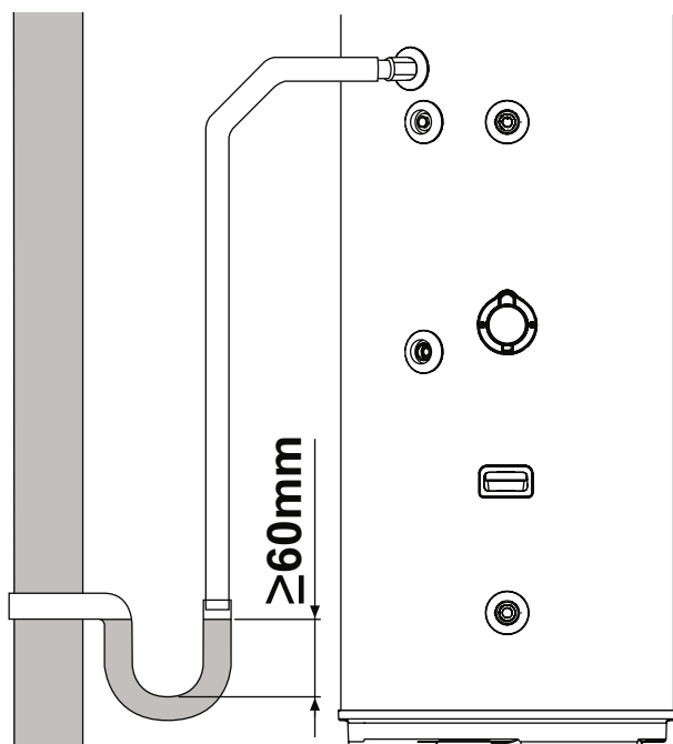
fig. 63- Ejemplos de conexión de drenaje de condensación a través de una trampilla
