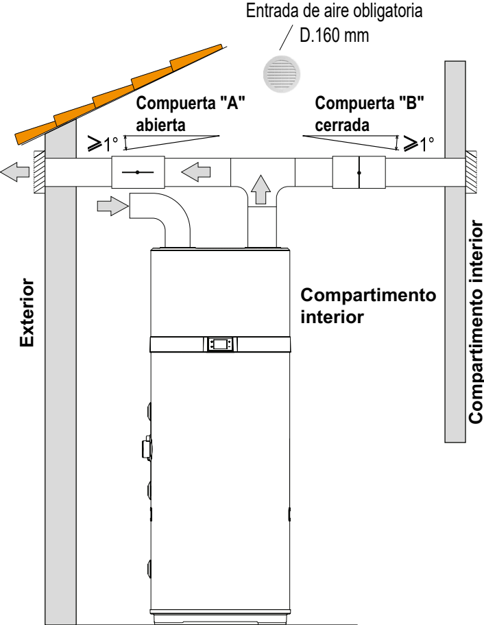
fig. 55- Ejemplo de instalación para la temporada invernal
