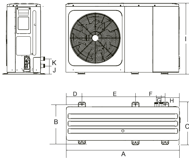
8/10/12/14/16 kW (unidad:mm)
