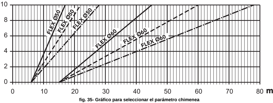
fig. 35- Gráfico para seleccionar el parámetro chimenea
