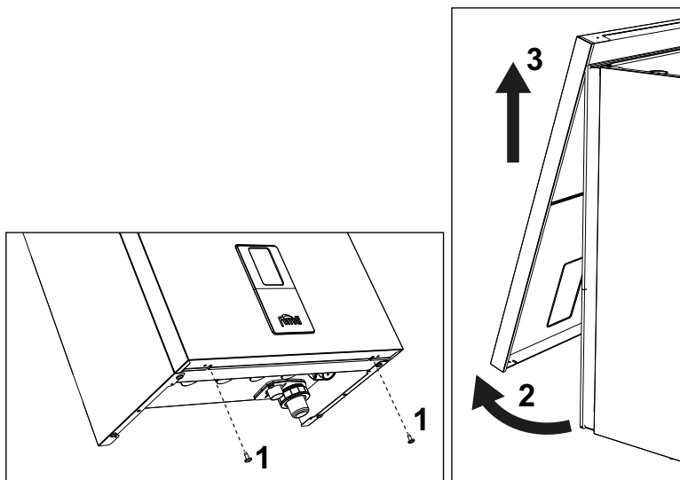
fig. 41- Apertura del panel frontal
