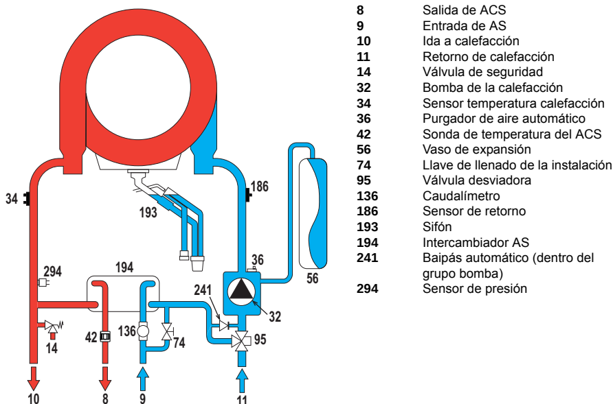
fig. 63- Circuito hidráulico
