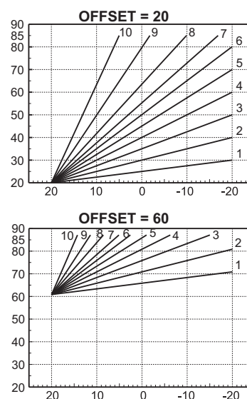
fig. 31- Déplacement parallèle des courbes de compensation
