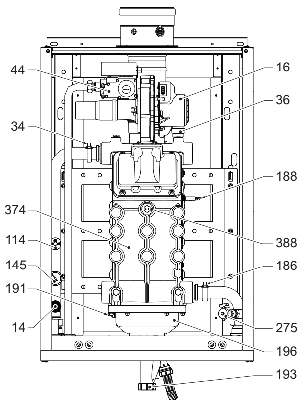
рис. 89- Общий вид, мод. FORCE W 60 и FORCE W 80
