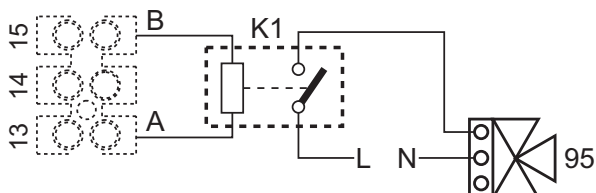
fig. 96- Racordarea valvei cu 3 căi cu 2 fire
