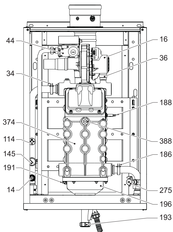
fig. 89- Vedere generală mod. FORCE W 60 și FORCE W 80
