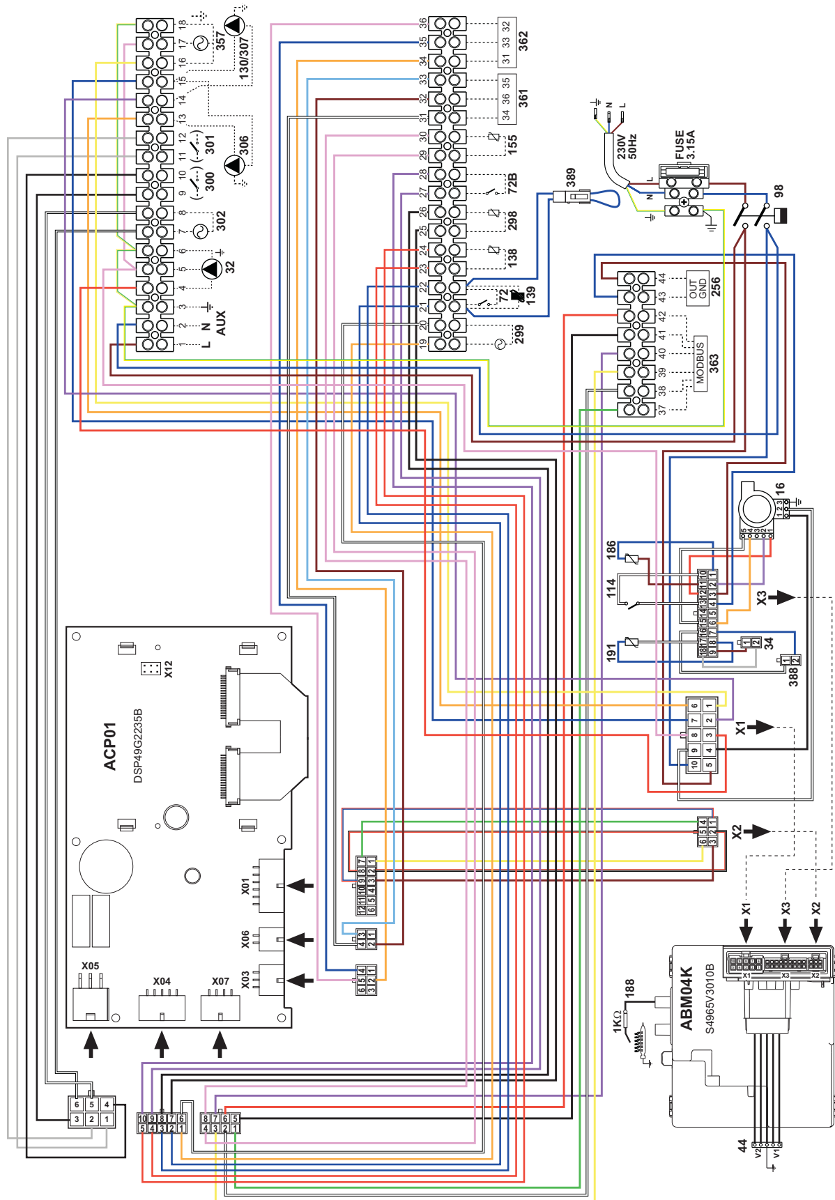
fig. 99- Schemă electrică modelele FORCE W 60 i FORCE W 80
