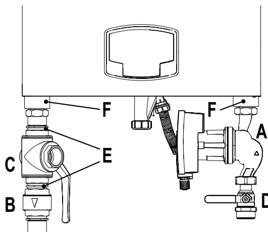
fig. 34- Chaudière avec les kits installés
