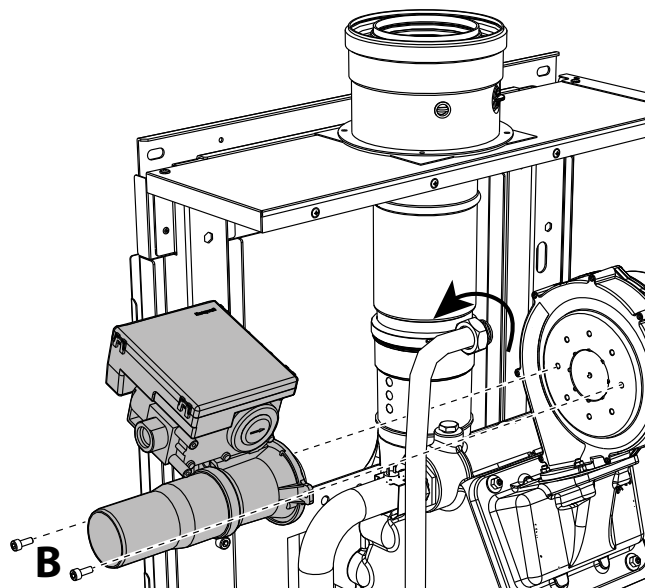
fig. 70- Modelele W 60 și W 80
