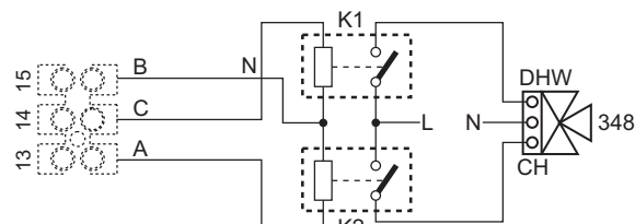
wygląd 97- Podłączenie zaworu 3-drożnego z 3 żyłami
