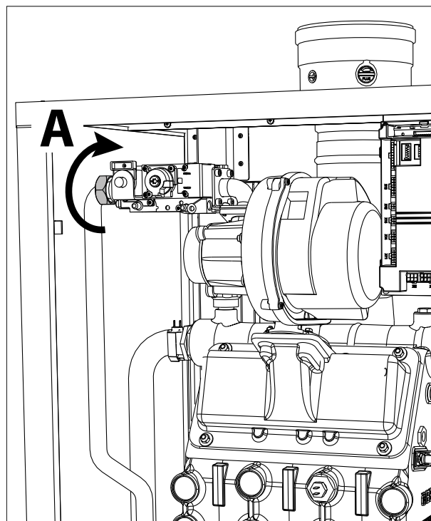
fig. 69- Modèles W 99, W 120 et W 150
