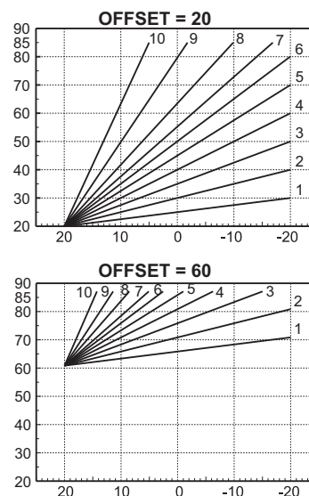
fig. 31 - Spostamento parallelo delle curve di compensazione
