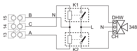
fig. 97- Racordarea valvei cu 3 căi cu 3 fire
