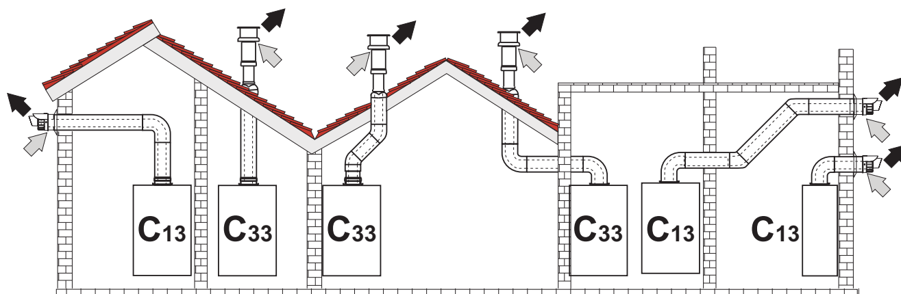
fig. 58- Exemple de racordare cu tuburi coaxiale
