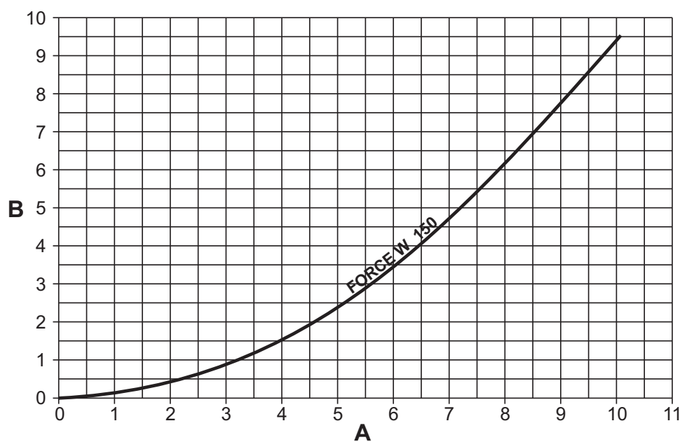
fig. 94- Diagrama de pérdida de carga modelos FORCE W 150
