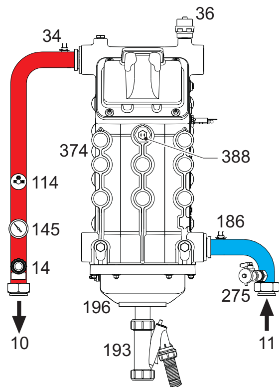
fig. 92- Circuito hidráulico
