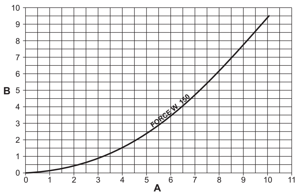
fig. 94- Diagramă pierderi de sarcină modelele FORCE W 150
