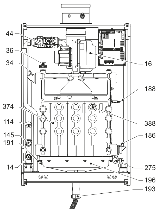
fig. 91- Vue générale mod. FORCE W 150
