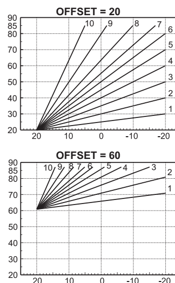
рис. 31- Параллельное смещение компенсационных кривых
