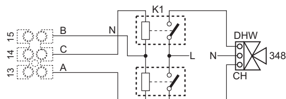
рис. 97- Подключение 3-х ходового клапана с 3 проводами
