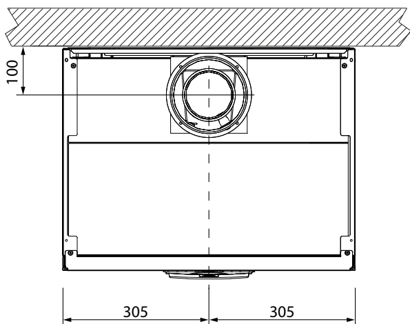
fig. 87- Vedere de sus
