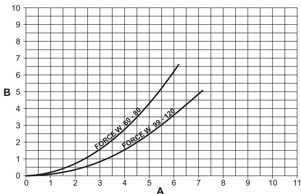
fig. 93- Diagramă pierderi de sarcină modelele FORCE W 60 - FORCE W 80 - FORCE W 99 - FORCE W 120
