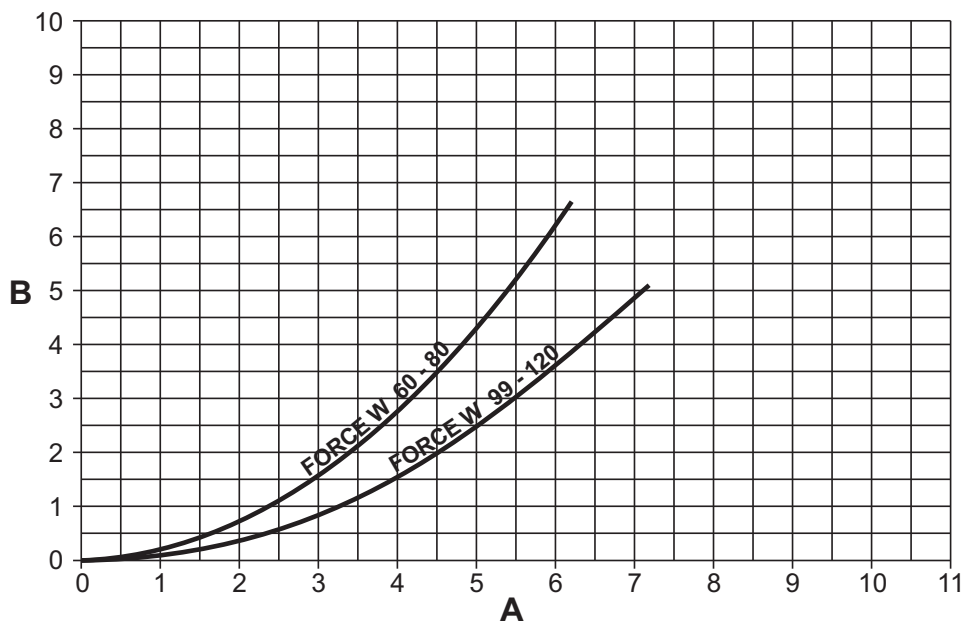
fig. 93- Diagramme perte de charge modèles FORCE W 60 - FORCE W 80 - FORCE W 99 - FORCE W 120
