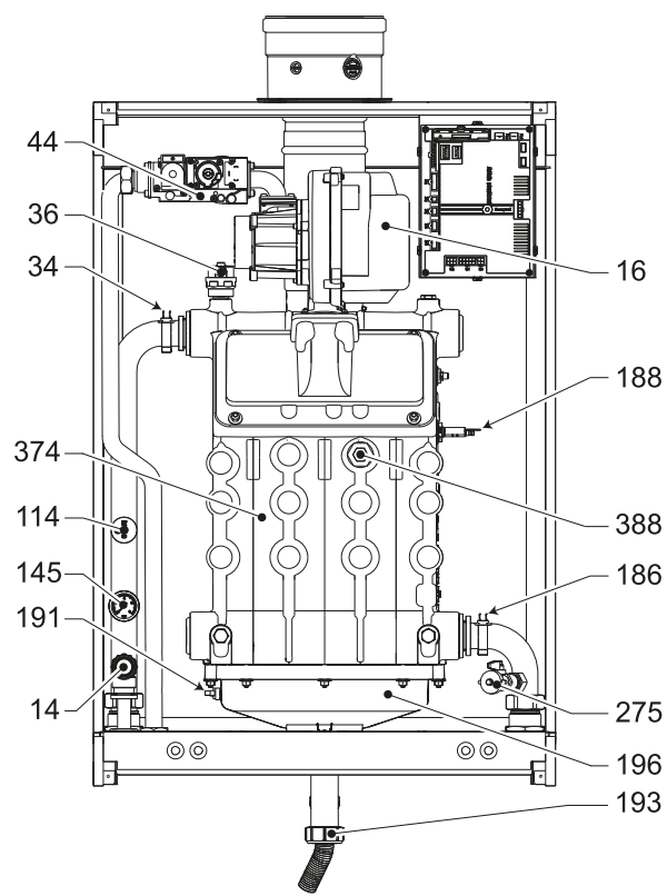
рис. 90- Общий вид, мод. FORCE W 99 и FORCE W 120
