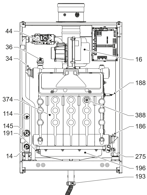
рис. 91- Общий вид, мод. FORCE W 150
