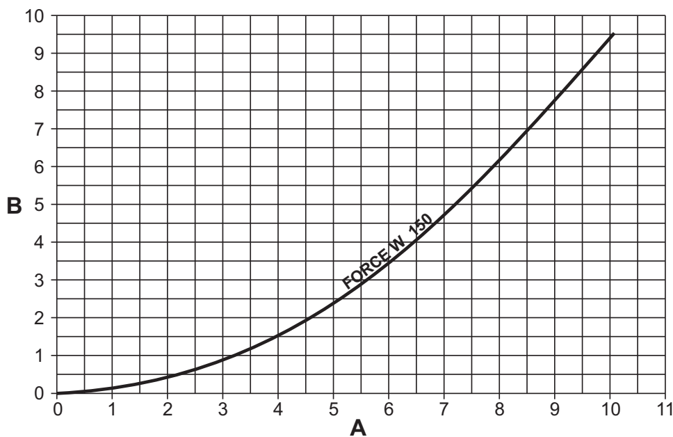
fig. 94 - Diagramma perdita di carico modelli FORCE W 150
