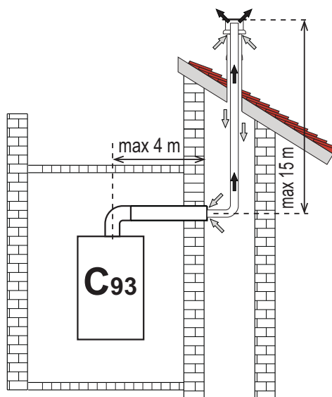
wygląd 62- Przykłady podłączenia do przewodów zbiorczych (⇨ = Powietrze / ⇨ = Spaliny)
