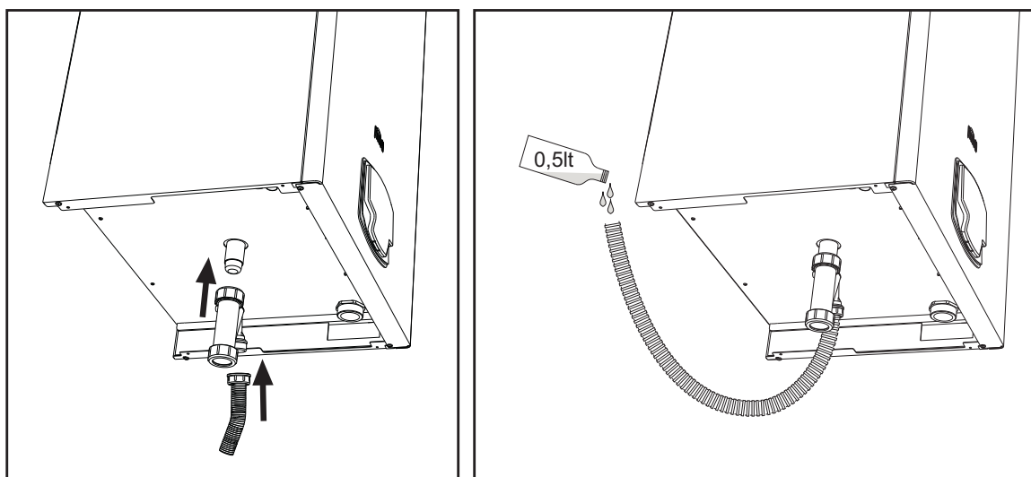
fig. 67- Racordarea evacuării condensului
