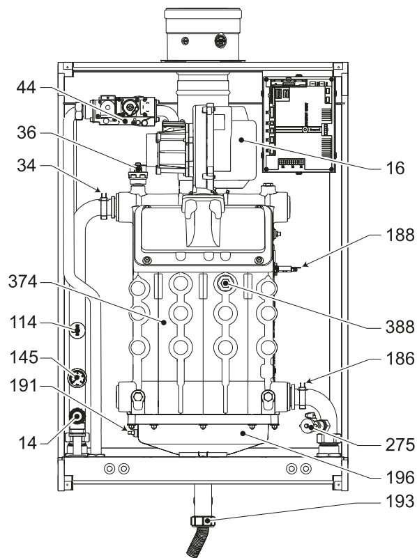
fig. 90 - Vista generale mod. FORCE W 99 e FORCE W 120
