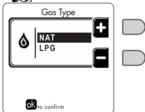
fig. 75- Selectarea tipului de gaz
