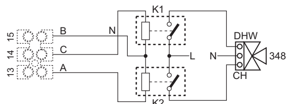
fig. 97- Raccordement de la vanne 3 voies à 3 fils
