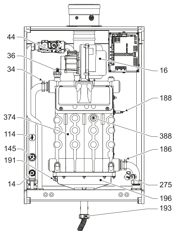
fig. 90- Vedere generală mod. FORCE W 99 și FORCE W 120
