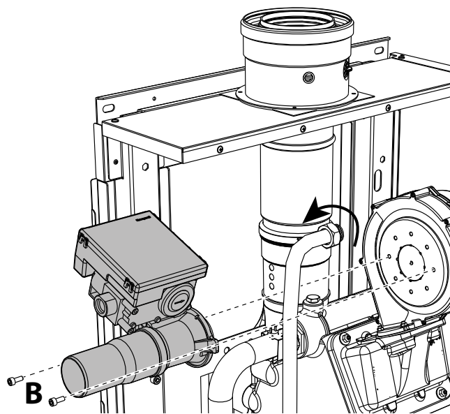
wygląd 70- Modele W 60 i W 80
