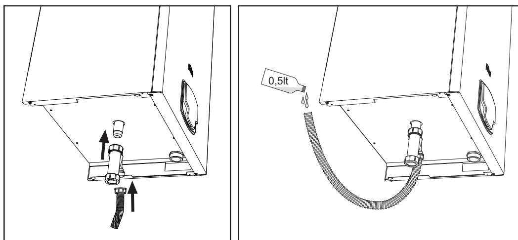
wygląd 67- Podłączenie spustu kondensatu
