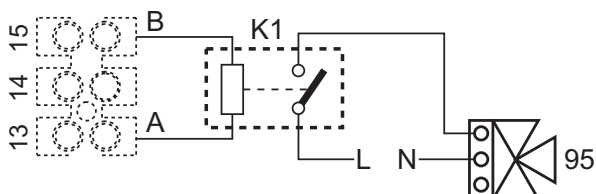
wygląd 96- Podłączenie zaworu 3-drożnego z 2 żyłami
