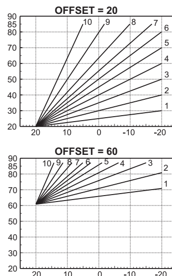
fig. 31- Deplasarea paralelă a curbelor de compensare
