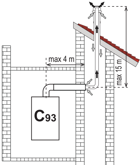
fig. 62- Exemple de racordare la hornuri (⇨ = Aer / ⇨ = Gaze arse)
