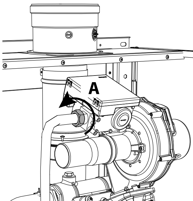
wygląd 68- Modele W 60 i W 80
