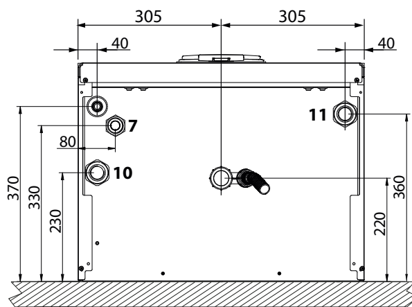
fig. 88- Vedere de jos
