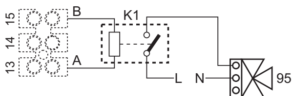
fig. 96- Raccordement de la vanne 3 voies à 2 fils
