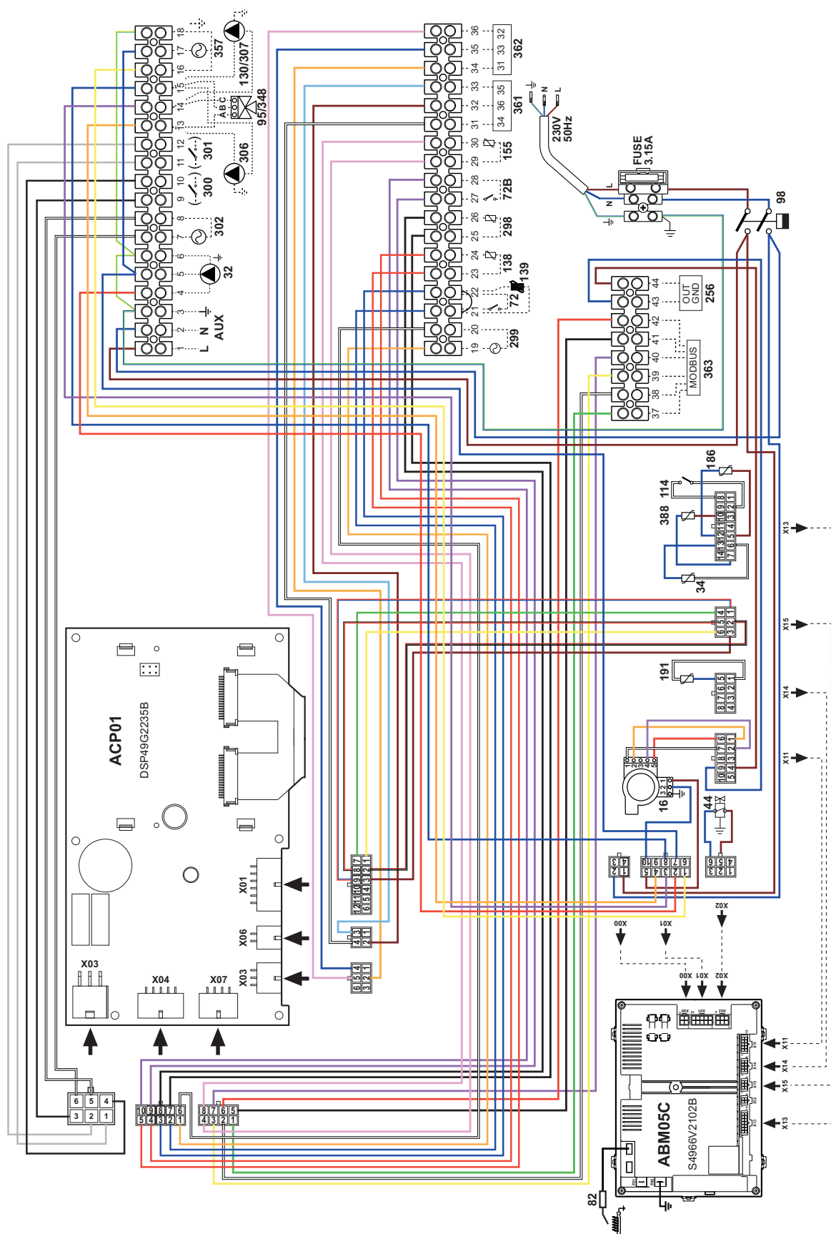
fig. 100 - Schema elettrico modelli FORCE W 99, FORCE W 120 e FORCE W 150
