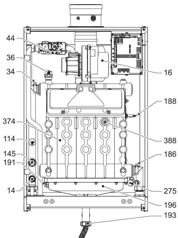
wygląd 91- Widok ogólny mod. FORCE W 150
