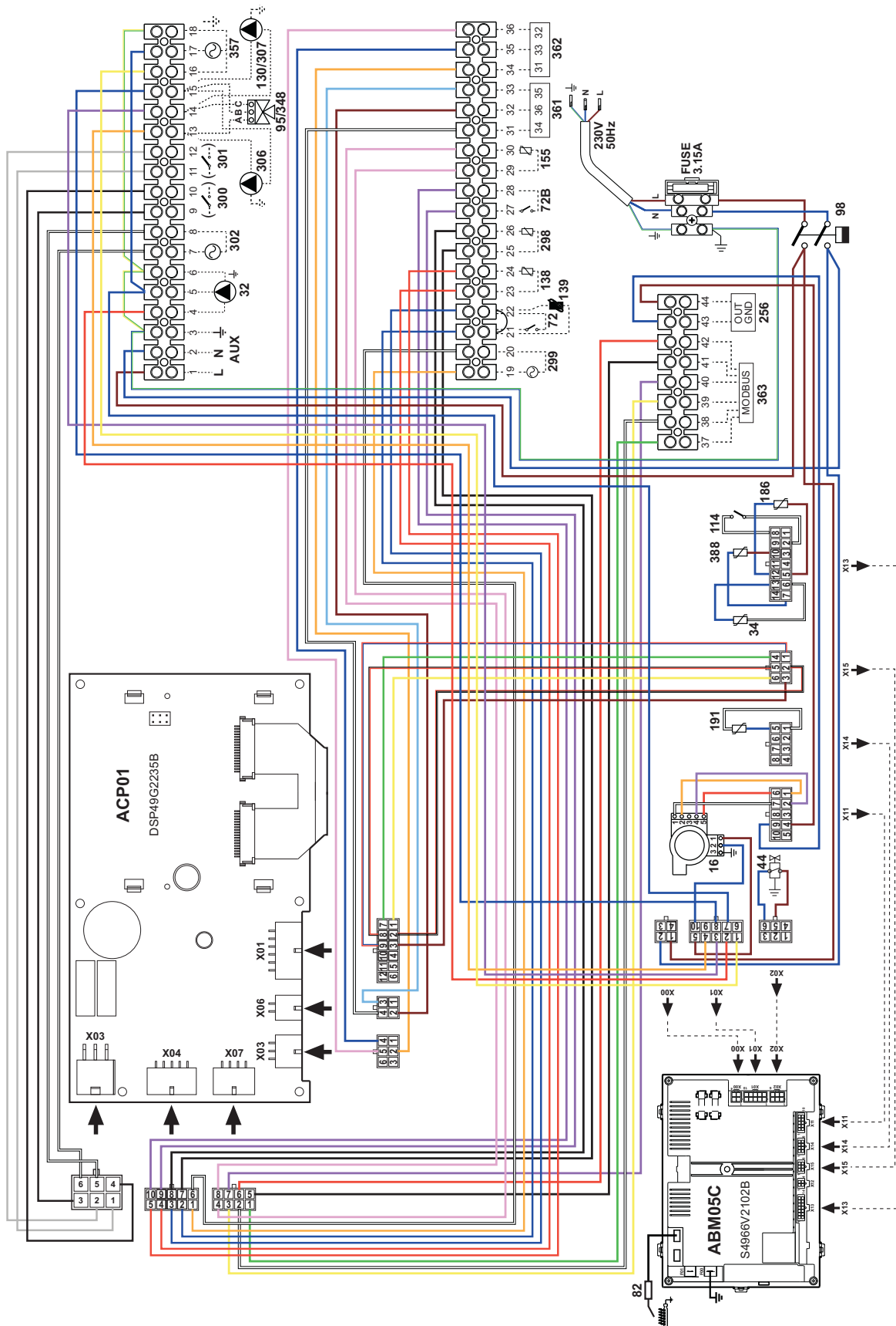
fig. 100- Esquema eléctrico modelos FORCE W 99, FORCE W 120 y FORCE W 150
