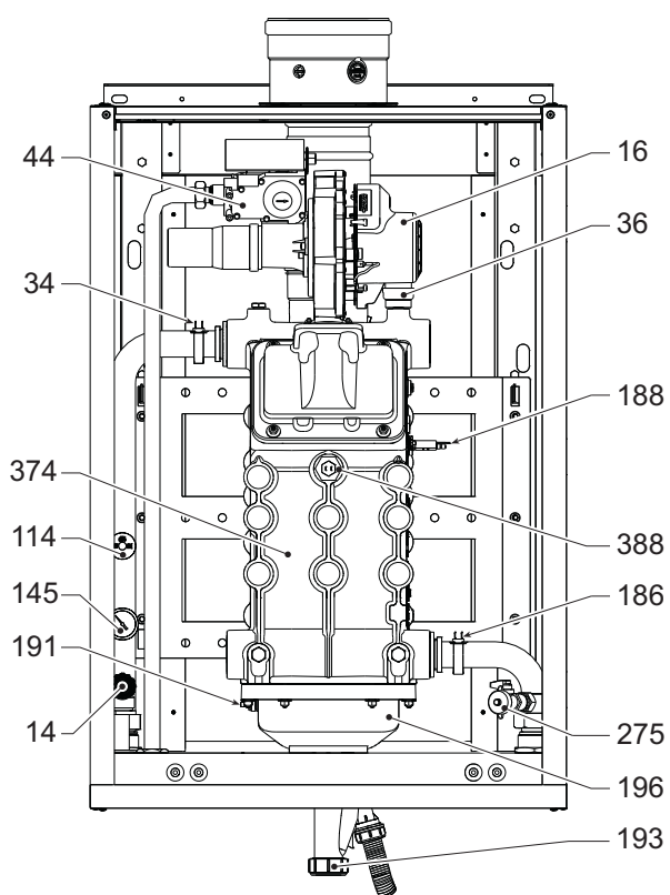
wygląd 89- Widok ogólny mod. FORCE W 60 i FORCE W 80
