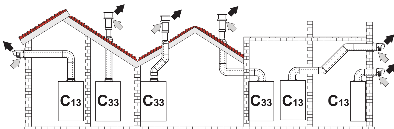
wygląd 58- Przykłady połączenia przewodami współosiowymi
