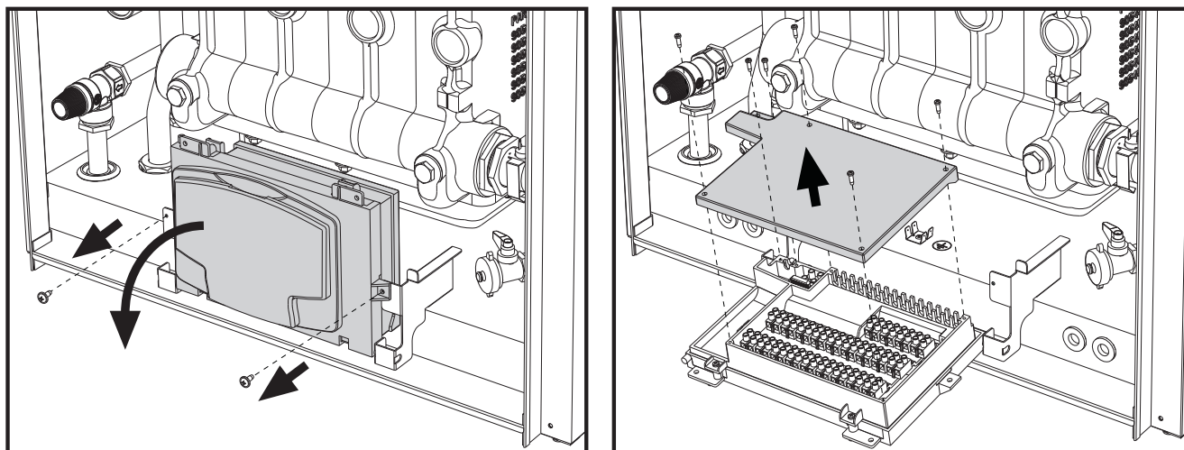
fig. 52- Bornier électrique
