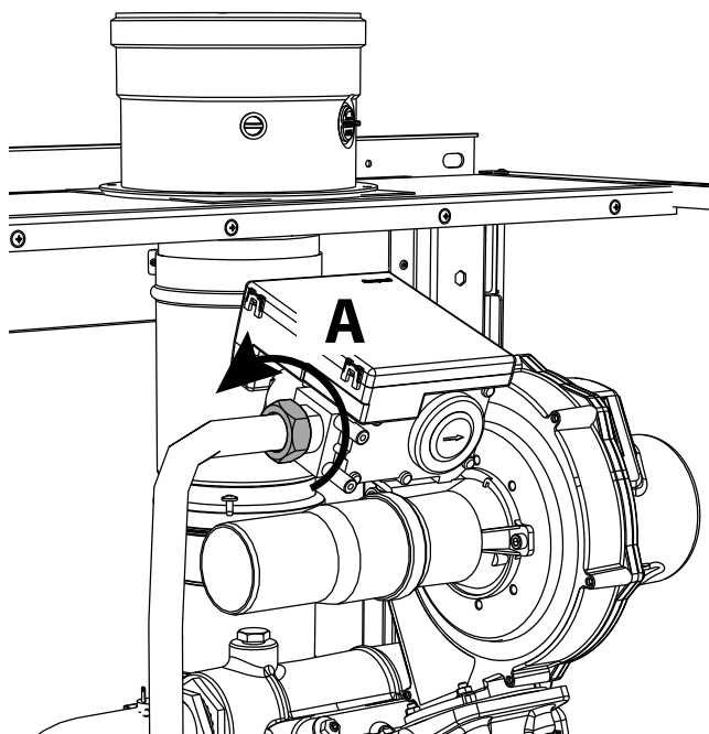
fig. 68- Modelele W 60 și W 80
