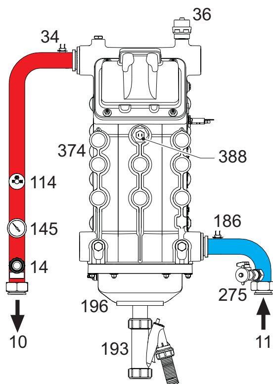
fig. 92- Circuitul hidraulic
