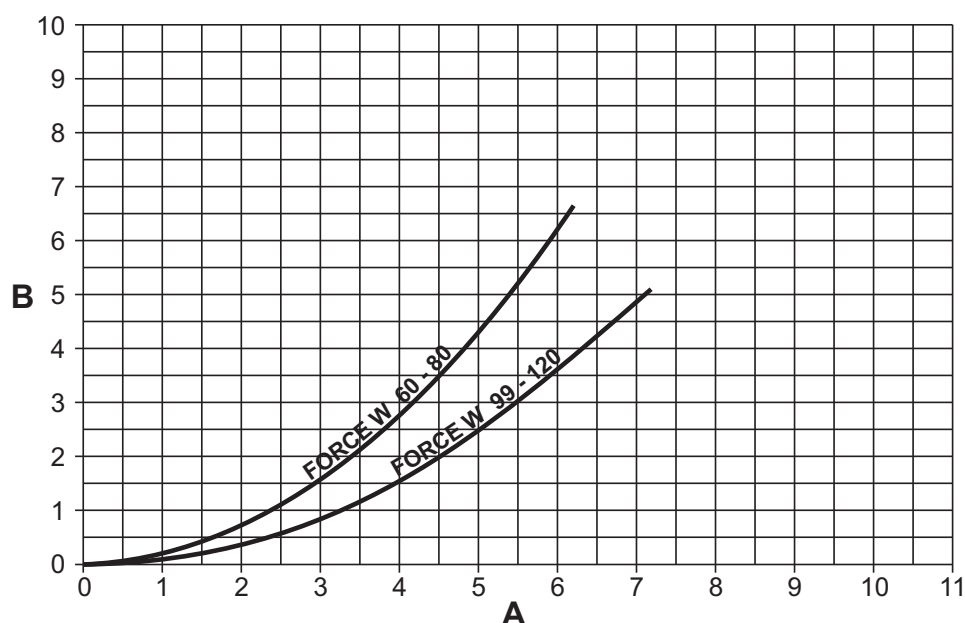
fig. 93- Diagrama de pérdida de carga modelos FORCE W 60 - FORCE W 80 - FORCE W 99 - FORCE W 120
