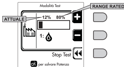
fig. 79 - Modalità TEST (esempio potenza riscaldamento = 80%)
