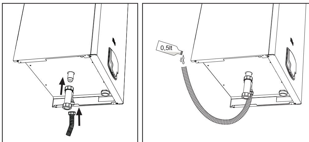
fig. 67- Raccordement de l'évacuation des condensats
