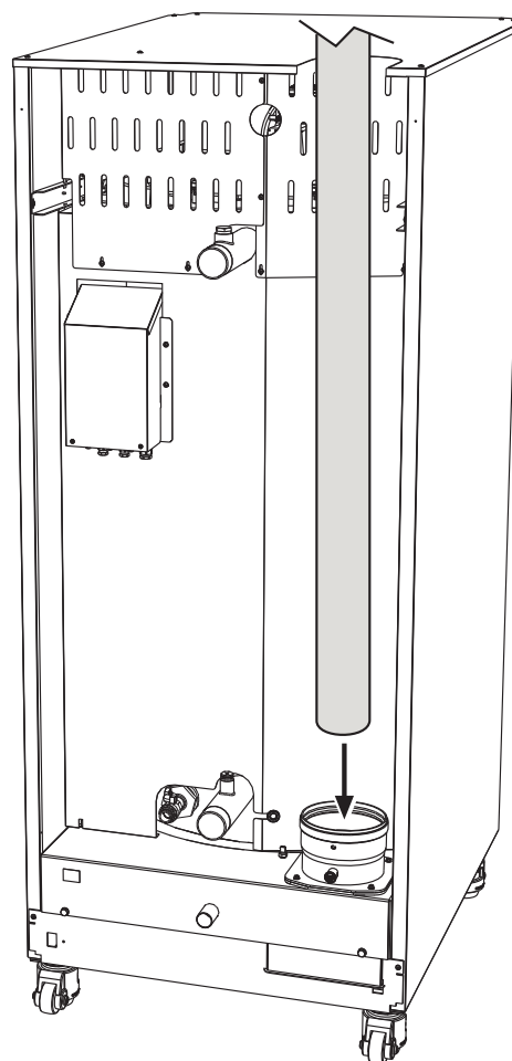
рис. 57- Выход дымов
