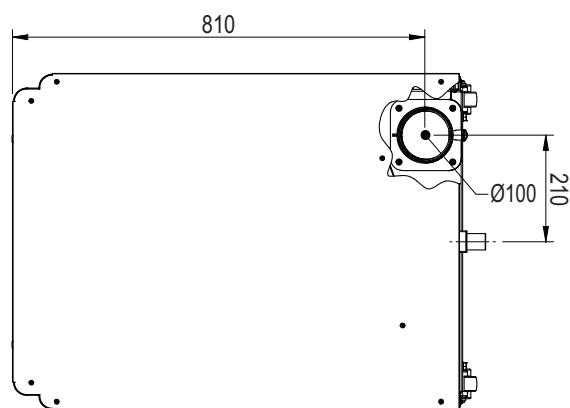
рис. 78- Сверху
