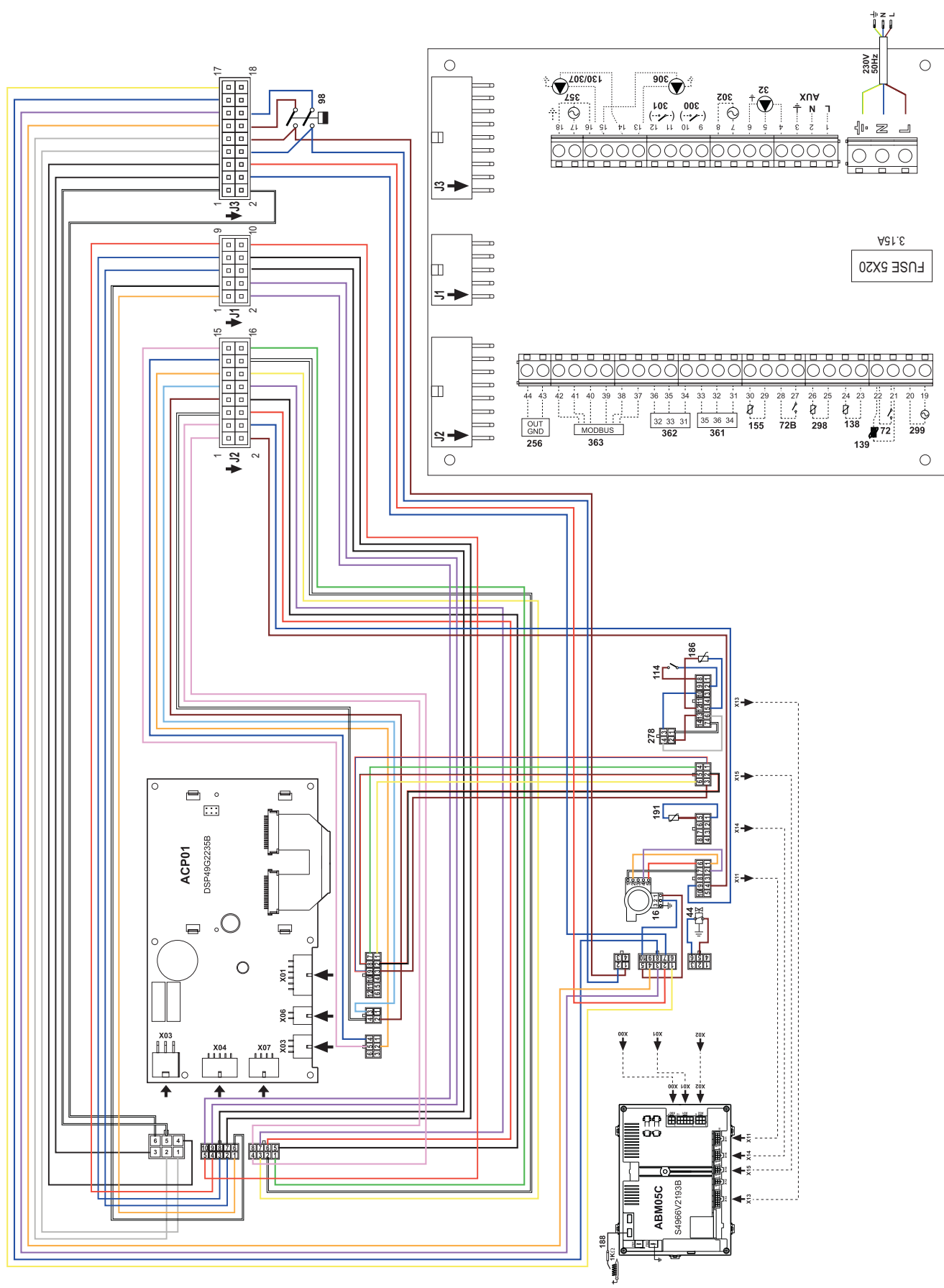
fig. 96 - Schema elettrico OPERA 125 e 160
