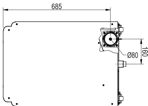
fig. 75- Haut
