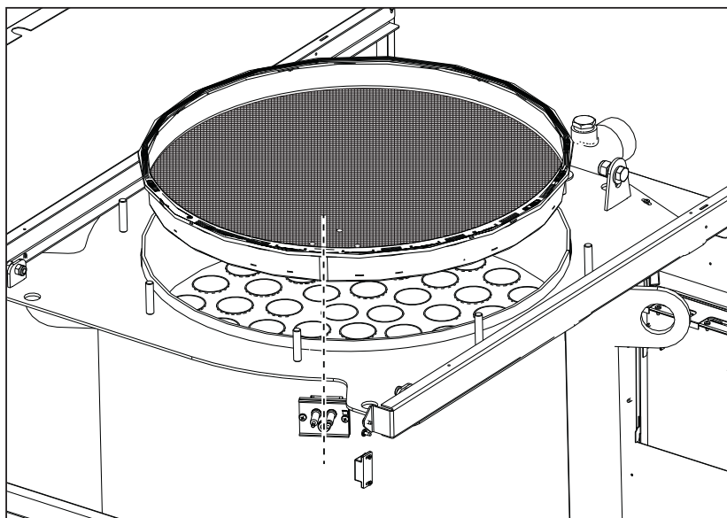
fig. 67 - Allineamento bruciatore
