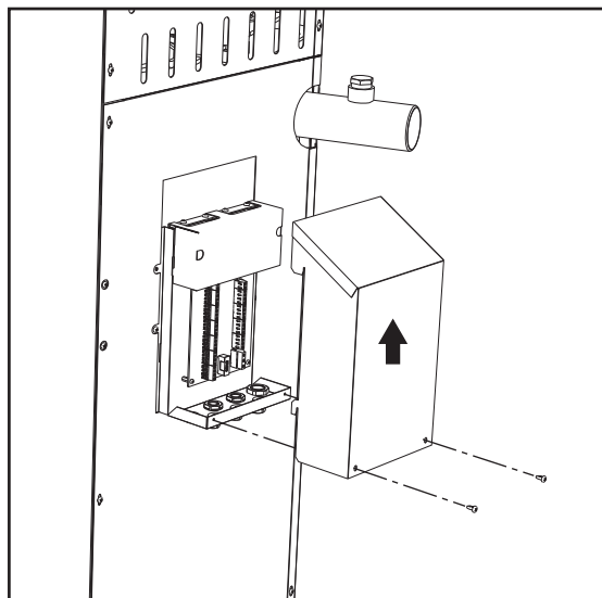
fig. 55 - Morsettiera elettrica
