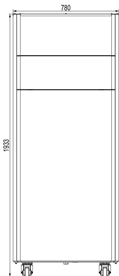
рис. 79- Спереди
