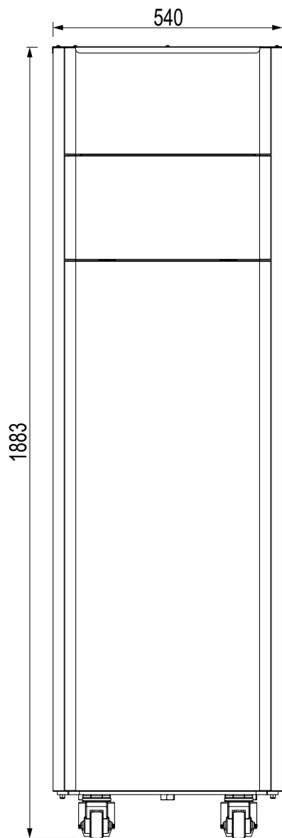
рис. 73- Спереди
