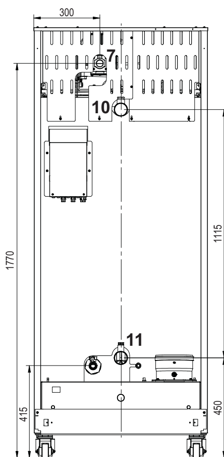
fig. 81- posterior 220
