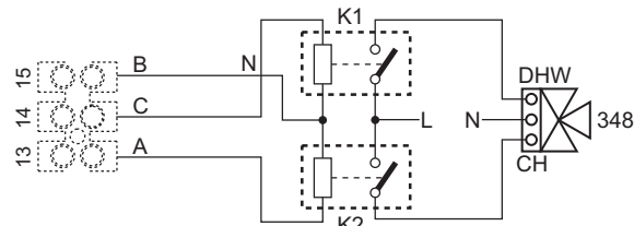
рис. 93- Подключение 3-х ходового клапана с 3 проводами
