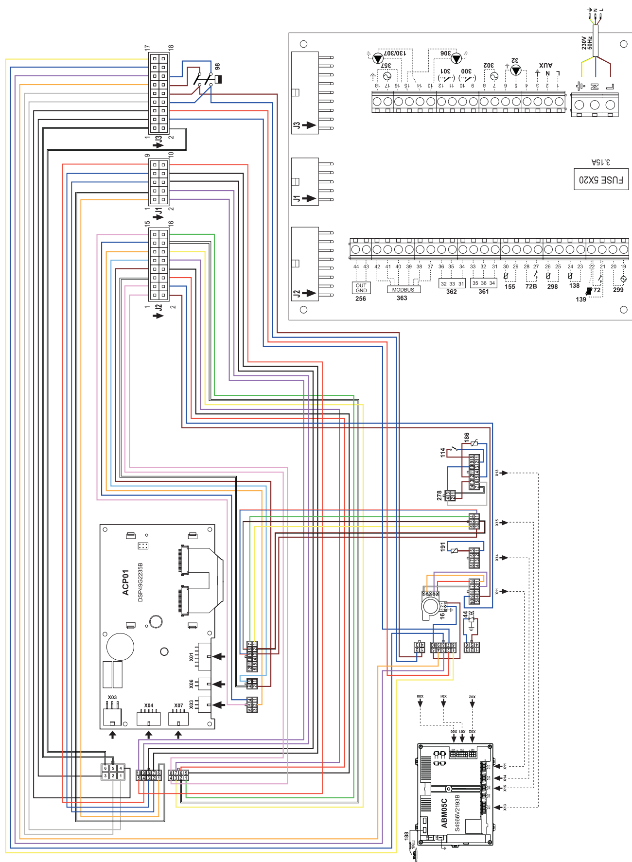
рис. 96- Электрическая схема OPERA 125 и 160
