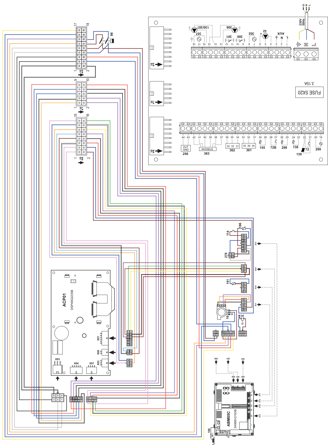
fig. 96- Schéma électrique OPERA 125 et 160
