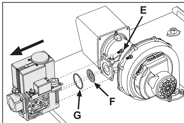
fig. 61- Modèle OPERA 220
