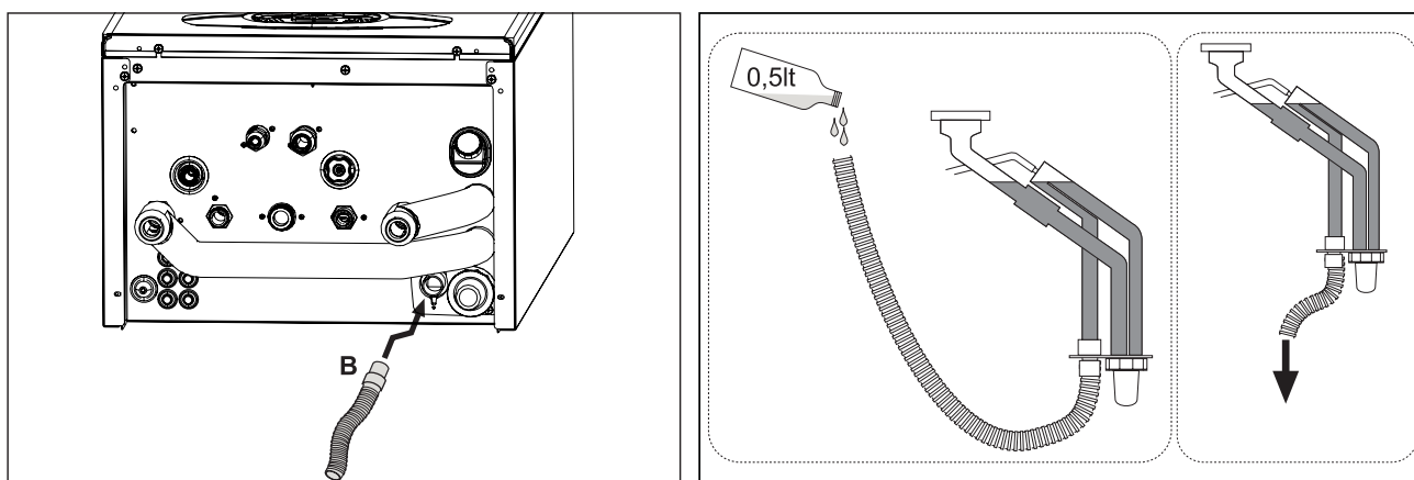
fig. 41 - Collegamento scarico condensa
