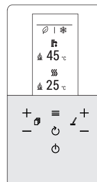
fig. 2 - interfaccia utente
