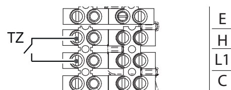
fig. 46 - Termostato metodo B (1 zona)
