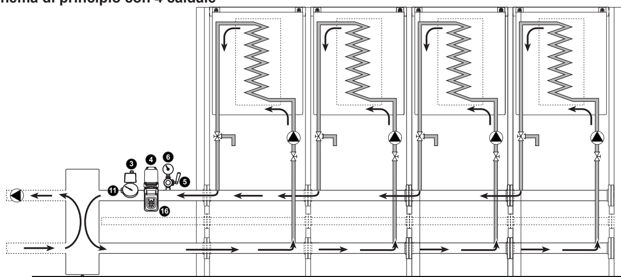
Schema di principio con 4 caldaie
