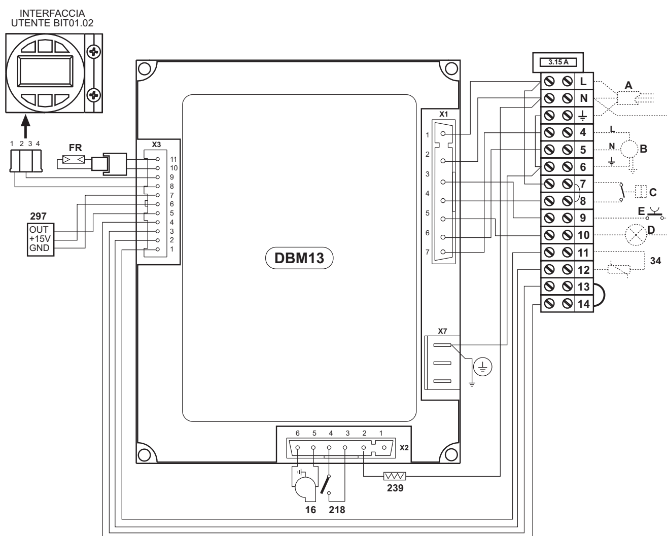
fig. 13 - Esquema eléctrico
