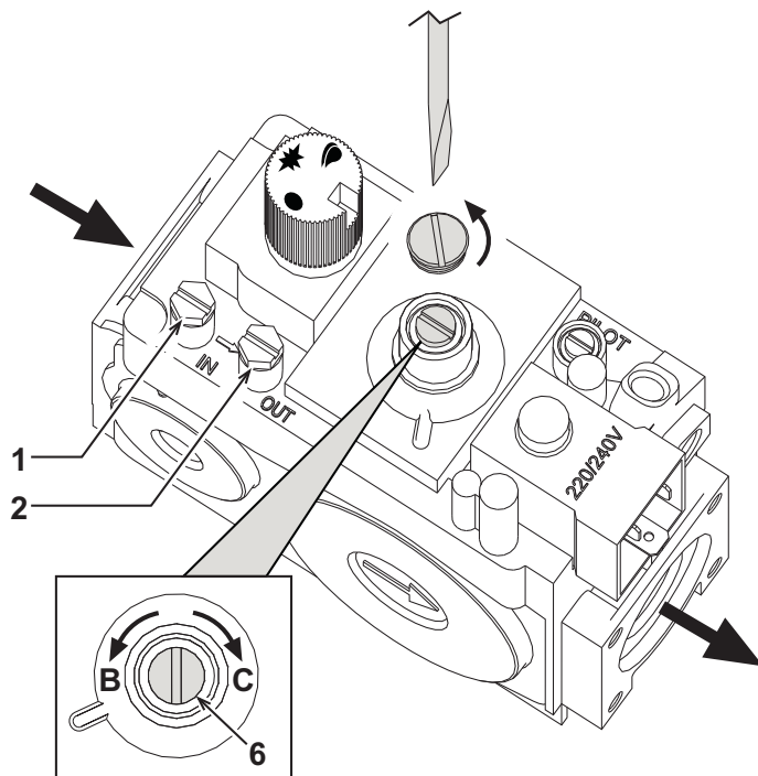
рис. 7 - Регулирование давления
