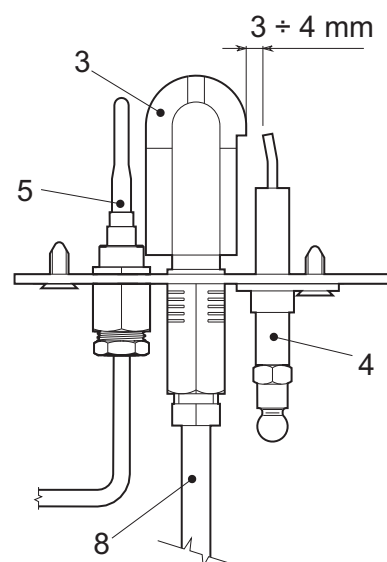
рис. 11 - Пилотная горелка
