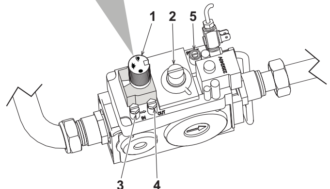
рис. 2 - Газовый клапан
