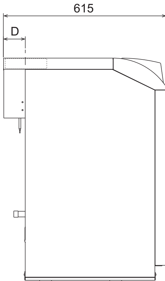
рис. 13 - Вид сбоку
