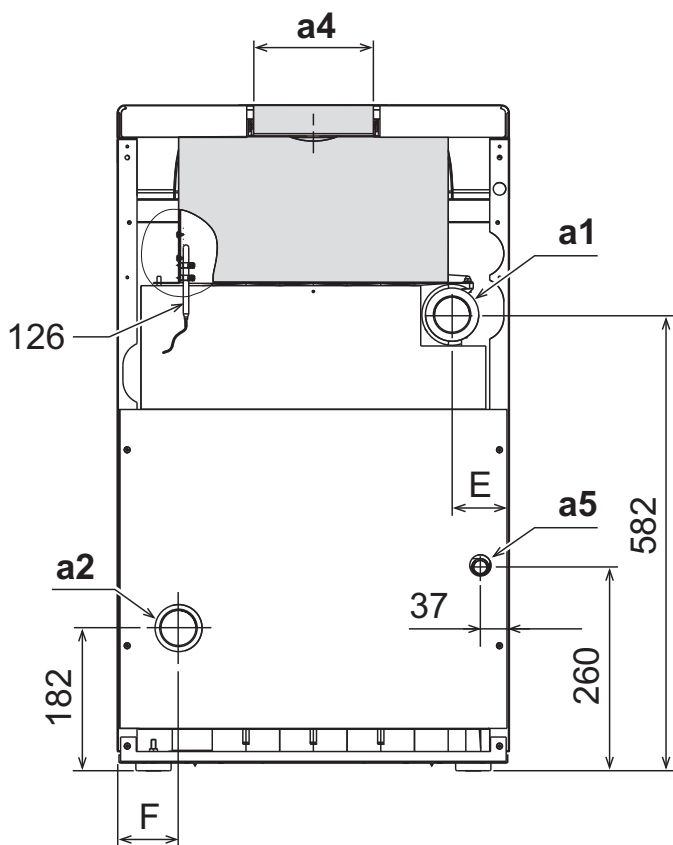
рис. 14 - Вид сзади
