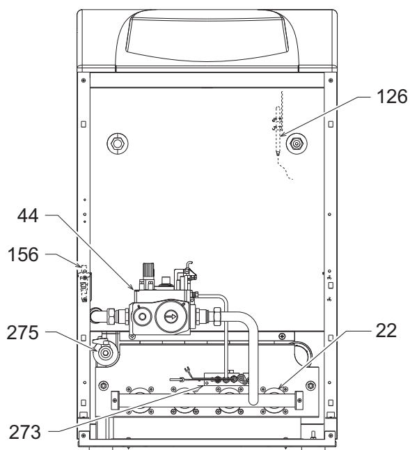
рис. 15 - Общий вид
