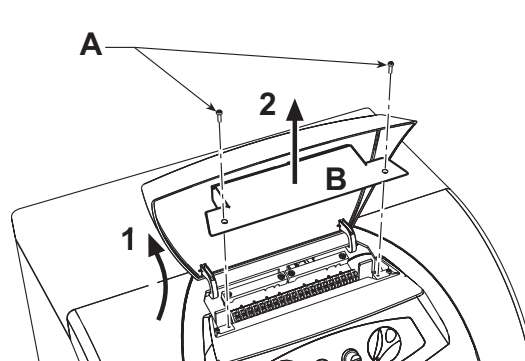
рис. 3 - Доступ к клеммной коробке
