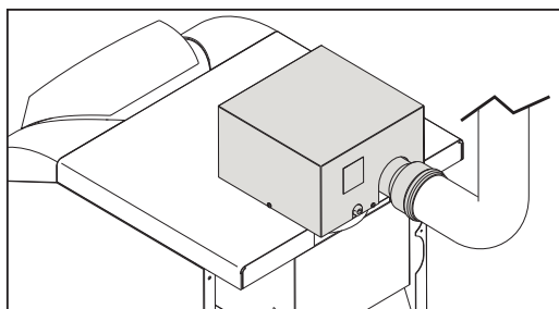
рис. 4 - Комплект дымососа
