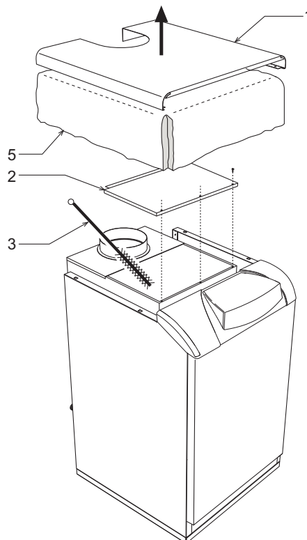
рис. 9 - Очистка котла
