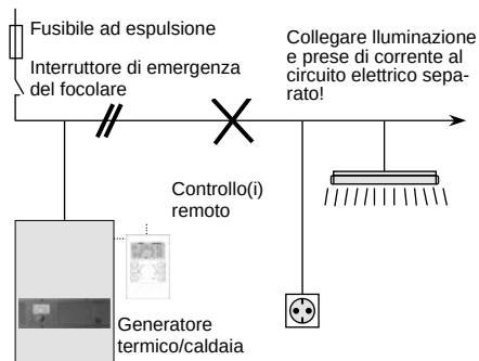
Fig. 3: Instradamento dei cavi elettrici nel focolare
