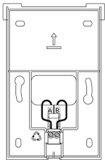
Supporto di allacciamento (parte superiore rimossa)
