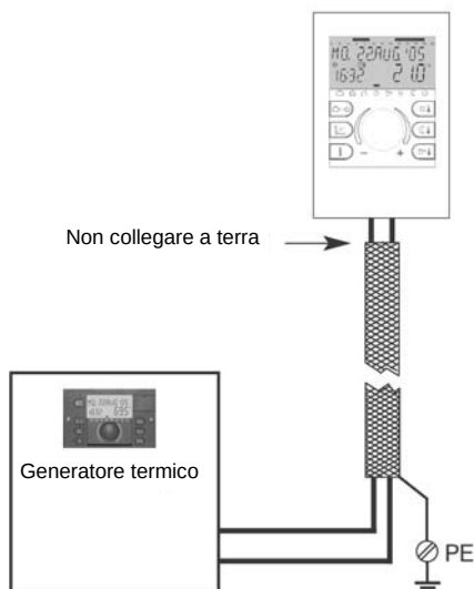
Fig. 4: Collegamento a terra della schermatura da un sola parte
