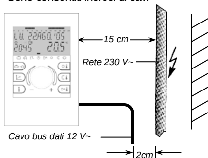
Fig. 1: Distanze minime per installazione elettrica
