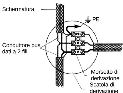
Fig. 5: Collegamento a terra bus dati a stella
