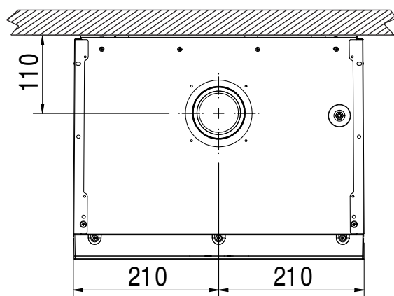
рис. 37- Вид сверху
