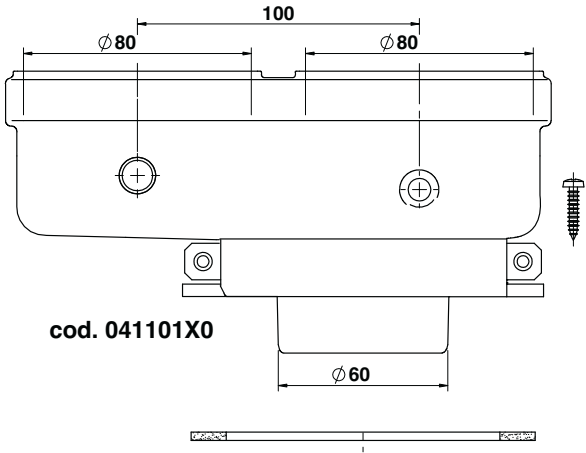
рис. 17- Исходная принадлежность для раздельных труб
