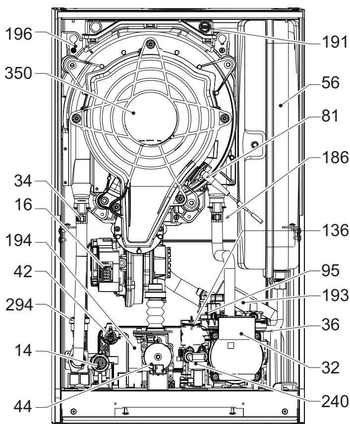
рис. 42- Общий вид
