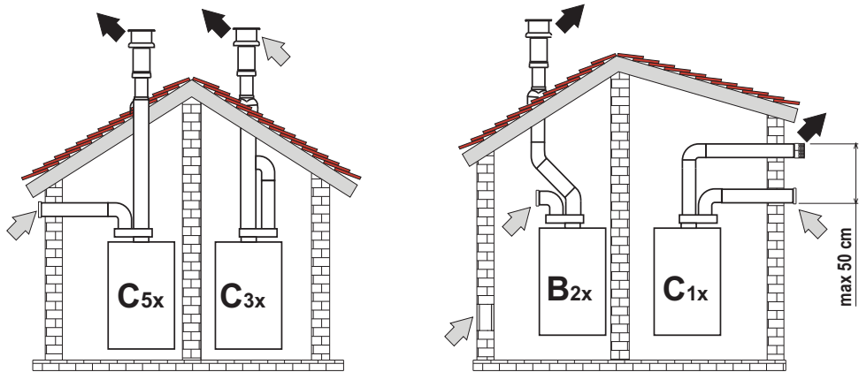
рис. 16- Примеры подсоединения с помощью раздельных труб (□ = Воздух/ ▣ = Дымовые газы)
