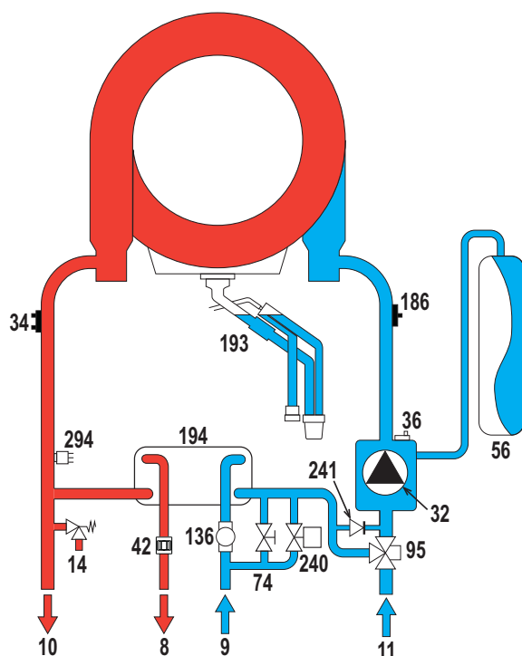
рис. 43- Гидравлический контур
