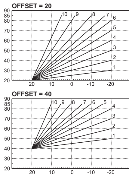
рис. 26- Пример параллельного смещения компенсационных кривых
