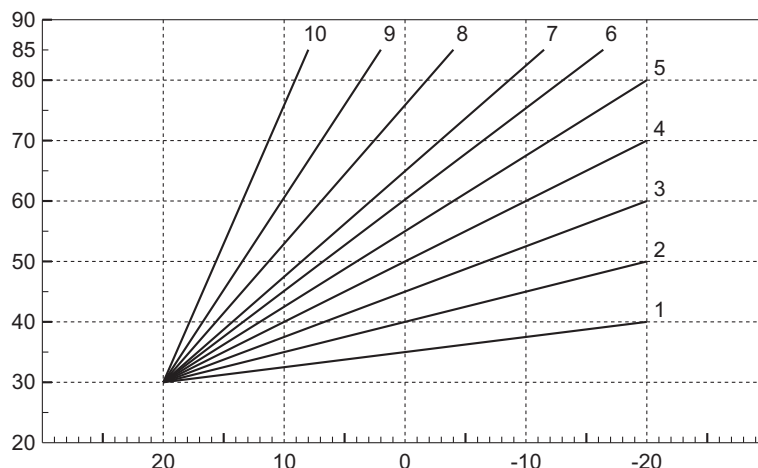
рис. 25- Компенсационные кривые
