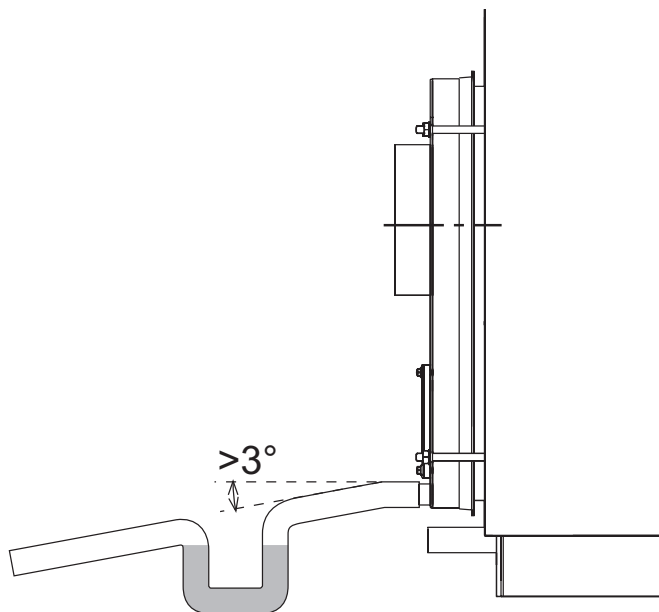
Fig. 8 - Condensate discharge
