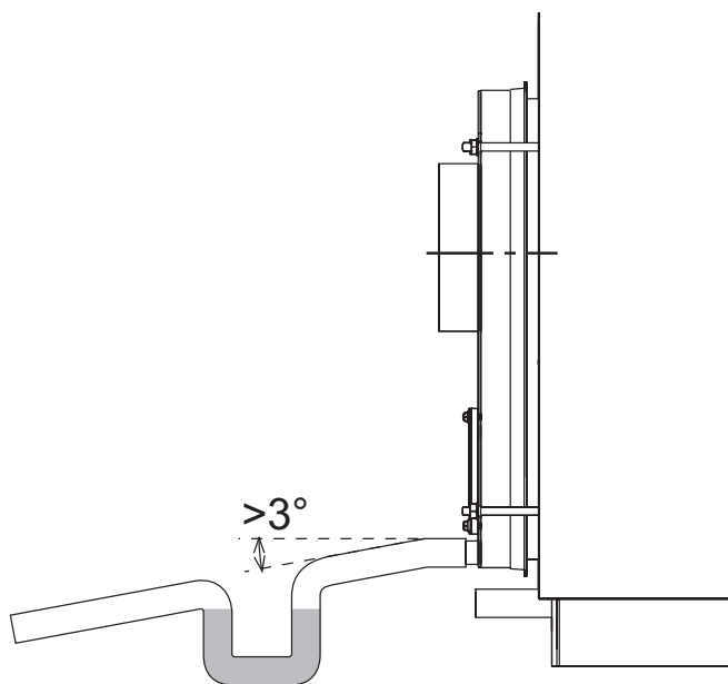
fig. 8 - Scarico condensa
