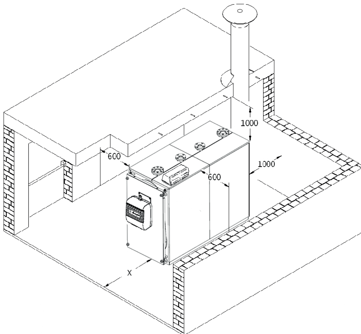
Fig. 6 - Local de instalación
