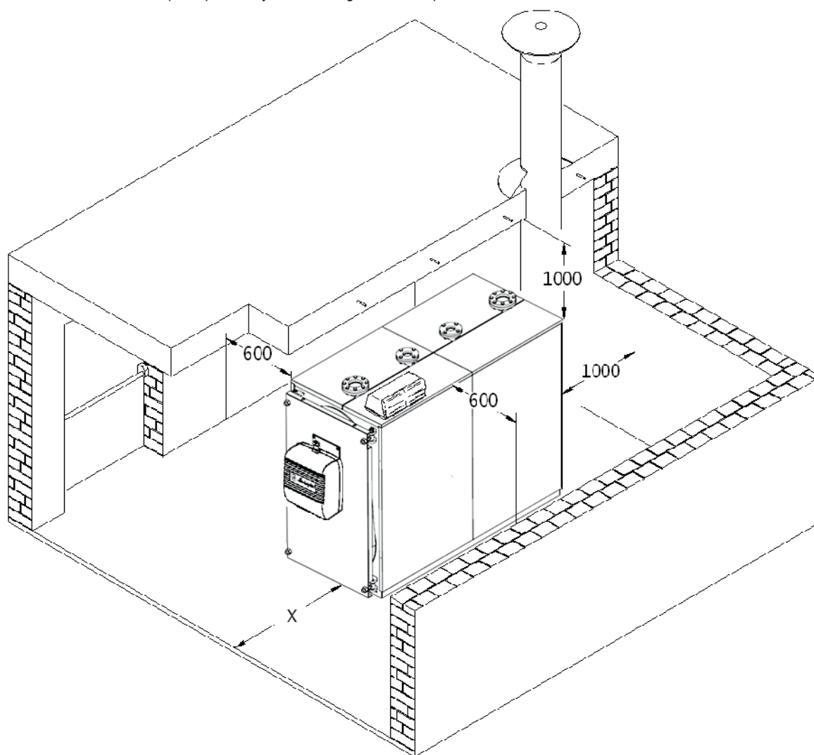
Fig. 6 - Local d'installation
