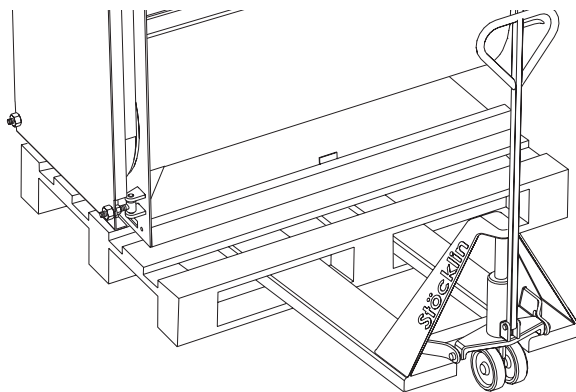
Fig. 5 - Emplazamiento
