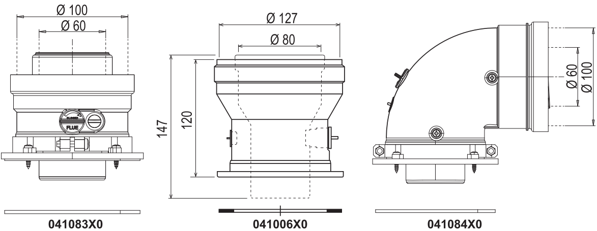
Рис. 21. Исходные принадлежности для коаксиальных воздухопроводов
