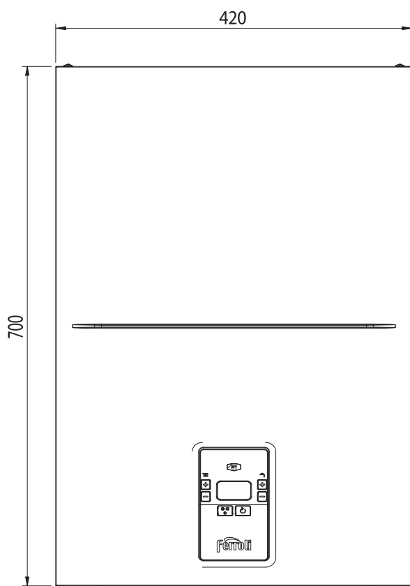
Рис. 36. Вид спереди
