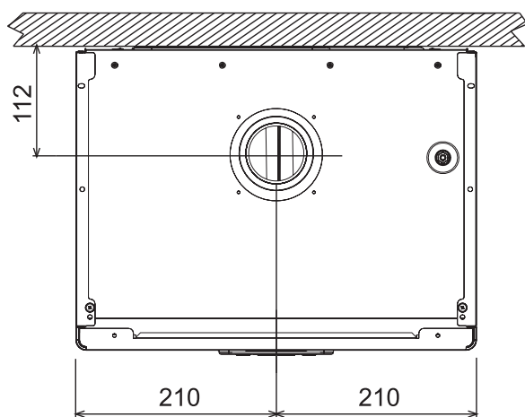
Рис. 38. Вид сверху
