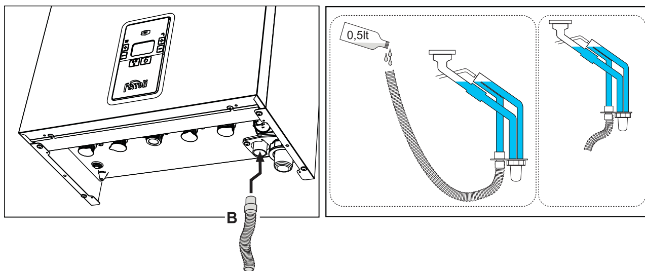
Рис. 28. Подсоединение трубы для слива конденсата
