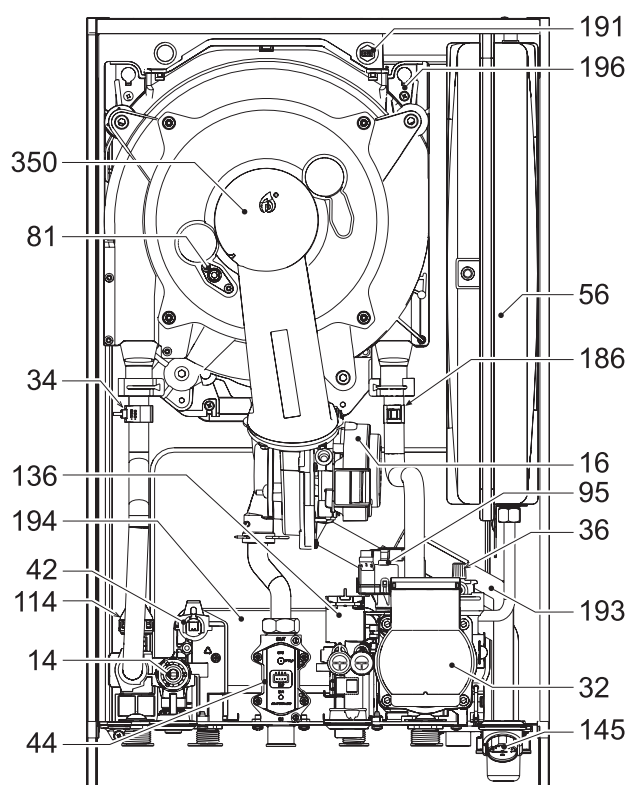
Рис. 40. Конструкция
