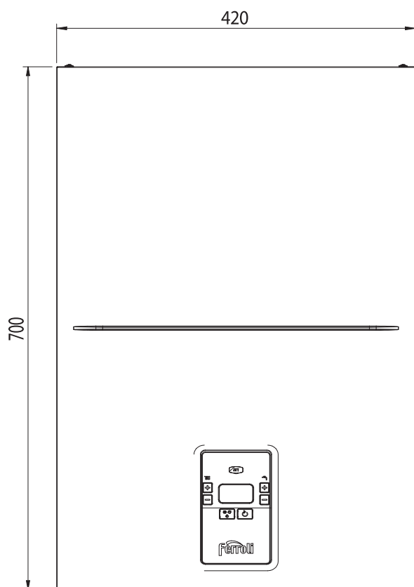
Рис. 32. Вид спереди
