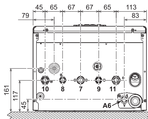
Рис. 37. Вид сбоку
