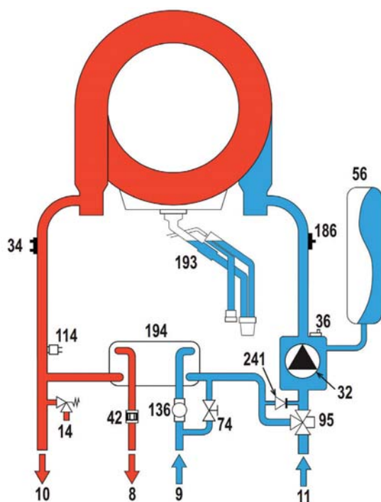
Рис. 41. Гидравлическая схема
