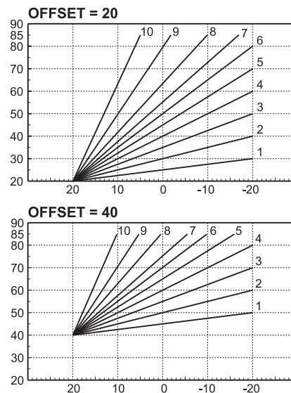
Рис. 15. Пример параллельного смещения компенсационных кривых
