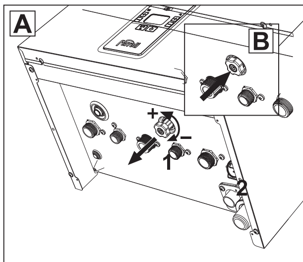
Рис. 16. Ручка заполнения системы
