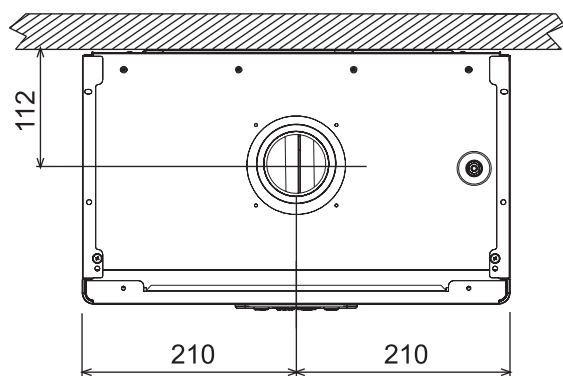
Рис. 34. Вид сверху
