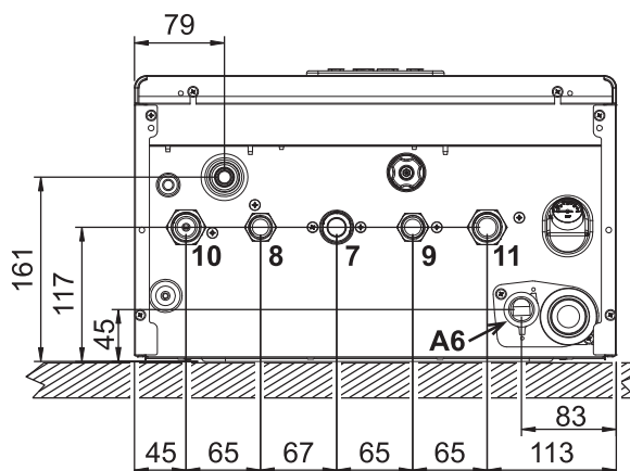
Рис. 35. Вид снизу
