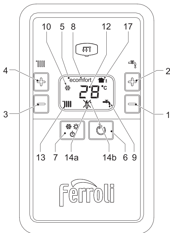
Рис. 1. Панель управления
