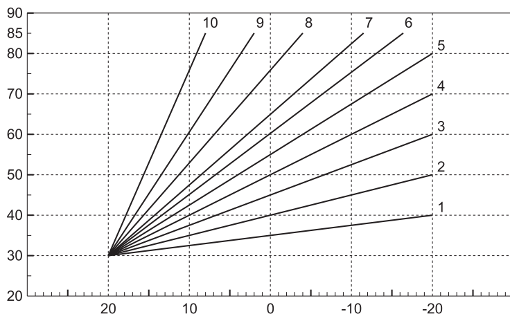
Рис. 14. Компенсационные кривые
