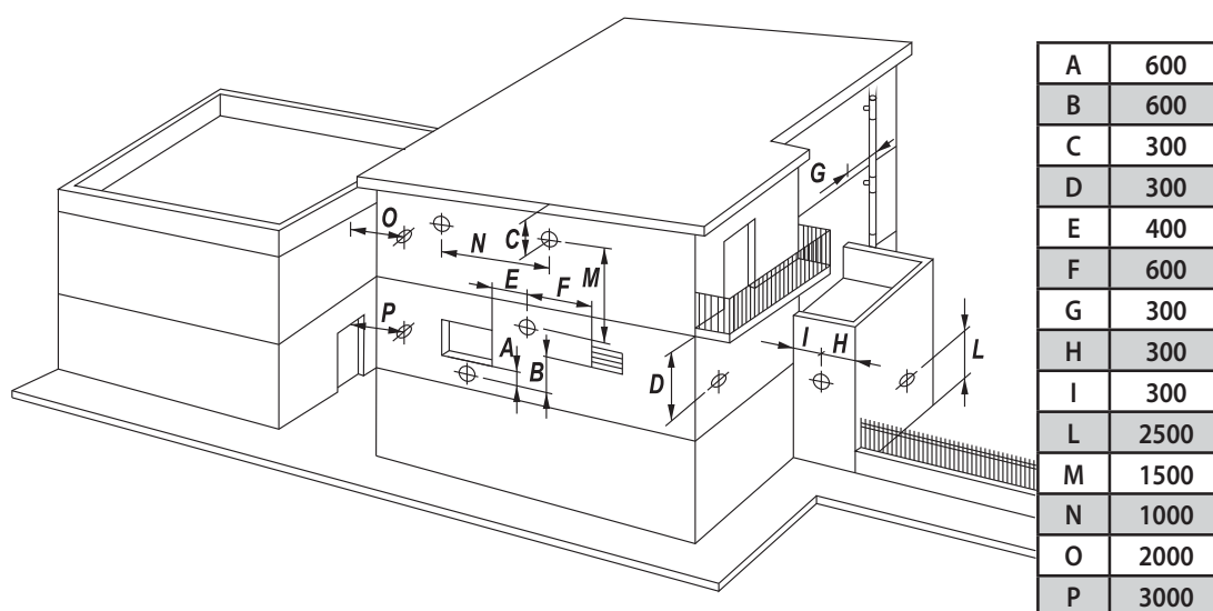
Варианты расположения оголовка дымохода
