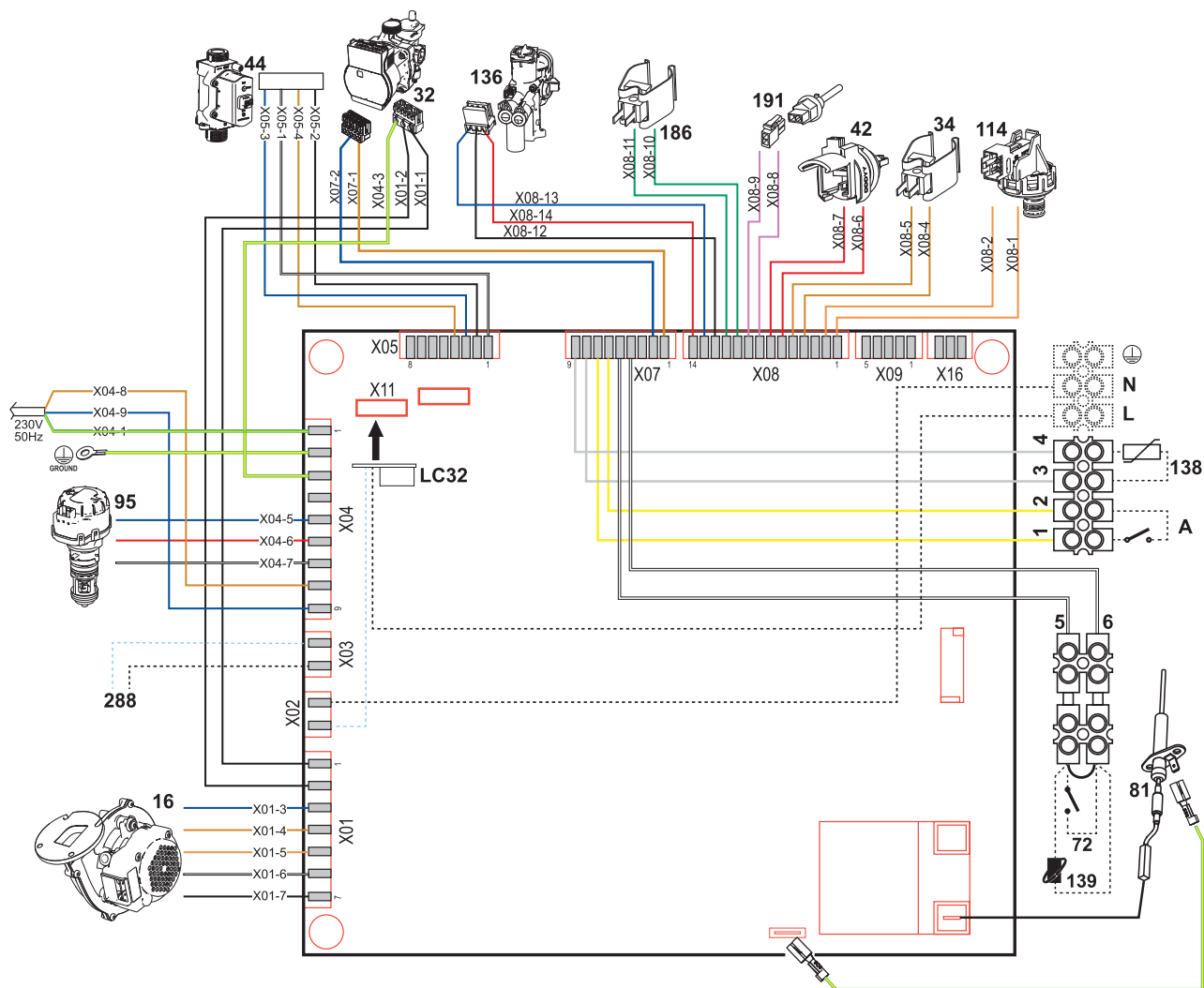
Рис. 45. Электрическая схема
