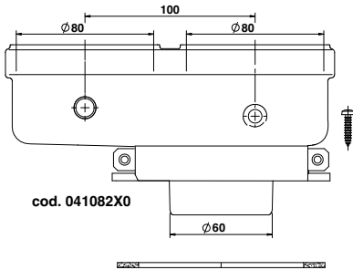
fig. 34- Accesoriu de pornire pentru conducte separate
