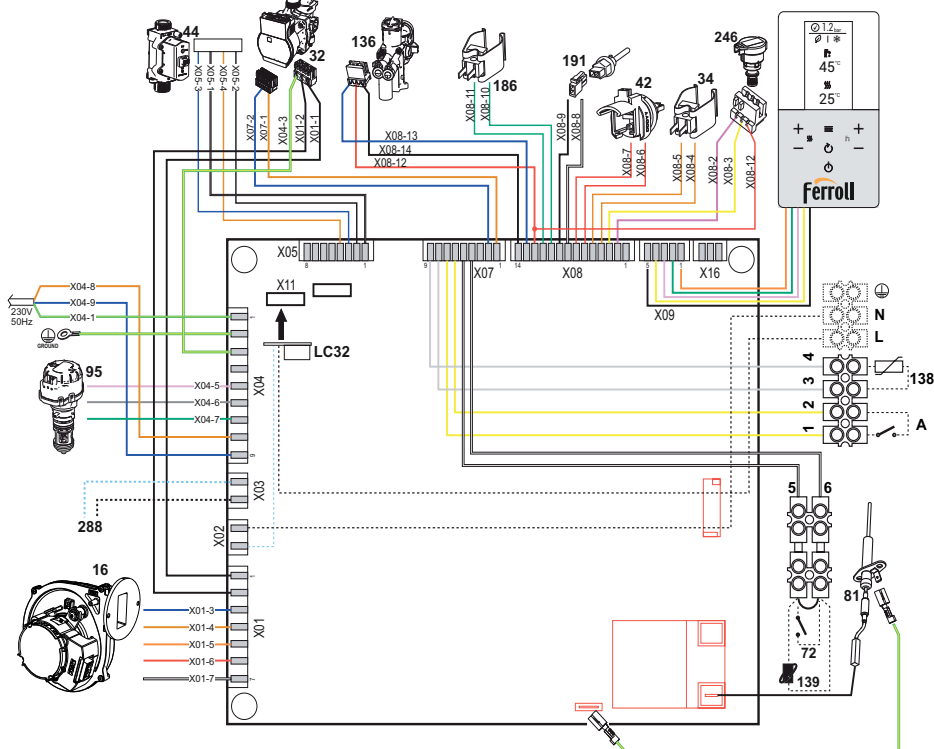
fig. 66- Schema electrică
