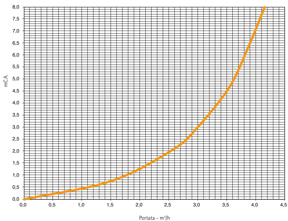
Diagrammi circolatori
