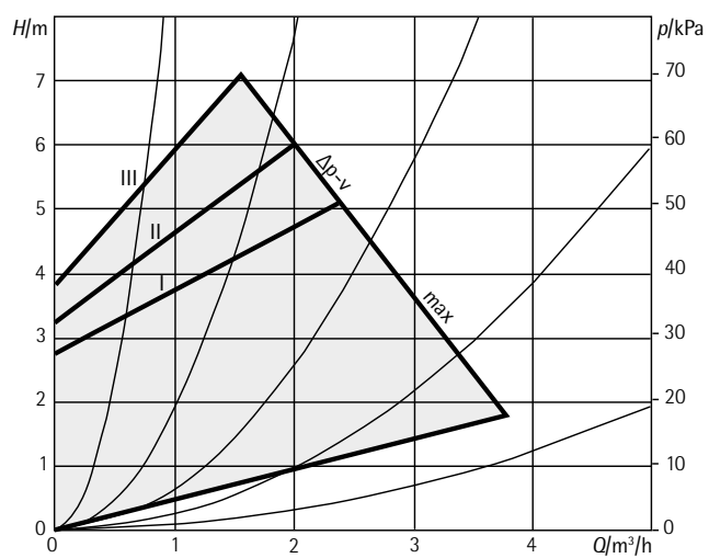
Diagrammi circolatori
