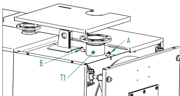
Fig. 13 - Fourreau des sondes et des bulbes
