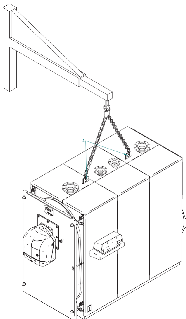
Fig. 3 - Emplazamiento
