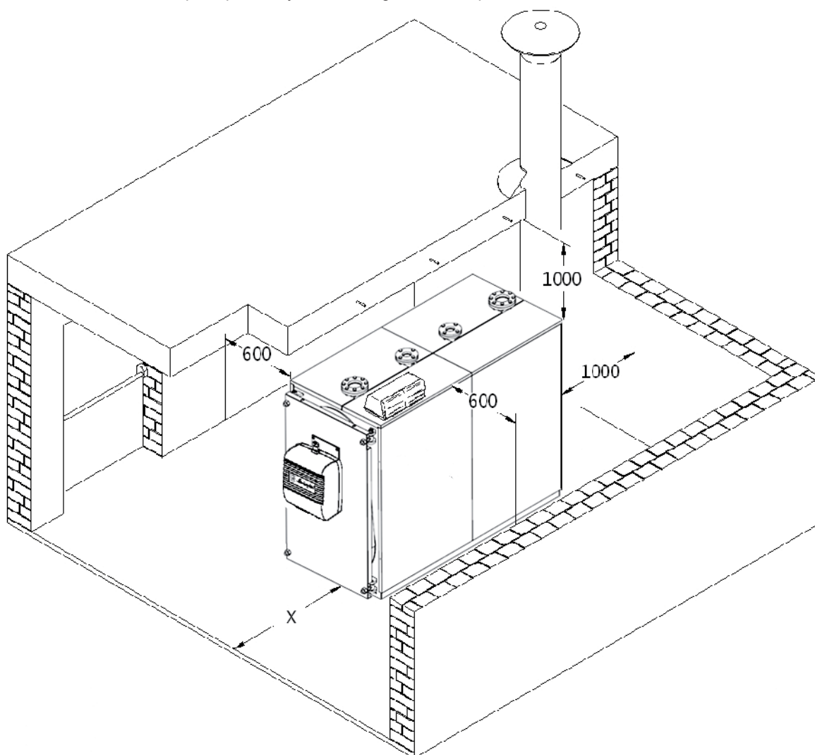
Fig. 4 - Local d'installation
