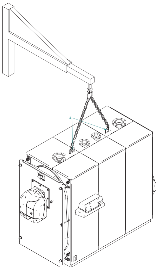
fig. 3 - Posizionamento
