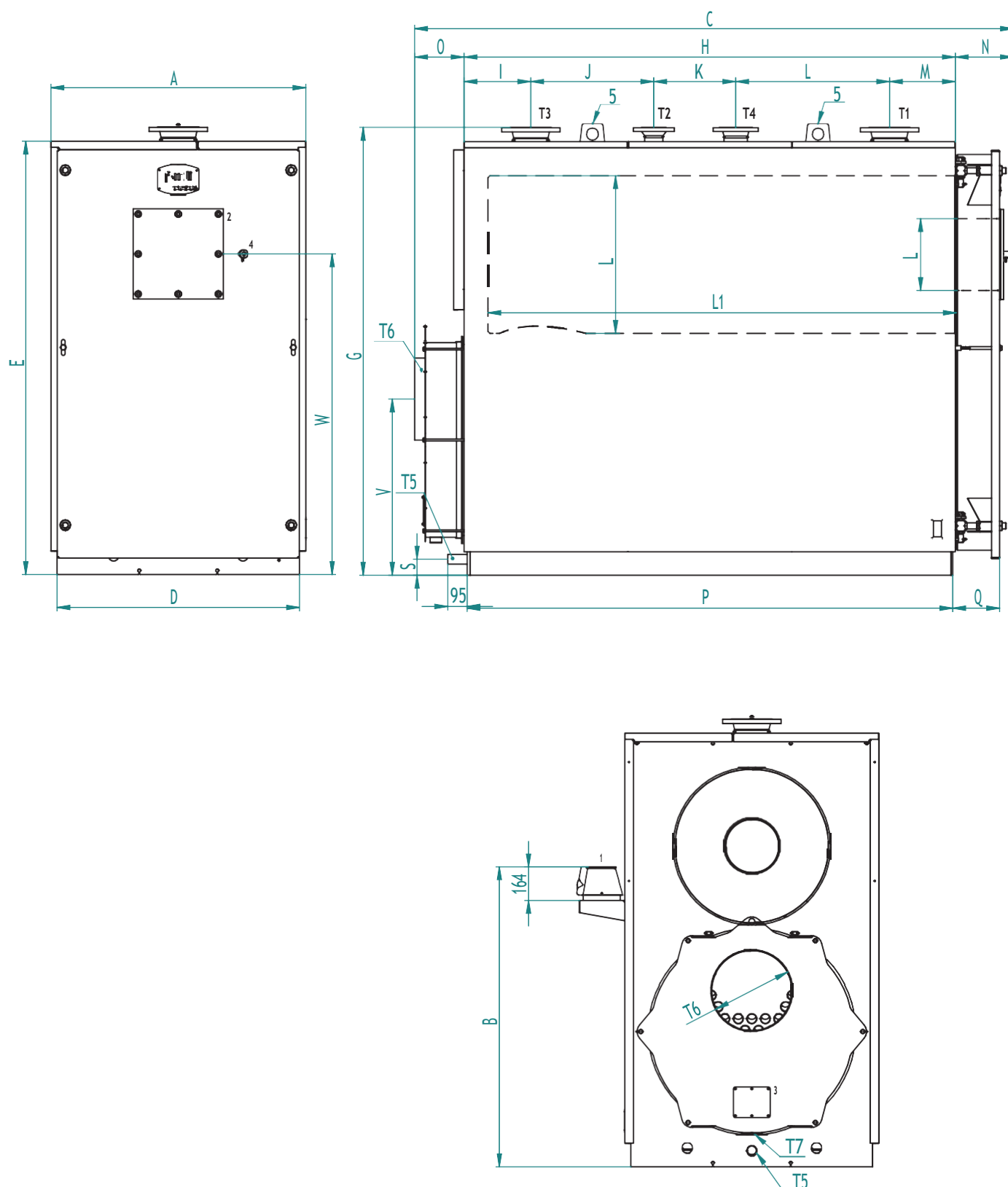
Fig. 2 - Dimensions et raccords
