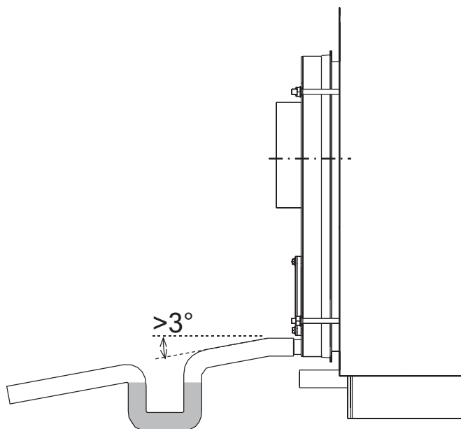
fig. 6 - Scarico condensa
