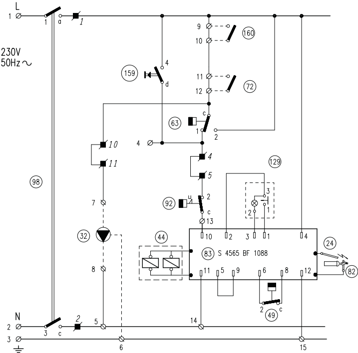
мал. 89 - Принципова електрична схема
