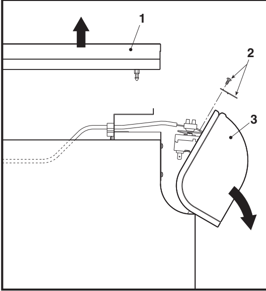
şek. 32 - Panelin açılması
