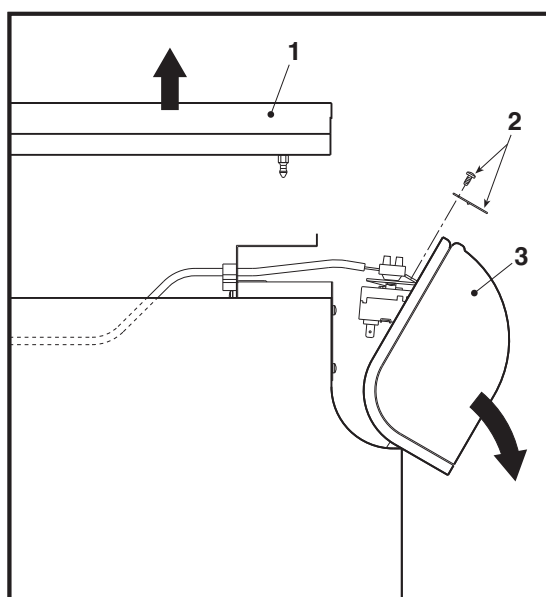
fig. 2 - Apertura cruscotto
