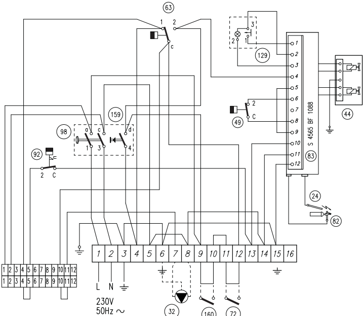
fig. 75 - Schéma électrique de raccordement
