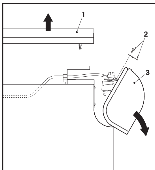
fig. 62 - Ouverture panneau de commande
