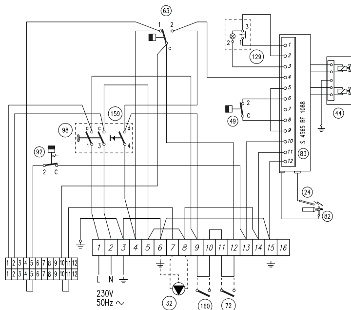
рис. 105 - Схема электрических соединений
