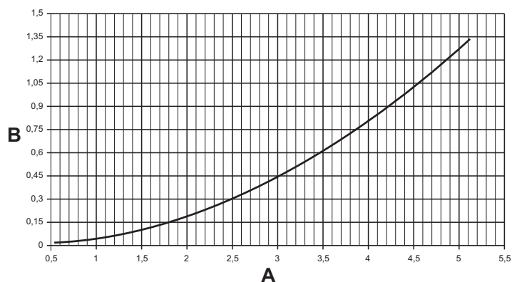
fig. 28 - Diagrama de pérdida de carga
