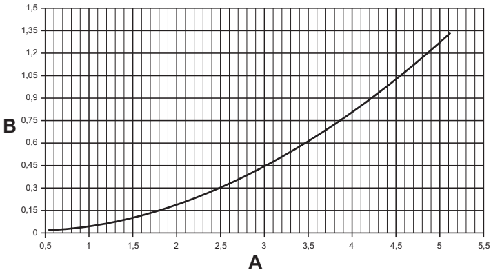
fig. 13 - Diagramma perdite di carico
