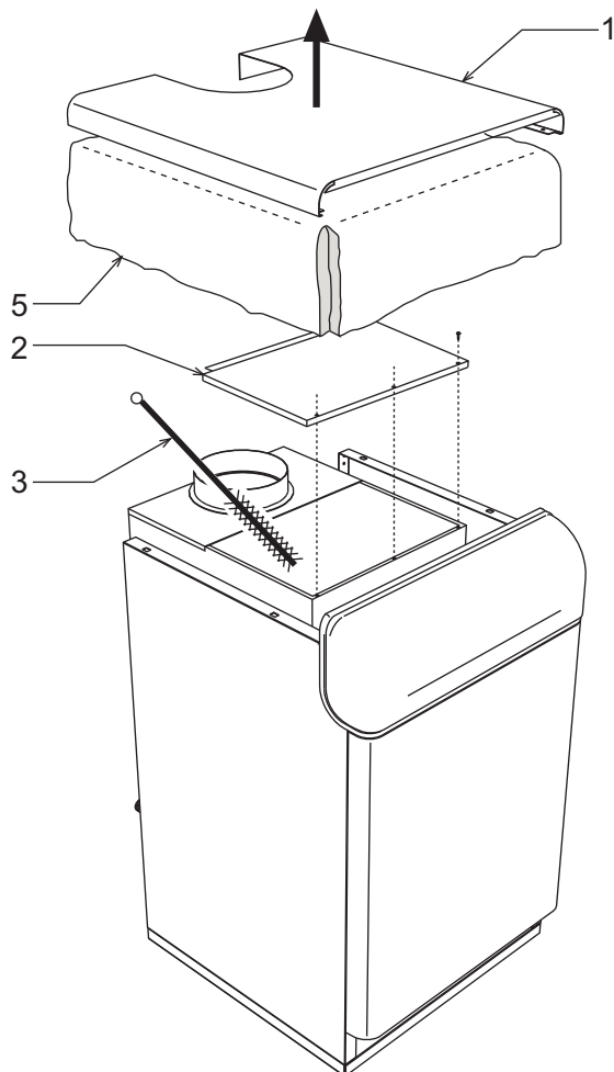
fig. 20 - Limpieza de la caldera
