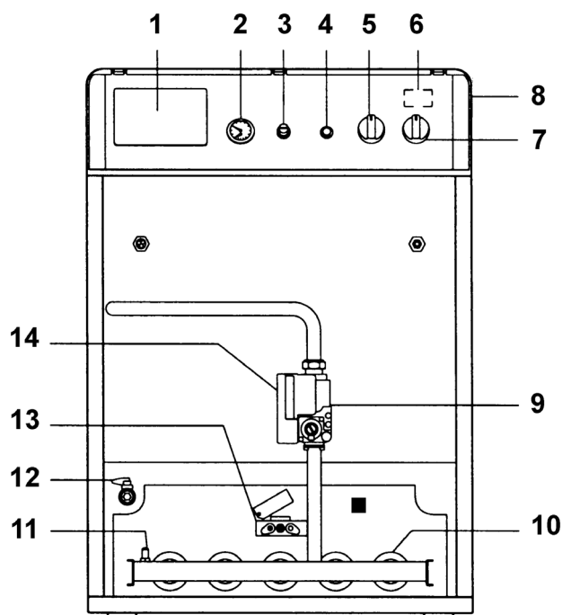
мал. 87 - Загальний вигляд
