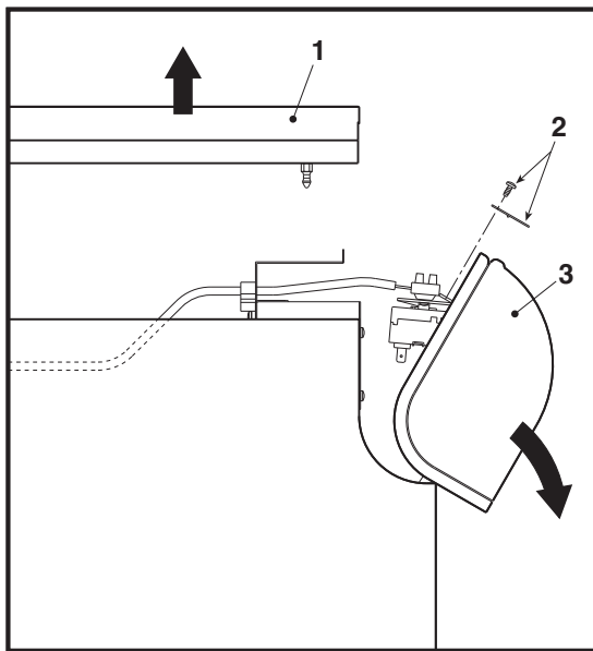
мал. 77 - Відкриття панелі приборів
