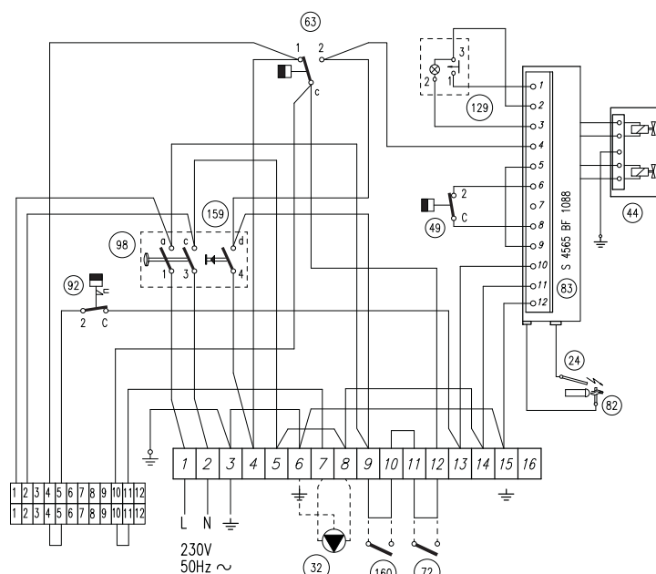
fig. 30 - Esquema eléctrico de conexión
