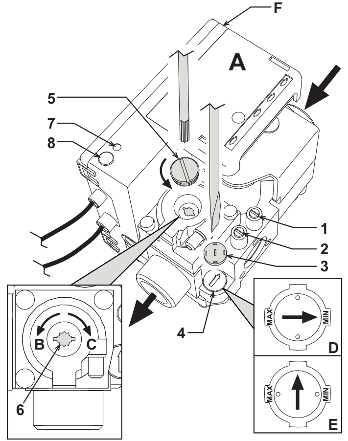
şek. 33 - Basıncın ayarlanması
