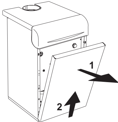
мал. 79 - Відкриття передньої панелі
