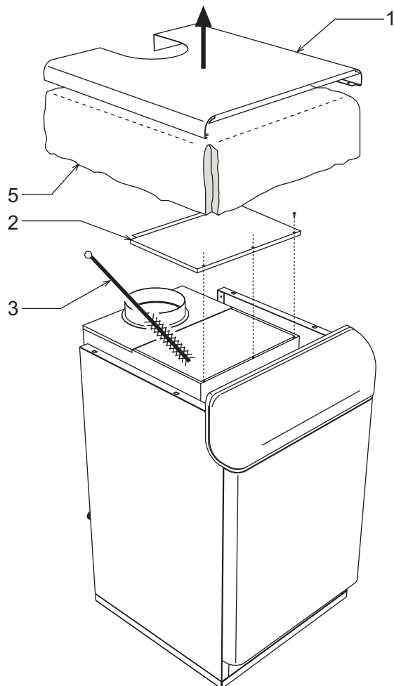
рис. 95 - Очистка котла
