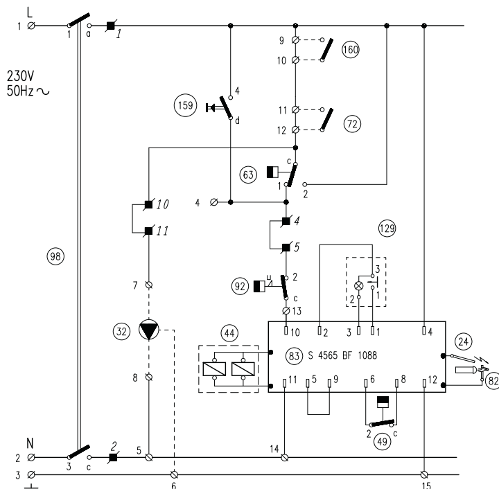
fig. 29 - Esquema eléctrico general
