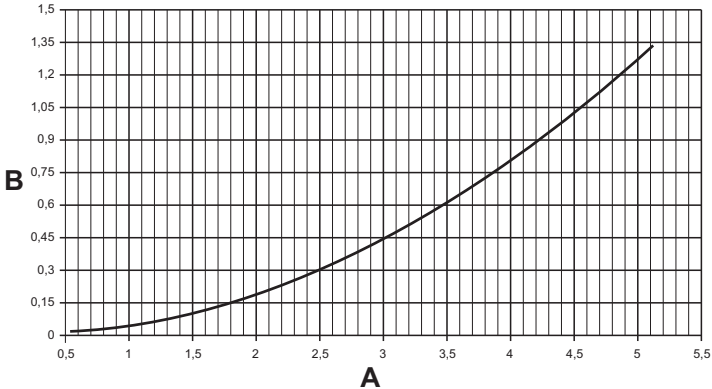
мал. 88 - Діаграма втрат напору
