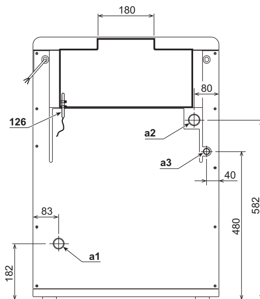
мал. 86 - Вид ззаду
