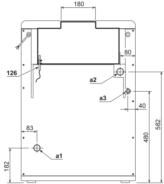
şek. 41 - Arkadan görünüm
