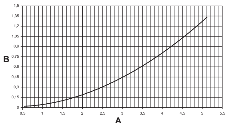
рис. 103 - Диаграмма потери напора
