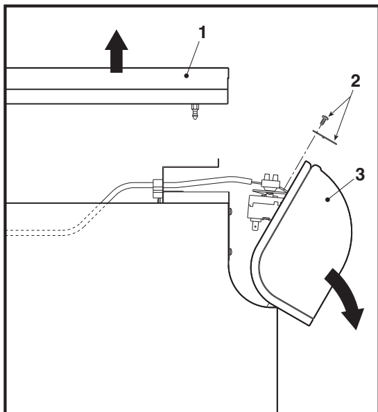
fig. 17 - Apertura del panel de mandos
