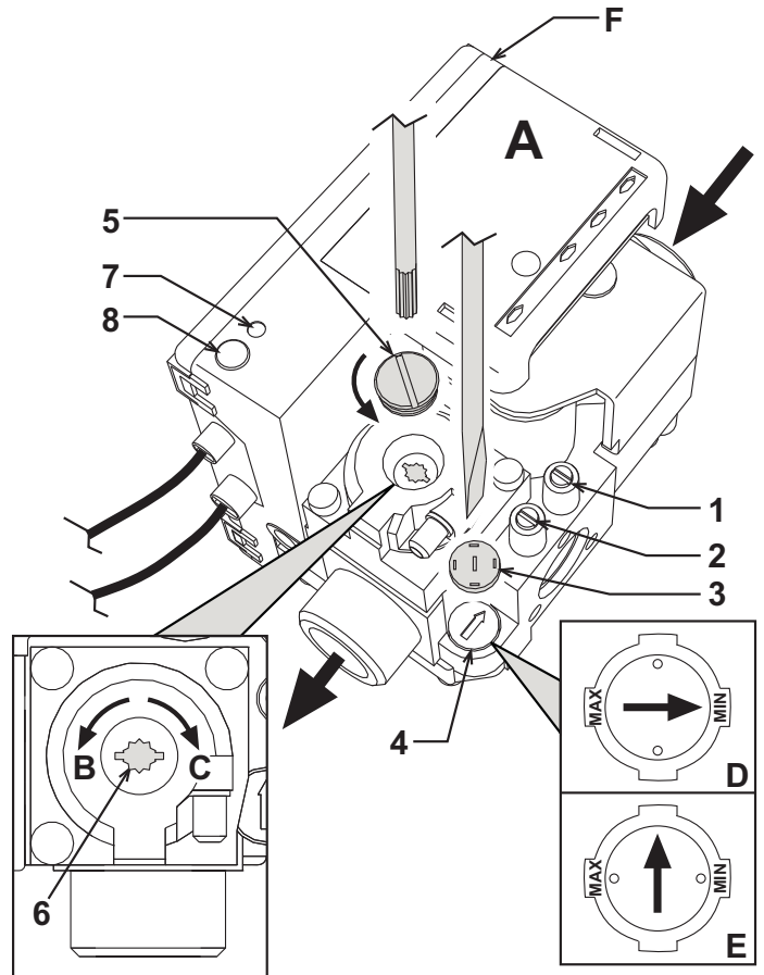
мал. 78 - Регулювання тиску
