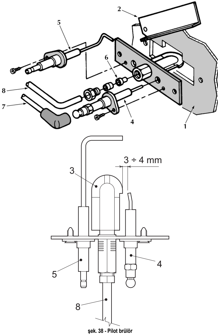
şek. 38 - Pilot brülör
