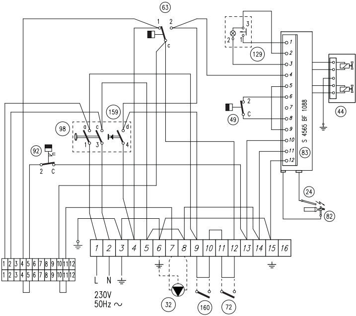
мал. 90 - Принципова електрична схема
