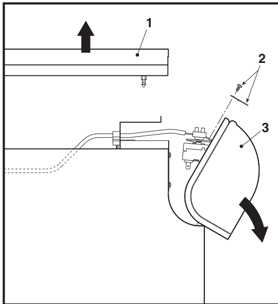
рис. 92 - Открытие панели управления
