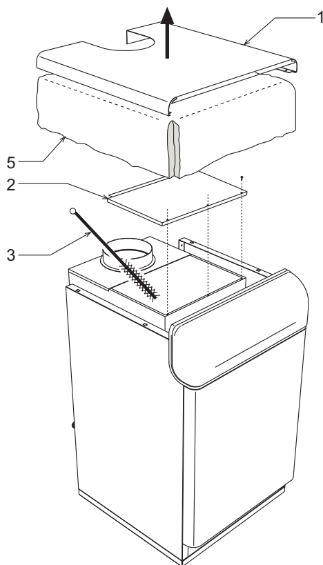
fig. 65 - Nettoyage de la chaudière
