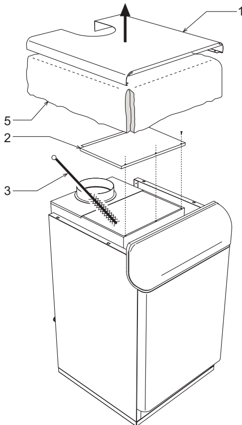
мал. 80 - Очищення котла
