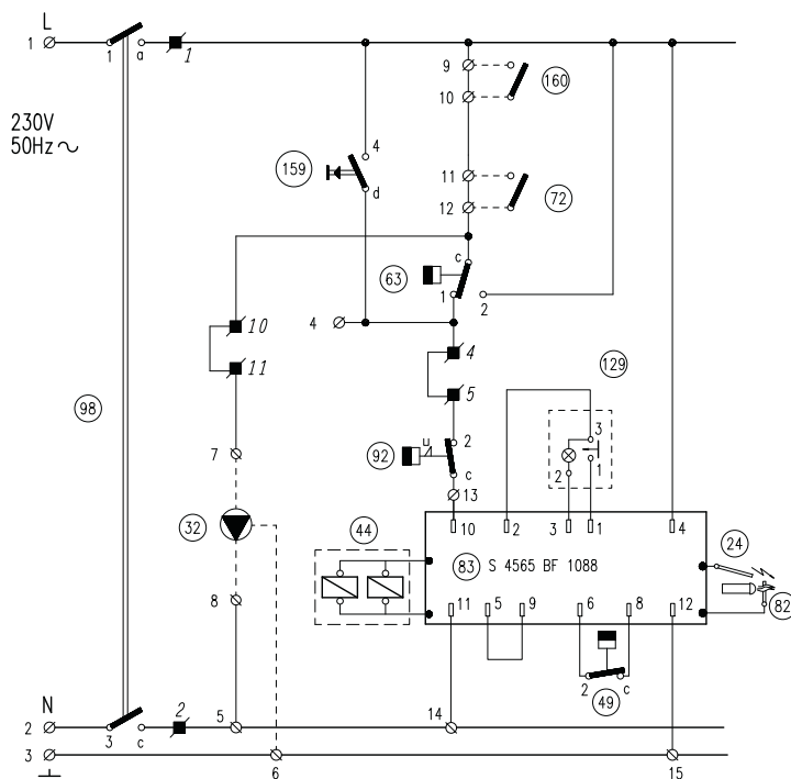
рис. 104 - Принципиальная электрическая схема
