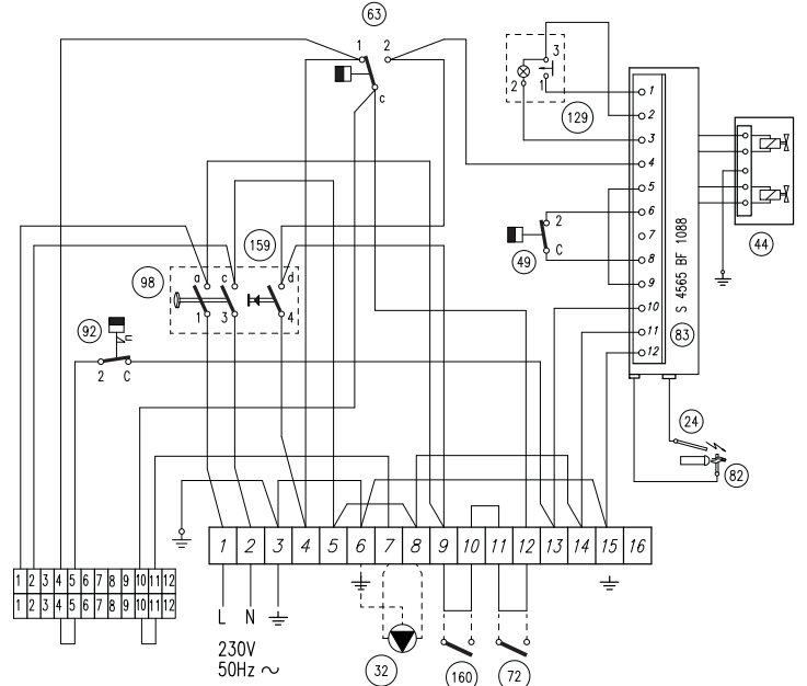
şek. 45 - Elektrik bağlantı şeması
