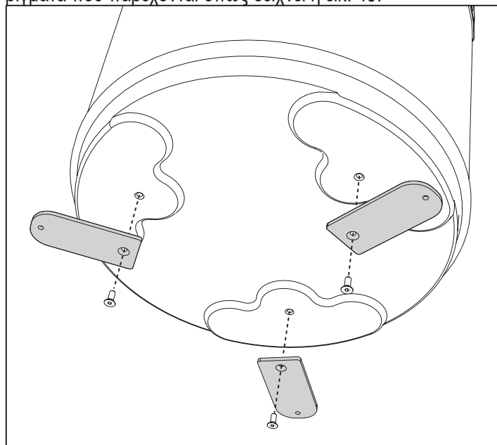
εικ. 49- Στερέωση των βραχιόνων
