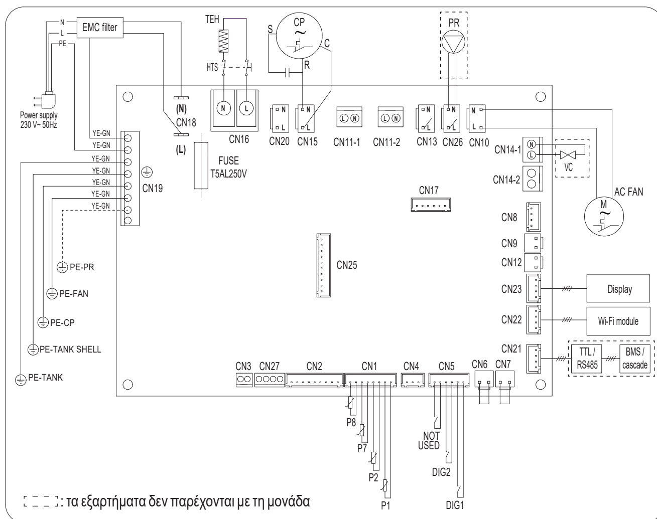
εικ. 68 - Ηλεκτρικό σχεδιάγραμμα του εξοπλισμού
