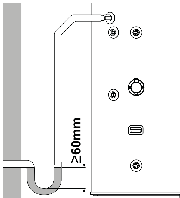
εικ. 63- Παραδείγματα σύνδεσης εκφόρτωσης συμπύκνωσης μέσα από έναν θερμοθάλαμο διακοπής
