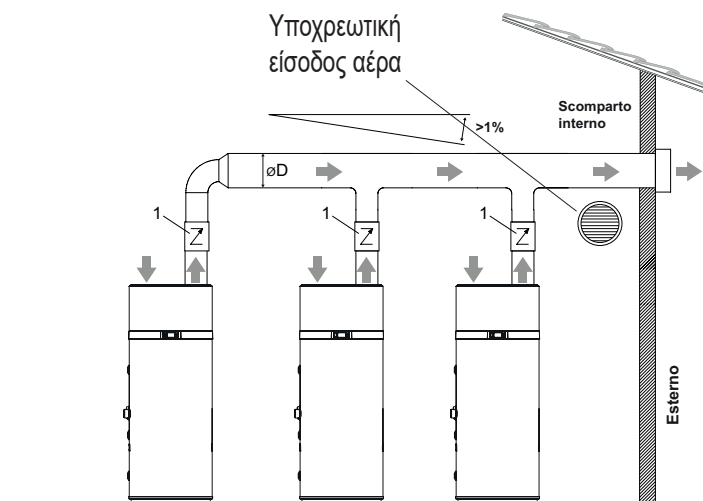
εικ. 53 - Παράδειγμα σύνδεσης εκκένωσης αέρα
