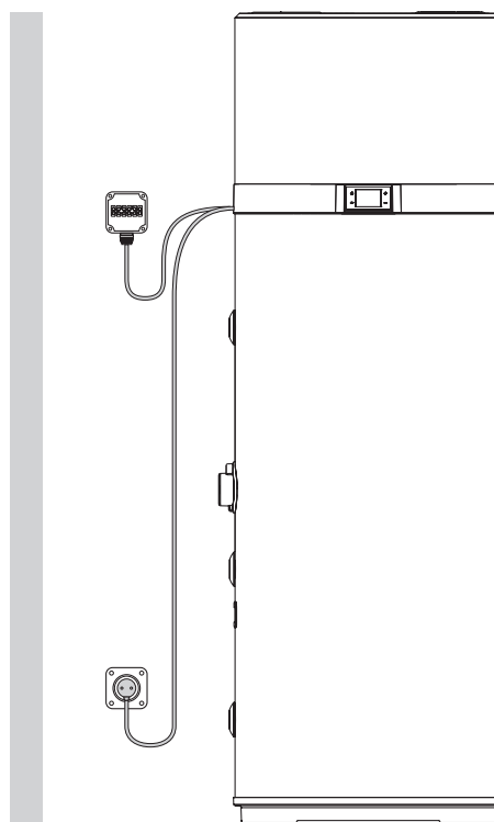
εικ. 66- Παράδειγμα απομακρυσμένης σύνδεσης
