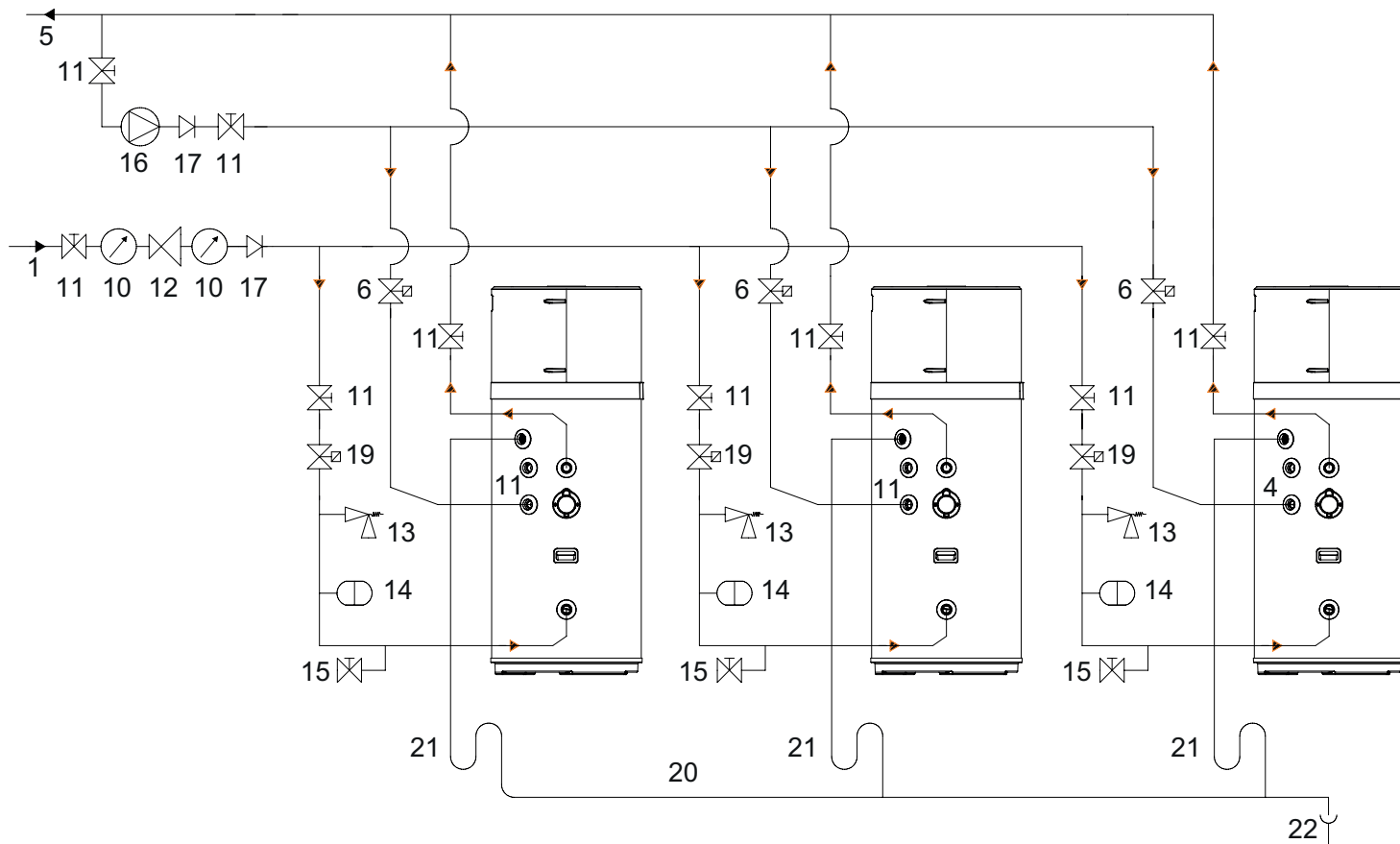
εικ. 60 - Παράδειγμα εγκατάστασης ύδρευσης ΧΩΡΙΣ θερμοστατική βαλβίδα μίξης
