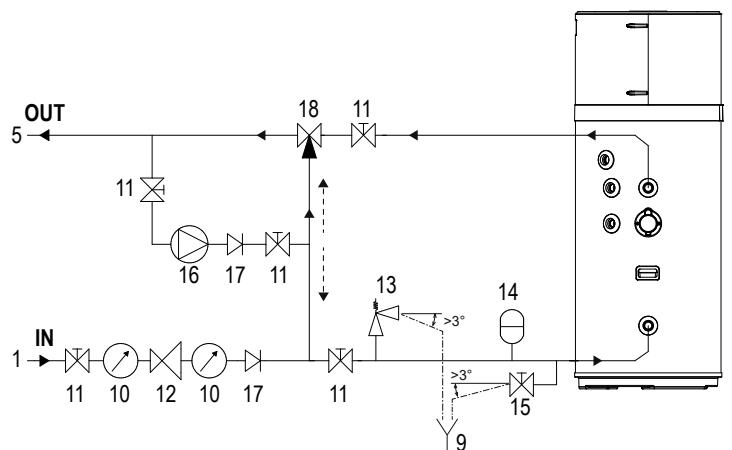
ΕΙΚ. 58 - Παράδειγμα εγκατάστασης νερού ΜΕ θερμοστατική βαλβίδα μίξης
