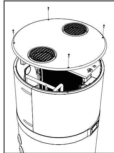
ΕΙΚ. 72- Αφαίρεση του άνω καπακιού
