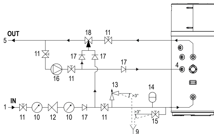
εικ. 59 - Παράδειγμα εγκατάστασης νερού ME θερμοστατική βαλβίδα μίξης
