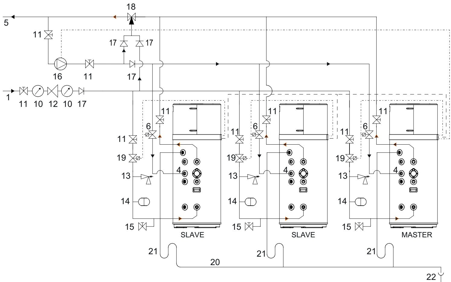
εικ. 62 - Παράδειγμα εγκατάστασης νερού ME θερμοστατική βαλβίδα μίξης (επανακυκλοφορία σε σύνδεση επανακυκλοφορίας νερού μονάδας)
