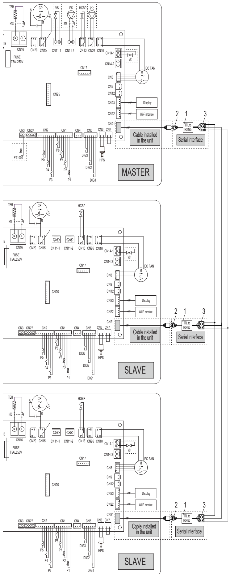
εικ. 70 - Διάγραμμα καλωδίωσης σε σειρά
