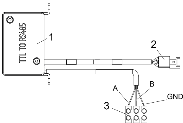
εικ. 69 - Kit σειριακής διεπαφής TTL-RS485
