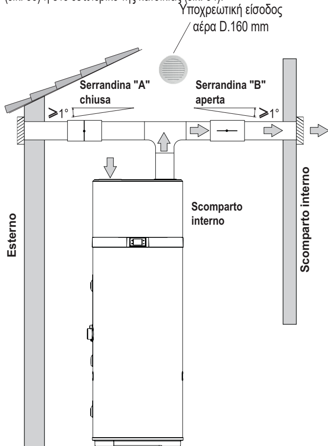
εικ. 54- Παράδειγμα εγκατάστασης κατά τη θερινή περίοδο
