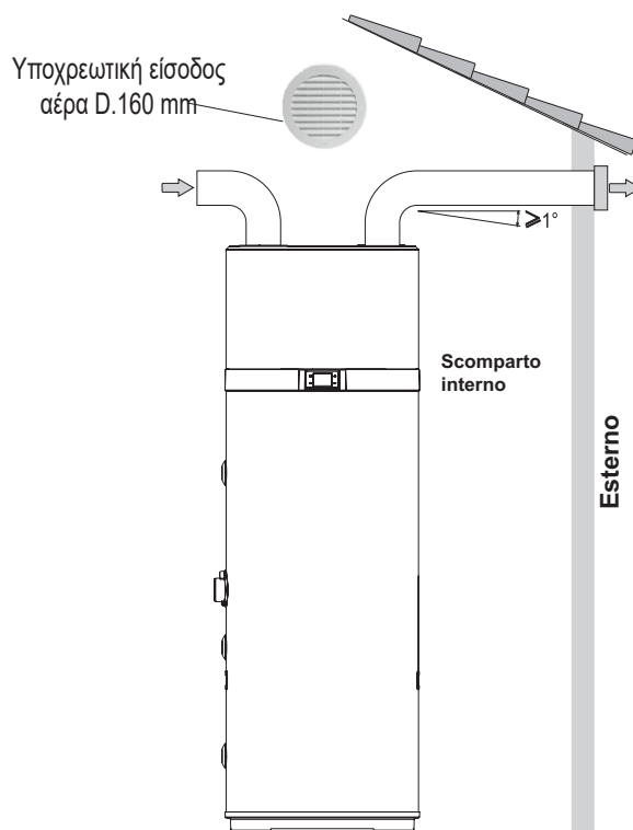
εικ. 52 - Παράδειγμα σύνδεσης εκκένωσης αέρα
