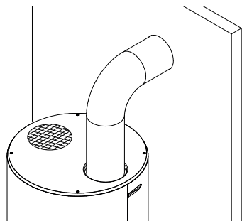
εικ. 51- Διάταξη καναλιών αέρα
