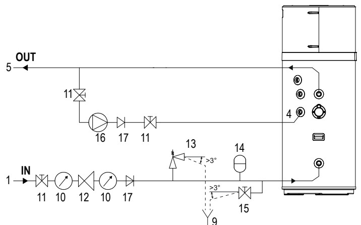
ΕΙΚ. 57 - Παράδειγμα εγκατάστασης ύδρευσης ΧΩΡΙΣ θερμοστατική βαλβίδα μίξης
