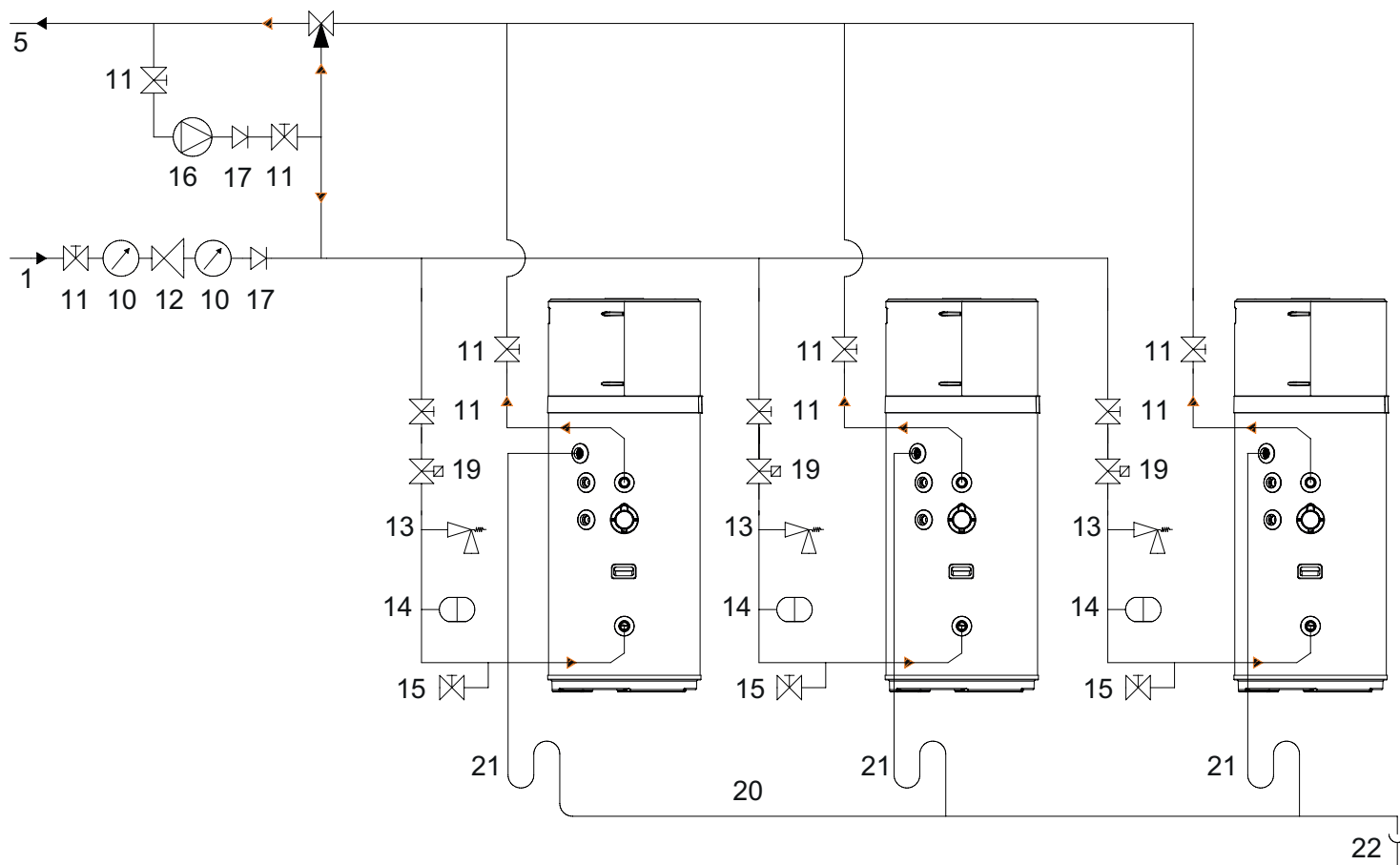
εικ. 61 - Παράδειγμα εγκατάστασης νερού ΜΕ θερμοστατική βαλβίδα μίξης (επανακυκλοφορία σε σύνδεση εισόδου κρύου νερού μονάδας)
