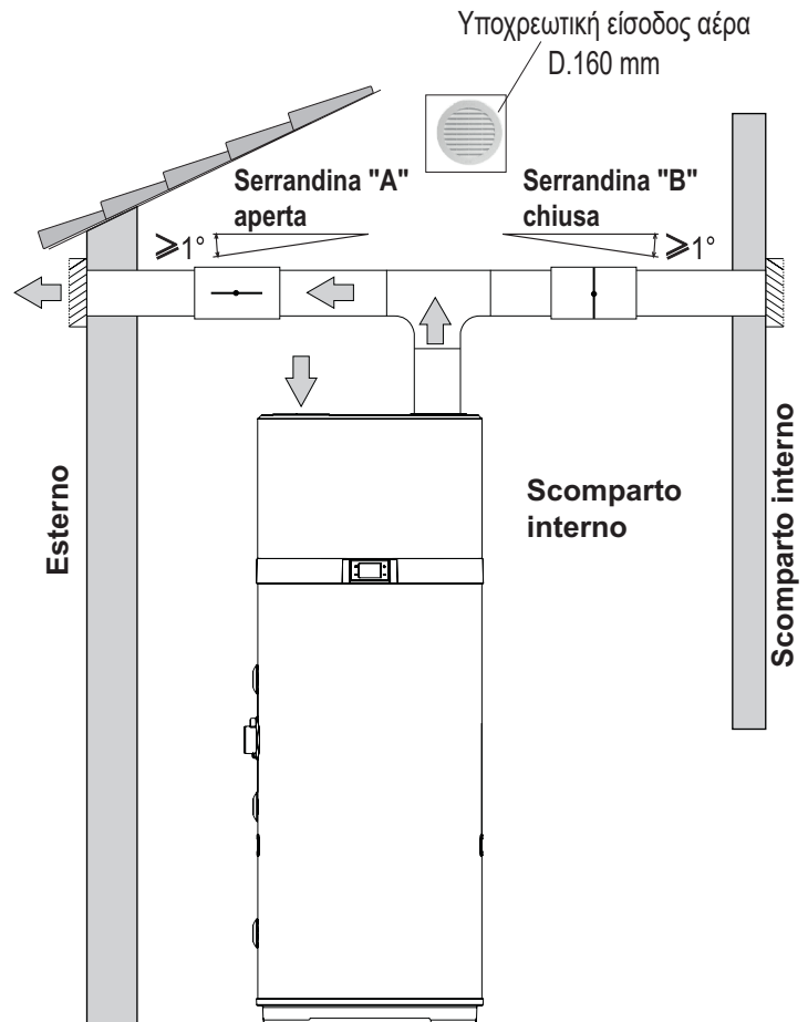
εικ. 55- Παράδειγμα εγκατάστασης κατά τη χειμερινή περίοδο
