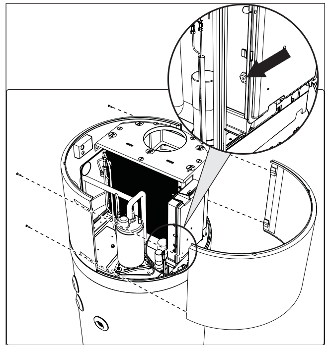
ΕΙΚ. 73- Αφαίρεση του εμπρός πάνελ
