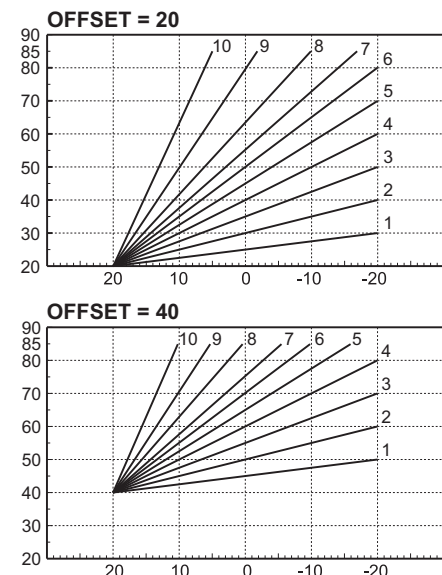
мал. 25- Пиклад паралельного пересування компенсаційних кривих
