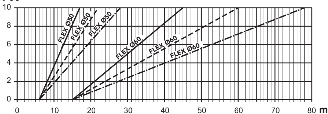
мал. 40- Графік для вибору параметра димоходу
