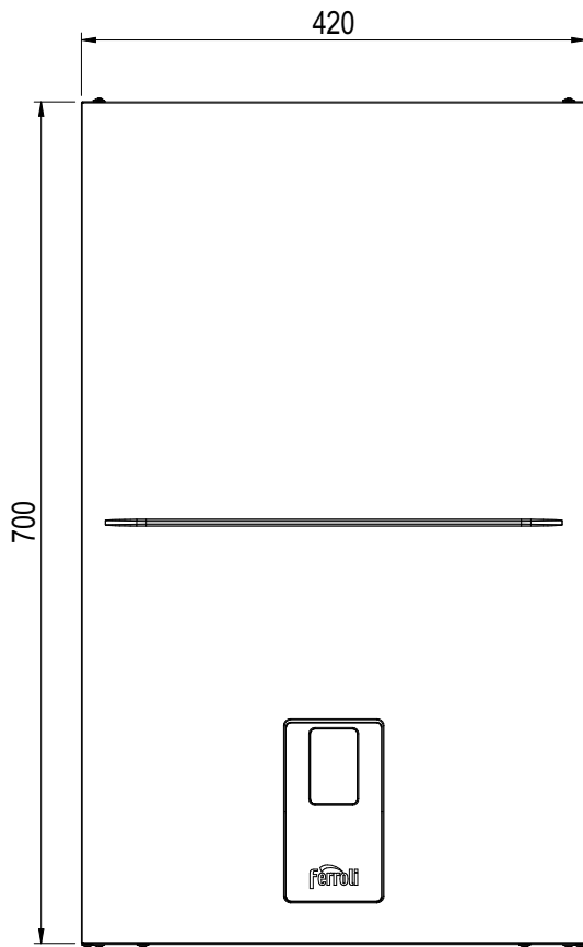
мал. 73- Вигляд спереду
