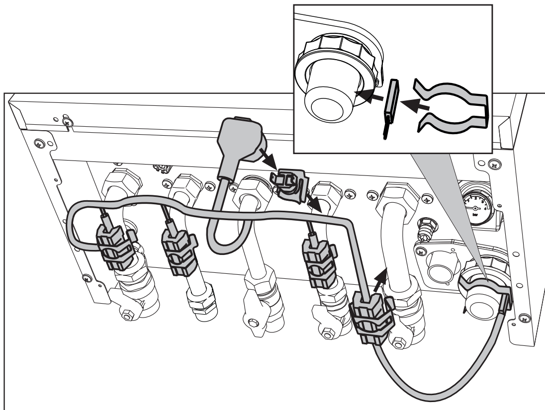
мал. 49- Комплект для захисту від замерзання
