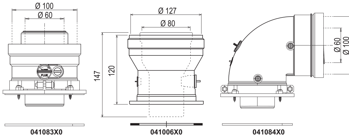
мал. 32- Початкові елементи для коаксiальних трубопроводiв
