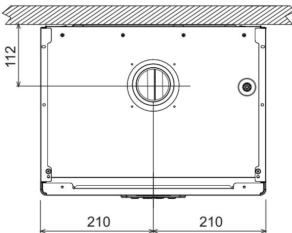
мал. 75- Вигляд зверху
