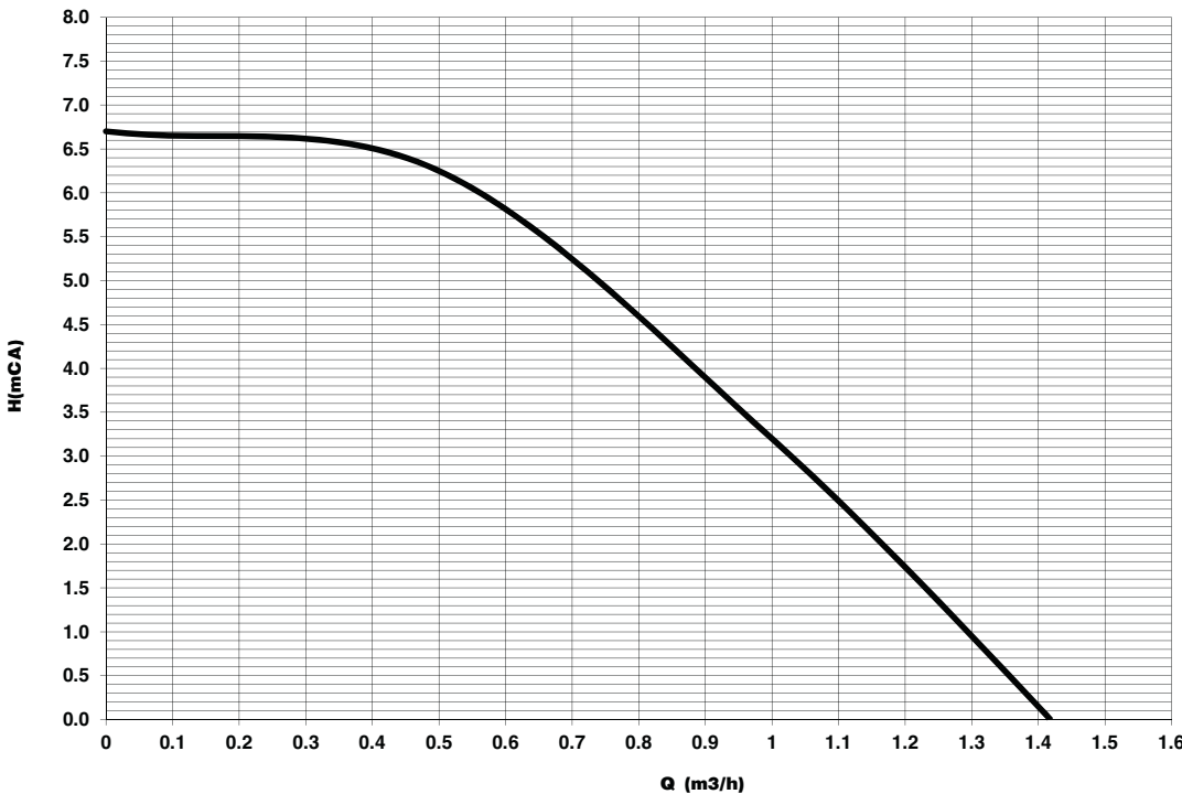
мал. 79- Залишковий напір, що досягається в системі
