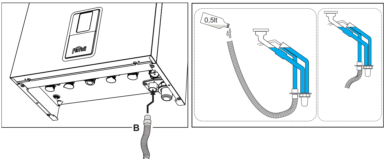
мал. 52- Підключення зливу конденсату
