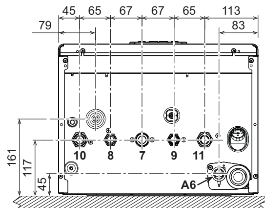
мал. 76- Вигляд знизу
