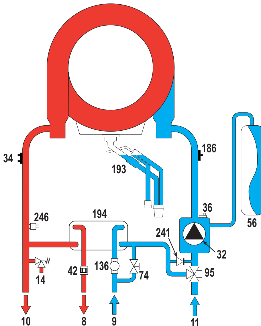
мал. 78- Гідравлічний контур
