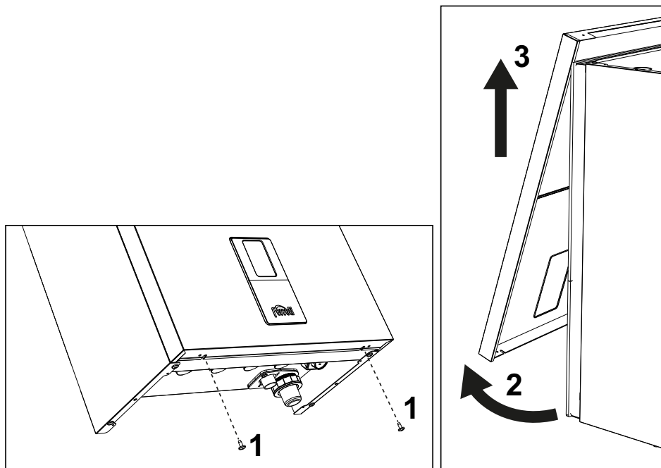
мал. 56- Відкриття передньої панелі
