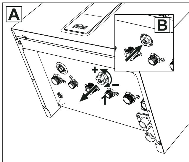
мал. 26- Ручка для заправлення
