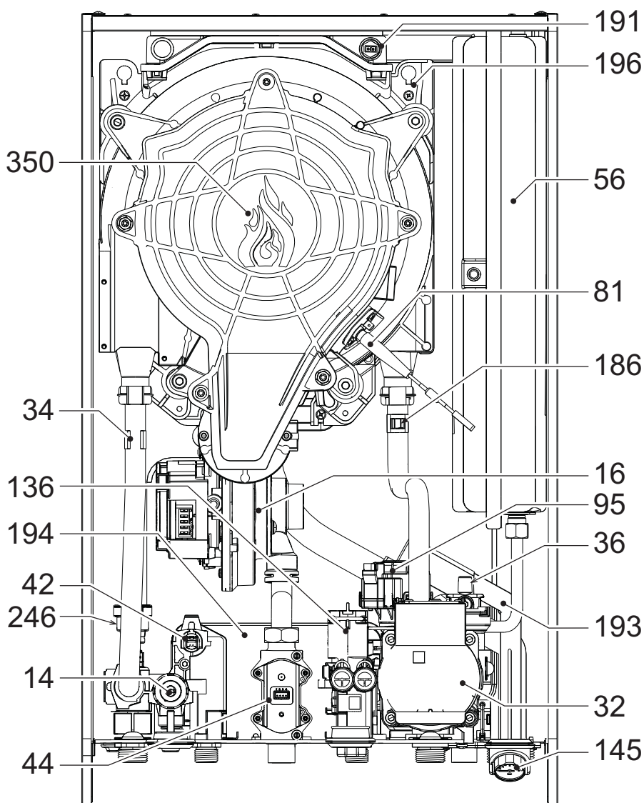
мал. 77- Загальний вигляд
