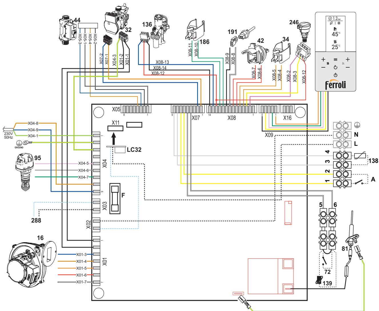
мал. 81- Електрична схема
