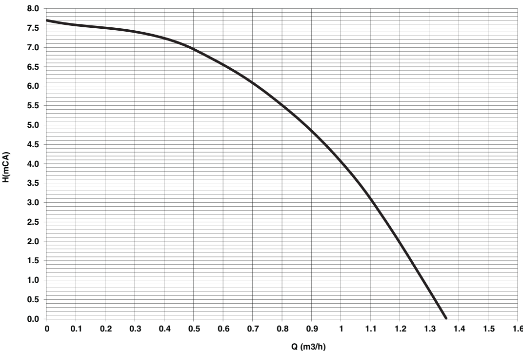
мал. 80- Залишковий напір, що досягається в системі
