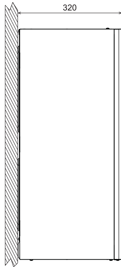
мал. 74- Вигляд збоку
