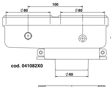
мал. 36- Початковий елемент для відокремлених труб
