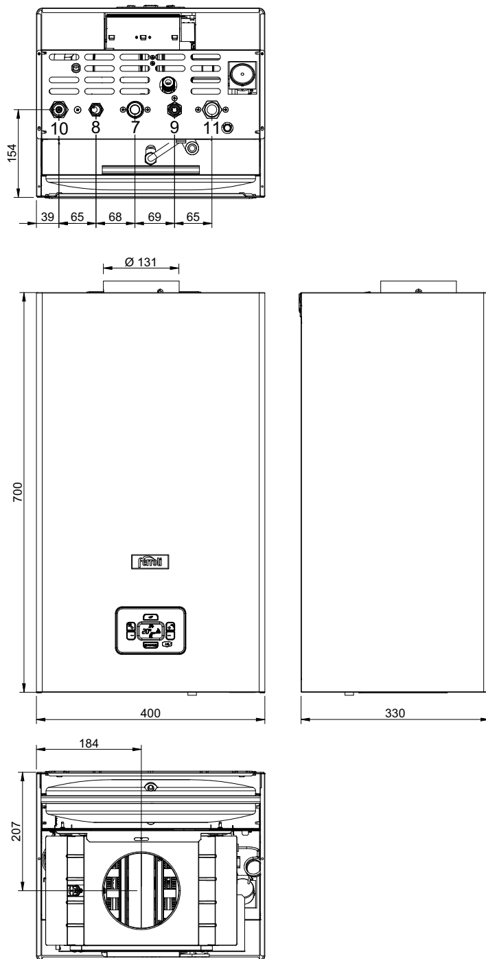
мал. 15- Розміри та під'єднувальні розміри моделі DIVA D C24
