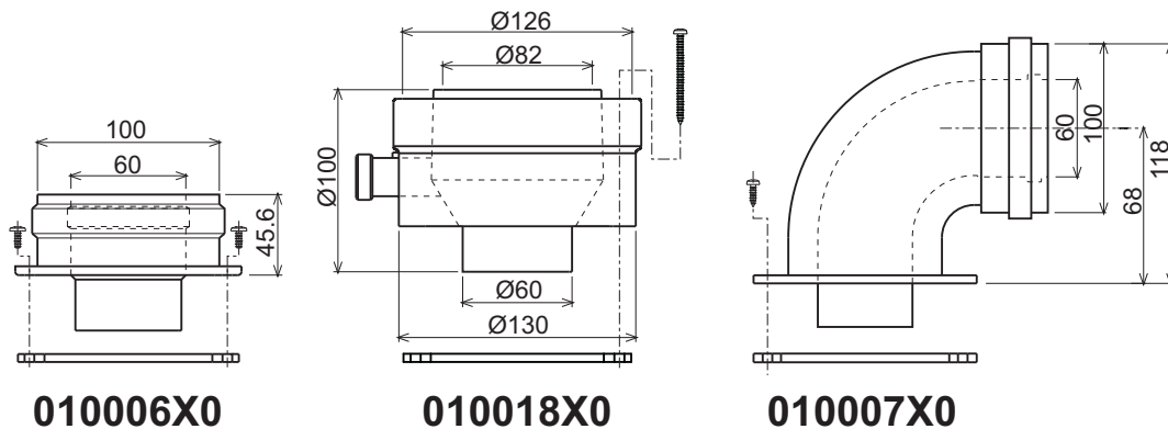
мал. 30- Початкові елементи для коаксiальних трубопроводів
