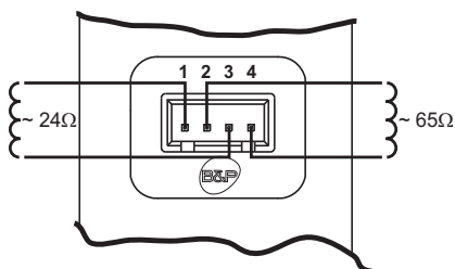
мал. 38 - Підключення газового клапану
