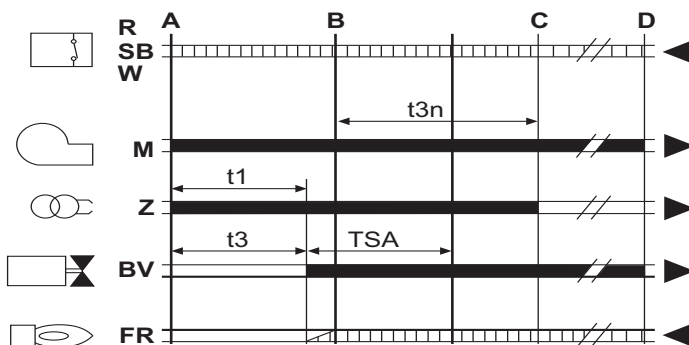
fig. 30 - Cycle de l'appareil
