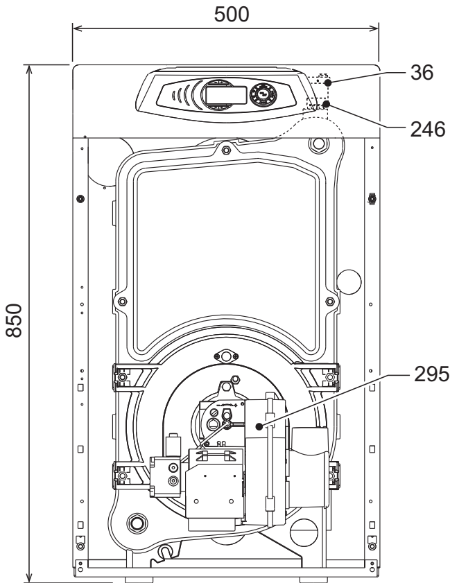
fig. 33 - Afmetingen aansluitingen en hoofdcomponenten
