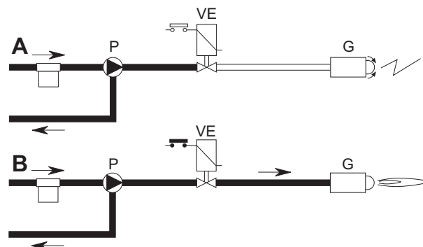
ΕΙΚ. 29 - Ενεργοποίηση
