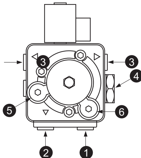
fig. 24- Pomp ITALPUMP
