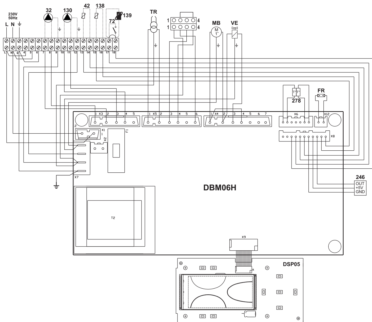
fig. 37 - Schakelschema
