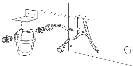
fig. 17 - Installatie brandstoffilter
