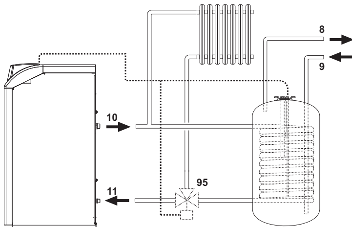
wygląd 16- Schemat podłączeń do zewnętrznego podgrzewacza
