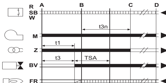
fig. 30 - Ciclo dell'apparecchiatura
