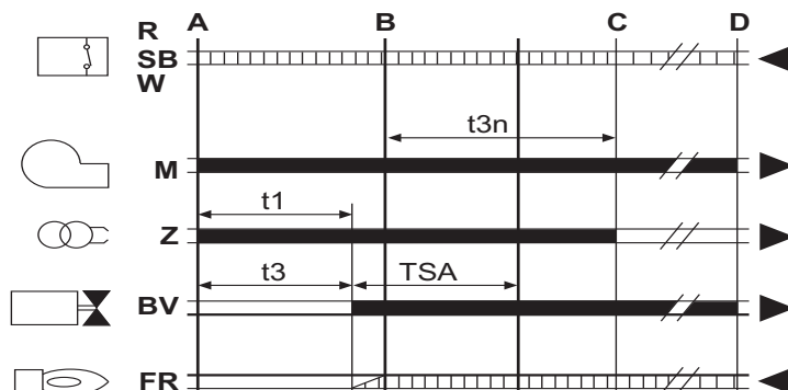
fig. 30 - Ciclo del aparato
