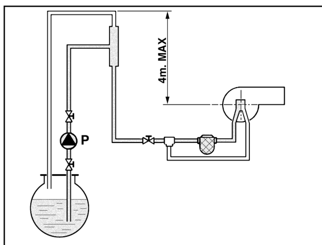
fig. 21 - Alimentazione ad anello
