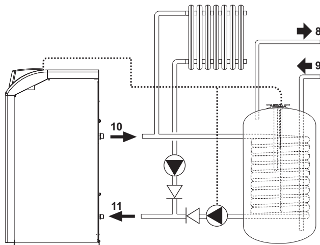
fig. 16 - Schéma de branchement à un ballon externe
