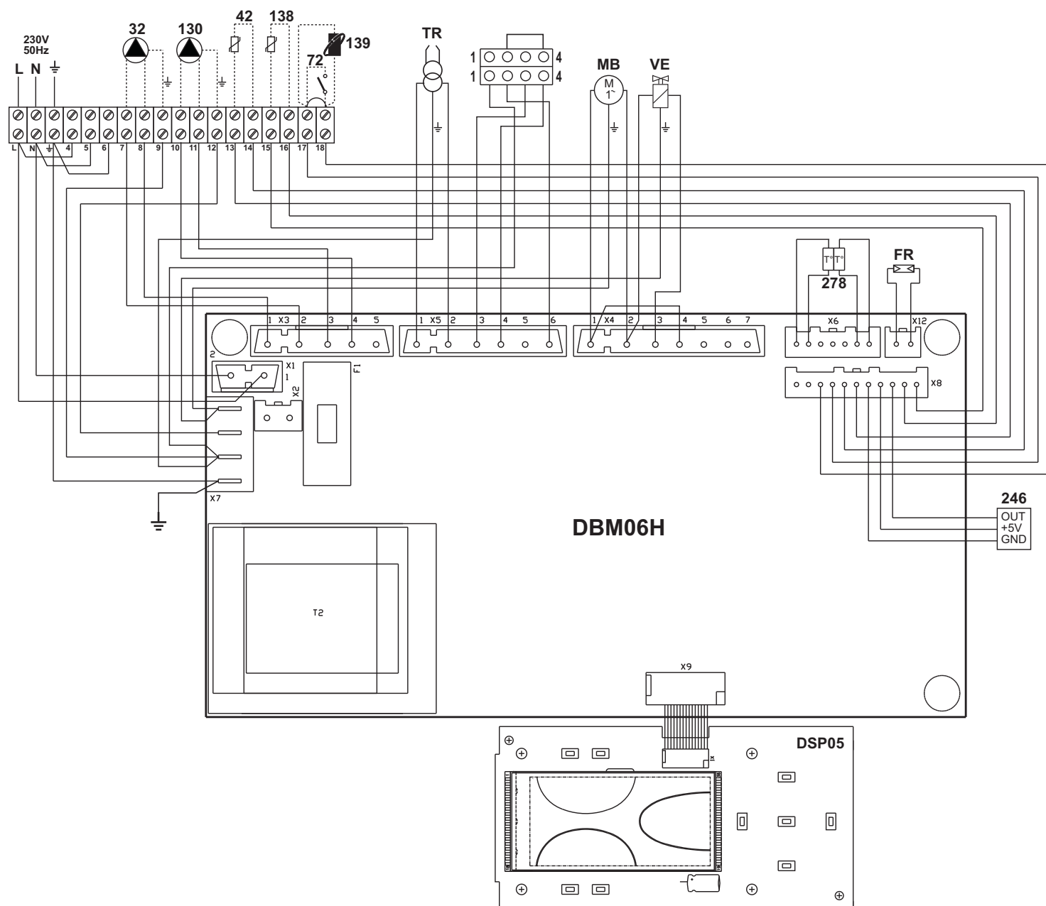
fig. 37 - Schéma électrique
