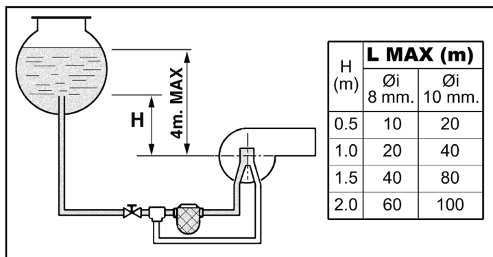
fig. 18 - Zwaartekrachtvoeding
