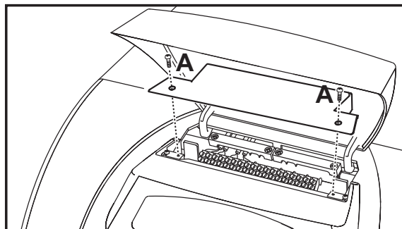
wygląd 22 - Dostęp do elektrycznej skrzynki zaciskowej
