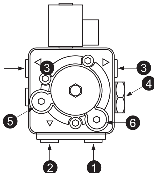
ΕΙΚ. 24- Αντλία ITALPUMP
