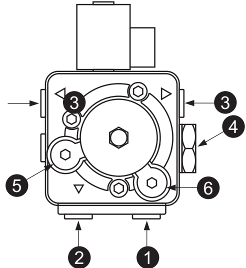
fig. 24- Pompe ITALPUMP
