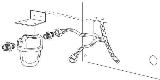
ΕΙΚ. 17 - Τοποθέτηση φίλτρου πετρελαίου
