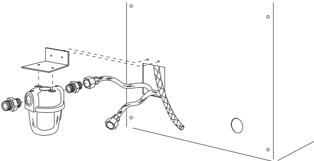
fig. 17 - Instalación del filtro del combustible
