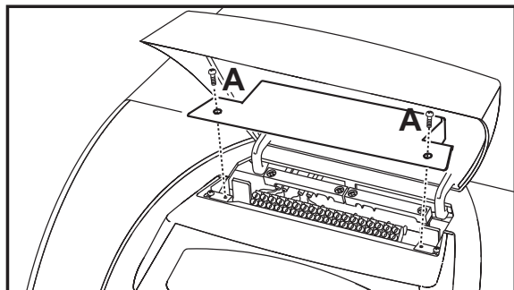
ΕΙΚ. 22 - Accesso alla morsettiera
