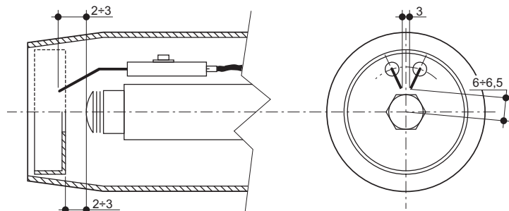
fig. 28 - Posizione elettrodi - deflettore
