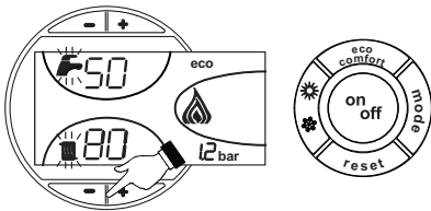
fig. 23 - Modo TEST
