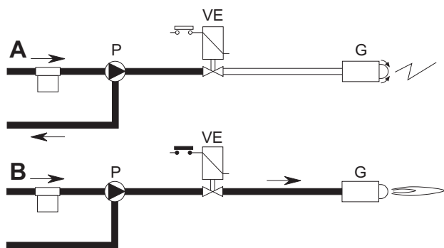
fig. 29 - Allumage
