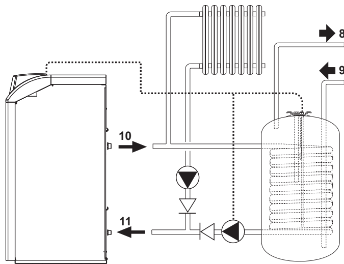
ΕΙΚ. 16 - Σχεδιάγραμμα σύνδεσης εξωτερικού θερμαντήρα
