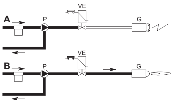
wygląd 29- Zapłon
