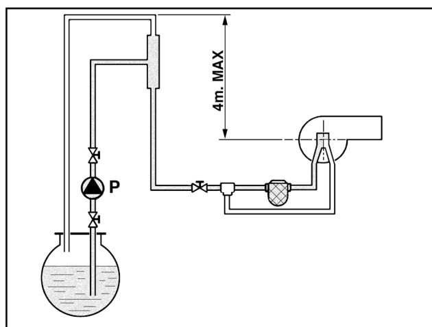
fig. 21 - Alimentation par anneau
