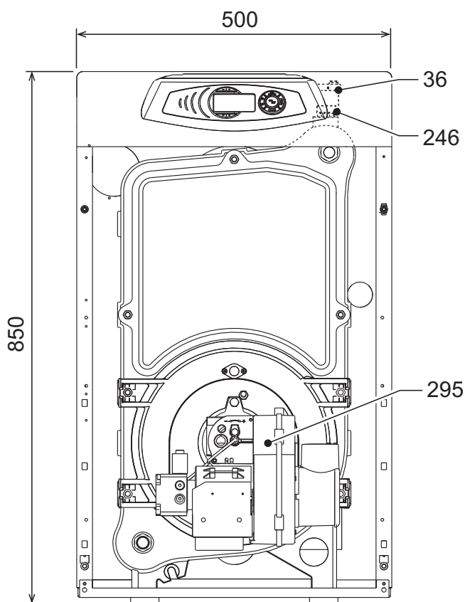
ΕΙΚ. 33 - Διαστάσεις, συνδέσεις και κύρια εξαρτήματα
