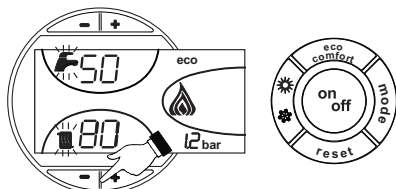
ΕΙΚ. 23 - Λειτουργία TEST
