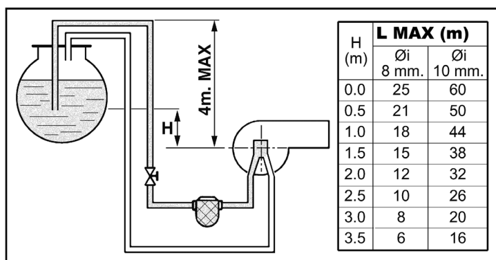
wygląd 20- Zasilanie syfonowe
