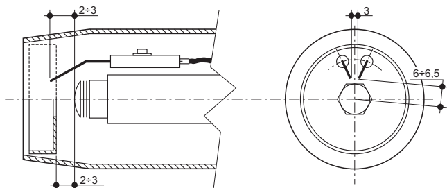
wygląd 28- Pozycja elektrod - deflektora
