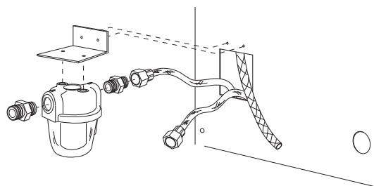
fig. 17 - Installation filtre combustible
