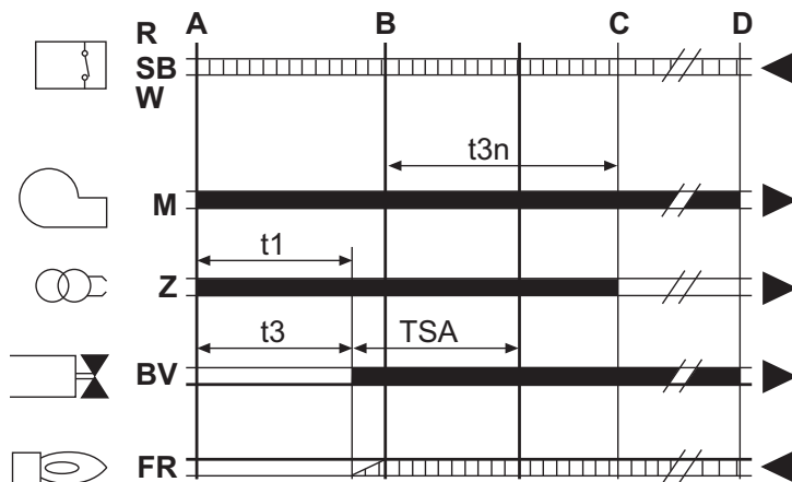
ΕΙΚ. 30 - Κύκλος συσκευής
