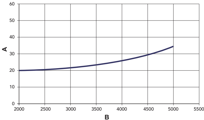
fig. 36 - Drukhoogteverlies
