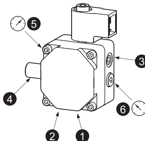
fig. 25 - Pompa DANFOSS
