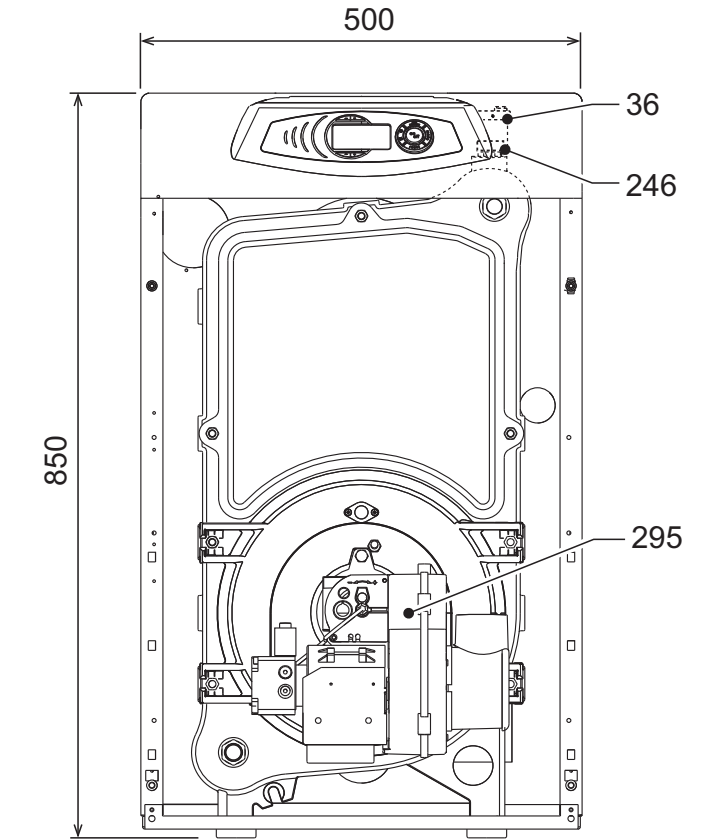
fig. 33 - Dimensions raccords et composants principaux
