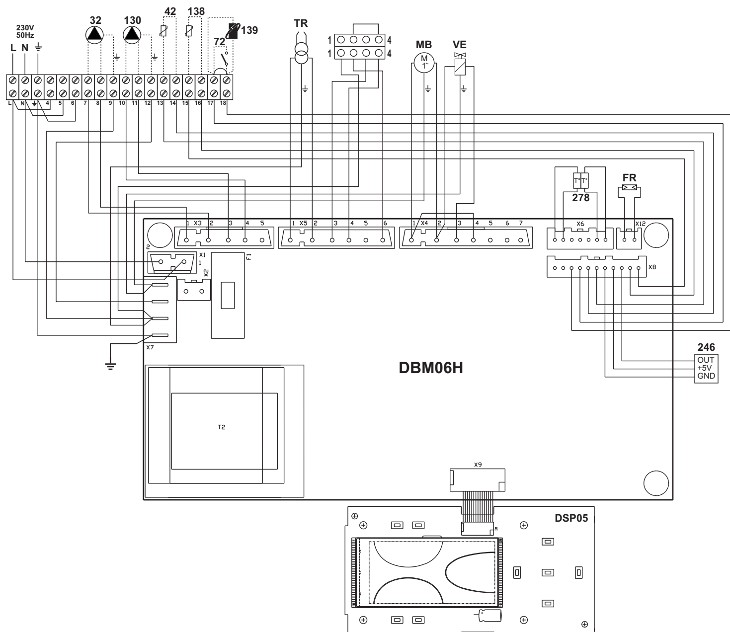
ΕΙΚ. 37 - Ηλεκτρολογικό διάγραμμα
