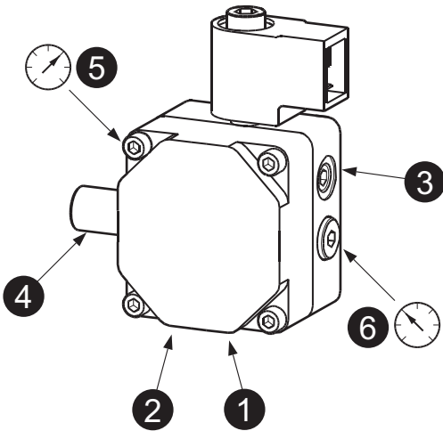
fig. 25- Bomba DANFOSS
