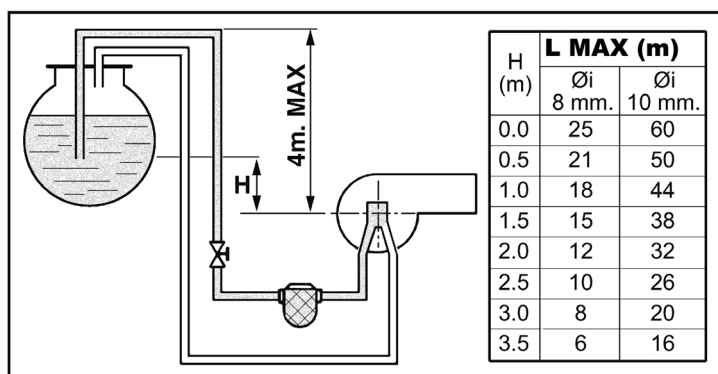
ΕΙΚ. 20 - Τροφοδοσία μέσω σιφονιού
