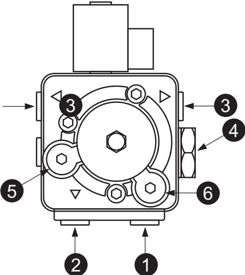
fig. 24- Bomba ITALPUMP
