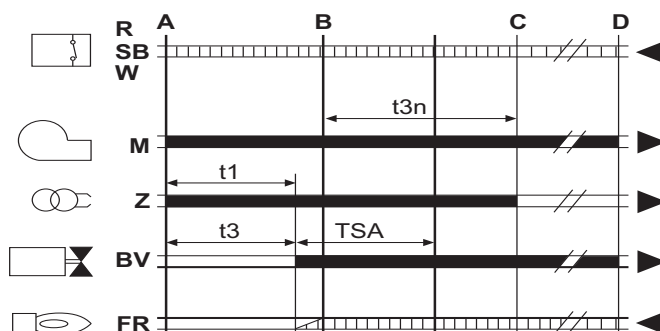
fig. 30 - Cyclus van het apparaat
