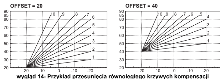
wygląd 14- Przykład przesunięcia równoległego krzywych kompensacji
