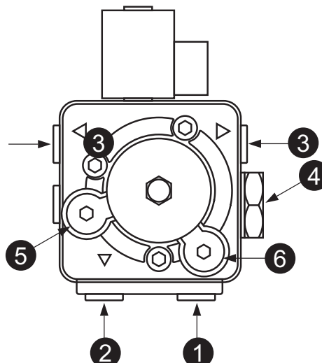
fig. 24 - Pompa ITALPUMP
