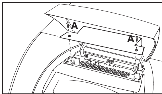
fig. 22 - Accesso alla morsettiere
