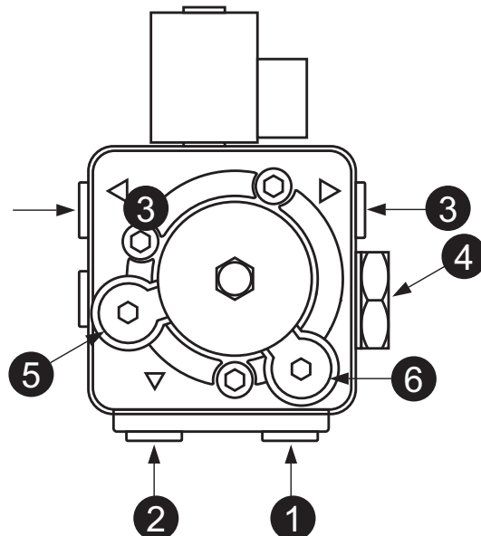
wygląd 24- Pompa ITALPUMP
