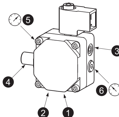
ΕΙΚ. 25- Αντλία DANFOSS
