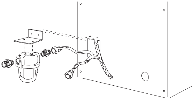
fig. 17 - Installazione filtro combustibile
