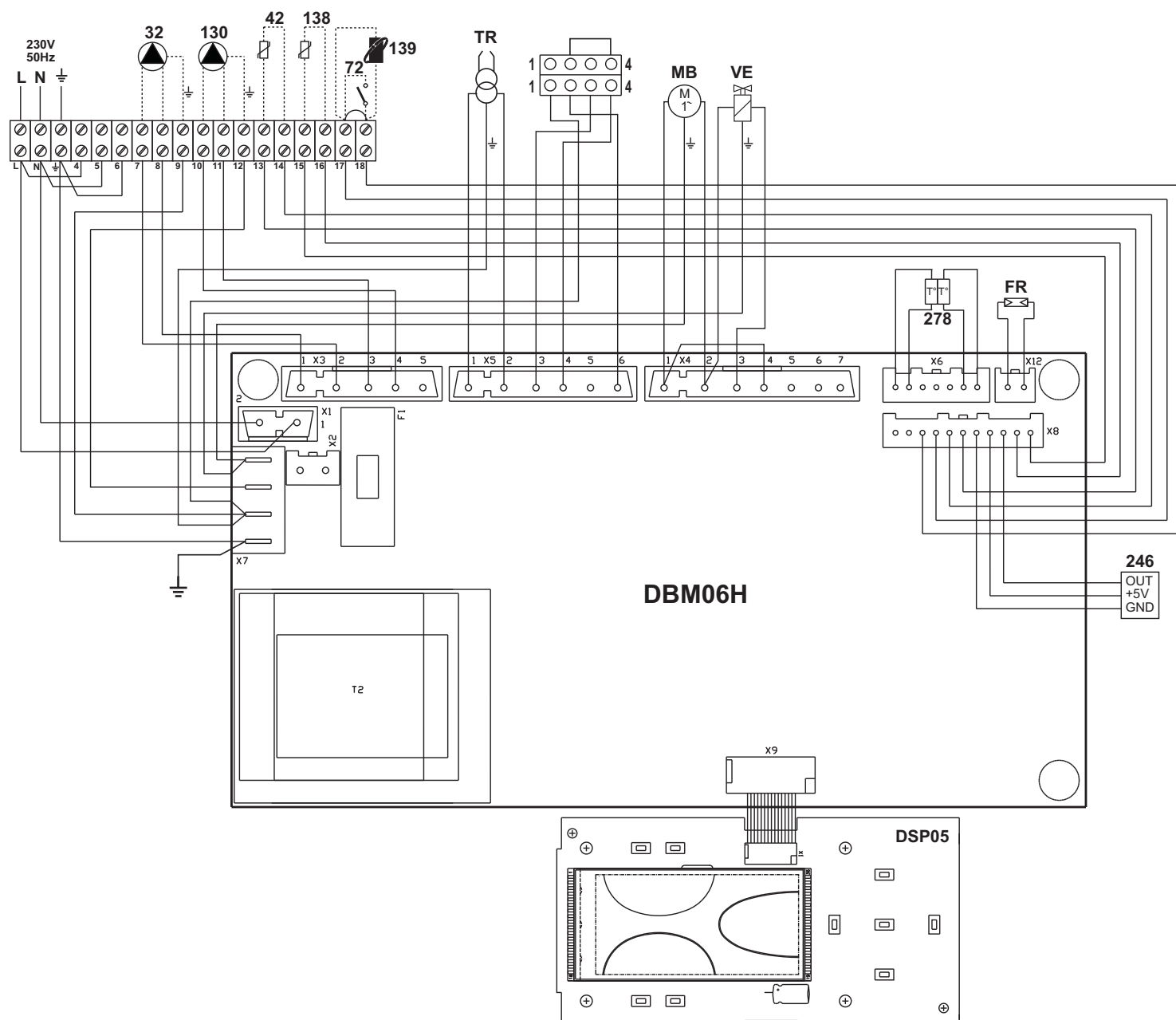
fig. 37 - Wiring diagram
