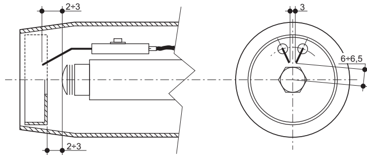
ΕΙΚ. 28- Θέση ηλεκτροδίων - διαφράγματος
