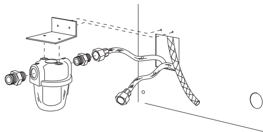
wygląd 17- Instalacja filtra paliwa
