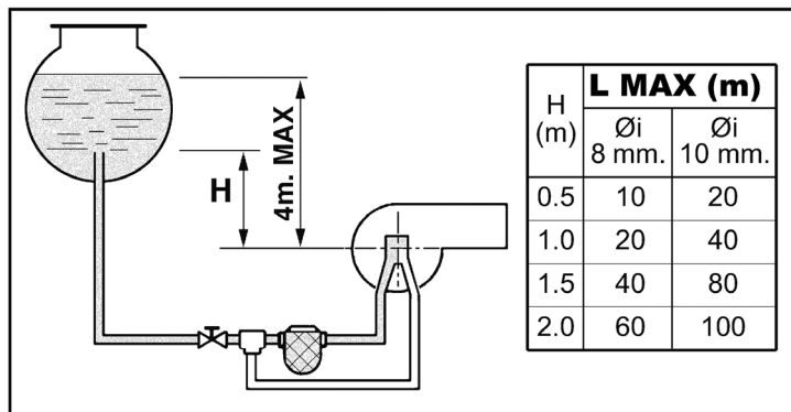
wygląd 18- Zasilanie grawitacyjne
