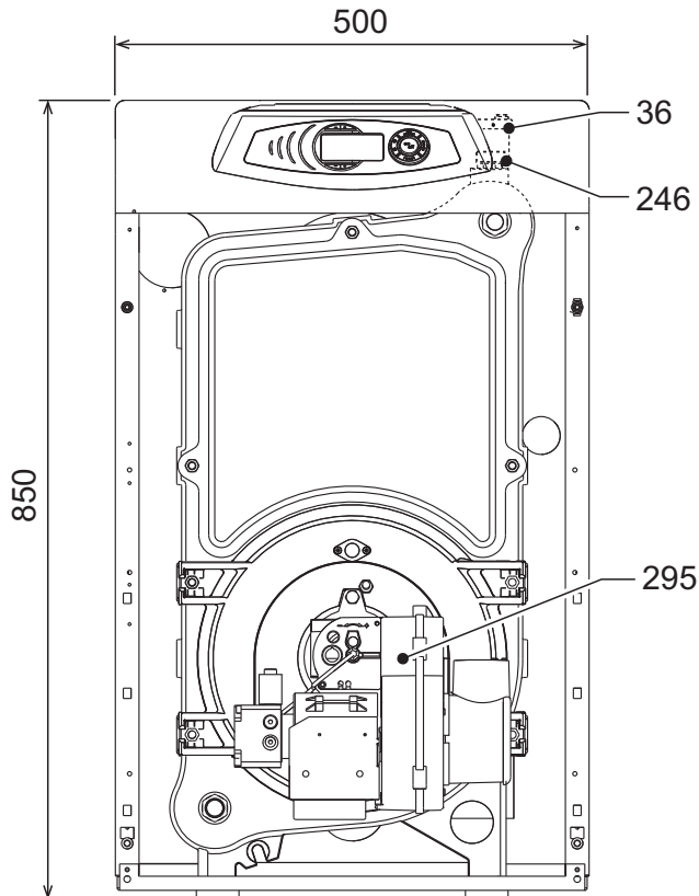
fig. 33 - Dimensiones de conexiones y componentes principales
