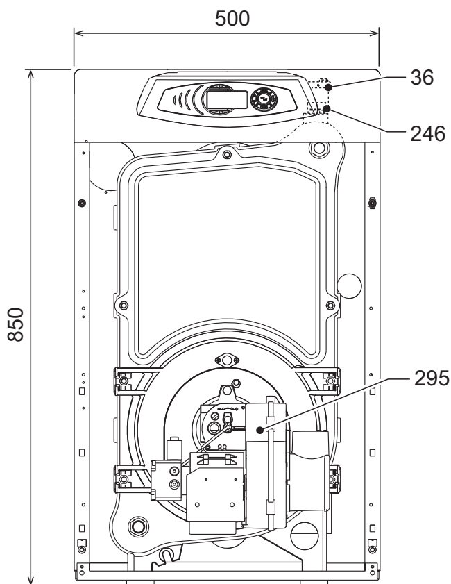
fig. 33 - Dimensione attacchi e componenti principali
