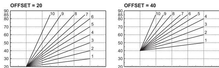
ΕΙΚ. 14 - Παράδειγμα παράλληλης μετατόπισης των καμπυλών αντίσταθμησης
