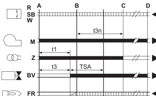
wygląd 30- Cykl urządzenia
