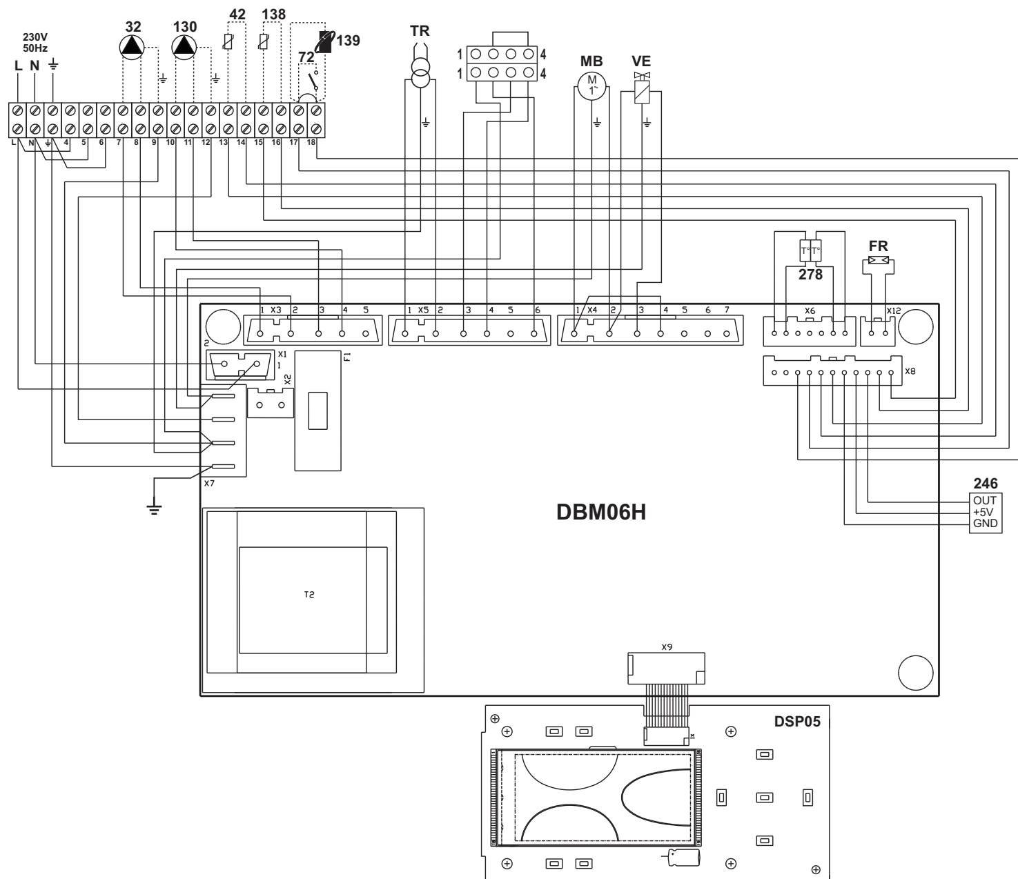
wygląd 37- Schemat elektryczny
