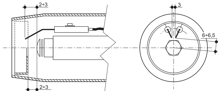
fig. 28- Position des électrodes - déflecteur
