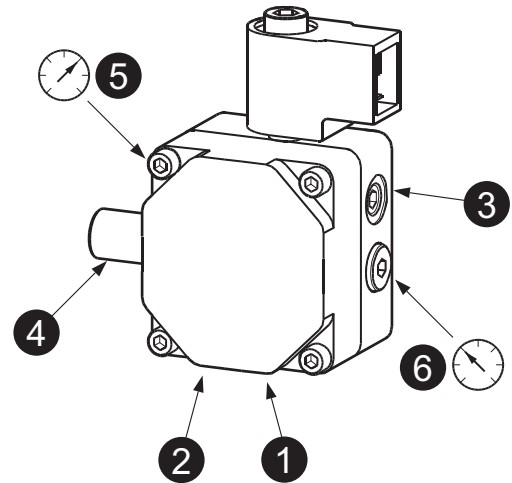
fig. 25- Pompe DANFOSS
