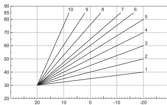
fig. 13 - Courbes de compensation
