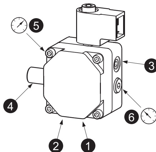
fig. 25- Pomp DANFOSS
