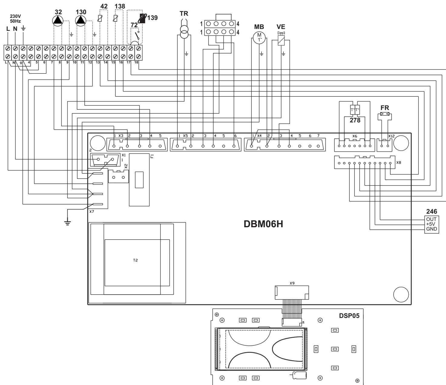
fig. 37 - Esquema eléctrico
