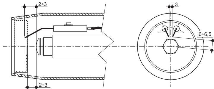
fig. 28- Plaats elektroden - deflector
