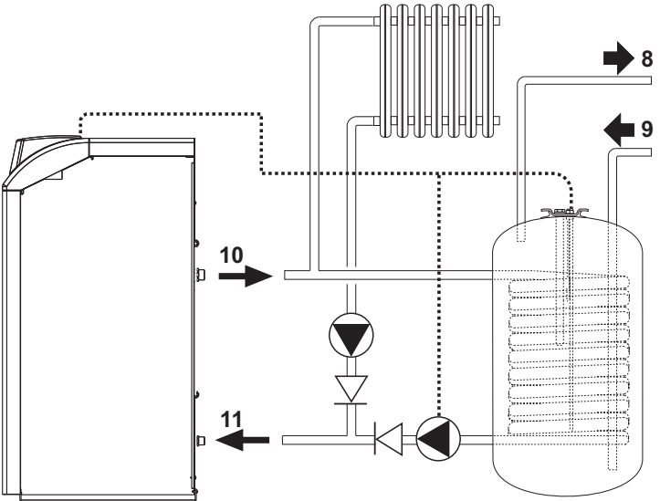
fig. 16 - Esquema para la conexión a un acumulador exterior
