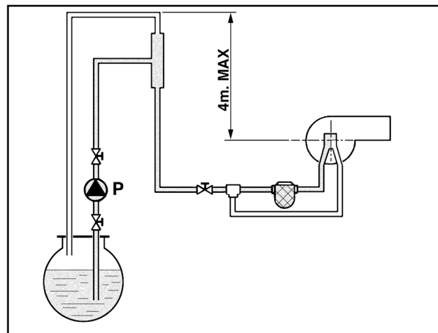
ΕΙΚ. 21 - Τροφοδοσία μέσω δακτυλίου
