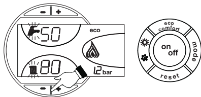
wygląd 23- Tryb TEST
