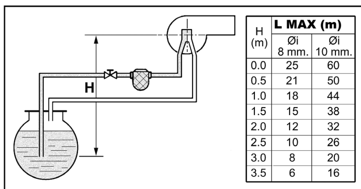
wygląd 19- Zasilanie za pomocą zasysania
