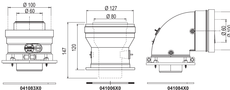
мал. 32- Початкові елементи для коаксialних трубопроводів
