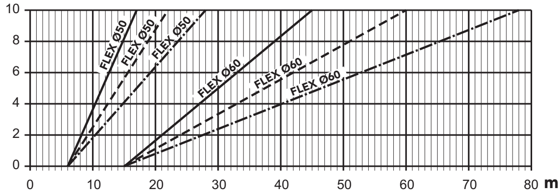
мал. 40- Графік для вибору параметра димоходу
