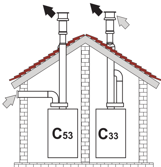
мал. 35- Приклади під'єднання за допомогою відокремлених труб
