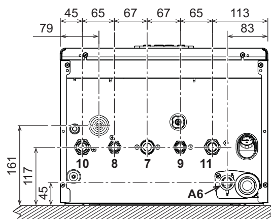
мал. 76- Вигляд знизу
