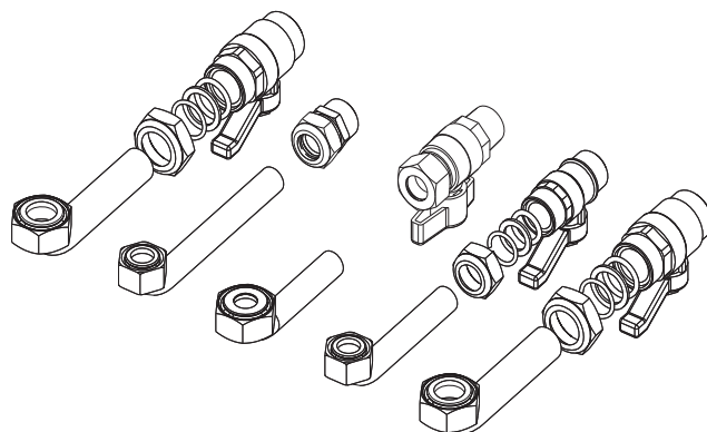
мал. 28- Комплект для гідротехнічного підключення
