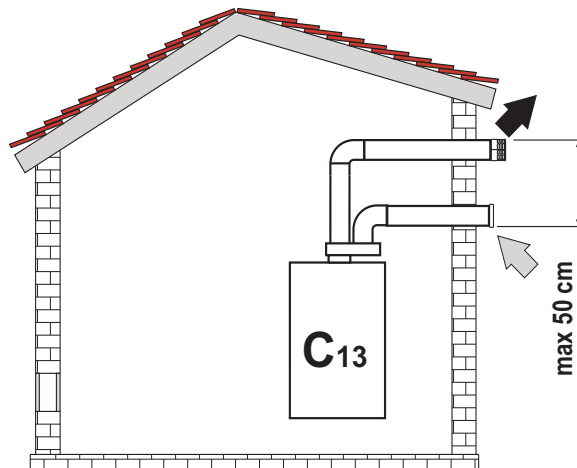
мал. 35- Приклади під'єднання за допомогою відокремлених труб
