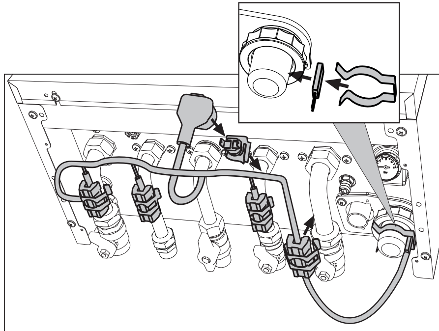
мал. 49- Комплект для захисту від замерзання
