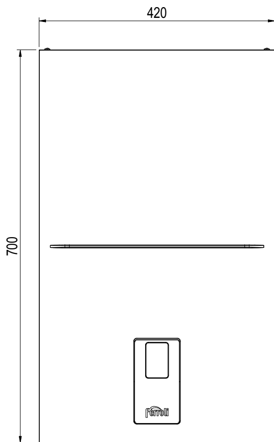
мал. 73- Вигляд спереду
