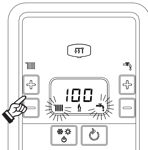
мал. 45- Тестовий режим TEST (потужність опалення = 100%)
