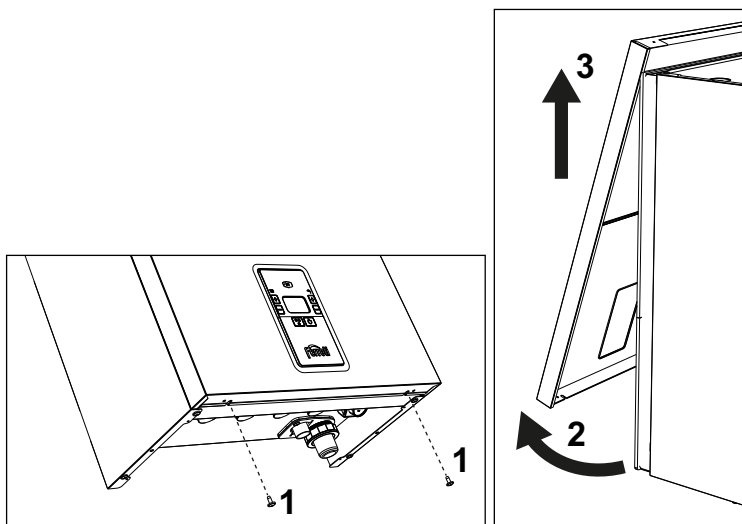
мал. 47- Відкриття передньої панелі
