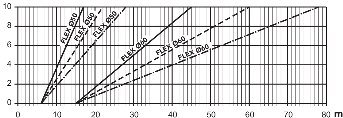
мал. 30- Графік для вибору параметра димоходу
