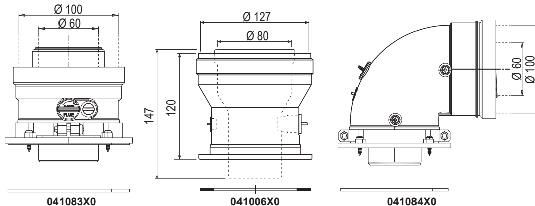
мал. 22- Початкові елементи для коаксіальних трубопроводів
