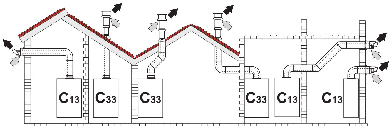
мал. 21- Приклади підключення за допомогою співвісних труб
