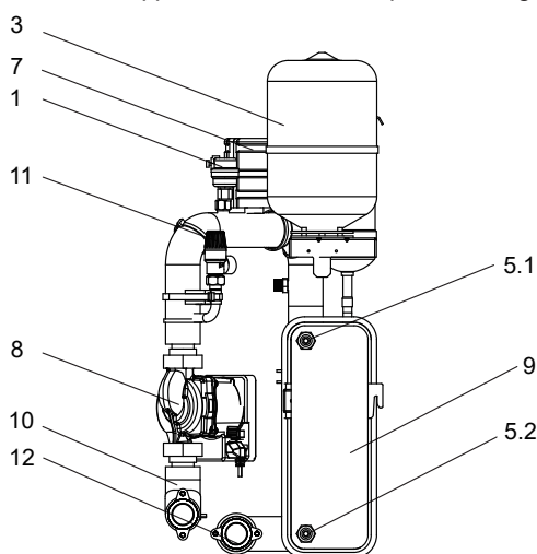
8-16 kW apparaat zonder back-upverwarming
