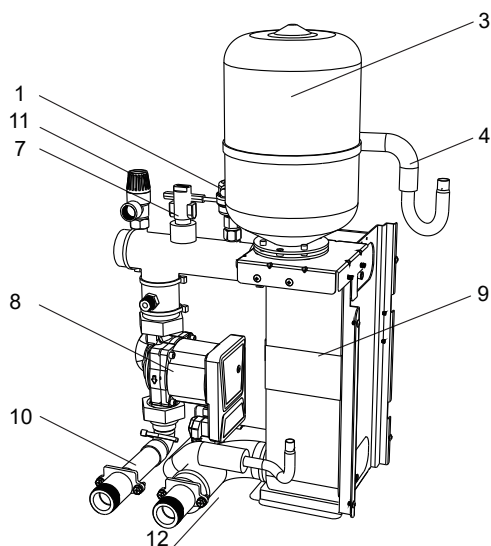
4/6 kW apparaat zonder back-upverwarming
