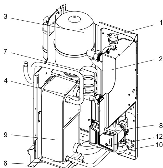
4/6 kW apparaat met back-upverwarming (optioneel)
