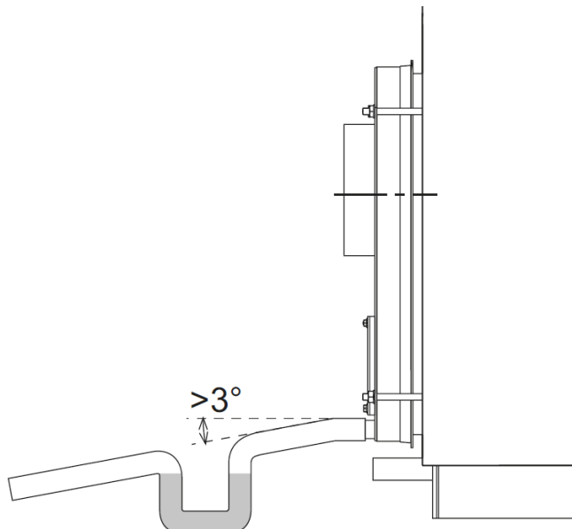
fig. 8 - Évacuation des condensats
