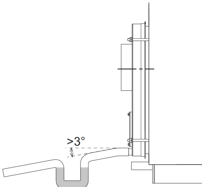
fig. 8 - Condensate discharge
