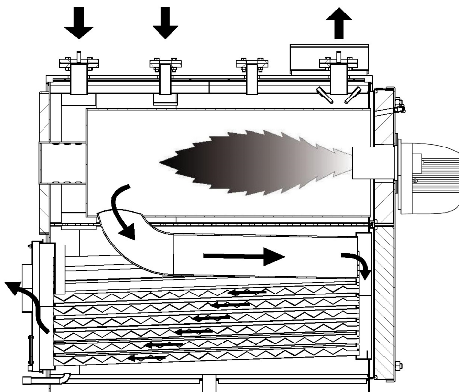
fig. 1 - Principe de fonctionnement
