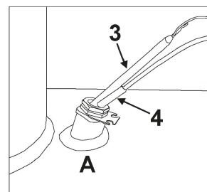
fig. 17 - Fourreau A
