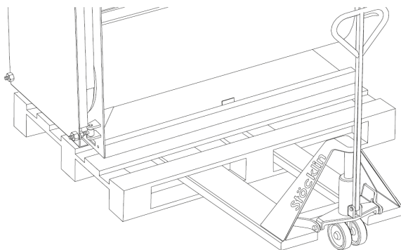
fig. 5 - Posizionamento
