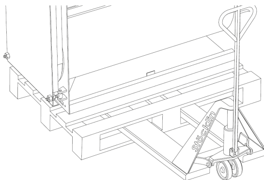
fig. 5 - Emplacement
