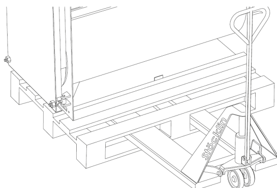
fig. 5 - Positioning
