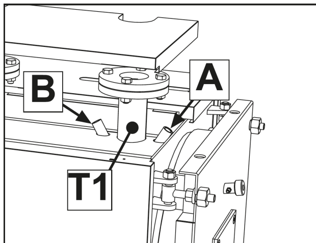
fig. 15 - Fourreau des sondes et des bulbes
