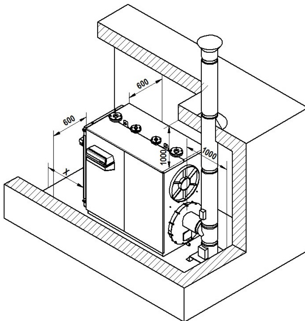
fig. 6 - Locale di installazione
