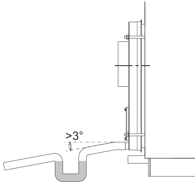
fig. 8 - Scarico condensa
