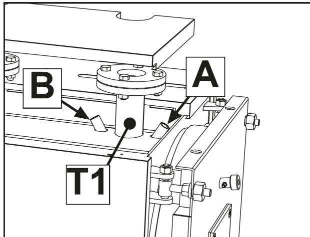
fig. 15 - Pozzetti inserimento sonde e bulbi
