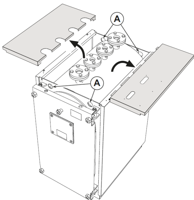
fig. 3 - Du modèle TP3 COND 65 au modèle TP3 COND 230
