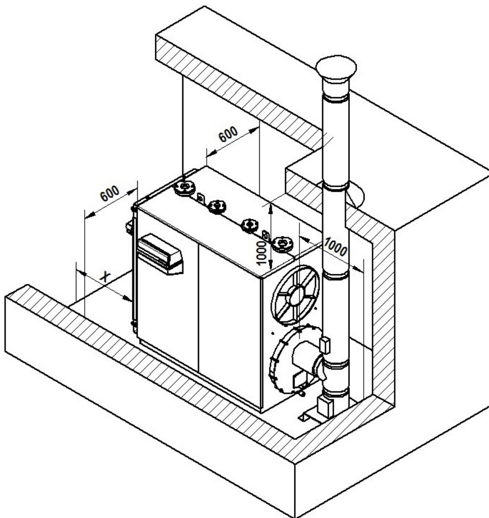
fig. 6 - Local d'installation
