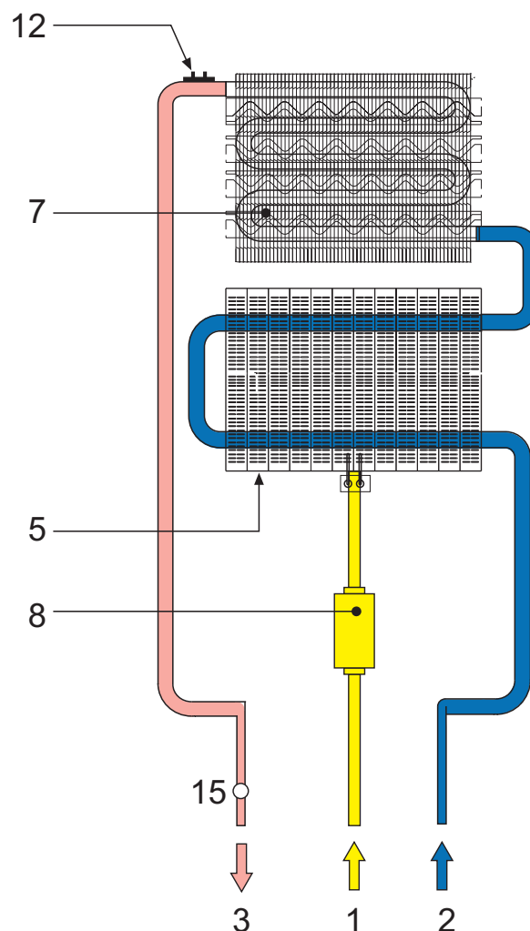
fig. 25 - Circuitul hidraulic
