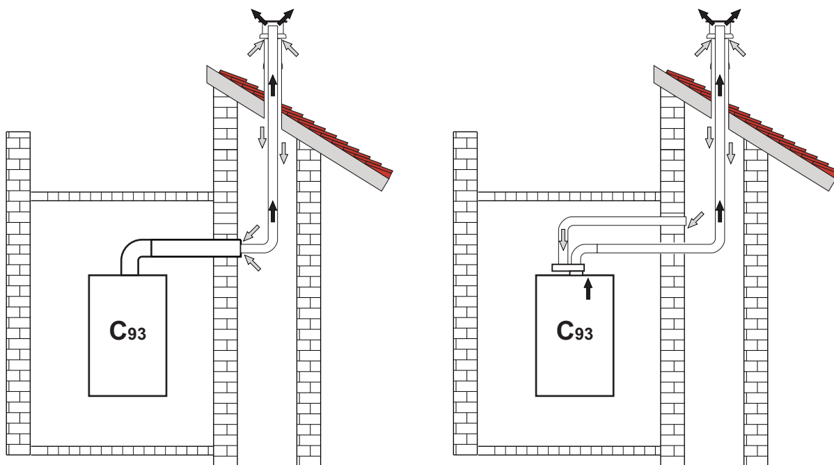
fig. 42- Aansluitvoorbeelden op rookkanalen (⇨ = Lucht ⇨ = Rook)
