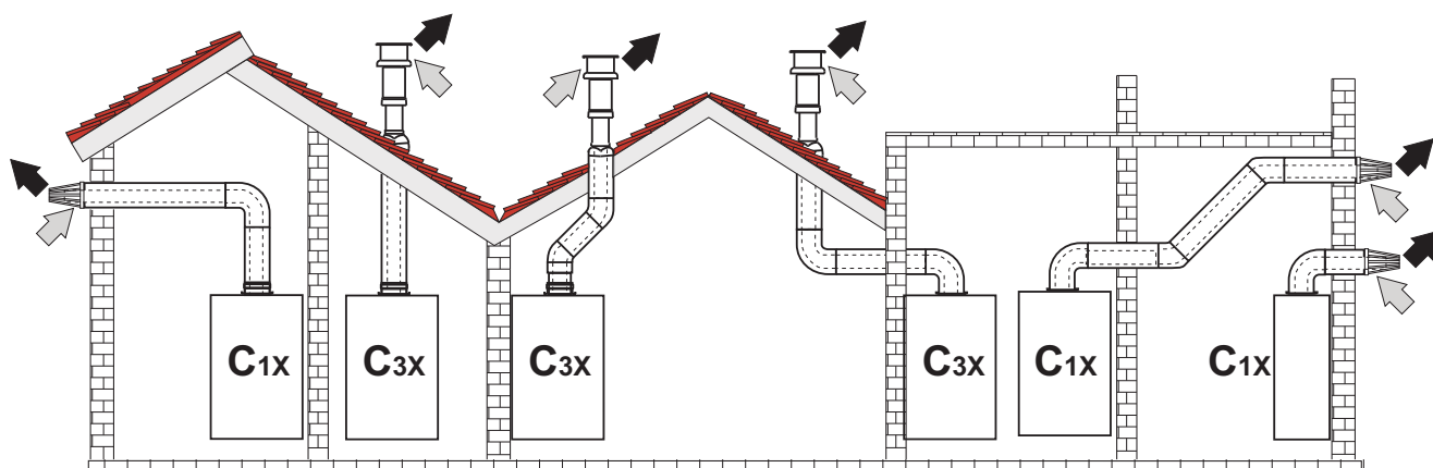
fig. 30- Aansluitvoorbeelden met coaxiale leidingen
