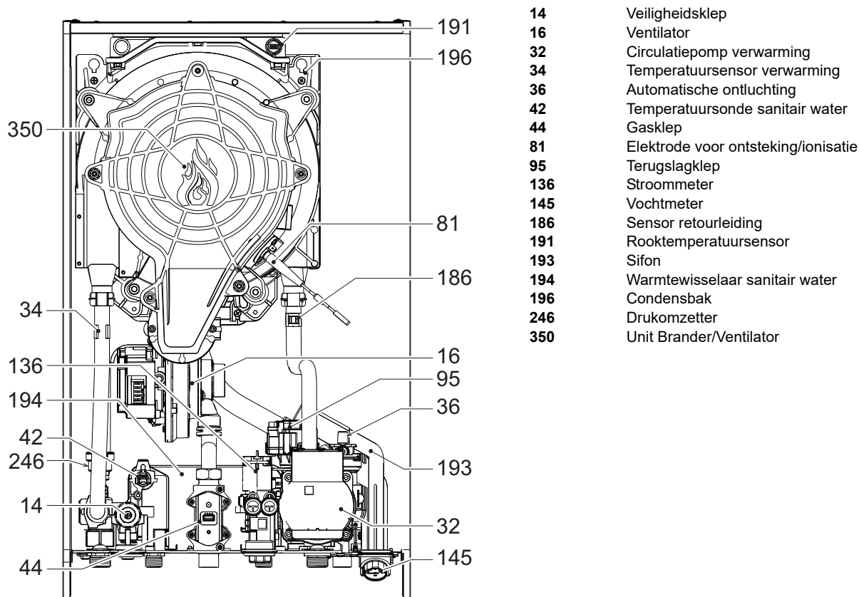
fig. 75- Aanzichttekening
