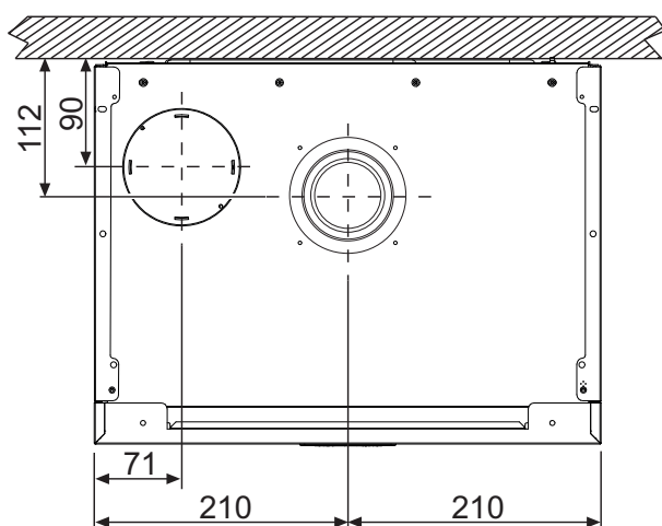
fig. 73 - Bovenaanzicht
