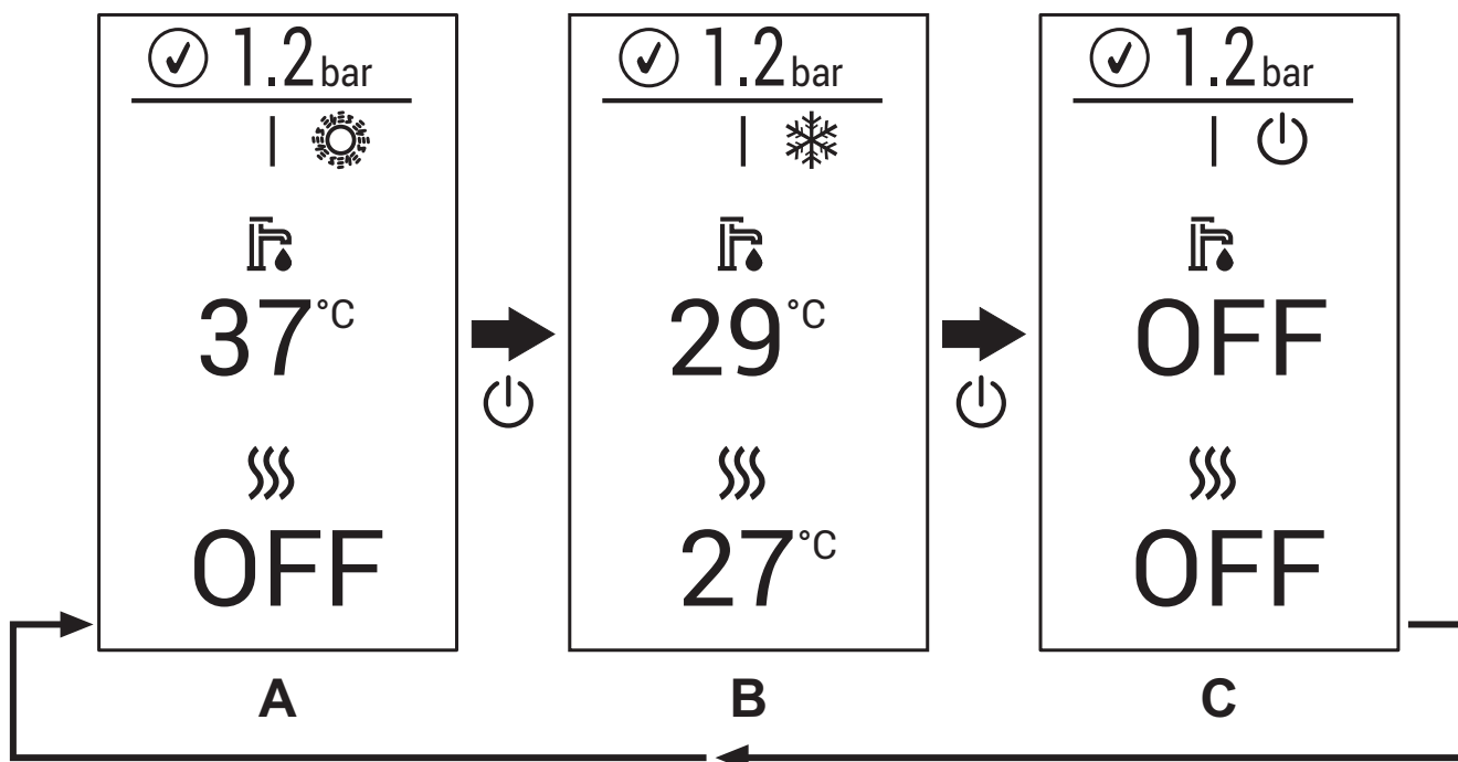
fig. 11- Uitschakelen verwarmingsketel
