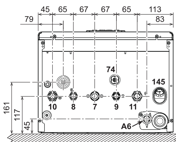
fig. 74 - Onderaanzicht
