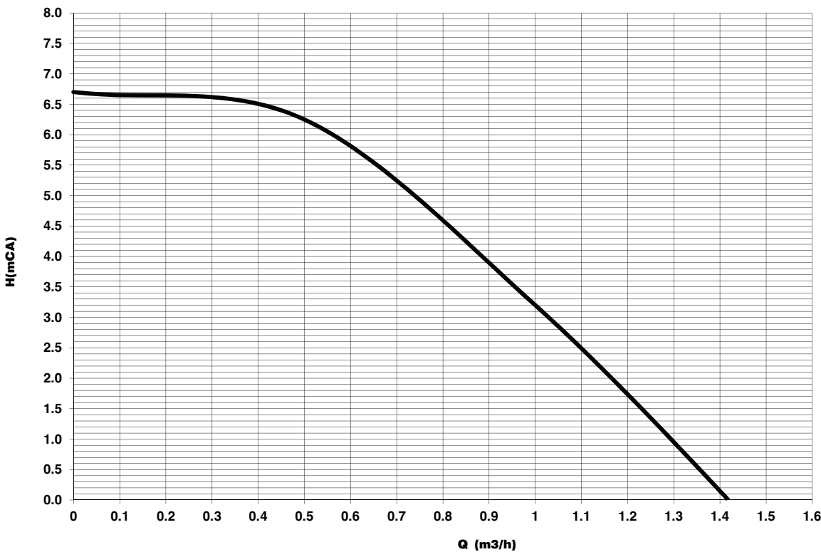
fig. 77- Overige beschikbare opvoerhoogte van de installatie
