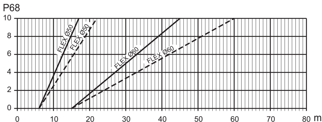
fig. 39- Grafiek voor keuze parameter schoorsteen
