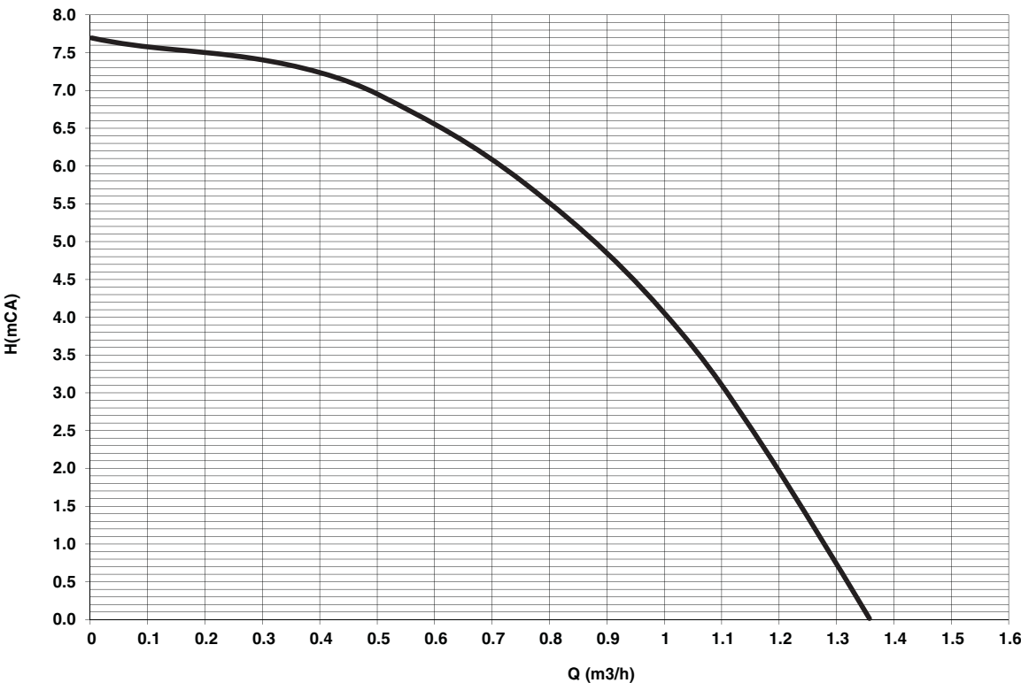
fig. 78- Overige beschikbare opvoerhoogte van de installatie
