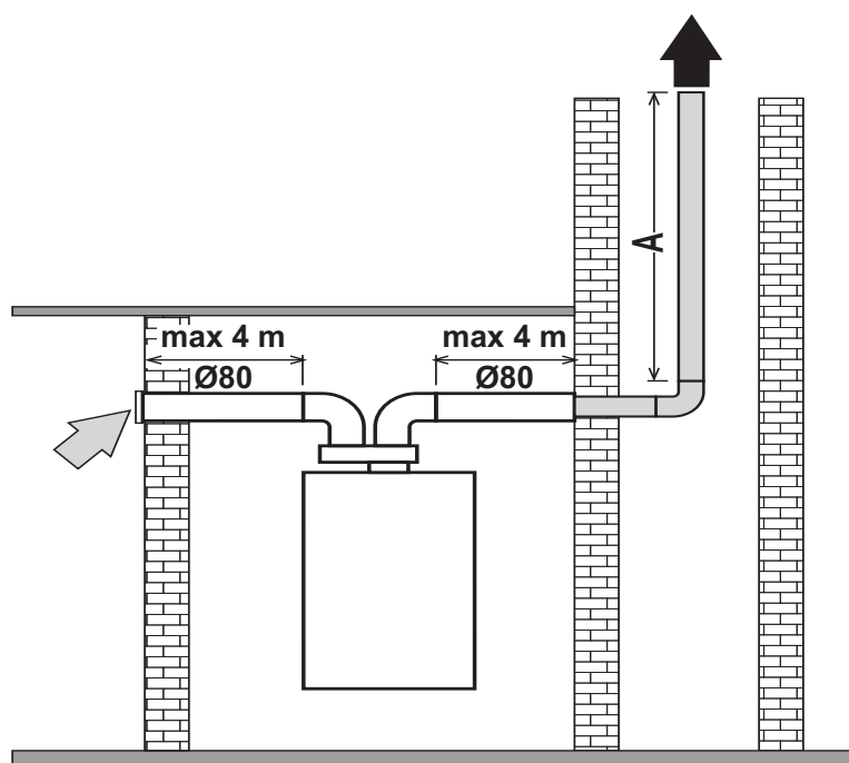
fig. 38- Schema voor alleen omkokering met een flexibele leiding
