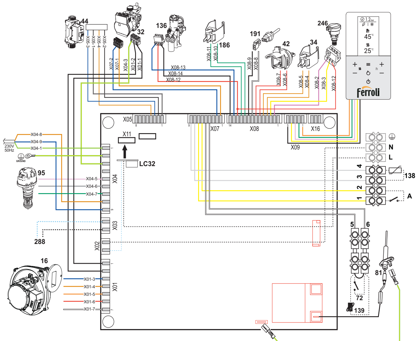
fig. 79- Schakelschema
