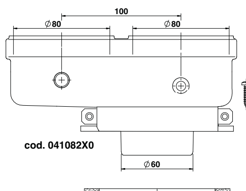
fig. 35- Startaccessoire voor gescheiden leidingen
