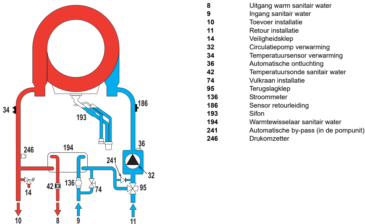
fig. 76- Watercircuit
