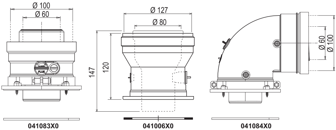
fig. 31- Startaccessoires voor coaxiale leidingen
