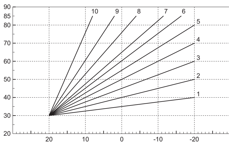
fig. 24- Compensatiecurven
