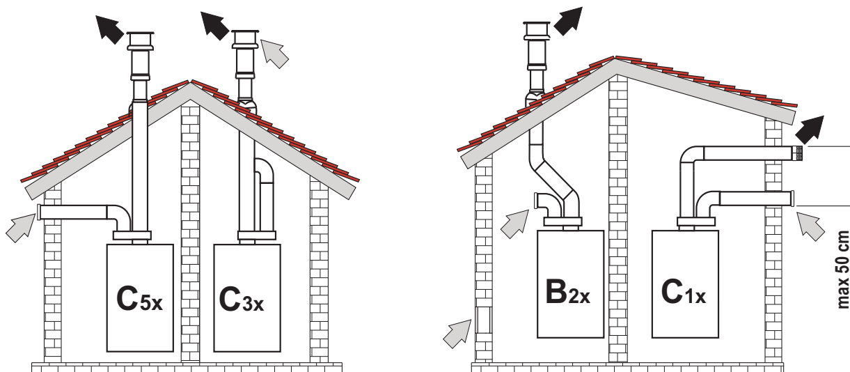
fig. 34- Aansluitvoorbeelden met gescheiden leidingen
