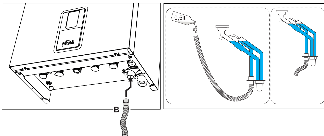
fig. 51- Aansluiting condensafvoer
