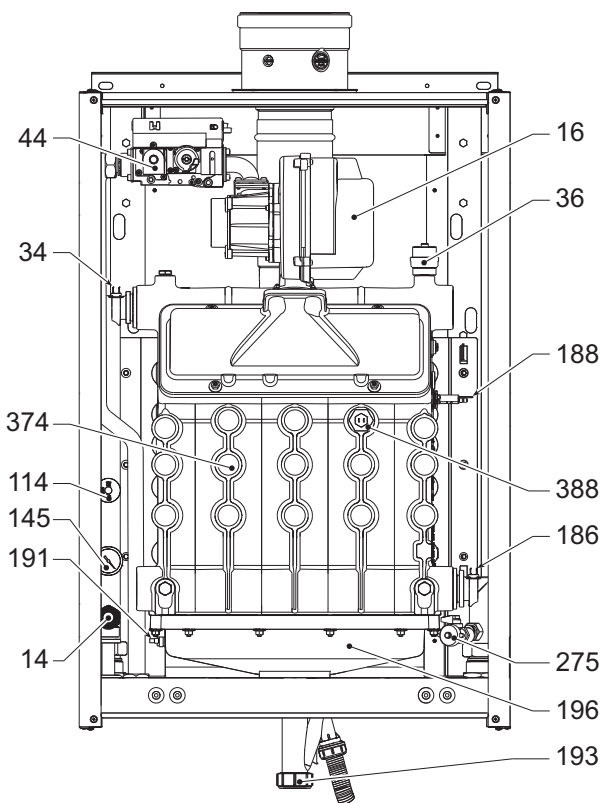
Slika 90- Opšti prikaz mod. FORCE W 150
