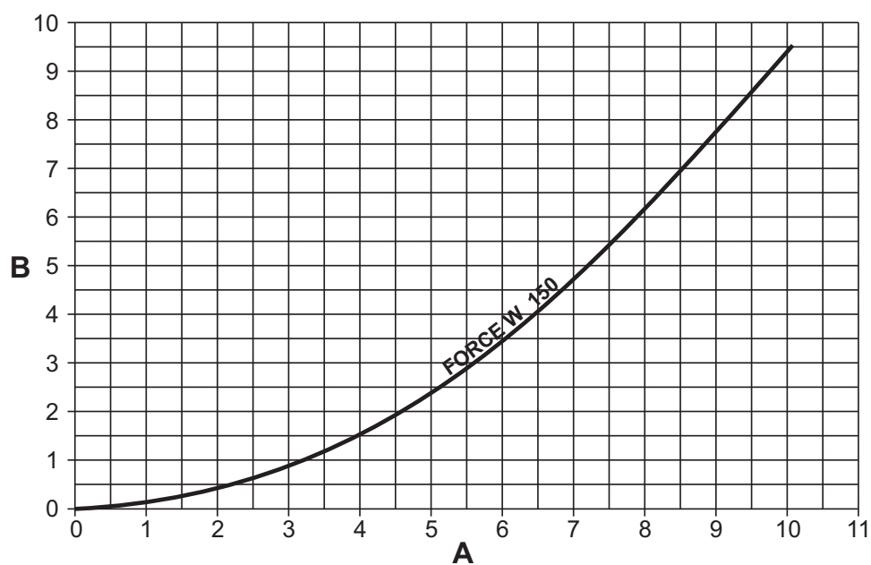
Slika 93- Dijagram gubitka pritiska modeli FORCE W 150
