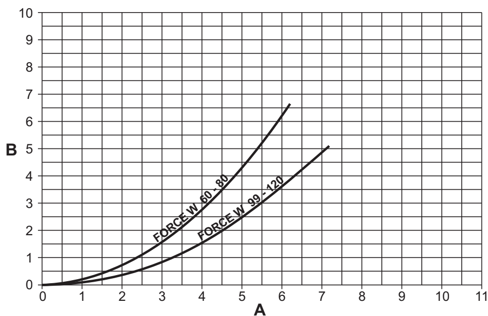
Slika 92- Dijagram gubitka pritiska modeli FORCE W 60 - FORCE W 80 - FORCE W 99 - FORCE W 120
