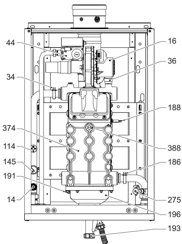
Slika 88- Opšti prikaz mod. FORCE W 60 i FORCE W 80
