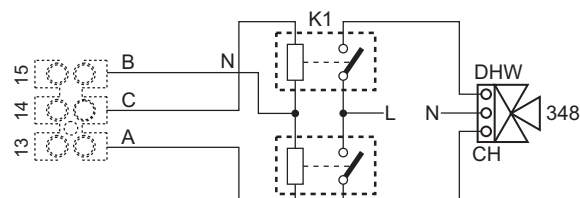
Slika 96- Povezivanje trokrakog ventila sa 3 žice
