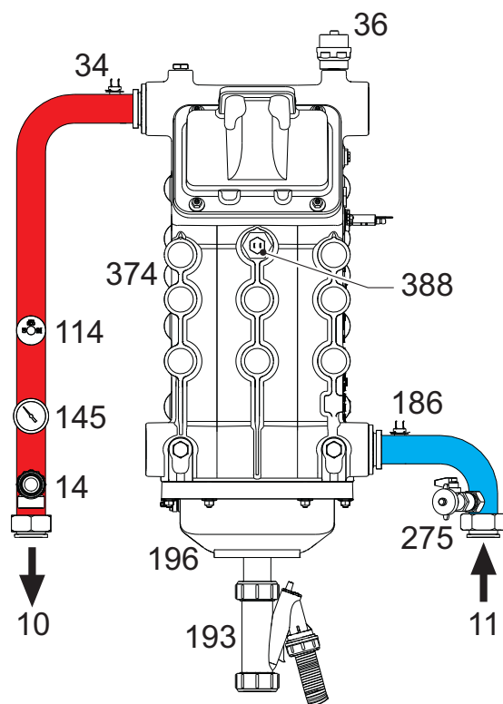
Slika 91- Hidraulički sistem
