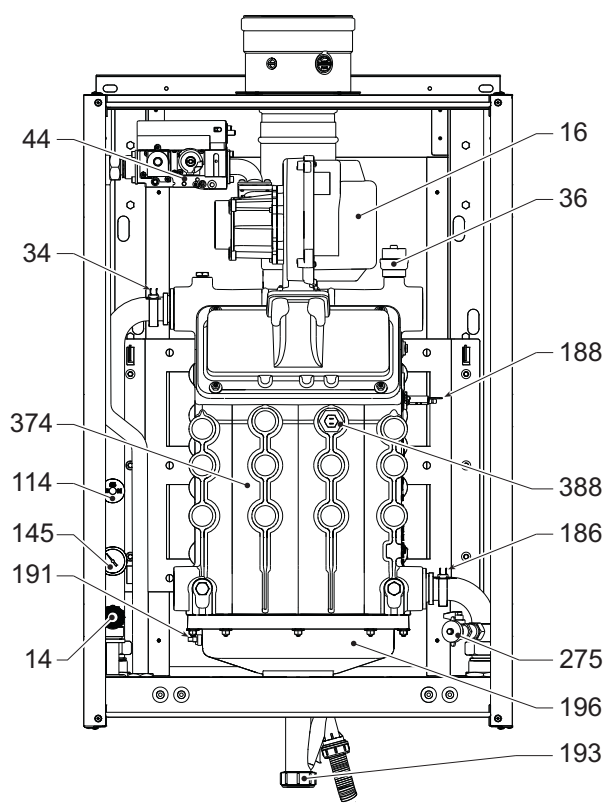
Slika 89- Opšti prikaz mod. FORCE W 99 i FORCE W 120
