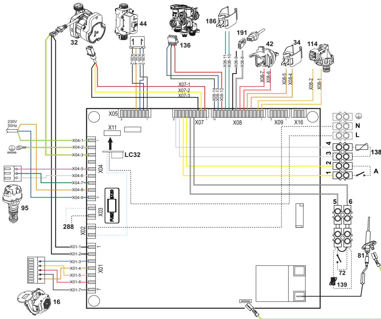
slika 60- Električna šema
