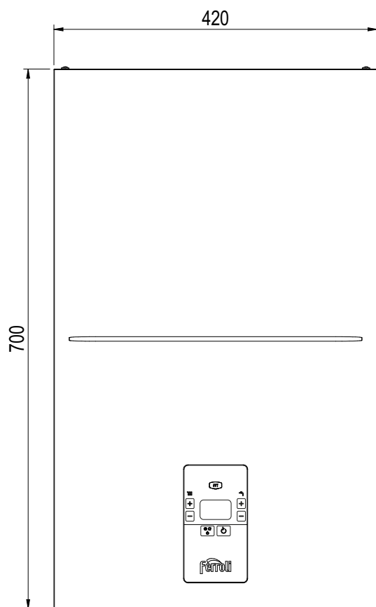
slika 53- Pogled spreda
