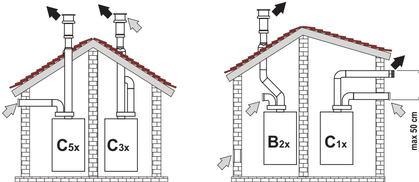
fig. 34- Exemple de racordare cu tuburi separate
