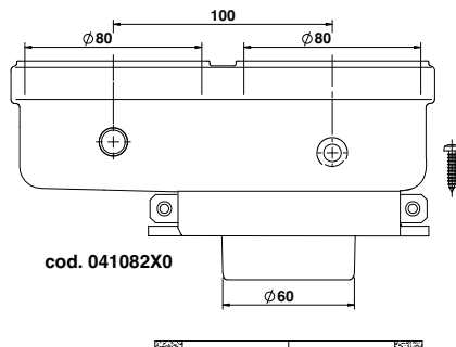
fig. 35- Accesoriu de pornire pentru conducte separate
