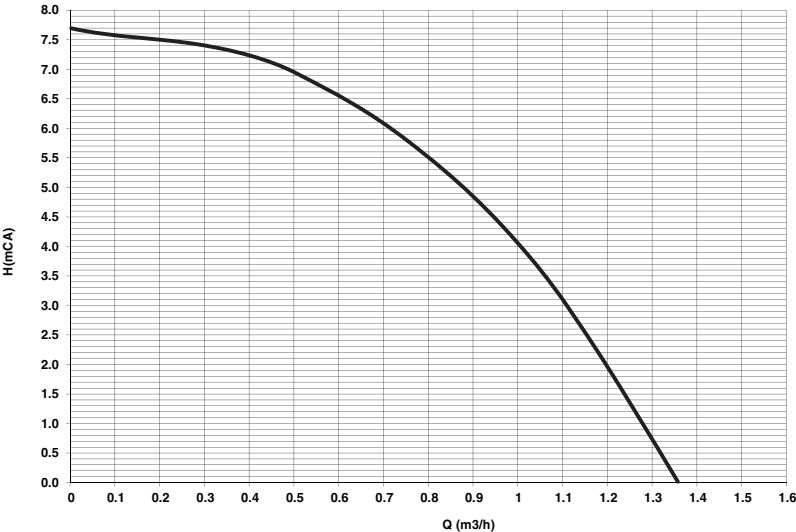
fig. 63- Înălțime de pompare reziduală disponibilă în instalație
