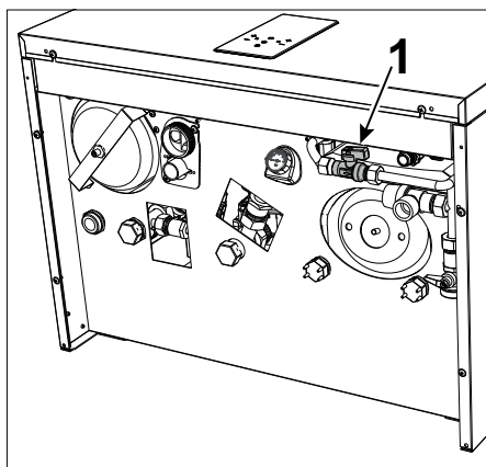
fig. 26- Buton de umplere
