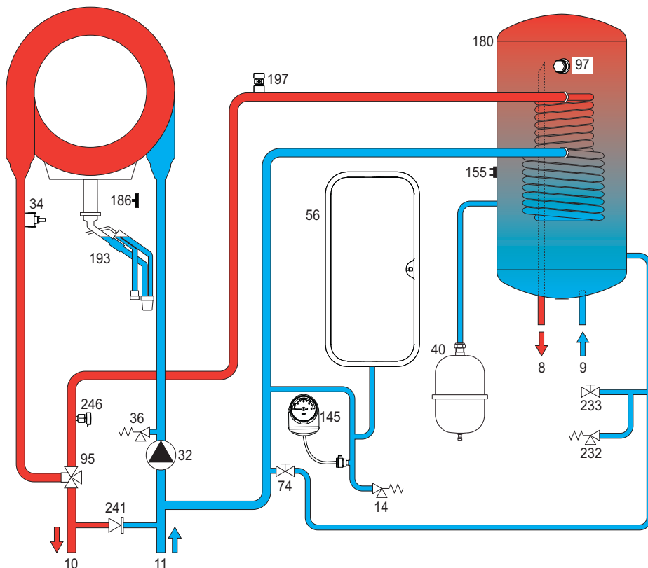
fig. 61- Circuitul hidraulic
