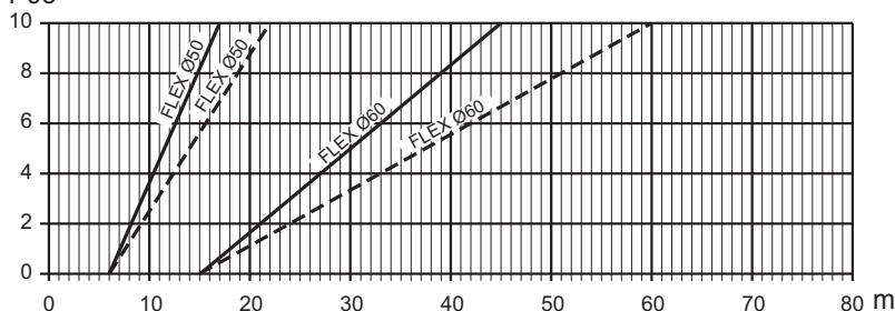
fig. 39- Grafic pentru alegerea parametrului pentru horn
