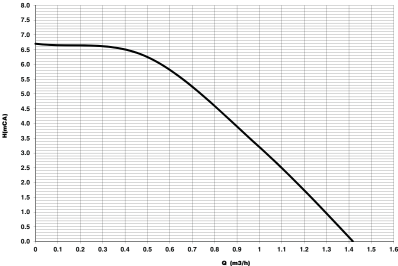
fig. 62- Înălțime de pompare reziduală disponibilă în instalație
