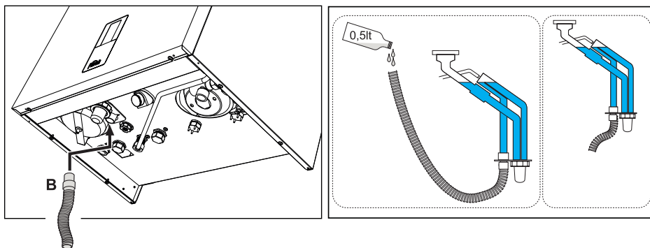
fig. 50- Racordarea evacuării condensului
