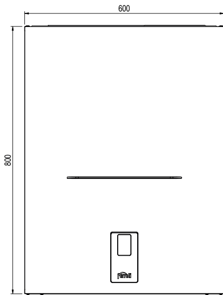
fig. 56- Vedere frontală
