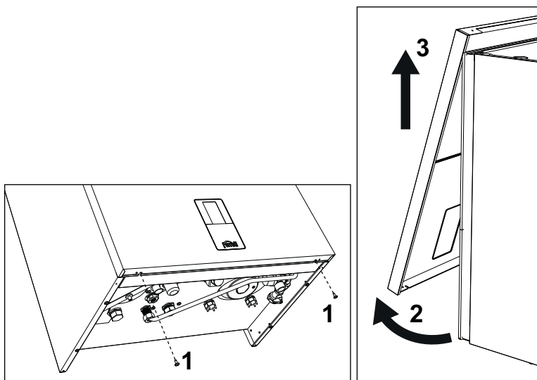
fig. 54- Deschiderea panoului frontal
