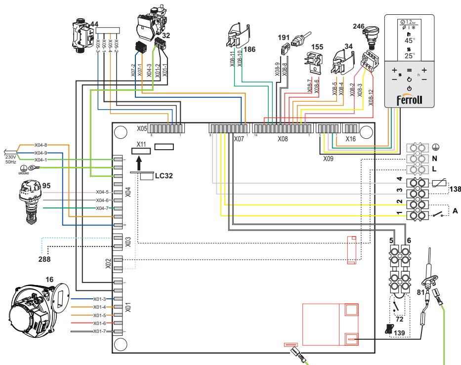
fig. 64- Schema electrică
