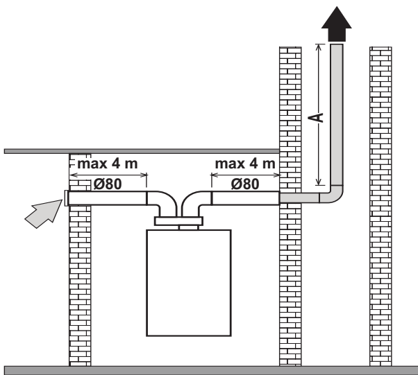
fig. 38- Schemă numai pentru tuburi flexibile
