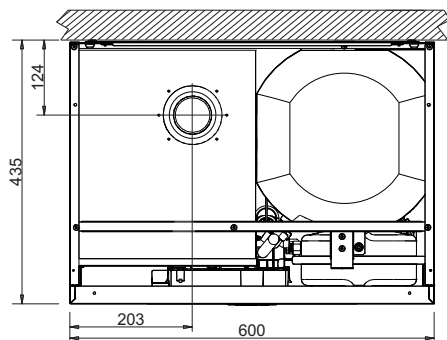
fig. 58- Vedere de sus
