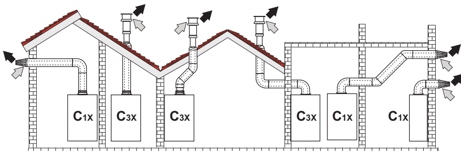
fig. 30- Exemple de racordare cu tuburi coaxiale
