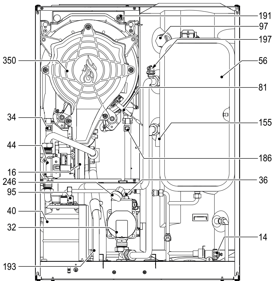
fig. 60- Vedere generală
