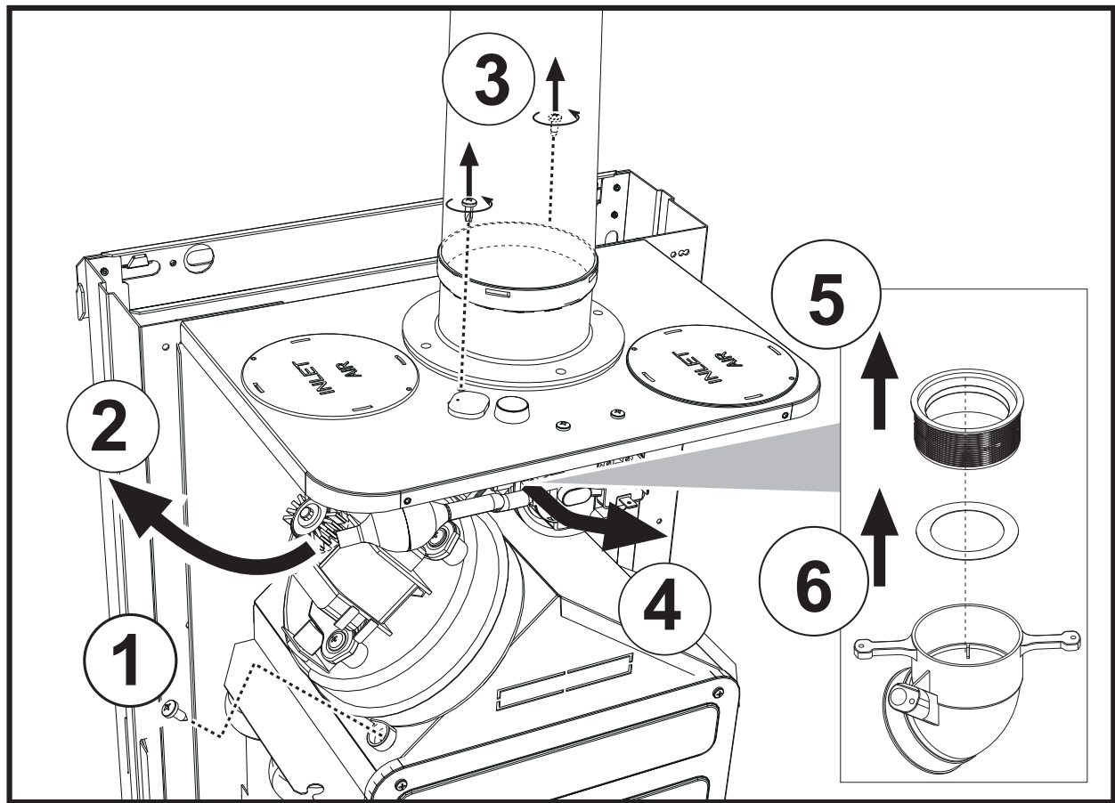
شكل 28 - استبدال الحاجز
