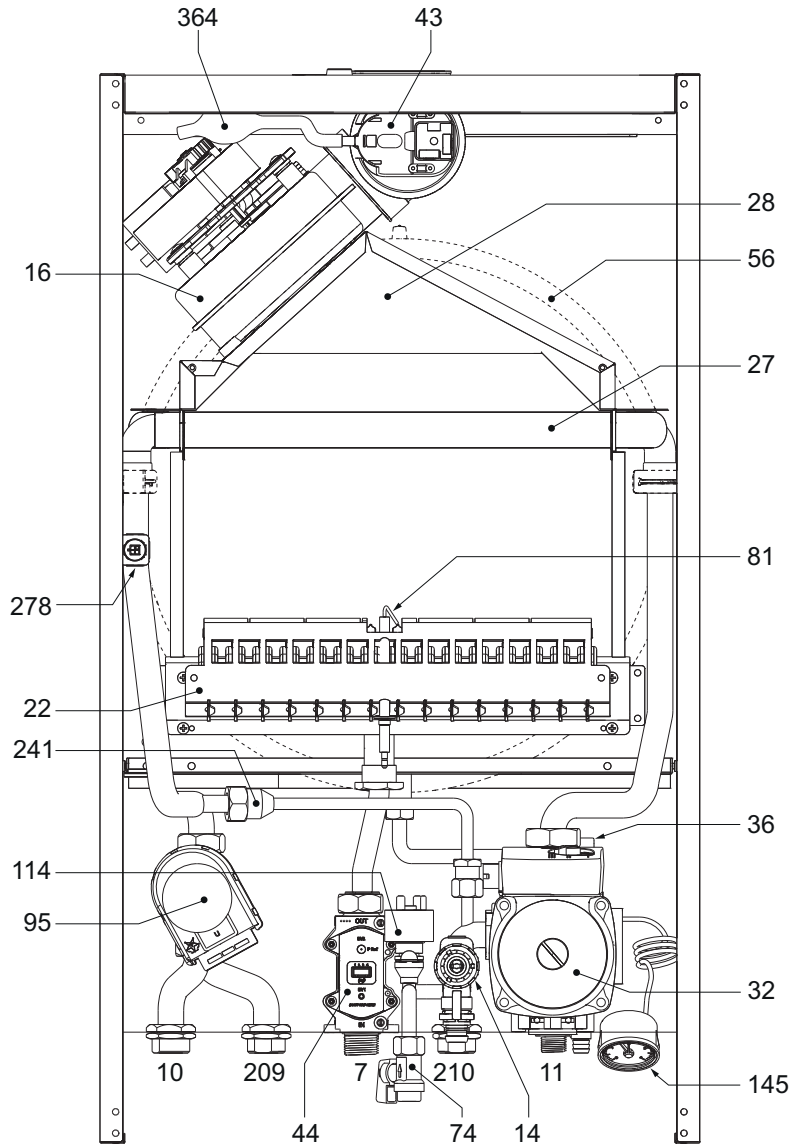
شكل 44 - منظر عام - DIVATOP D HF32
