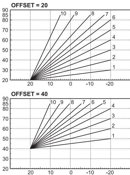
شكل 23 - مثال على النقل المتوازي لمنحنيات التعويض
