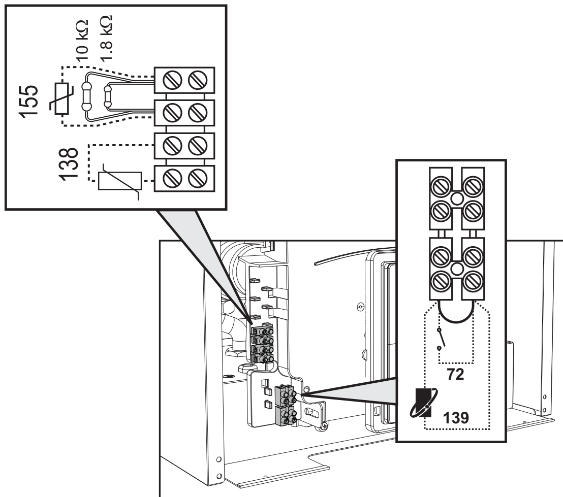
fig. 27- Accès au bornier
