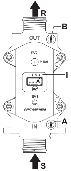
شكل 37 - صمام الغاز
