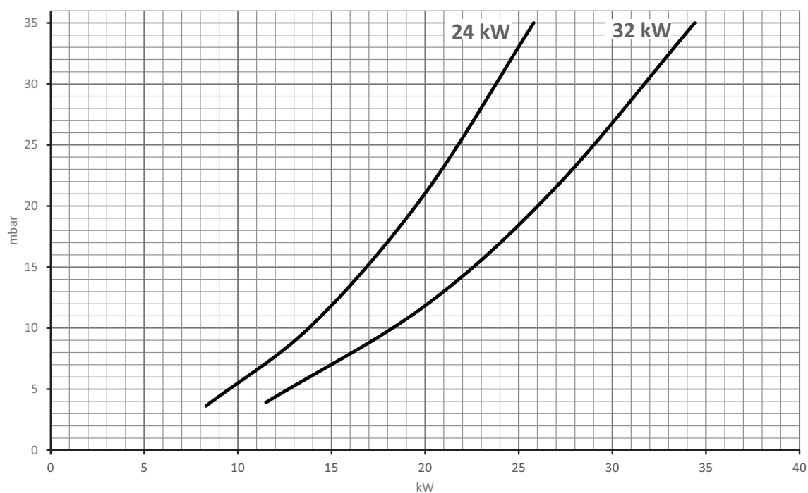
شكل 47 - مخطط للإصدارات العاملة بغاز البترول المسال
