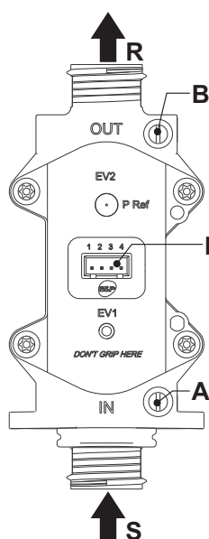
fig. 37 - Vanne à gaz
