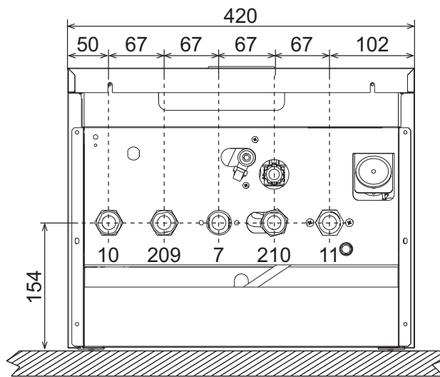
شكل 42 - أبعاد ووصلات الموديل DIVATOP D HF32
