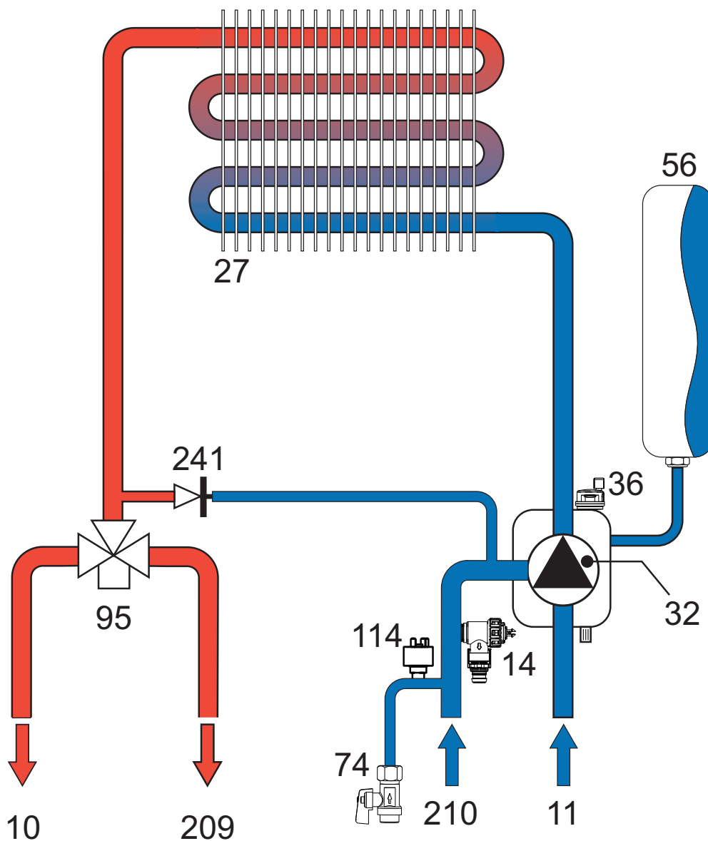
fig. 45- Circuit chauffage
