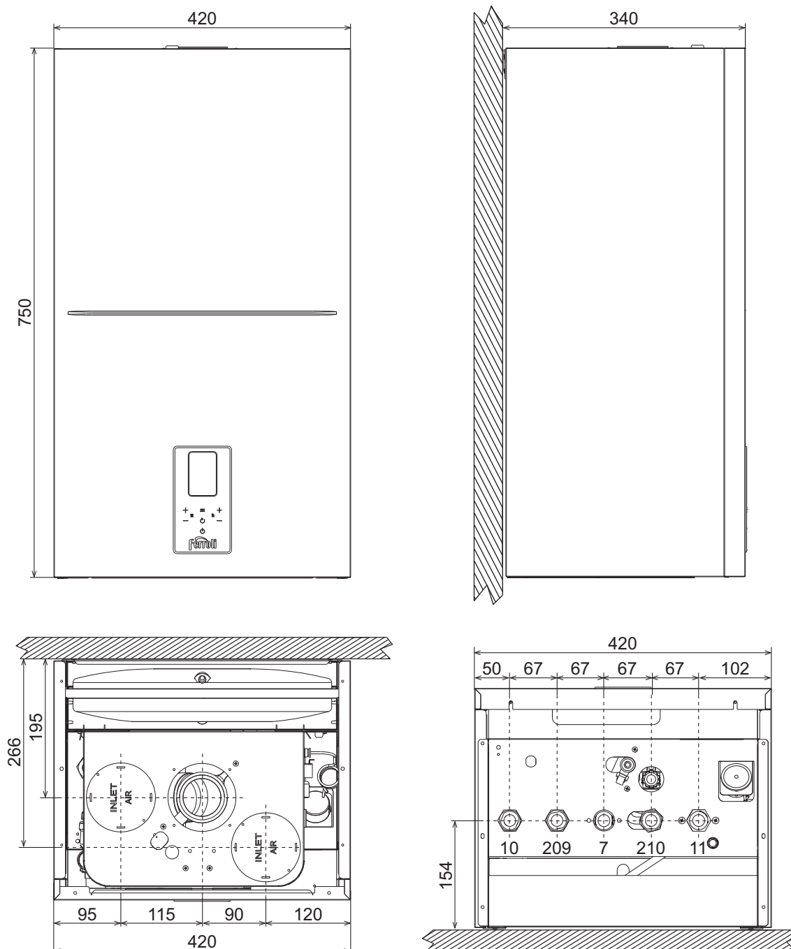
fig. 41- Dimensions et raccords modèle DIVATOP D HF24
