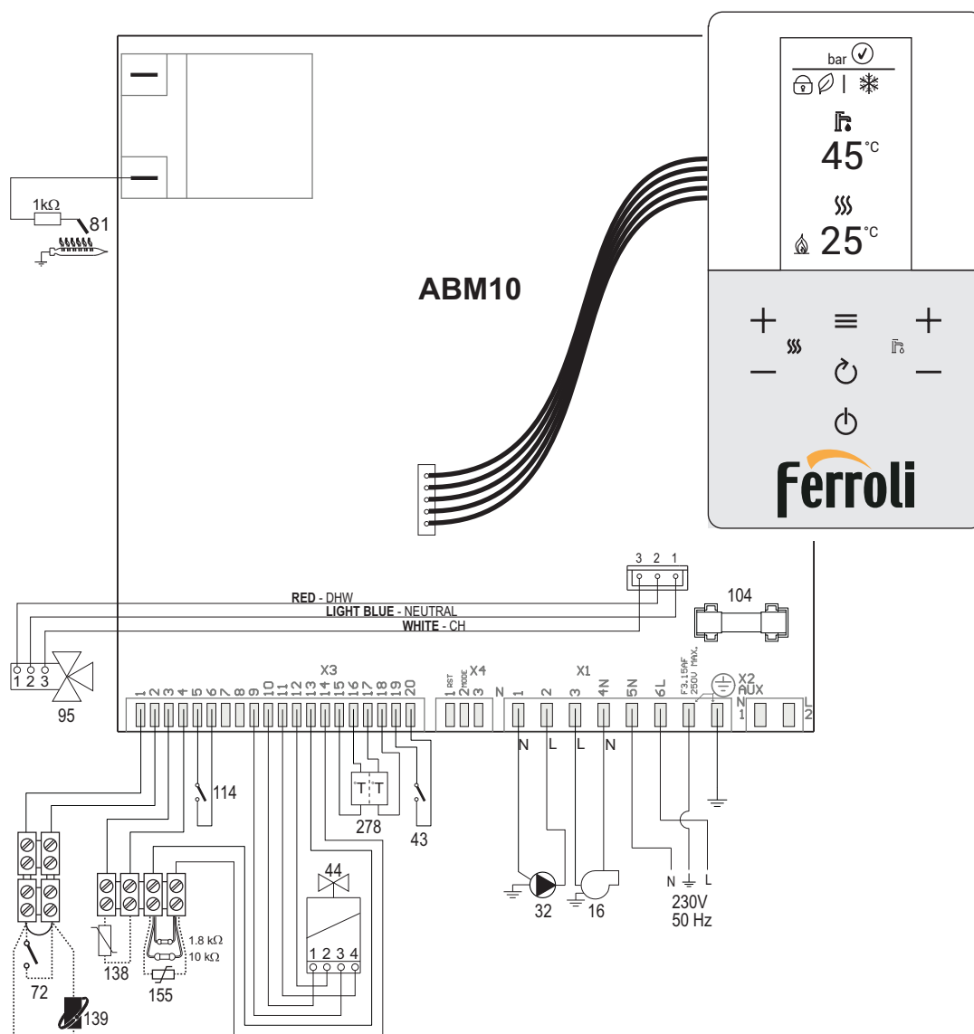
рис. 48- Электрическая схема
