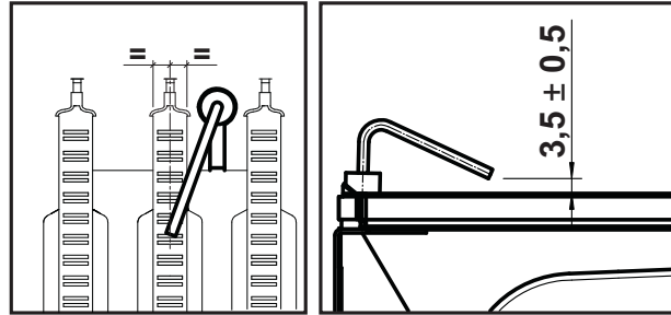
شكل 40 - وضع الإلكترود
