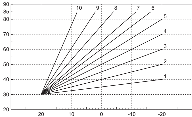
شكل 22 - منحنيات التعويض
