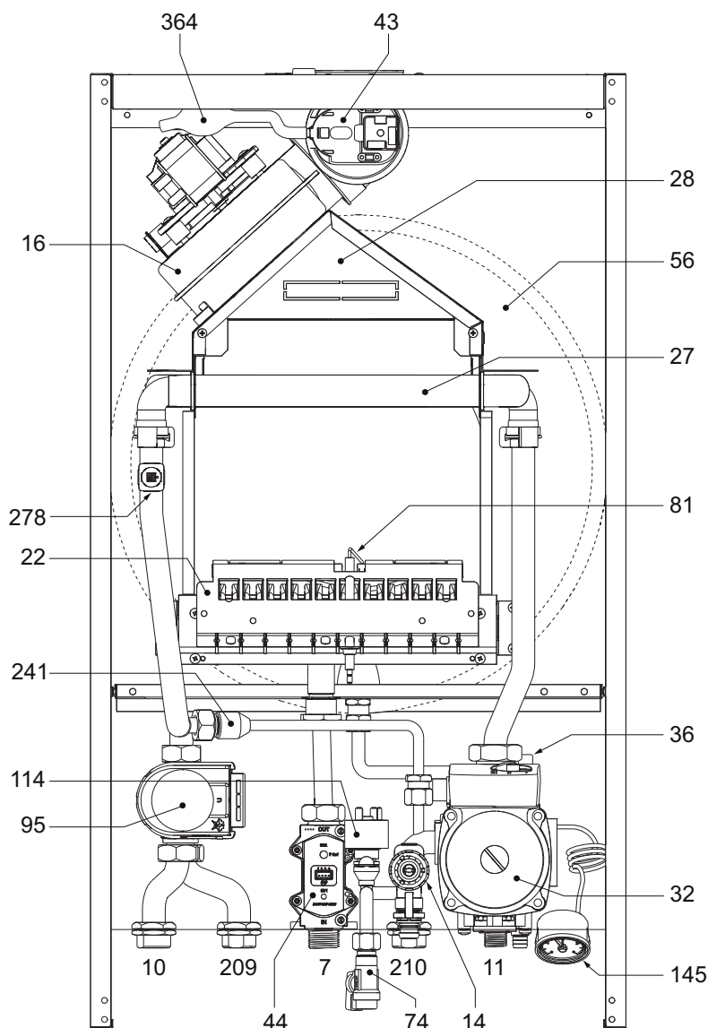
fig. 43- Vue générale - DIVATOP D HF24
