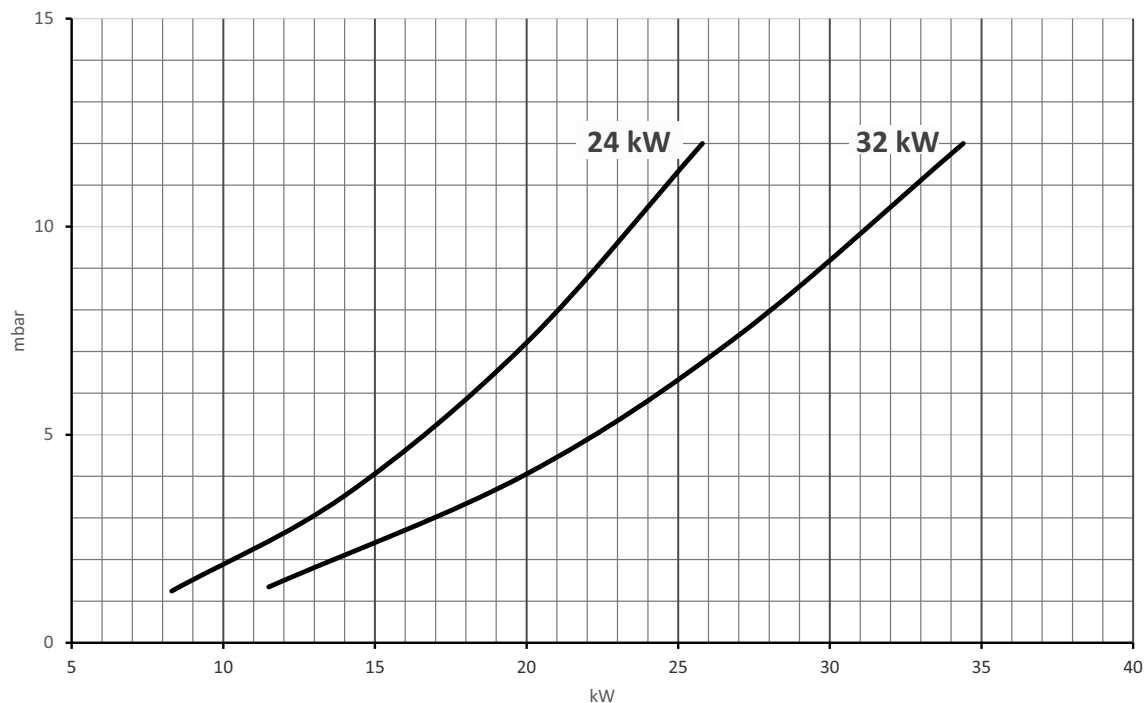
fig. 46- Diagramme pour versions au méthane
