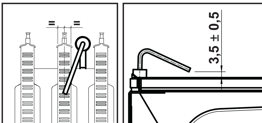
fig. 40- Mise en place de l'électrode
