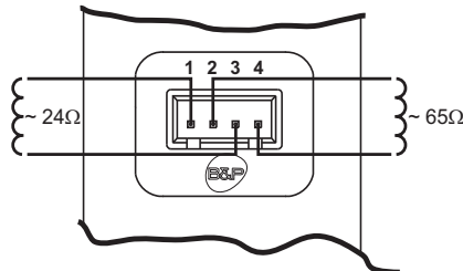
Slika 38- Priključak gasnog ventila
