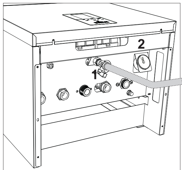
рис. 24- Кран для заливки воды
