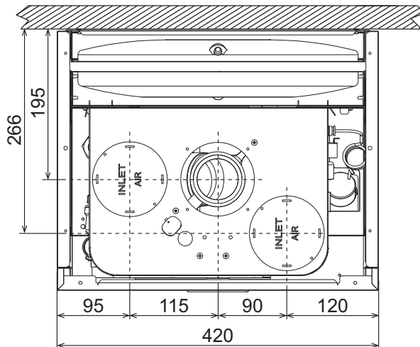
شكل 41 - أبعاد ووصلات الموديل DIVATOP D HF24
