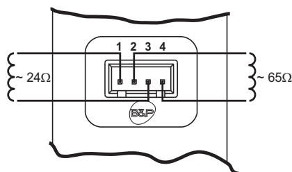
fig. 38 - Connexion soupape de gaz
