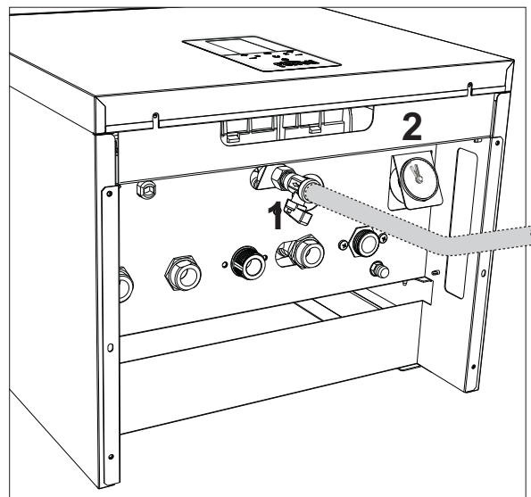
Slika 24- Slavina za punjenje
