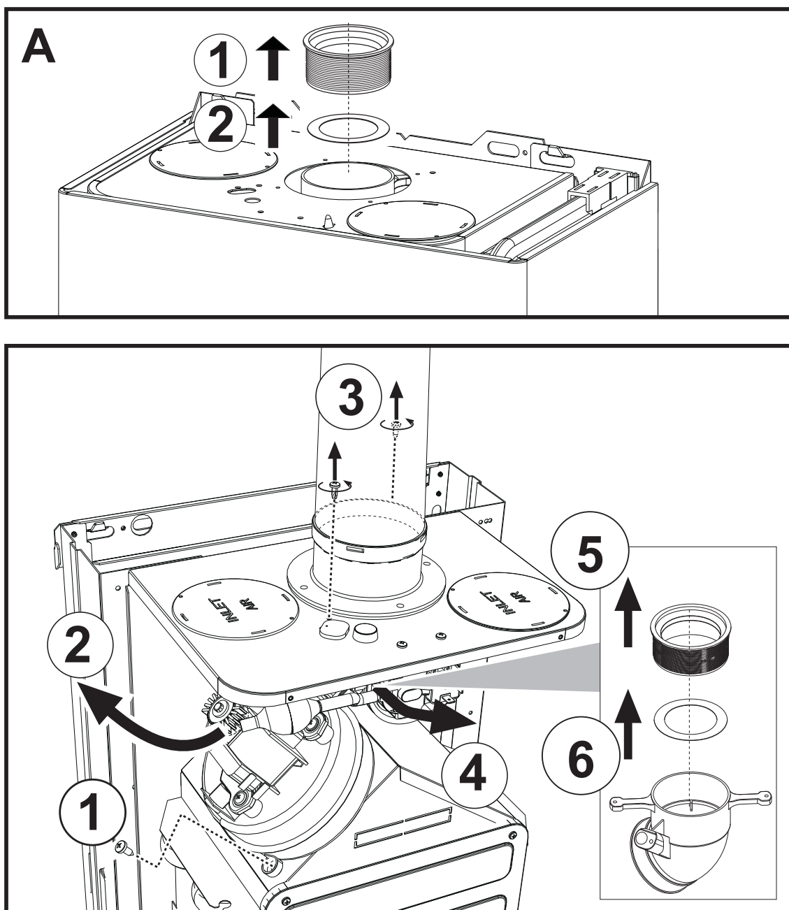
Slika 28- Zamena membrane
