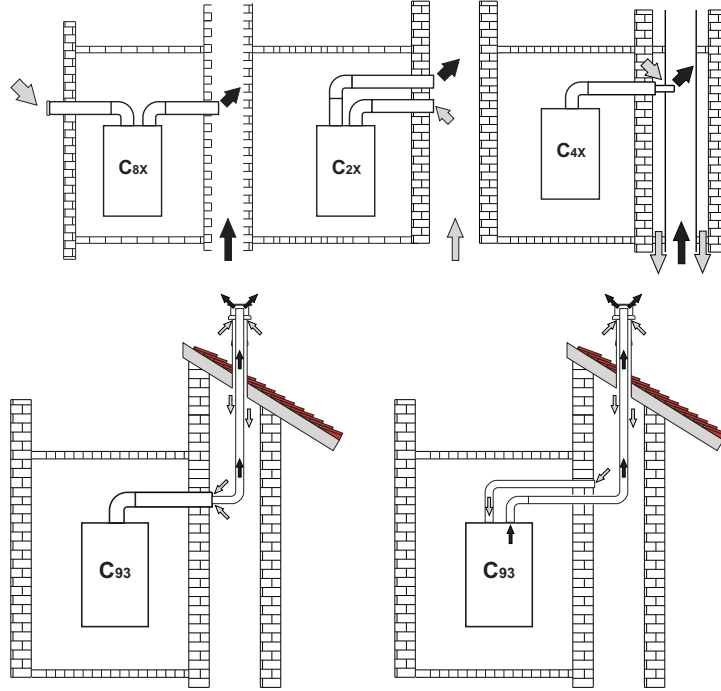
شكل 33 - أمثلة على التوصيل بالمدخن (الهواء / = الغادم)
