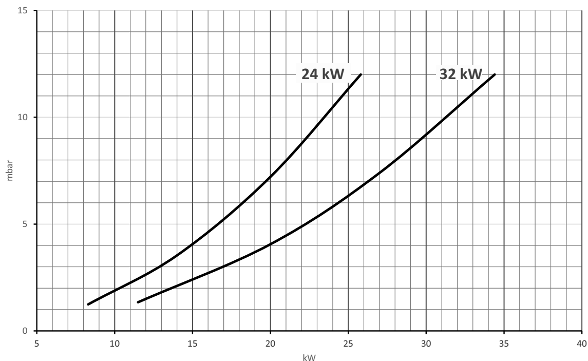
Slika 46- Dijagram za verzije na metan
