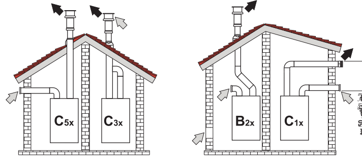
شكل 31 - أمثلة على التوصيل بالأنابيب المنفصلة (الهواء / العادم = العادم)
