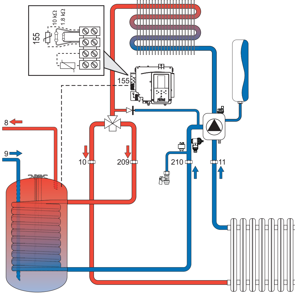
شكل 26 - مخطط التوصيل بسخان خارجي
