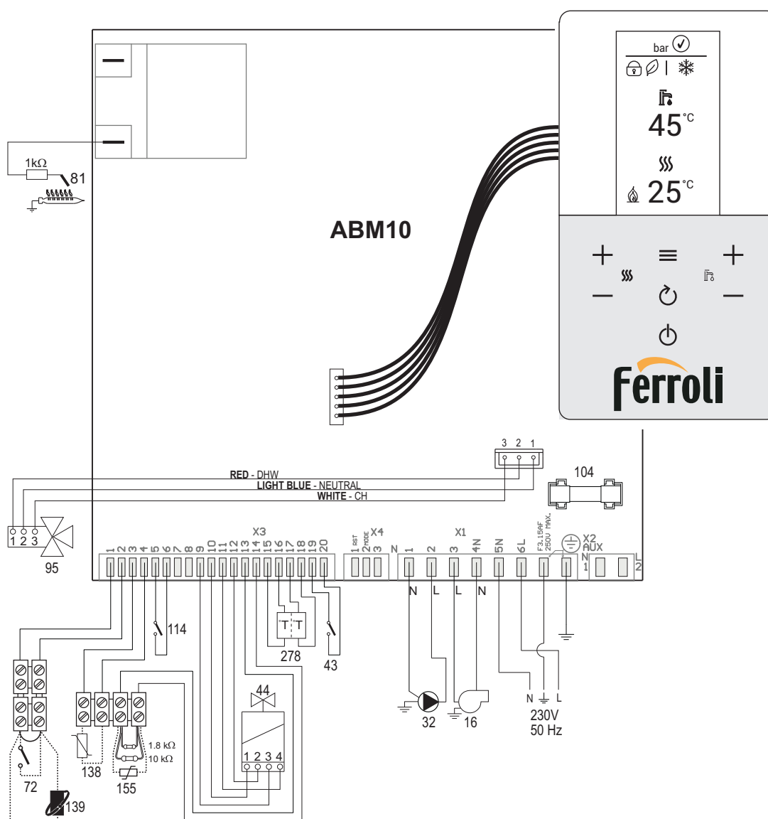
fig. 48- Schéma électrique
