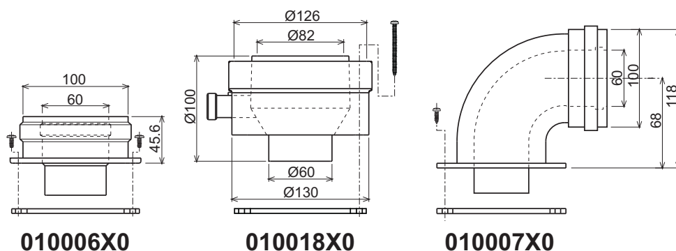
fig. 30- Accessoires de départ pour conduits coaxiaux
