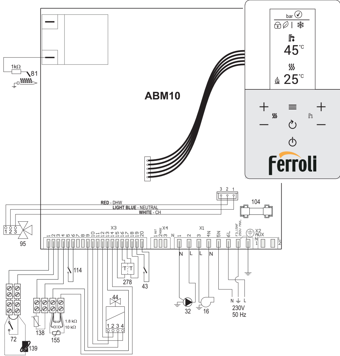
شكل 48 - المخطط الكهربائي
