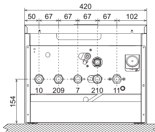
fig. 42- Dimensions et raccords modèle DIVATOP D HF32
