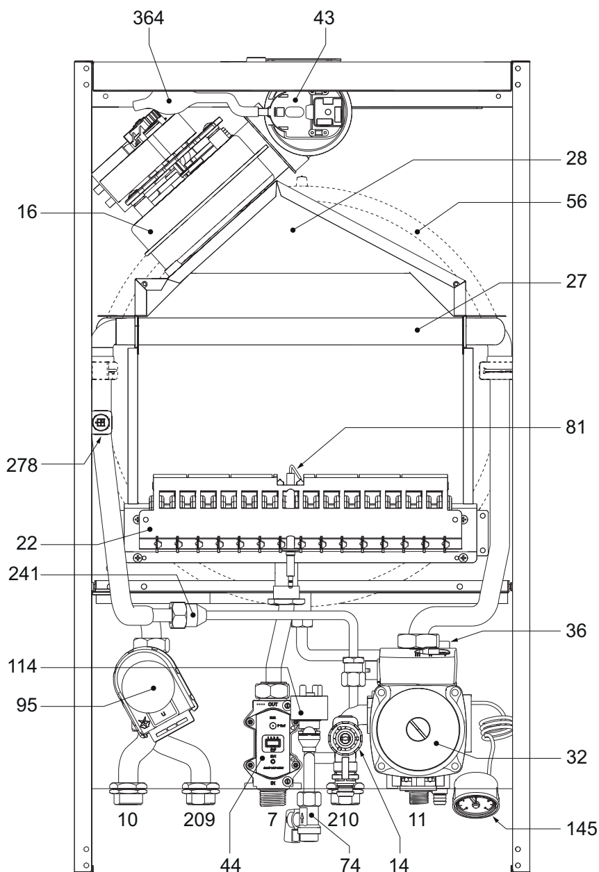
Slika 44- Opšti prikaz - DIVATOP D HF32
