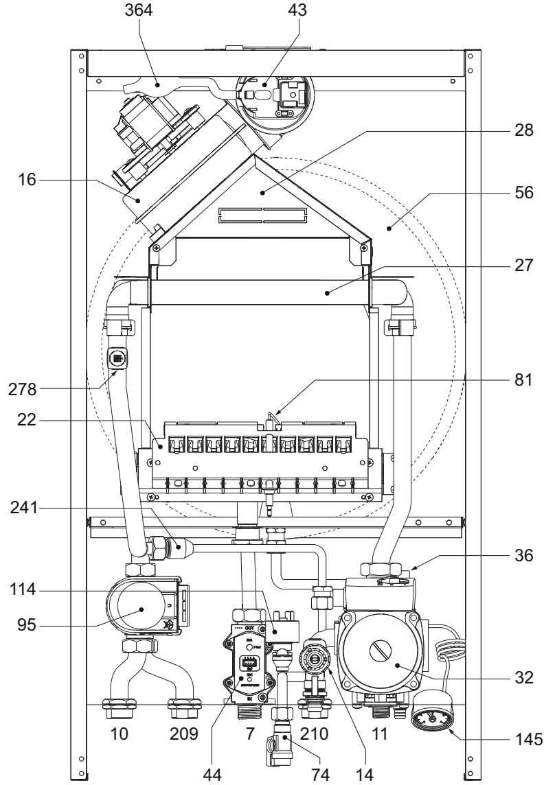
شكل 43 - منظر عام - DIVATOP D HF24
