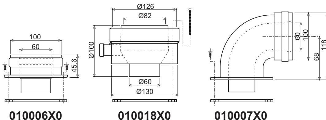
Slika 30- Početna oprema za koaksijalne vodove
