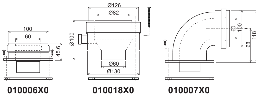
شكل 30 - ملحقات البدء للأنابيب متحدة المحور
