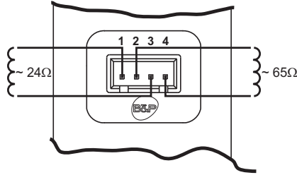
شكل 38 - توصيل صمام الغاز
