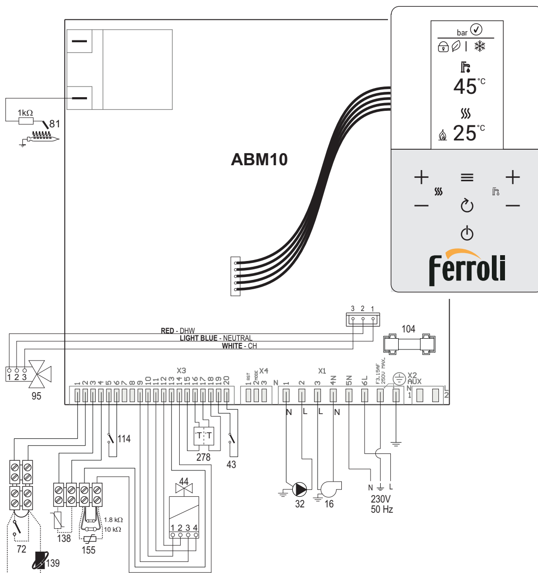
Slika 48- Električna šema
