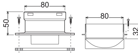
شكل 32 - ملحقات البدء الخاص بالأنابيب المنفصلة
