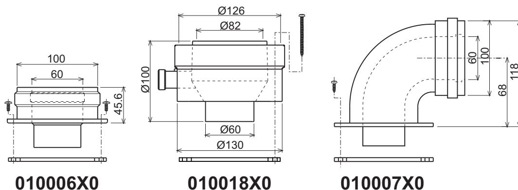
мал. 30- Початкові елементи для коаксіальних трубопроводів
