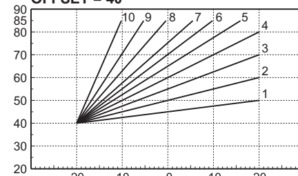
Slika 23- Primer paralelnog pomeranja krive kompenzacije
