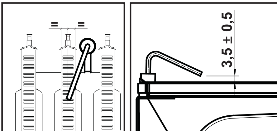
Slika 40- Pozicioniranje elektrode
