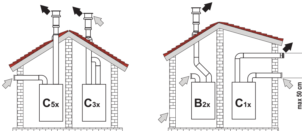
Slika 31- Primeri povezivanja sa odvojenim cevima (⇨ = Vazduh / ⇨ = Dimni gasovi)
