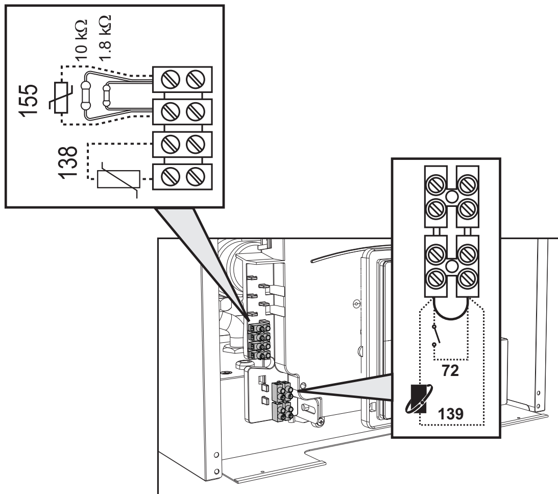
рис. 27- Доступ к клеммной колодке
