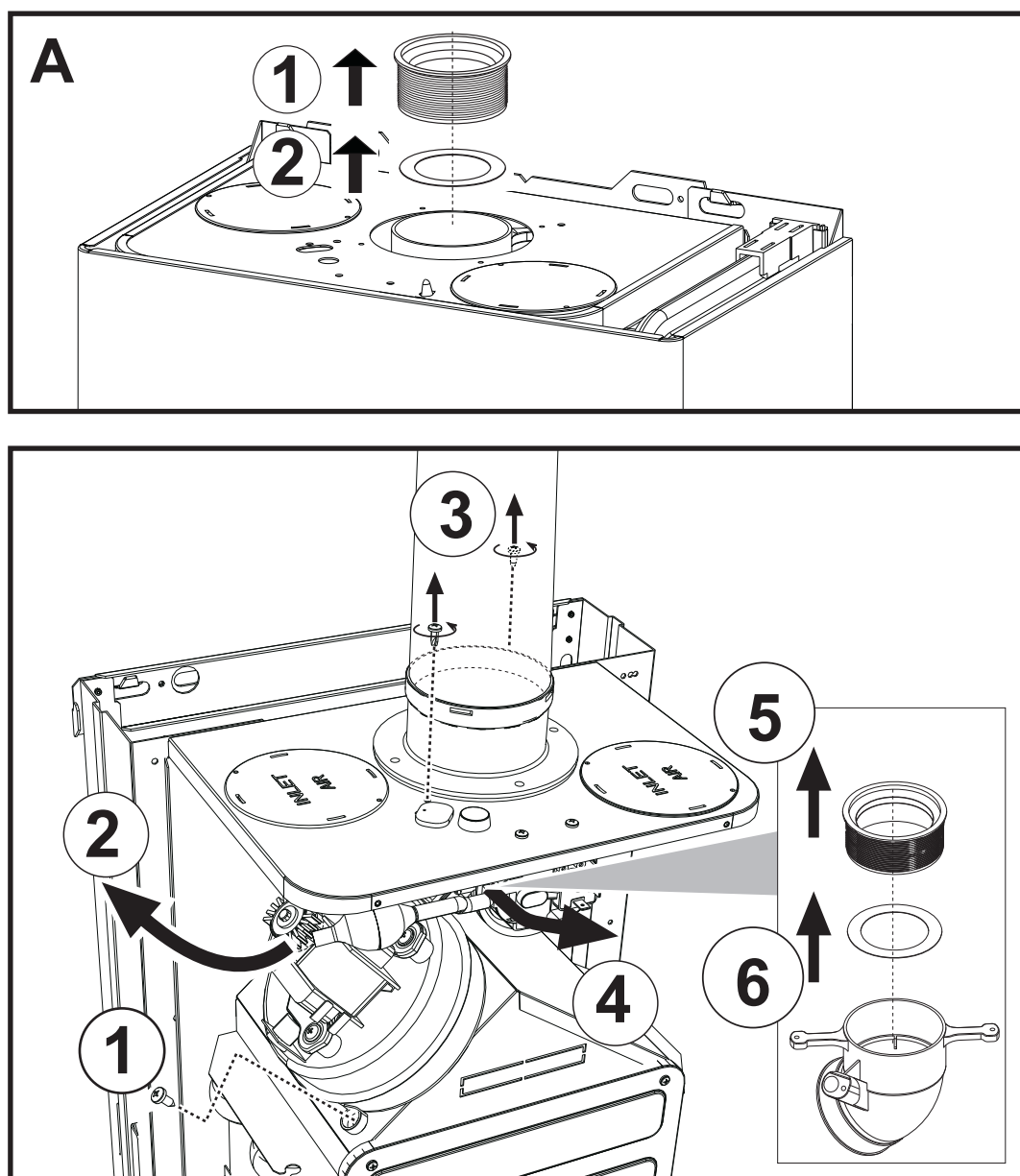
рис. 28- Замена диафрагмы
