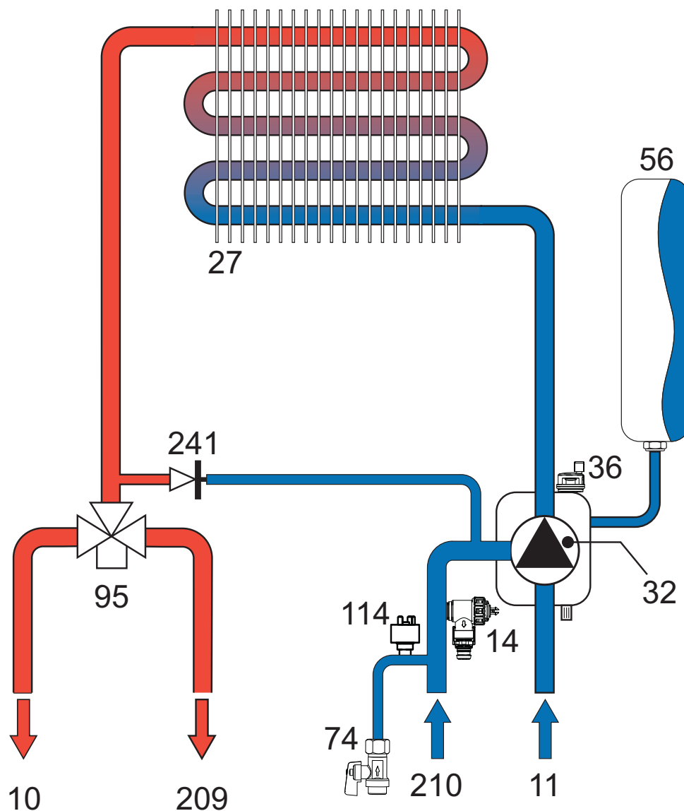
рис. 45- Контур отопления
