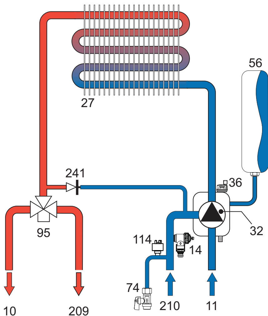
شكل 45 - دائرة التدفئة
