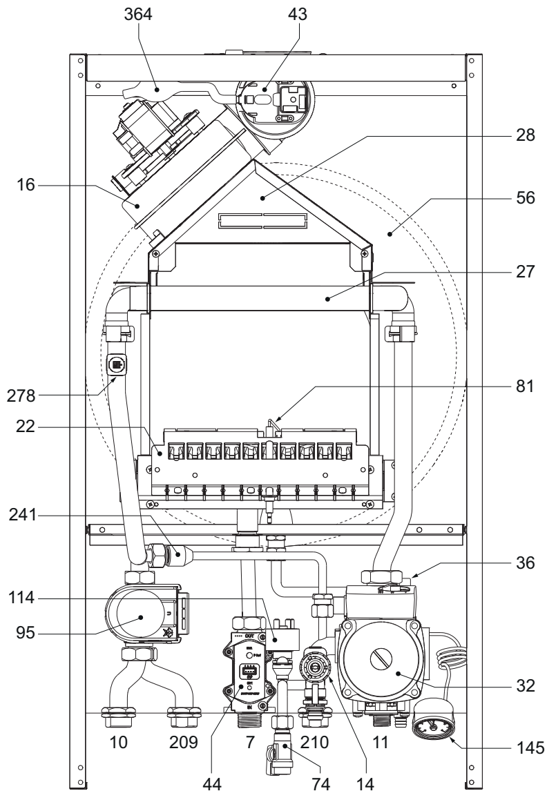
рис. 43- Общий вид - DIVATOP D HF24
