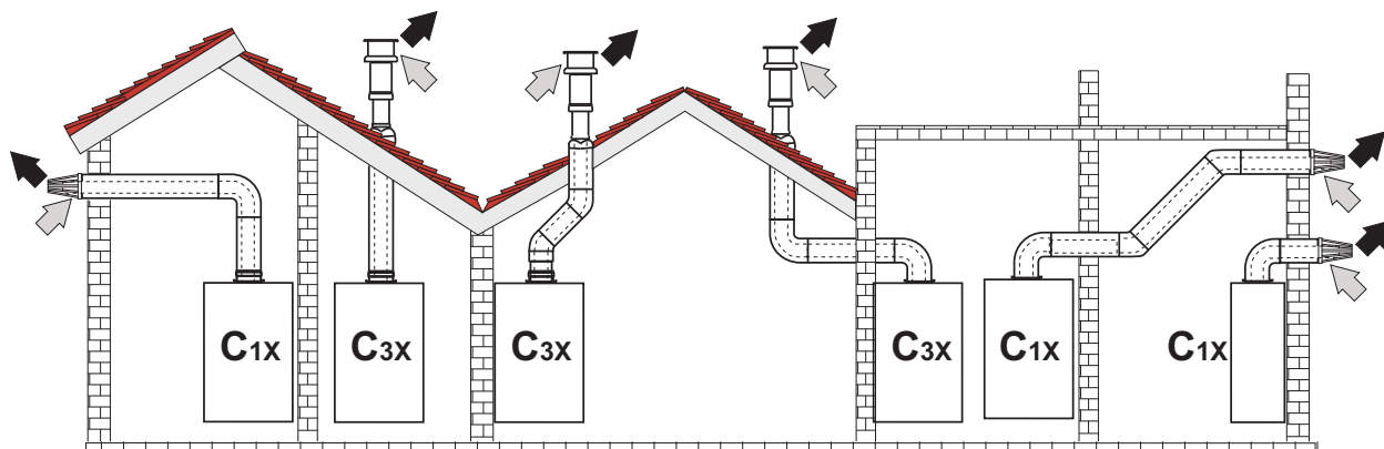
fig. 29- Exemples de raccordement avec tubes coaxiaux (⇐ = Air / ⇨ = Fumées)
