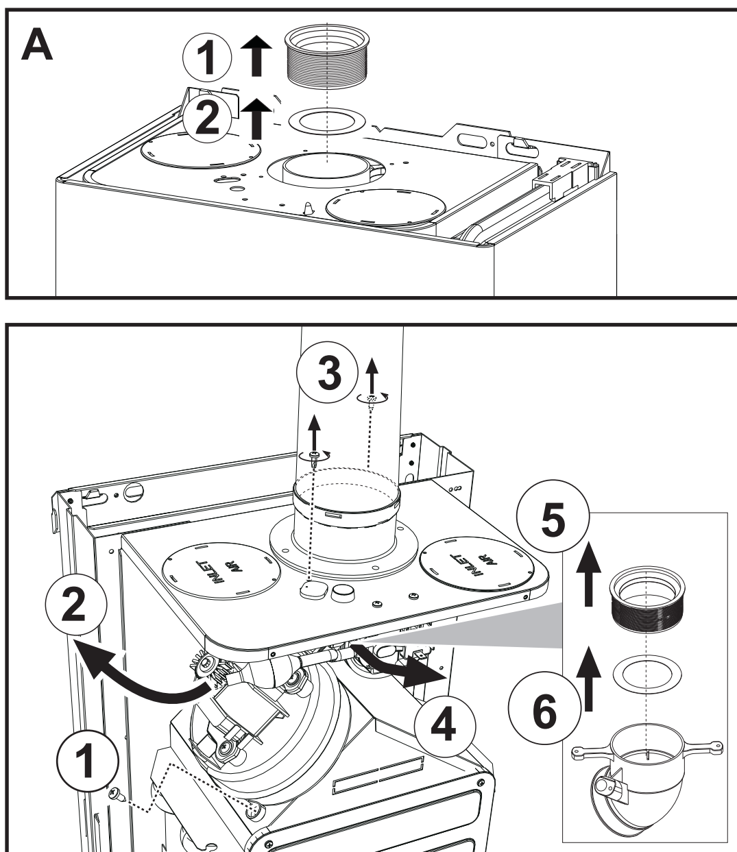
fig. 28- Remplacement du diaphragme
