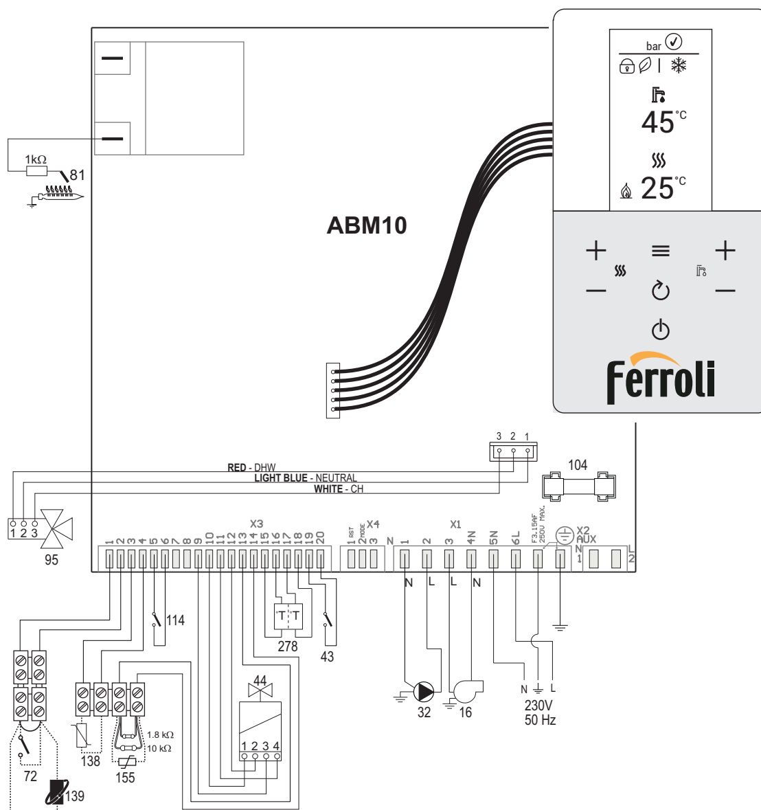
мал. 48- Електрична схема
