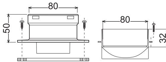
fig. 32 - Accessoire de départ pour conduits séparés
