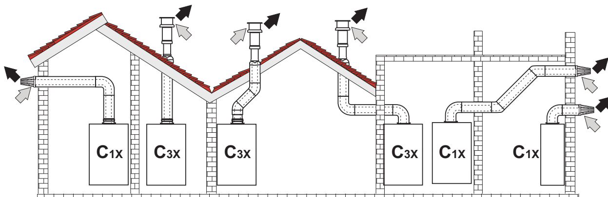
شكل 29 - أمثلة على التوصيل بالأنابيب متحدة المحور (الهواء / العادم = العادم)
