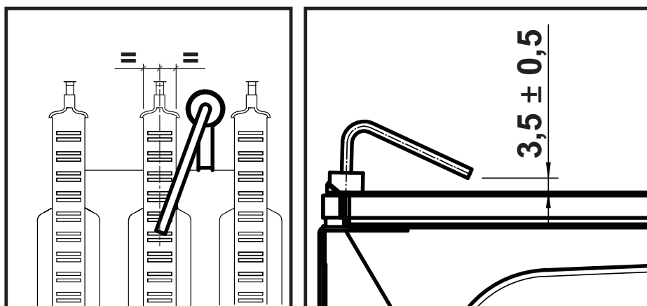
рис. 40- Расположение электрода
