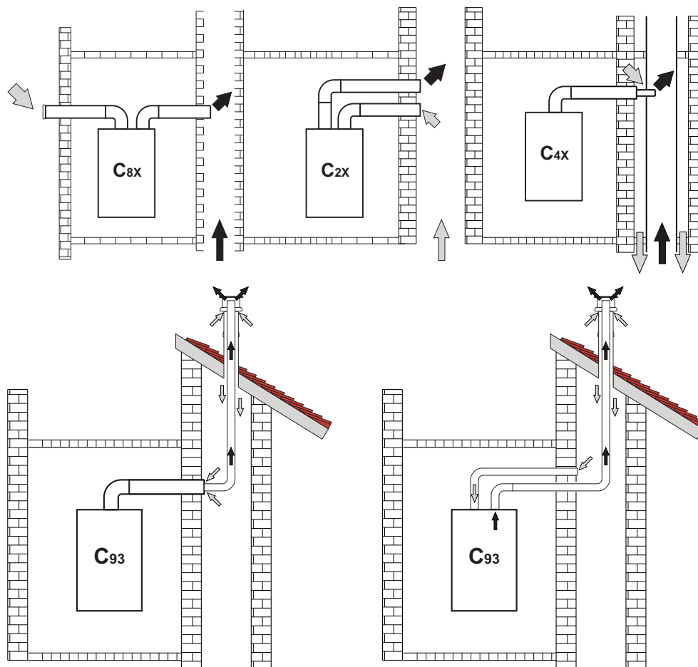
рис. 33 - Примеры подсоединения к дымоходам (⇐ = Воздух / ➡ = Дымовые газы)
