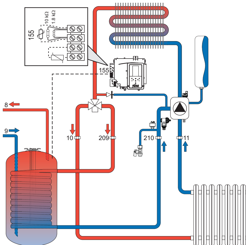
Slika 26- Šema za povezivanje na spoljni grejač
