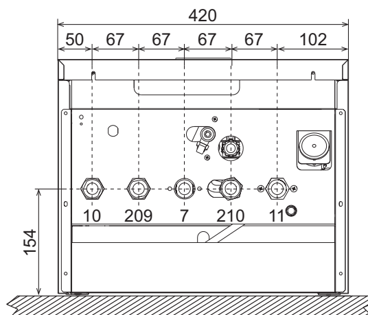
Slika 42- Dimenzije i nastavci modela DIVATOP D HF32
