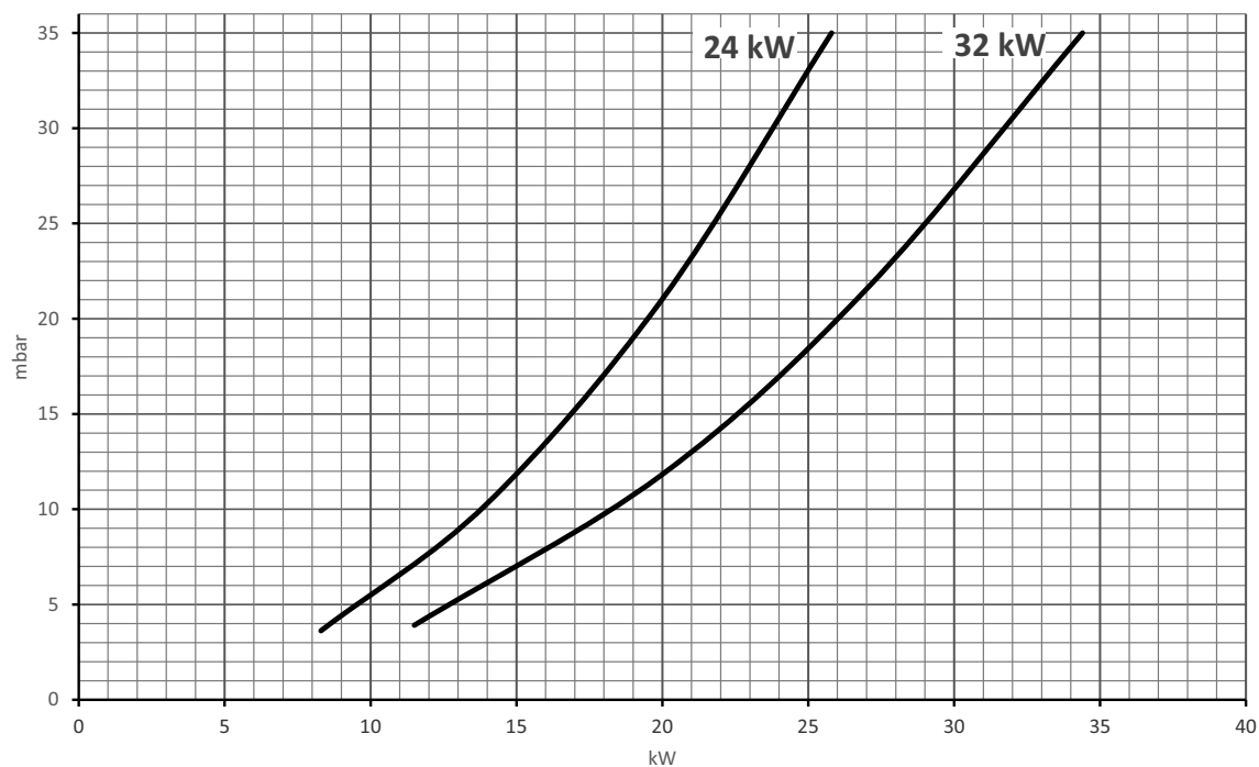
fig. 47- Diagramme pour versions au G.P.L
