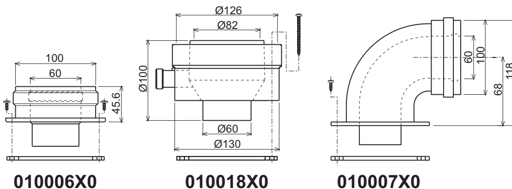
рис. 30- Исходные принадлежности для коаксиальных труб
