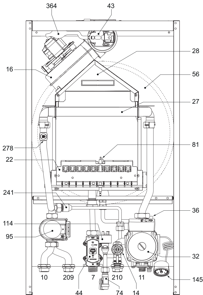
Slika 43- Opšti prikaz - DIVATOP D HF24
