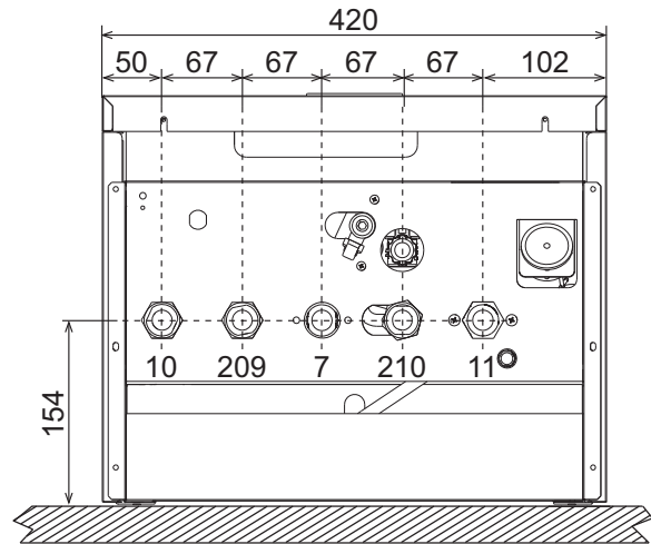
شكل 41 - أبعاد ووصلات الموديل DIVATOP D HF24
