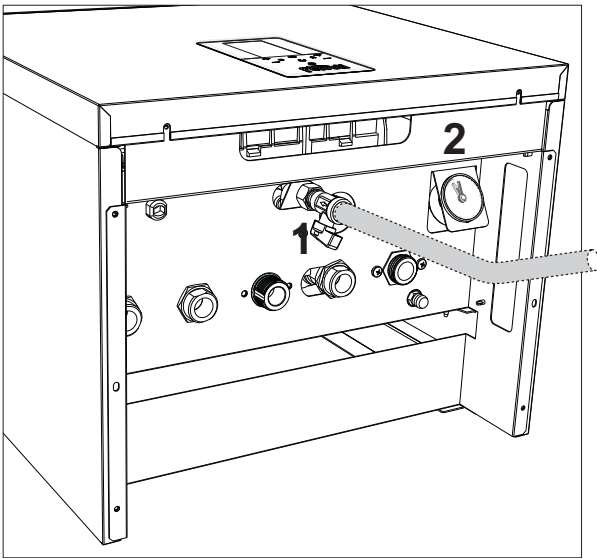
شكل 24 - صنبور الماء
