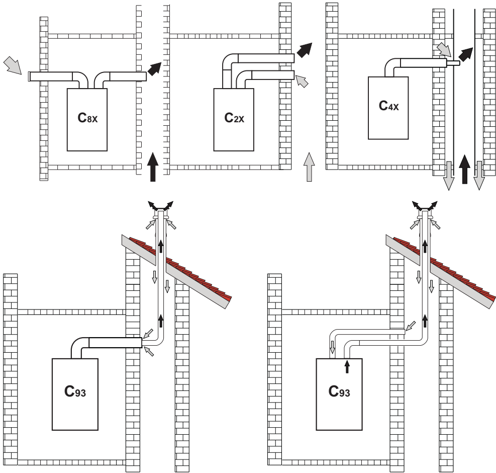
fig. 33 - Exemples de raccordement aux carnaux de fumées (⇨ = Air / ⇨ = Fumées)
