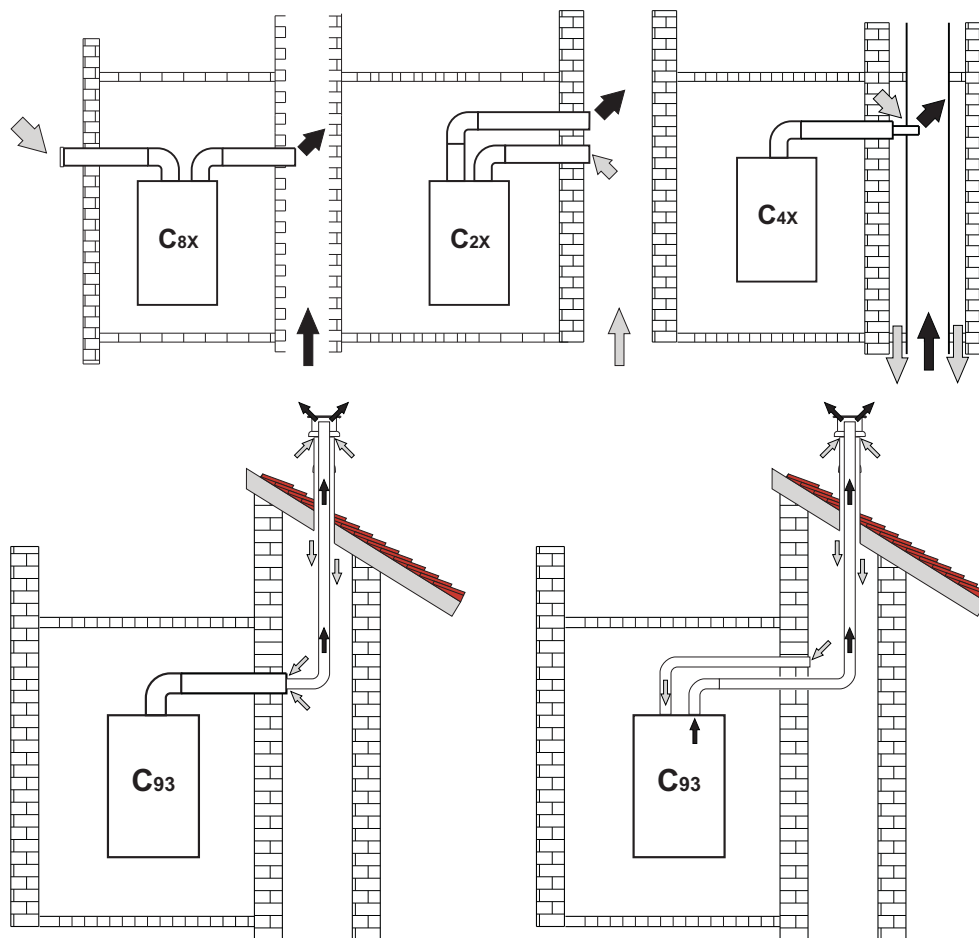
Slika 33- Primeri spajanja na dimovodne cevi (⇐ = Vazduh / ➡ = Dimni gasovi)
