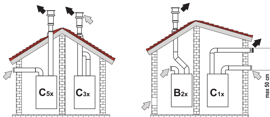
fig. 31 - Exemples de raccords avec des conduits séparés (⇨ = Air / ⇨ = Fumées)
