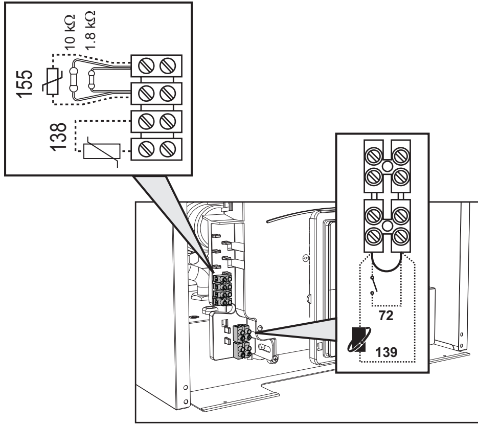
شكل 27 - الوصول إلى كتلة التوصيل الطرفية
