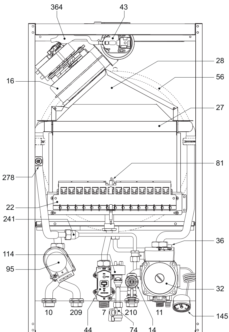
fig. 44- Vue générale - DIVATOP D HF32
