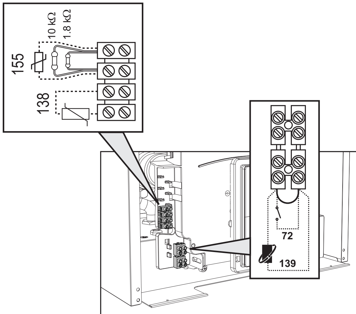
Slika 27- Pristup rednoj stezaljci
