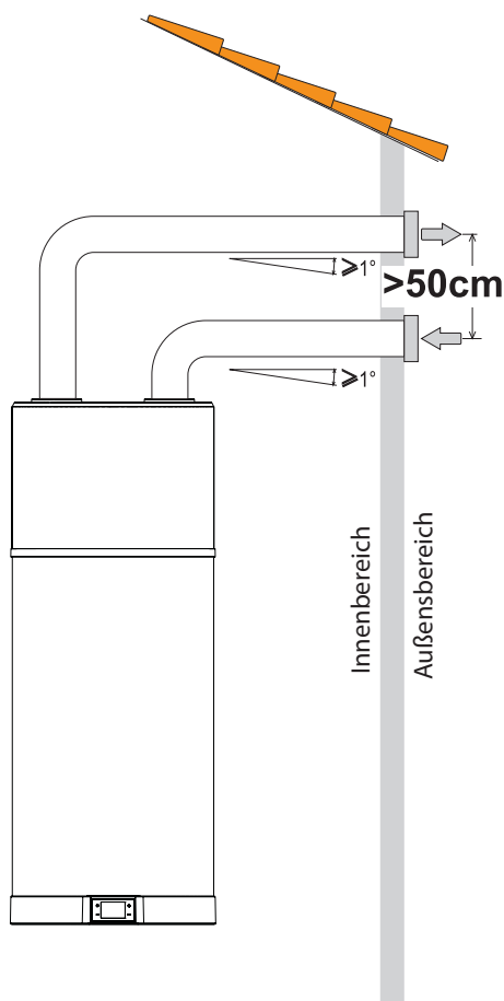
Abb. 54 - Beispiel für einen Luftauslassanschluss
