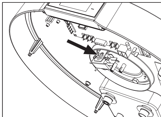
afb. 66 - Herstellen van de veiligheidsthermostaat
