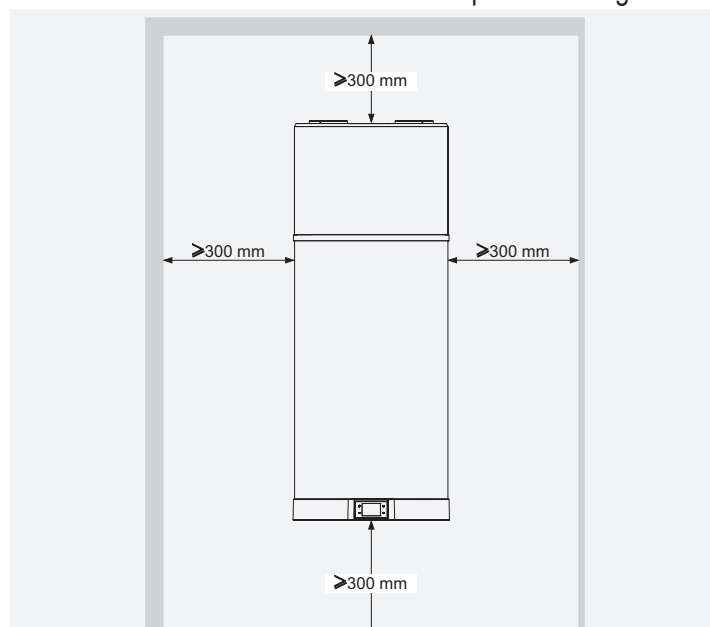
fig. 49 - Espaces minimum
