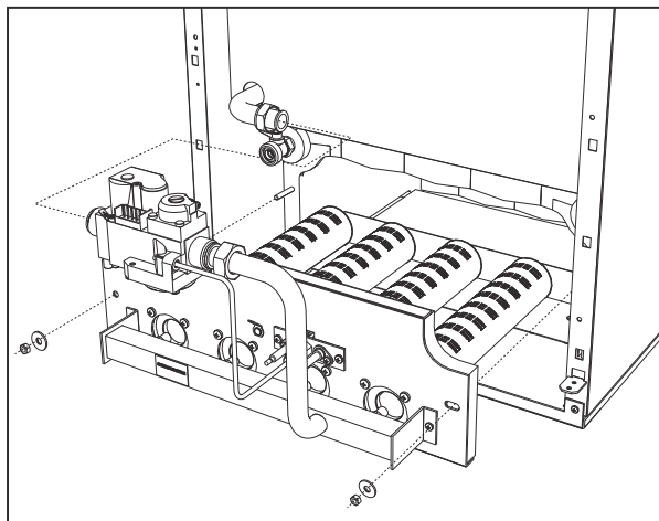
рис. 20 - Демонтаж горелок
