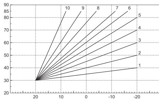
fig. 11 - Courbes de compensation
