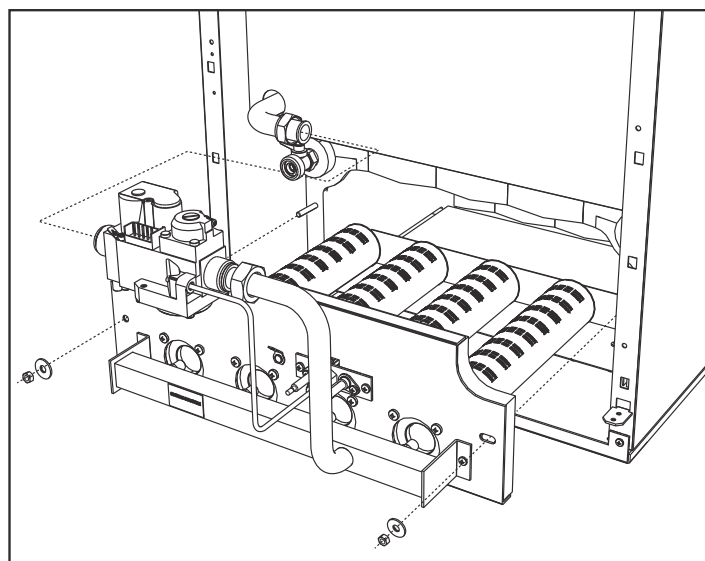
fig. 20 - Smontaggio bruciatori
