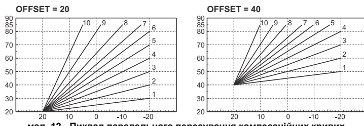
мал. 12 - Пиклад паралельного пересування компенсаційних кривих
