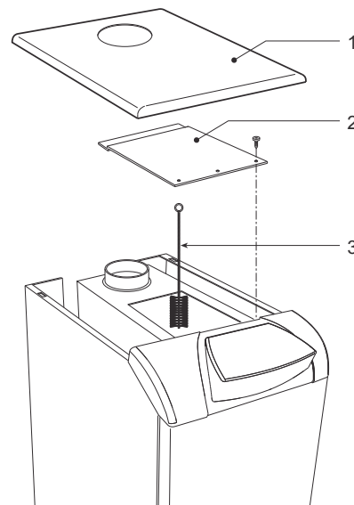
fig. 19 - Pulizia caldaia
