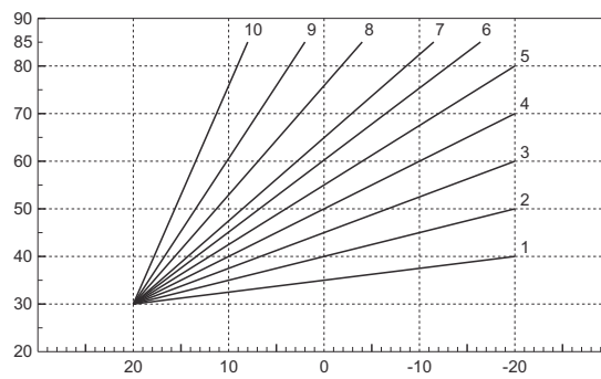
мал. 11 - Крива стиснення
