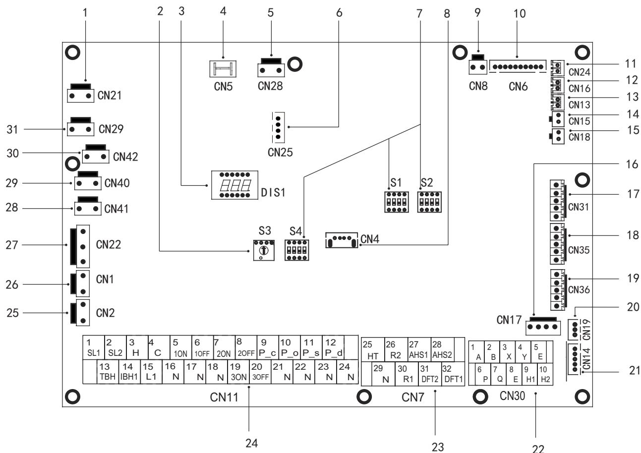
fig. 34 - Dettaglio scheda idronica pompa di calore
