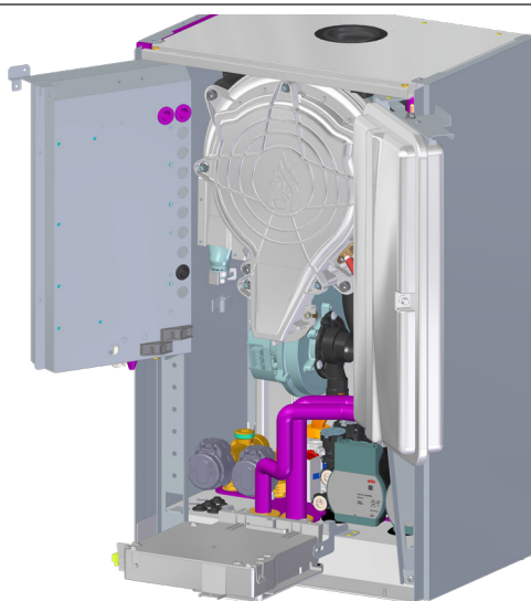
fig. 51 - accesso ai componenti interni
