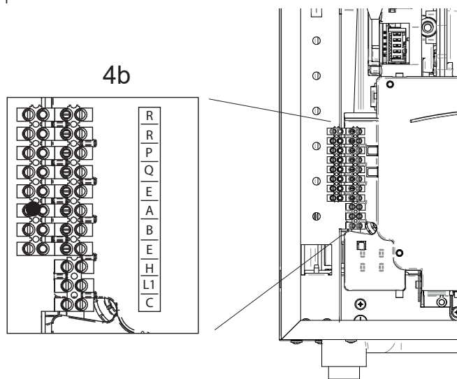
fig. 29 - Morsettiere utente
