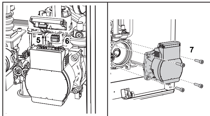
fig. 52 - Sostituzione/manutenzione circolatore della pompa di calore
