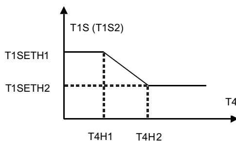
fig. 46 - Curva climatica 9 in modo riscaldamento
