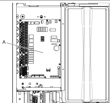
fig. 33 - scheda idronica pompa di calore
