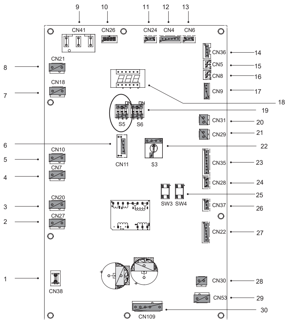
fig. 45 - Posizione del dip Switch S5 su scheda elettronica del circuito frigorifero
