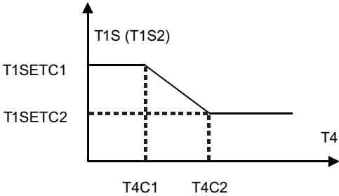
fig. 47 - Curva climatica 9 in modo raffreddamento
