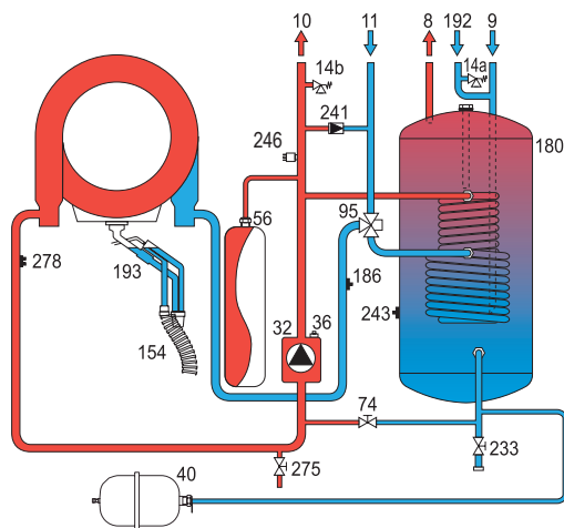
fig. 45 - Circuito idraulico
