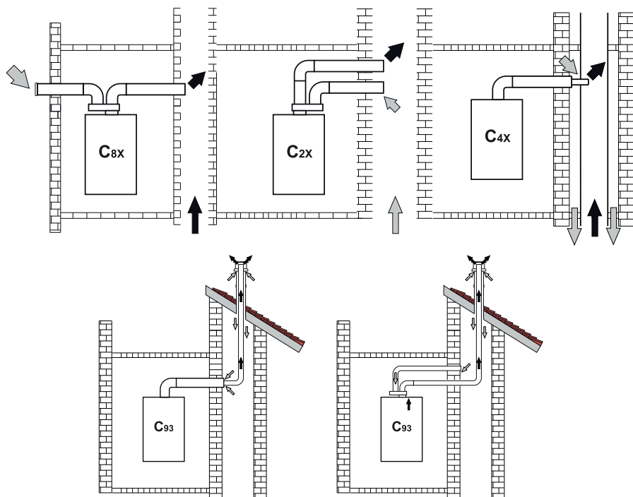
fig. 35 - Exemples de raccordement à carnaux de fumées ( = Air / = Fumées )
