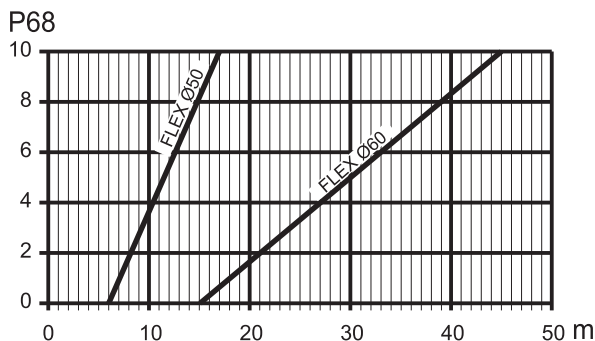
fig. 34 - Graphique pour la sélection du paramètre cheminée
