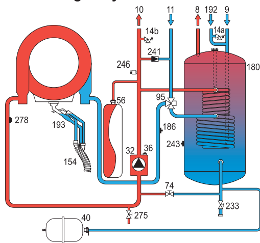
fig. 45 - Obieg wody
