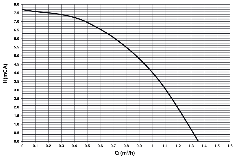
fig. 46 - Reszkowa wysokość podnoszenia dostępna dla instalacji
