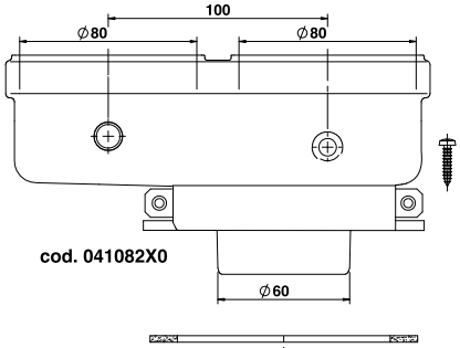
fig. 32 - Accessoire de départ pour conduits séparés
