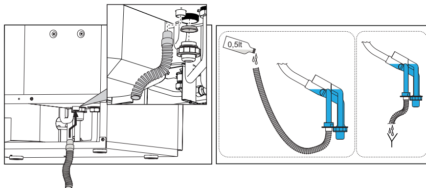
fig. 36 - Raccordement de l'évacuation des condensats
