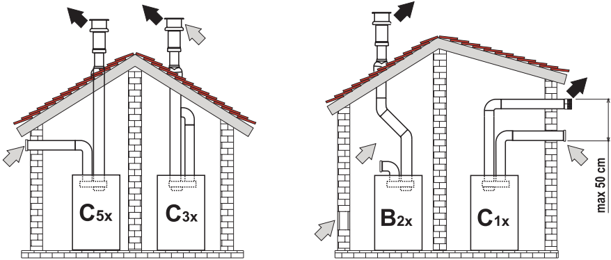
fig. 31 - Ejemplos de conexión con tubos separados ( ➡ = aire / ➡ = humos)
