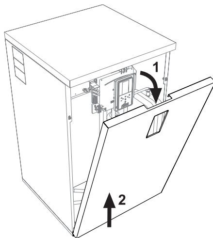
fig. 40 - Ouverture du panneau avant
