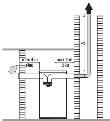
fig. 33 - Esquema solo para entubamiento con flexible
