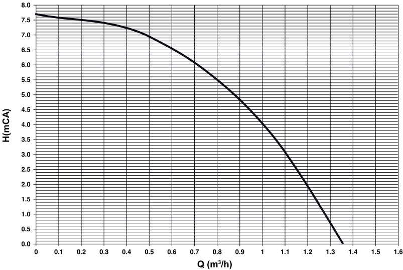
fig. 46 - Hauteur d'élévation résiduelle disponible à l'installation
