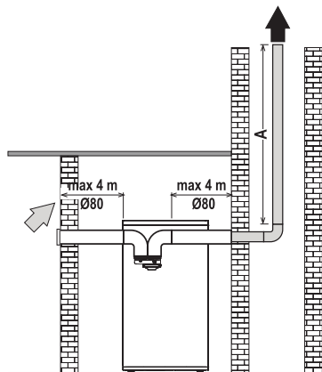
fig. 33 - Schéma pour tubage réalisé seulement avec un conduit souple
