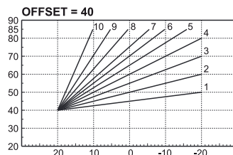
fig. 25 - Exemple de déplacement parallèle des courbes de compensation
