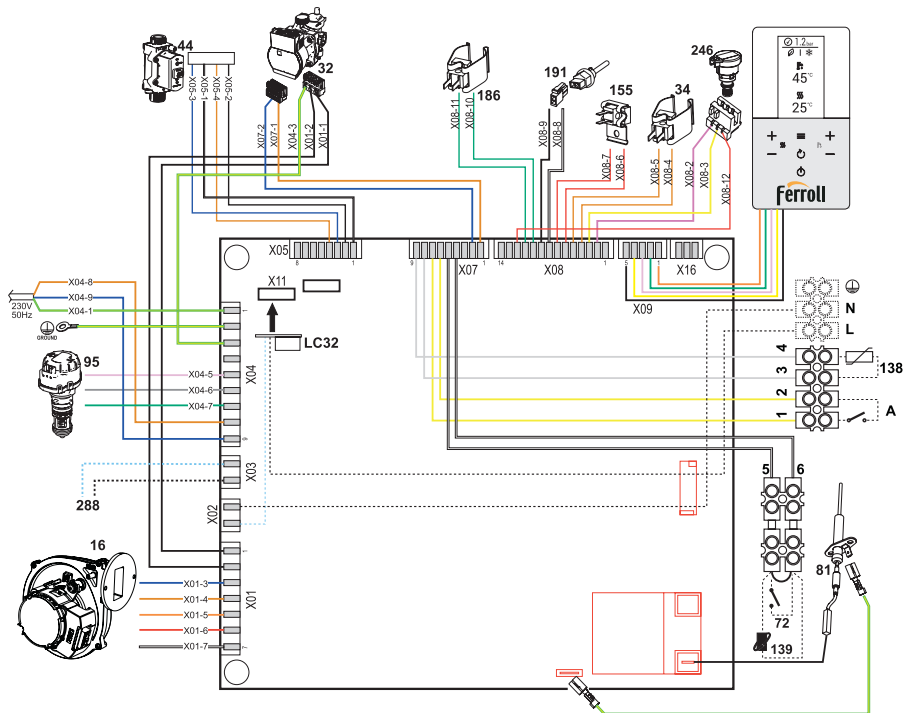
fig. 47 - Schemat elektryczny
