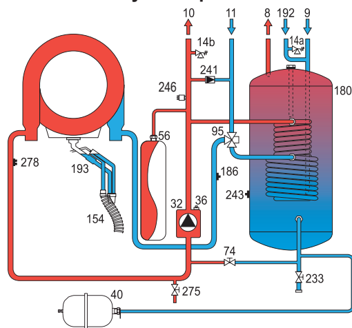
fig. 45 - Circuit hydraulique
