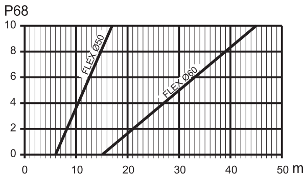
fig. 34 - Wykres wyboru parametrów komina
