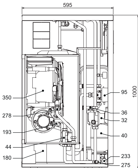
fig. 42 - Widok z boku
