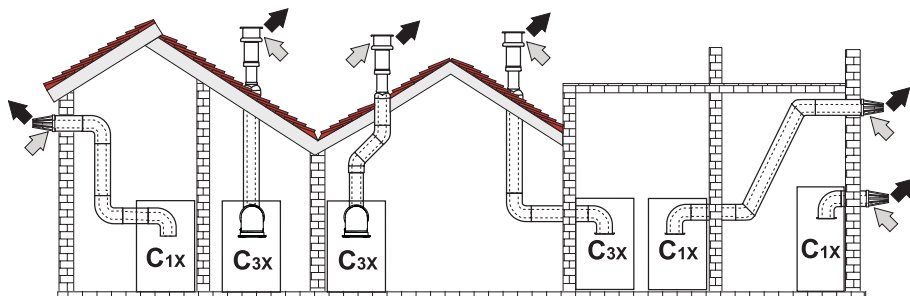
fig. 29 - Exemples de raccordement avec des tuyaux coaxiaux ( → = Air / → = Fumées)
