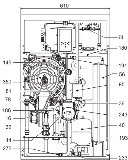
fig. 41 - Widok z przodu
