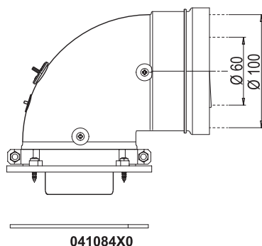
fig. 30 - Accessoires de départ pour conduits coaxiaux
