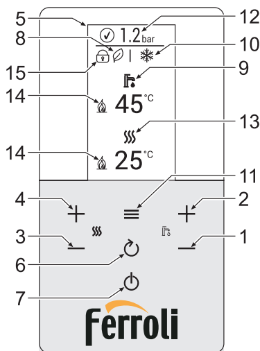
fig. 1 - Tableau de commande
