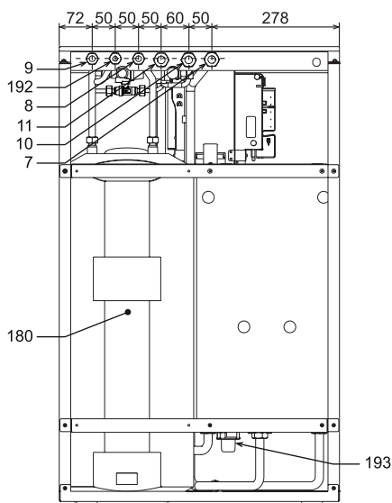
fig. 43 - Widok z tyłu
