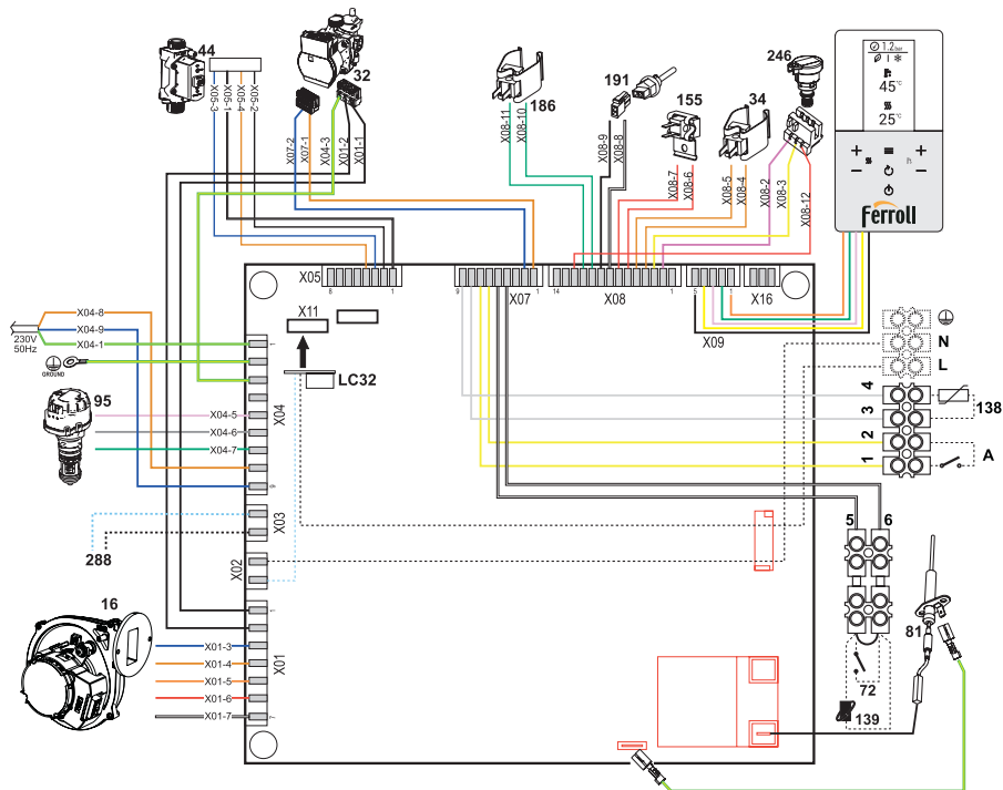
fig. 47 - Schema elettrico
