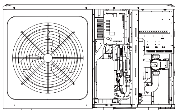
Σύστημα ψυκτικού
