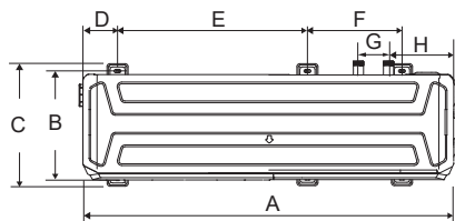
4/6 kW (μονάδα: mm)
