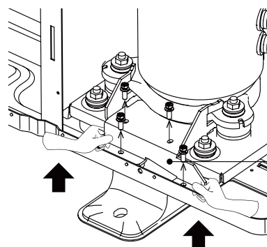
Αφαιρέστε το στήριγμα μεταφοράς
