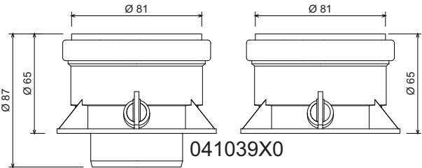
рис. 18 - Соединительный элемент для раздельных труб
