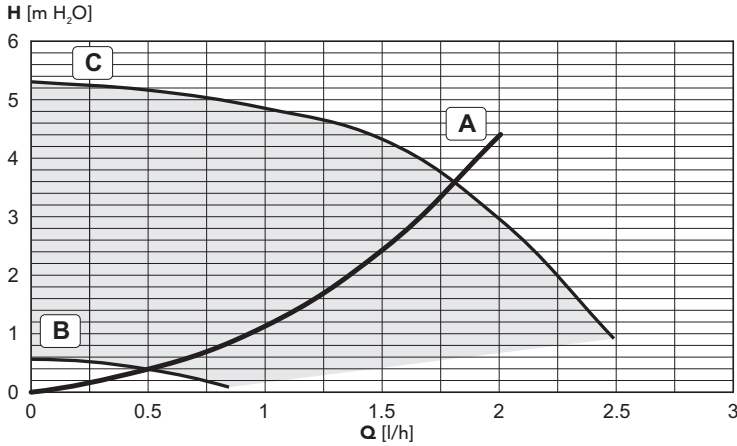
şek. 28 - Sirkülatör yük / basınç kayıpları BLUEHELIX TECH 25 C
