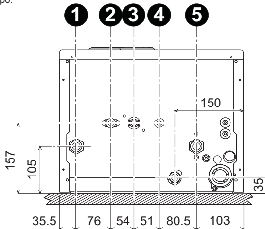
fig. 13 - Conexiones hidráulicas
