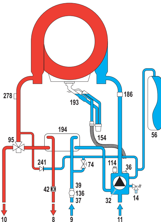
fig. 27 - Circuit hydraulique
