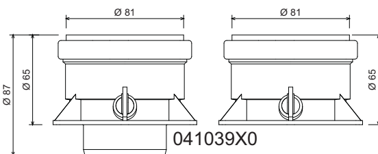
мал. 18 Початковий елемент для відокремлених трубопроводів
