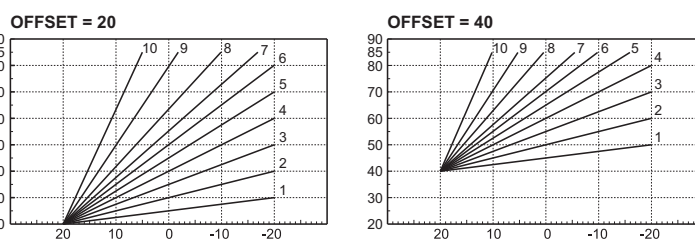
рис. 11 - Пример параллельного смещения компенсационных характеристик
