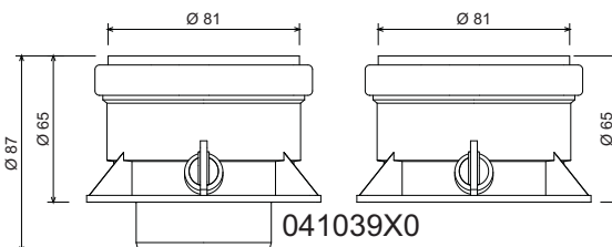
fig. 18 - Accessoire de départ pour conduits séparés
