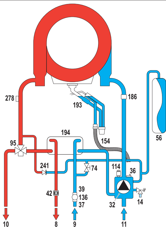
fig. 27 - Circuito hidráulico
