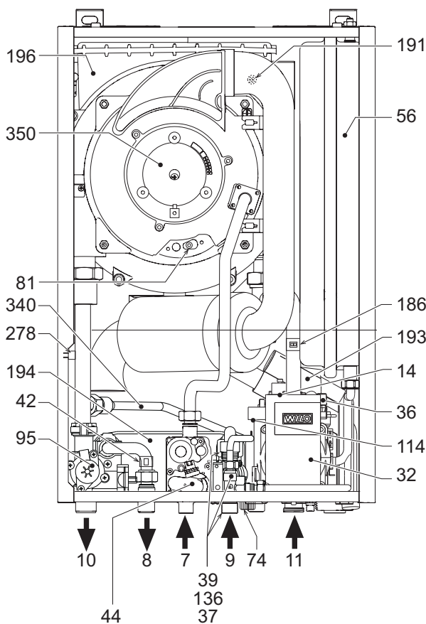
рис. 26 - Общий вид
