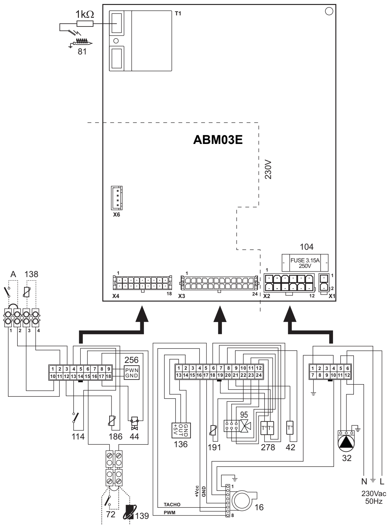
fig. 30 - Schéma électrique
