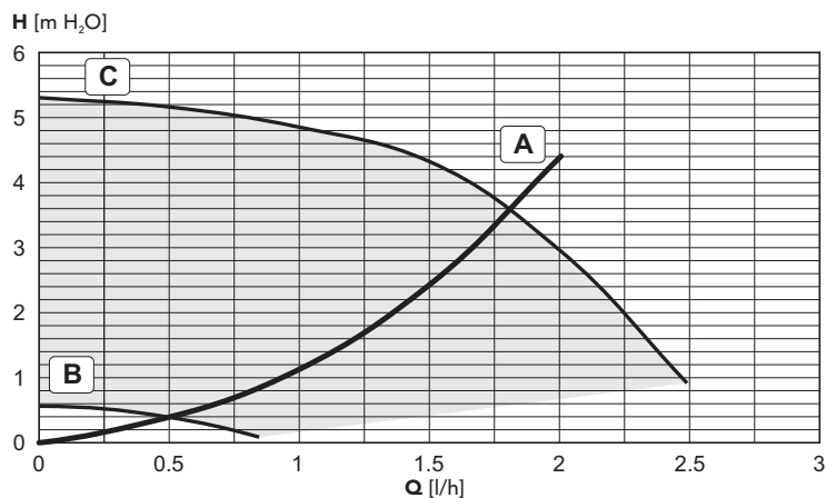
fig. 28 - Pertes de charge/pression circulateur BLUEHELIX TECH 25 C
