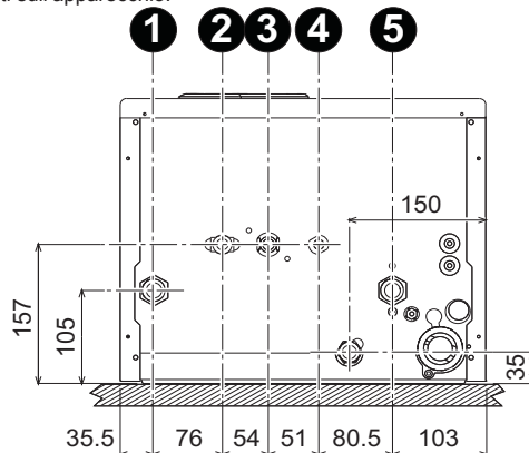
fig. 13 - Attacchi idraulici
