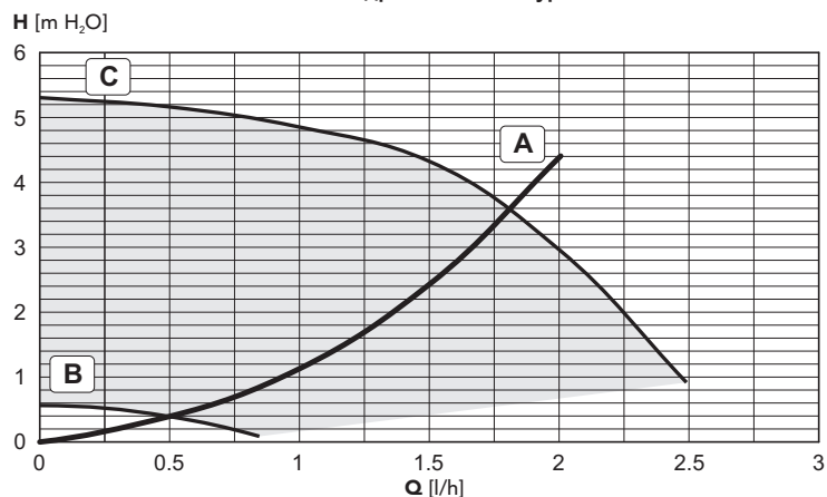
мал. 28 - Втрати напору / Напір циркуляційних насосів BLUEHELIX TECH 25 C
