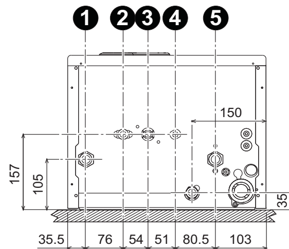
fig. 13 - Racorduri hidraulice
