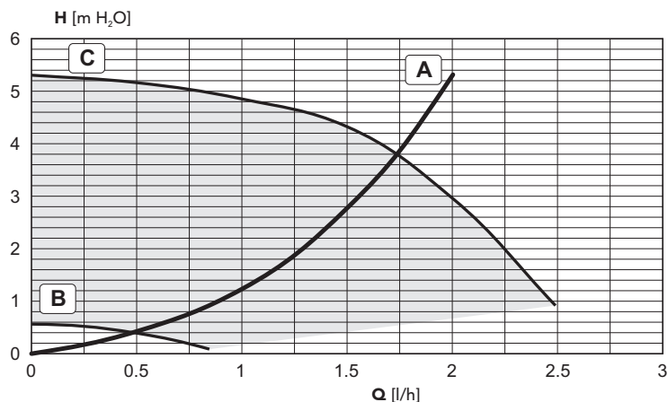
fig. 29 - Pertes de charge/pression circulateur BLUEHELIX TECH 35 C
