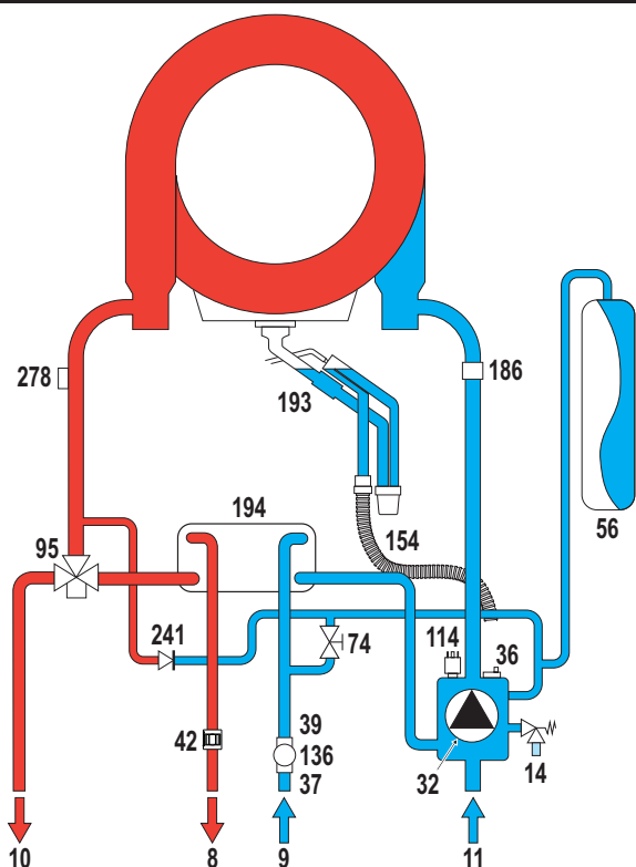
мал. 27 - Гідравлічний контур
