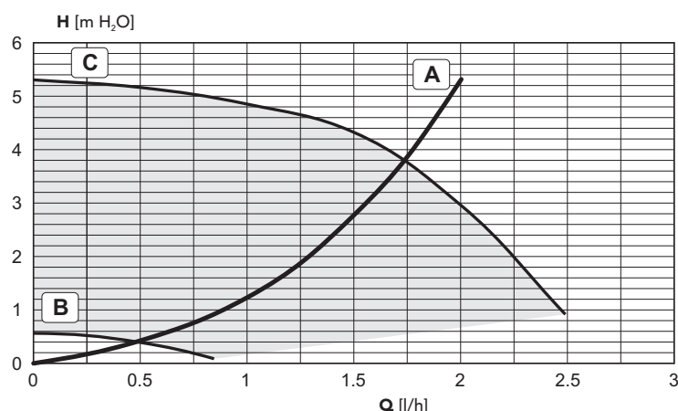
рис. 29 - Потеря напора/Напор циркуляционных насосов BLUEHELIX TECH 35 C
