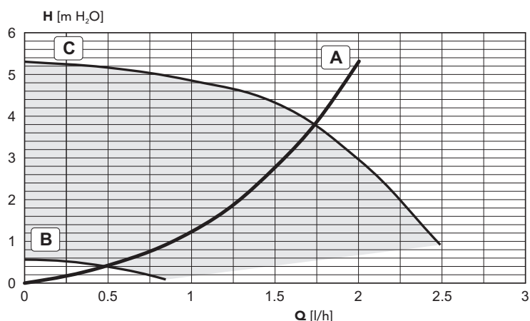
fig. 29 - Pierdere de sarcină / Înălțime de pompă de circulație BLUEHELIX TECH 35 C
