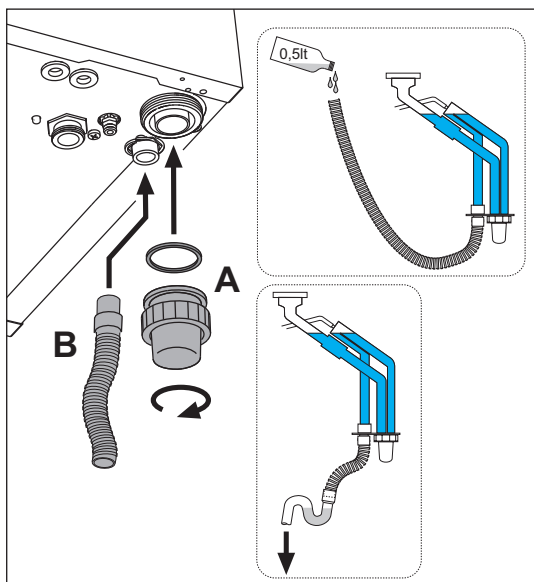
fig. 20 - Collegamento scarico condensa
