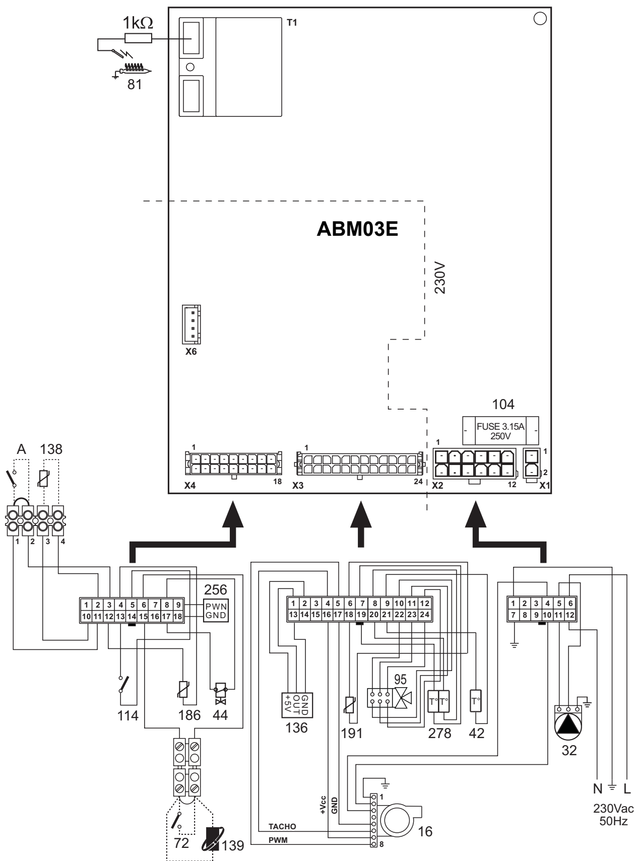
fig. 30 - Wiring diagram
