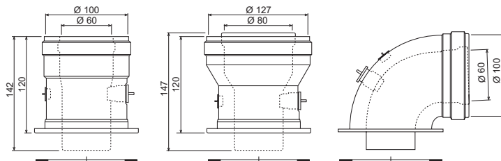
мал. 16 - Початкові елементи для коаксіальних трубопроводів
