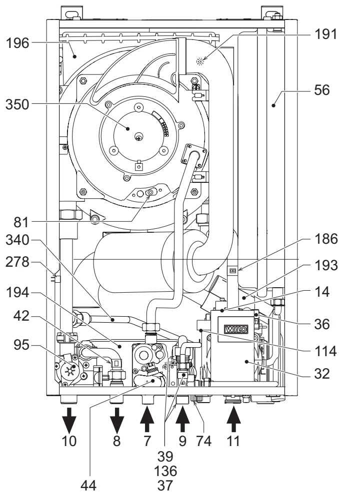
fig. 26 - Vista general
