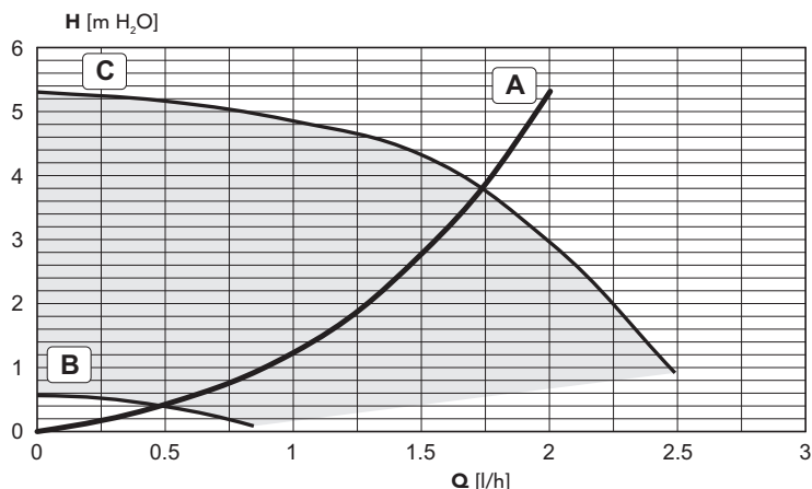
мал. 29 - Втрати напору / Напір циркуляційних насосів BLUEHELIX TECH 35 C
