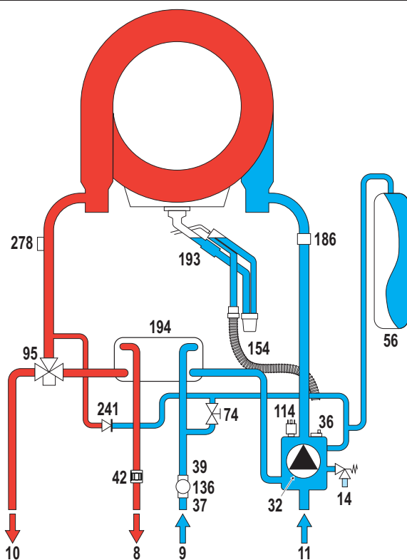
fig. 27 - Circuito idraulico
