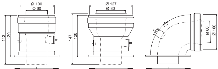
рис. 16 - Элементы для коаксиальных воздухопроводов
