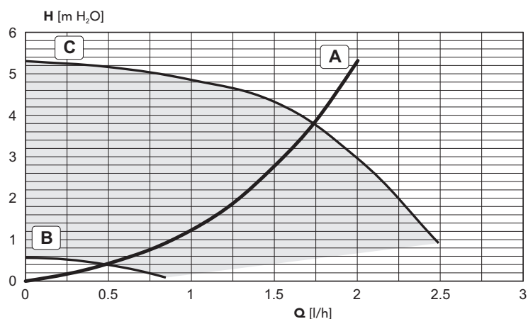
fig. 29 - Perdite di carico / prevalenza circolatore BLUEHELIX TECH 35 C
