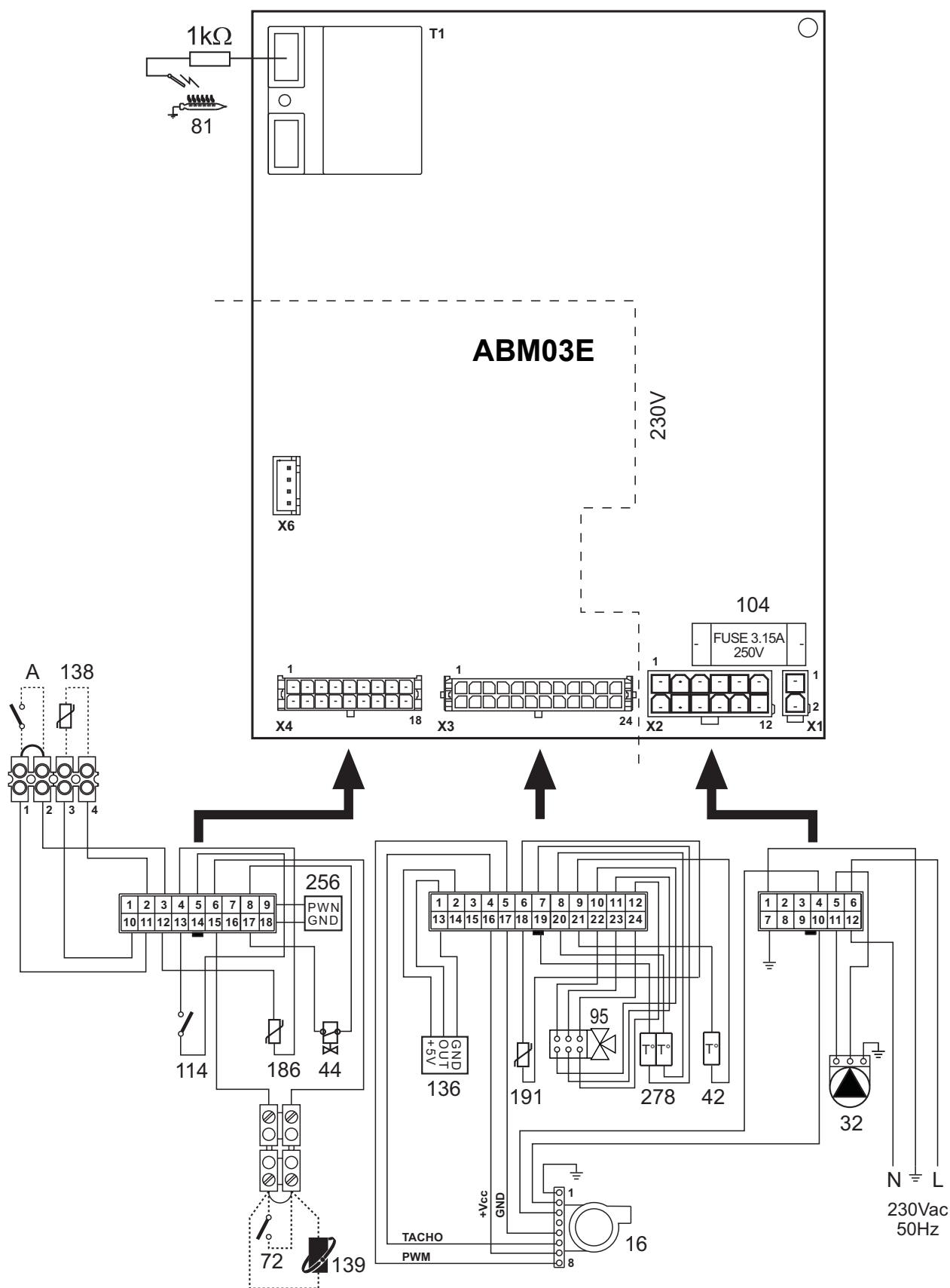
мал. 30 - Електрична схема
