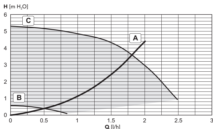
рис. 28 - Потеря напора/Напор циркуляционных насосов BLUEHELIX TECH 25 C
