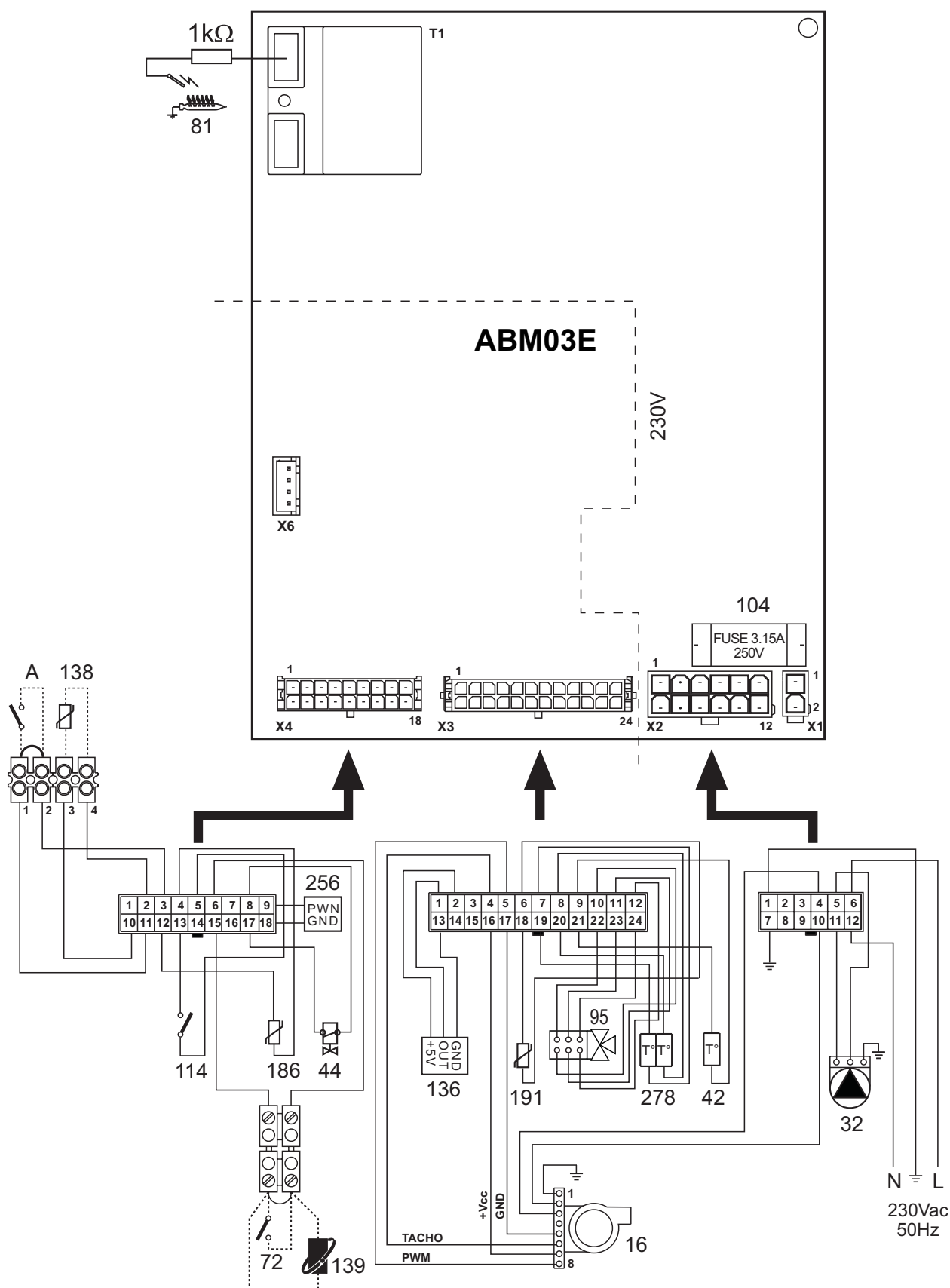
fig. 30 - Esquema eléctrico
