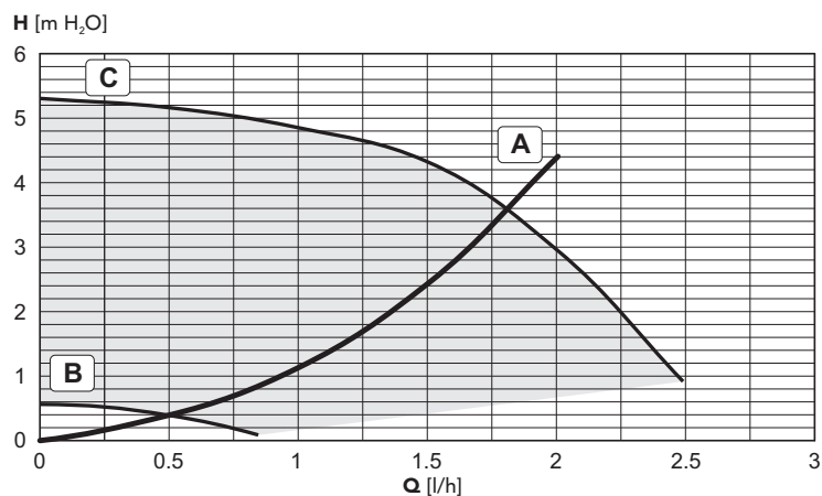
fig. 28 - Perdite di carico / prevalenza circolatore BLUEHELIX TECH 25 C
