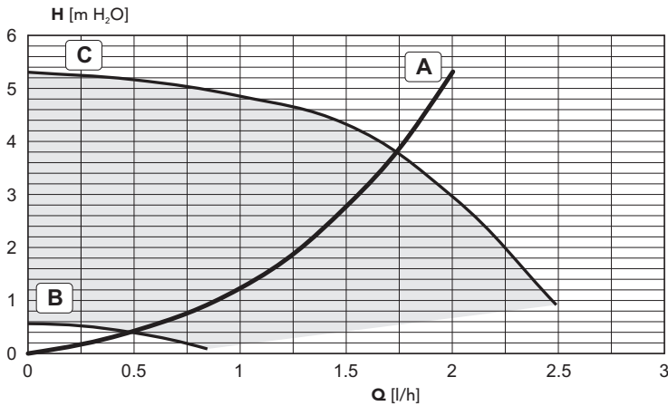
şek. 29 - Sirkülatör yük / basınç kayıpları BLUEHELIX TECH 35 C
