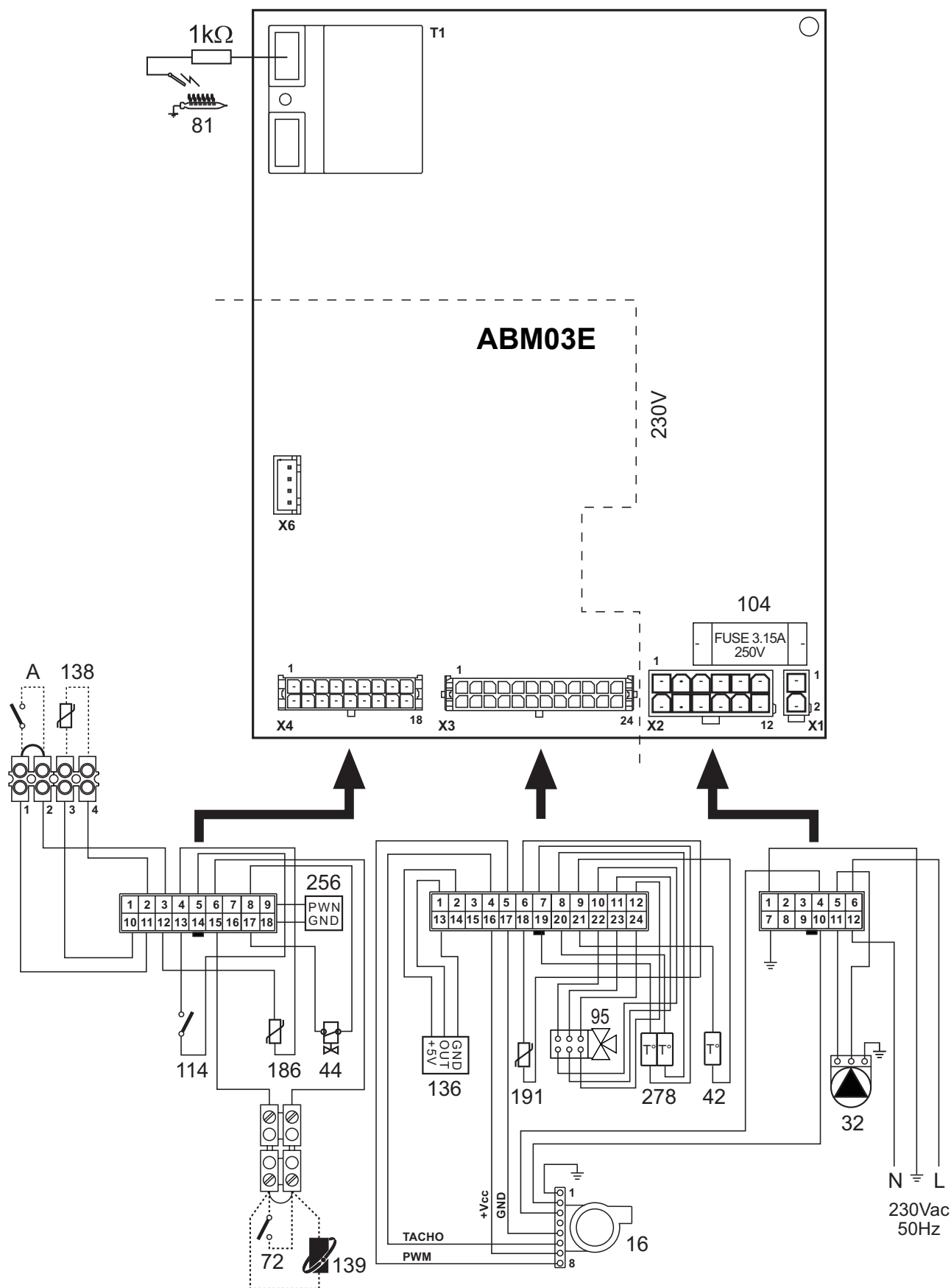
fig. 30 - Schema elettrico
