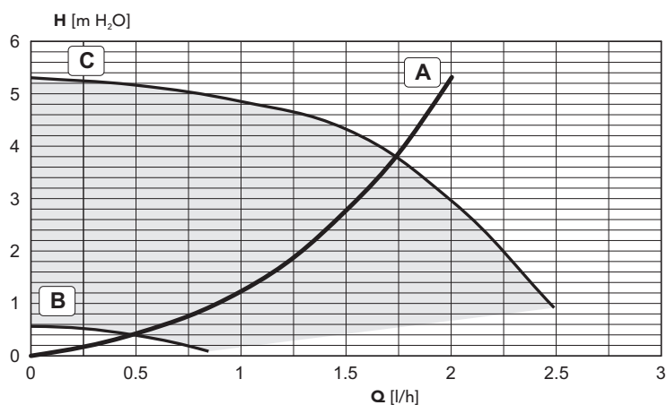
fig. 29 - Pérdida de carga/altura manométrica bomba BLUEHELIX TECH 35 C
