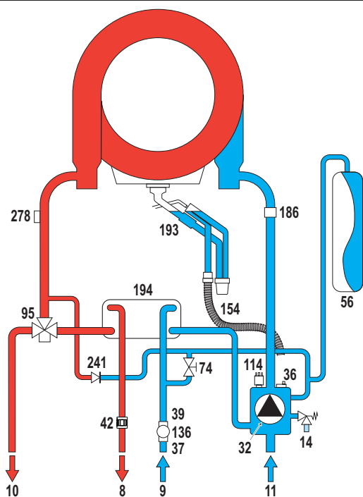
рис. 27 - Гидравлический контур
