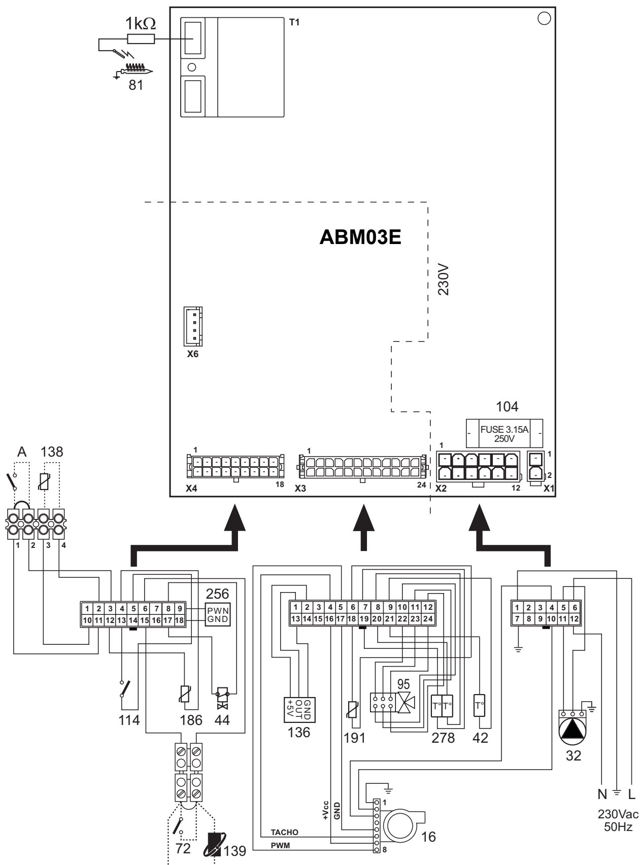
fig. 30 - Schemă electrică
