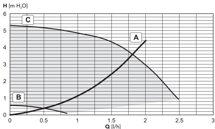
fig. 28 - Pérdida de carga/altura manométrica bomba BLUEHELIX TECH 25 C
