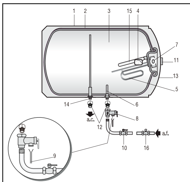
Figura 6 (Instalación horizontal)
