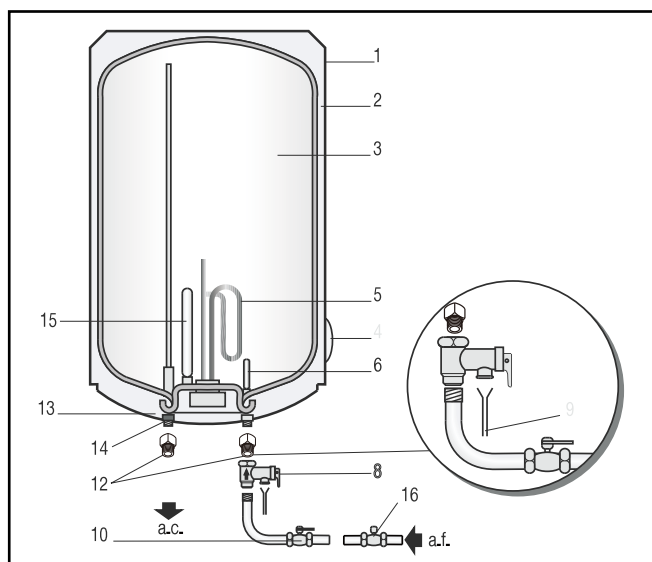
Figura 5 (Instalación vertical)
