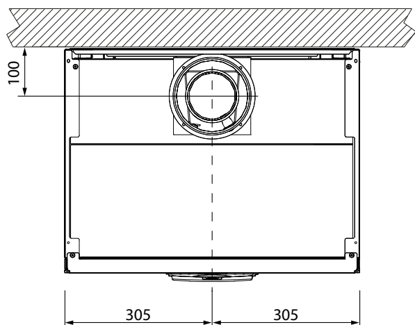
fig. 78- Vue de dessus
