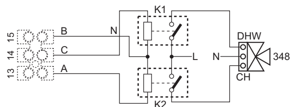
fig. 87- Raccordement de la vanne 3 voies à 3 fils
