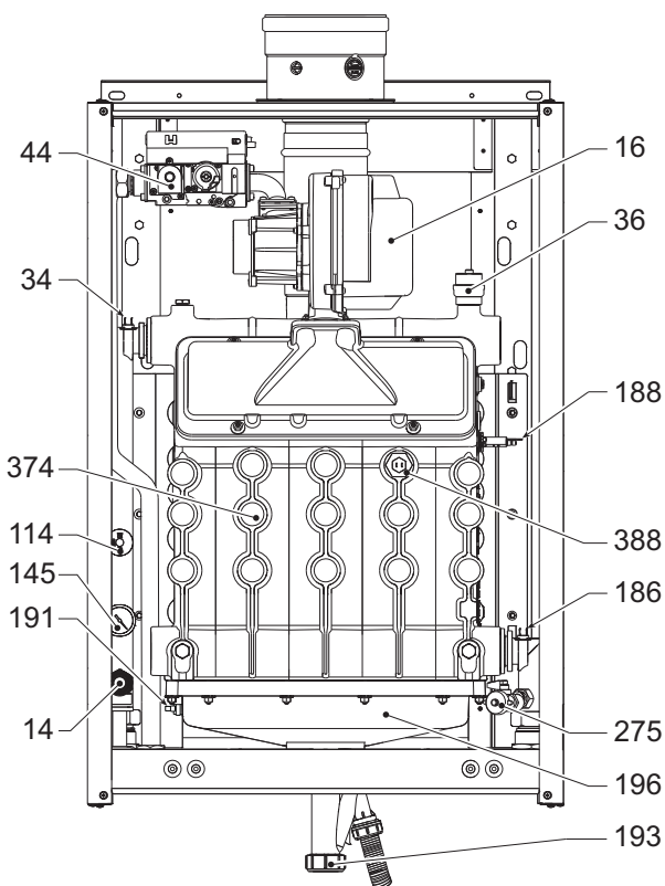
рис. 82- Общий вид, мод. FORCE W 150
