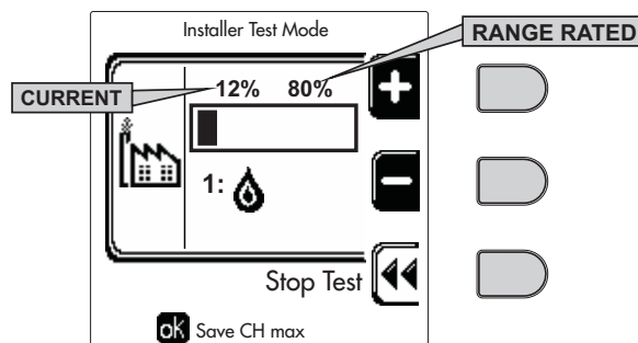
fig. 73 - Modalità TEST (esempio potenza riscaldamento = 80%)
