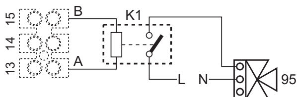
fig. 86- Raccordement de la vanne 3 voies à 2 fils
