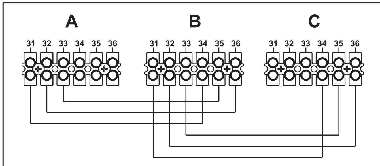
fig. 53- Conectare în cascadă
