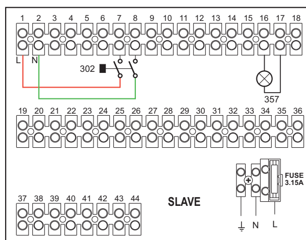
fig. 57- SLAVE
