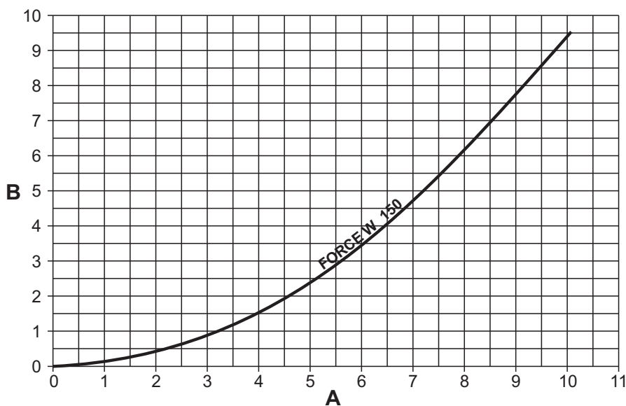
fig. 85 - Diagramma perdita di carico modelli FORCE W 150
