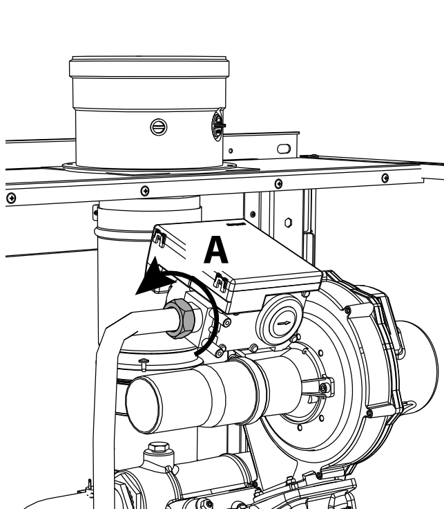
fig. 61- Modèles W 60 et W 80
