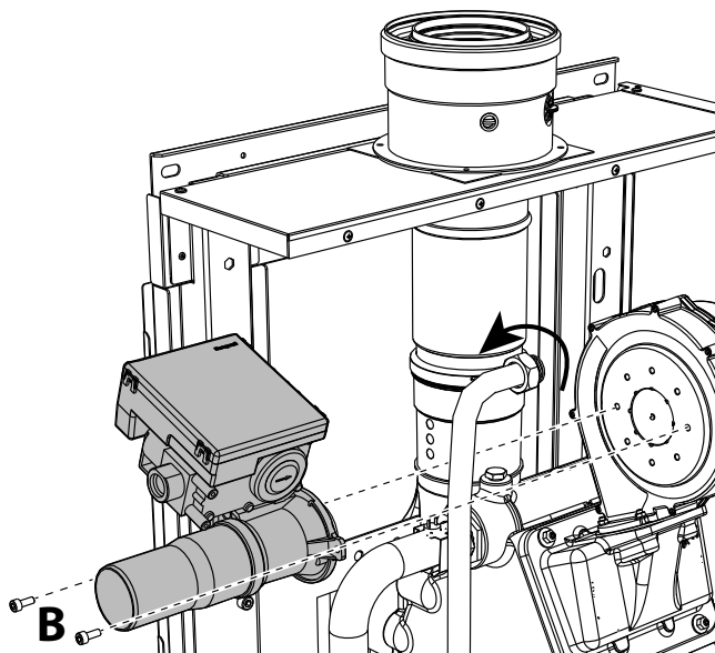
fig. 63- Modelele W 60 și W 80
