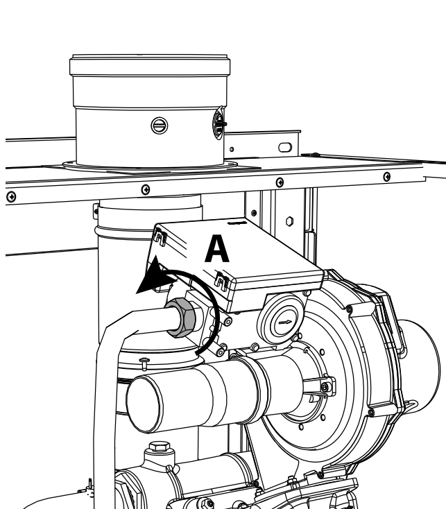
fig. 61- Modelos W 60 y W 80
