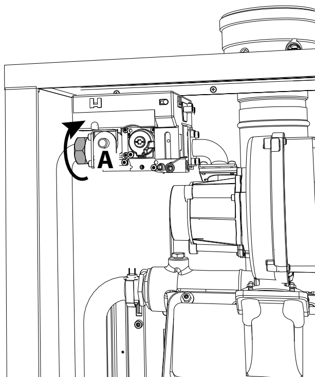
wygląd 62- Modele W 99, W 120 i W 150
