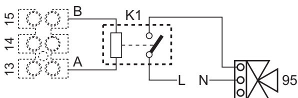
fig. 86- Conexión de la válvula de 3 vías con 2 hilos
