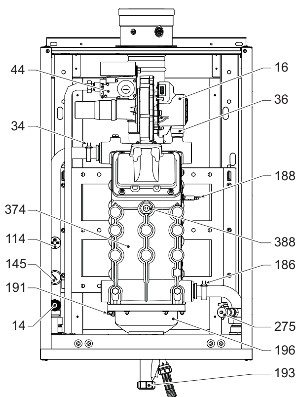
fig. 80 - Vista generale mod. FORCE W 60 e FORCE W 80
