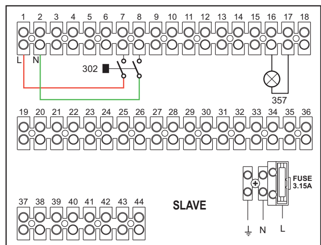
fig. 57- SLAVE
