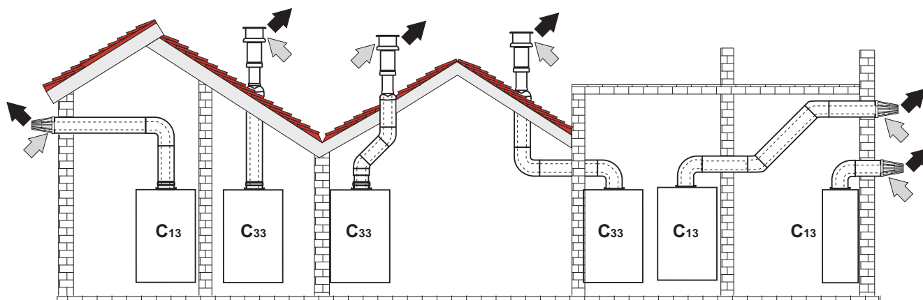
fig. 59- Exemple de racordare cu tuburi coaxiale (⇐ = Aer / ⇨ = Gaze arse)
