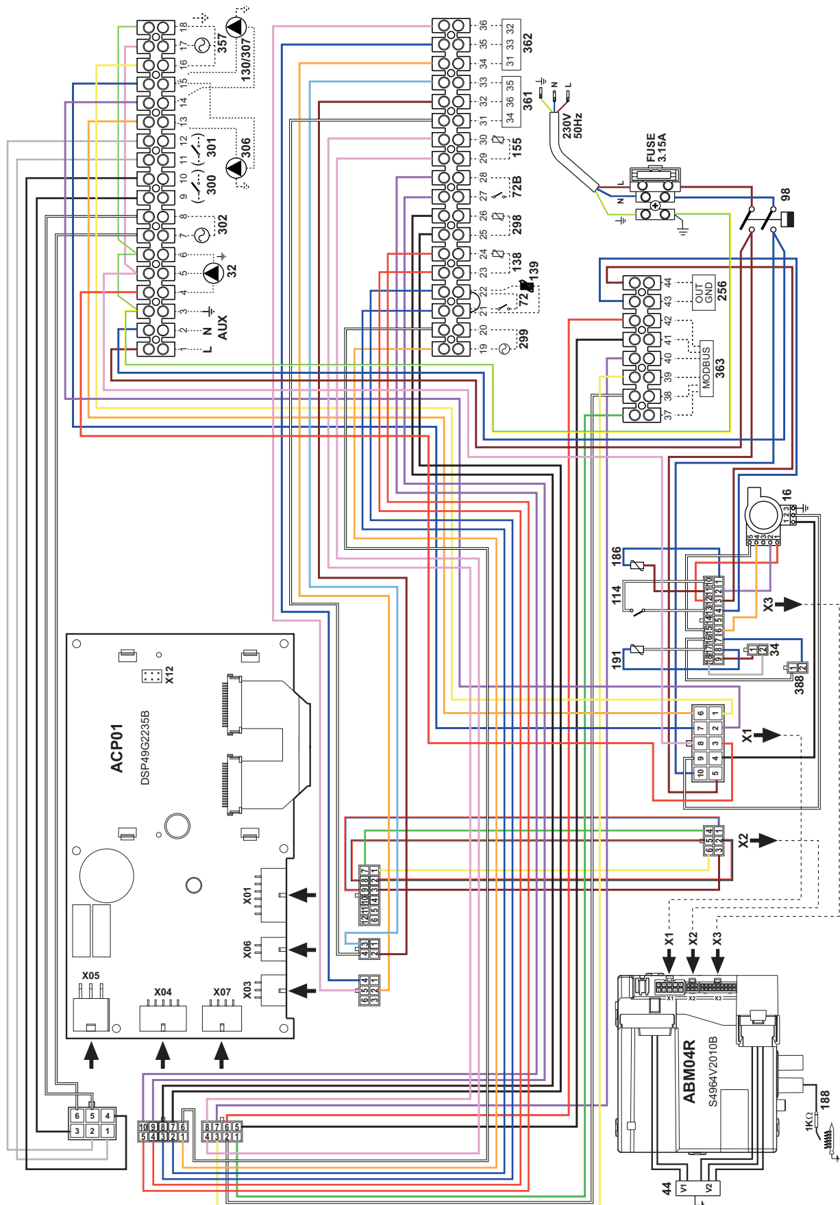
fig. 90- Esquema eléctrico modelos FORCE W 99, FORCE W 120 y FORCE W 150
