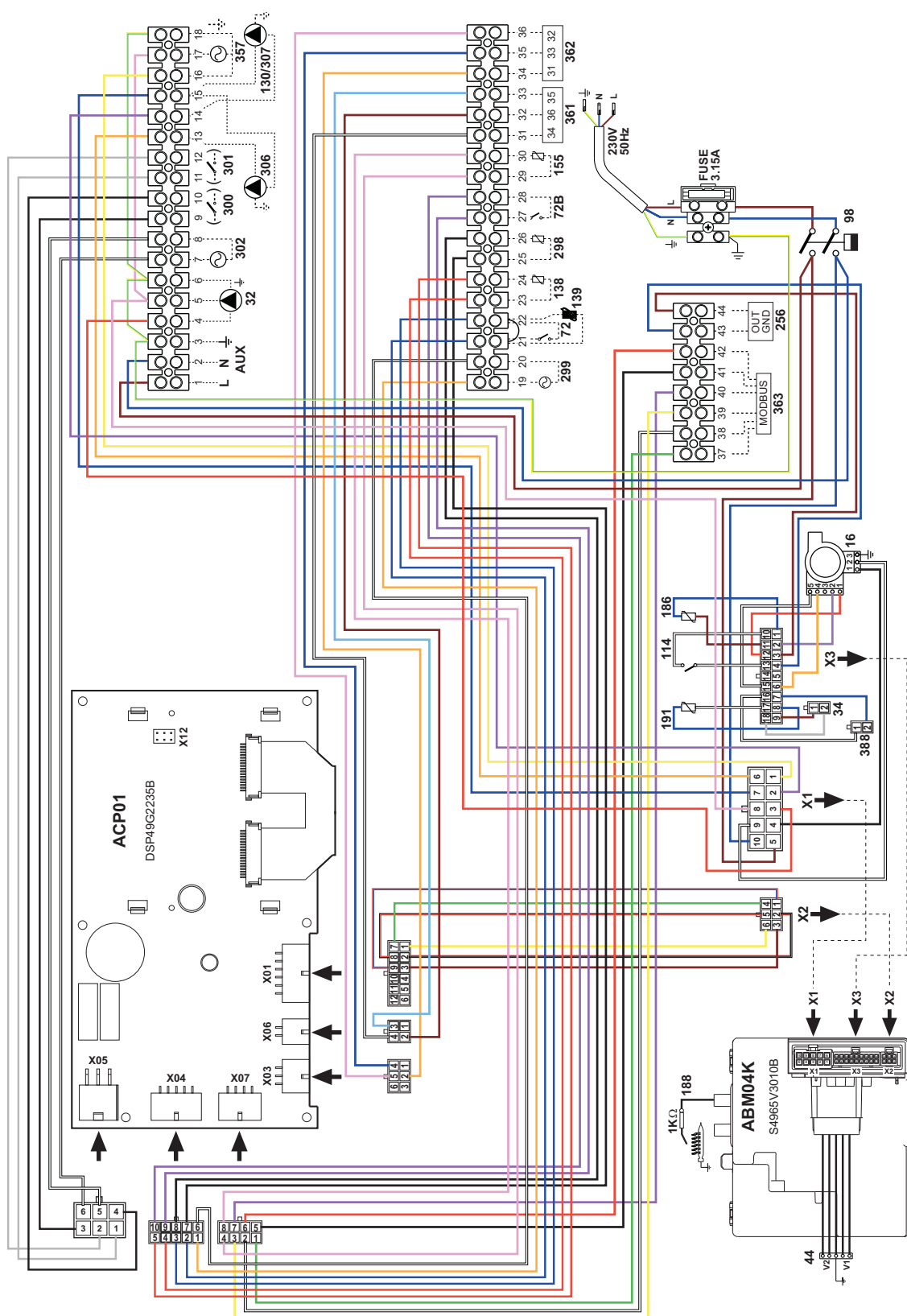
fig. 89- Esquema eléctrico modelos FORCE W 60 y FORCE W 80
