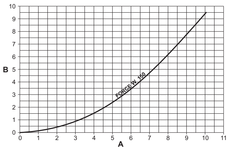
рис. 85- Диаграмма потери нагрузки для моделей FORCE W 150
