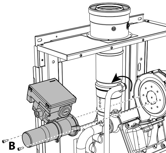
fig. 63- Modelos W 60 y W 80
