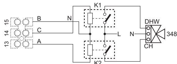
fig. 87- Racordarea valvei cu 3 căi cu 3 fire
