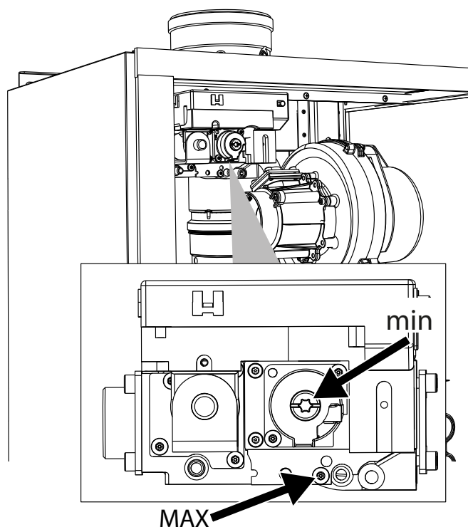
fig. 72- Regulación máxima y mínima modelos W 99, W 120 y W 150
