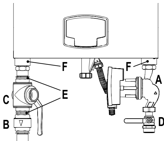
рис. 34- Котел с установленными комплектами
