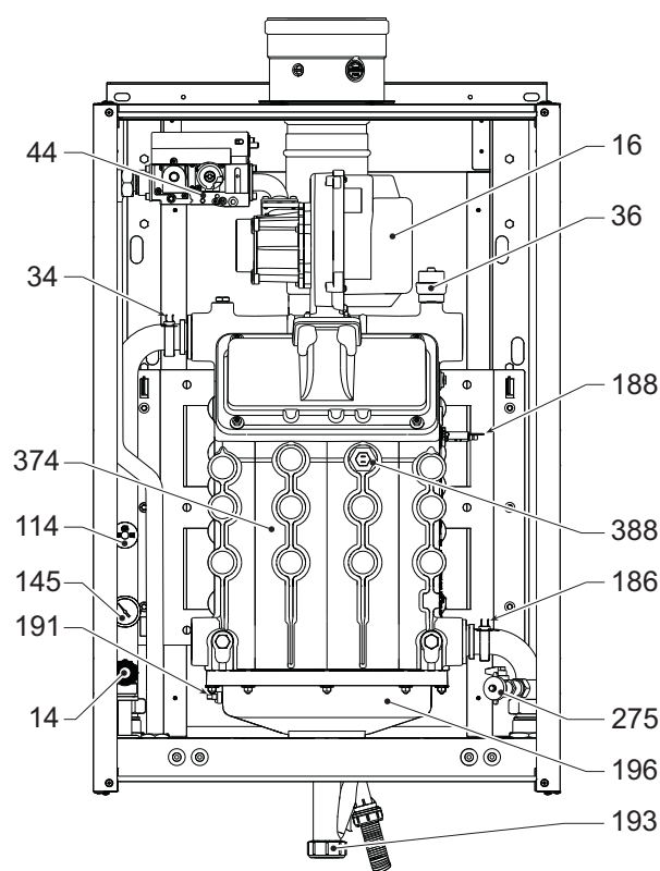
fig. 81- Vue générale mod. FORCE W 99 et FORCE W 120
