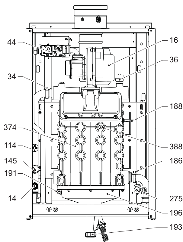
fig. 81 - Vista generale mod. FORCE W 99 e FORCE W 120
