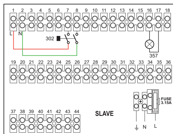
fig. 57- ESCLAVA
