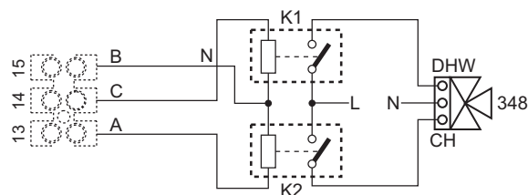
fig. 87- Conexión de la válvula de 3 vías con 3 hilos
