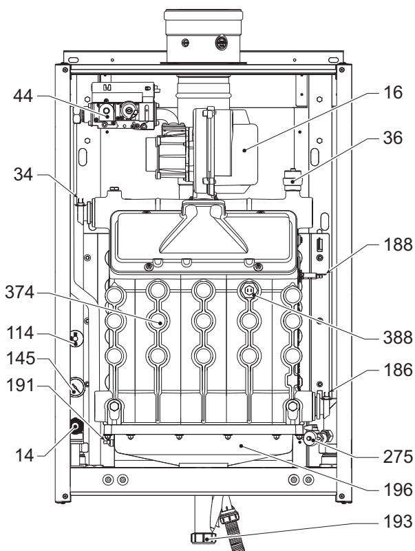
fig. 82- Vue générale mod. FORCE W 150
