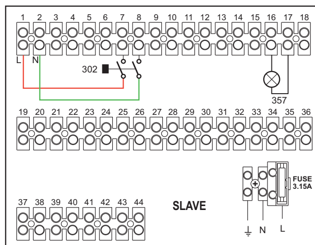
fig. 57- SLAVE
