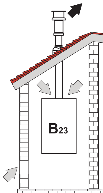
fig. 58 - Esempi di collegamento (⇨=Aria / ⇨=Fumi)
