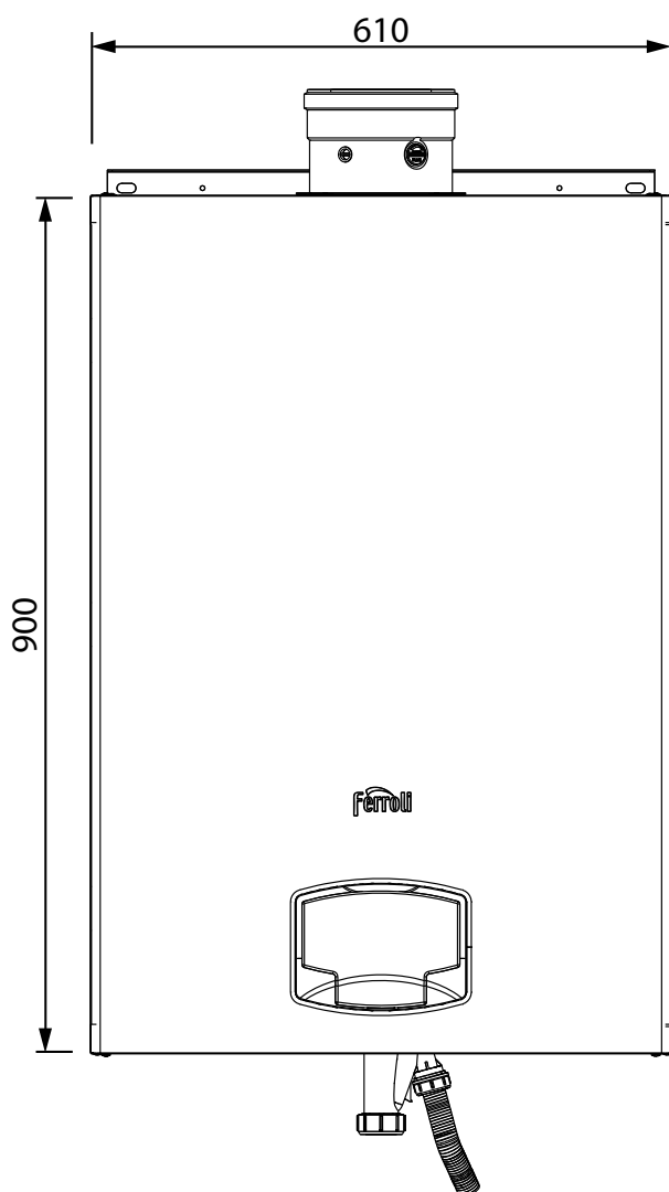
рис. 76- Вид спереди
