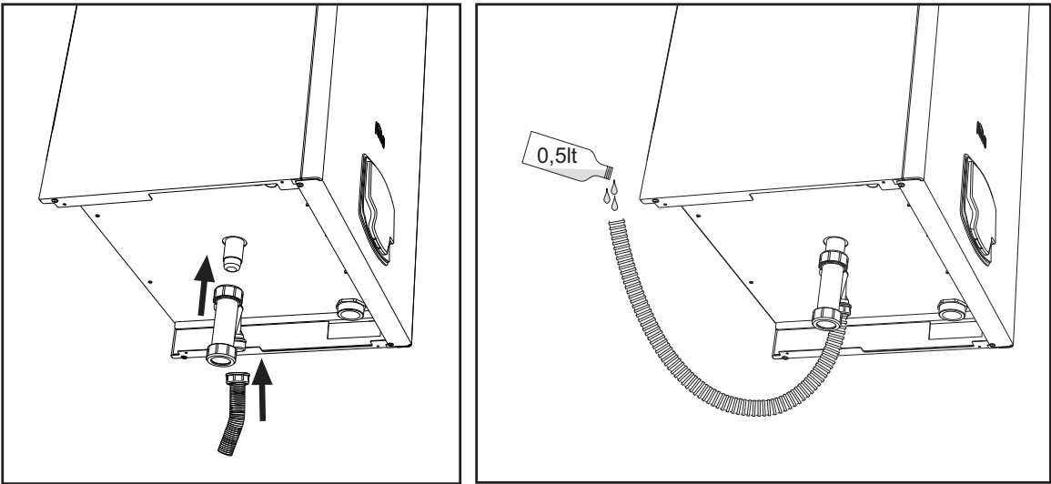
fig. 60- Conexión de la descarga de condensado
