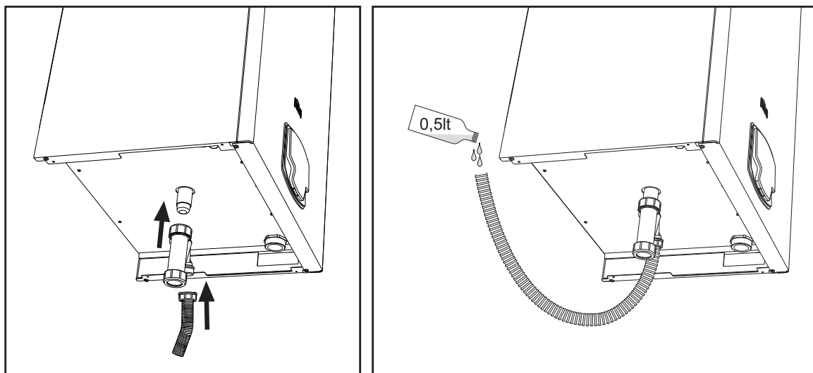
fig. 60- Raccordement de l'évacuation des condensats
