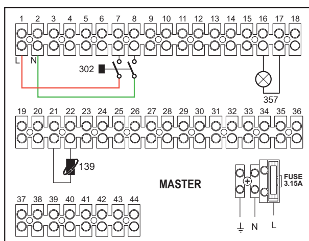
fig. 56- MASTER
