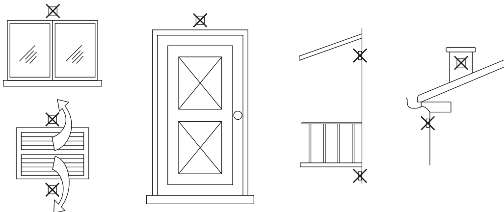
fig. 51- Poziționare nerecomandată a sondei externe
