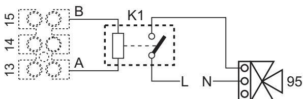
wygląd 86- Podłączenie zaworu 3-drożnego z 2 żyłami
