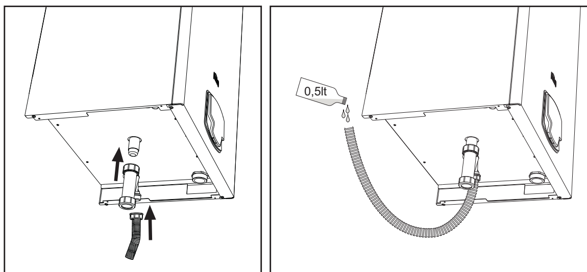
fig. 60- Racordarea evacuării condensului
