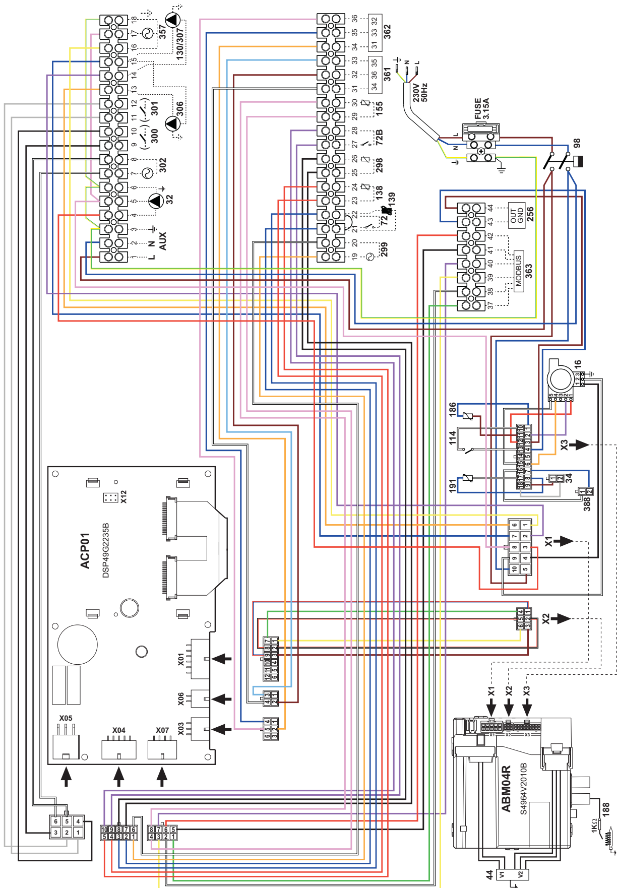
fig. 90 - Schema elettrico modelli FORCE W 99, FORCE W 120 e FORCE W 150
