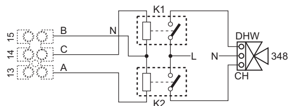
wygląd 87- Podłączenie zaworu 3-drożnego z 3 żyłami
