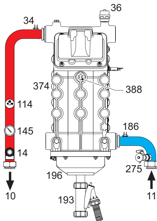
wygląd 83- Obwód hydrauliczny
