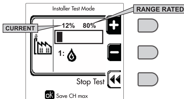
fig. 73- Modul TEST (exemplu putere de încălzire = 80%)
