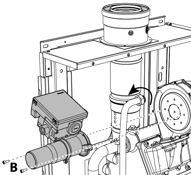
fig. 63- Modèles W 60 et W 80
