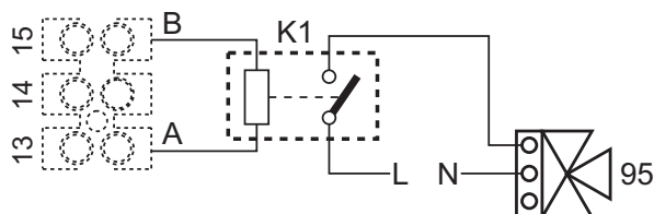
fig. 86- Racordarea valvei cu 3 căi cu 2 fire
