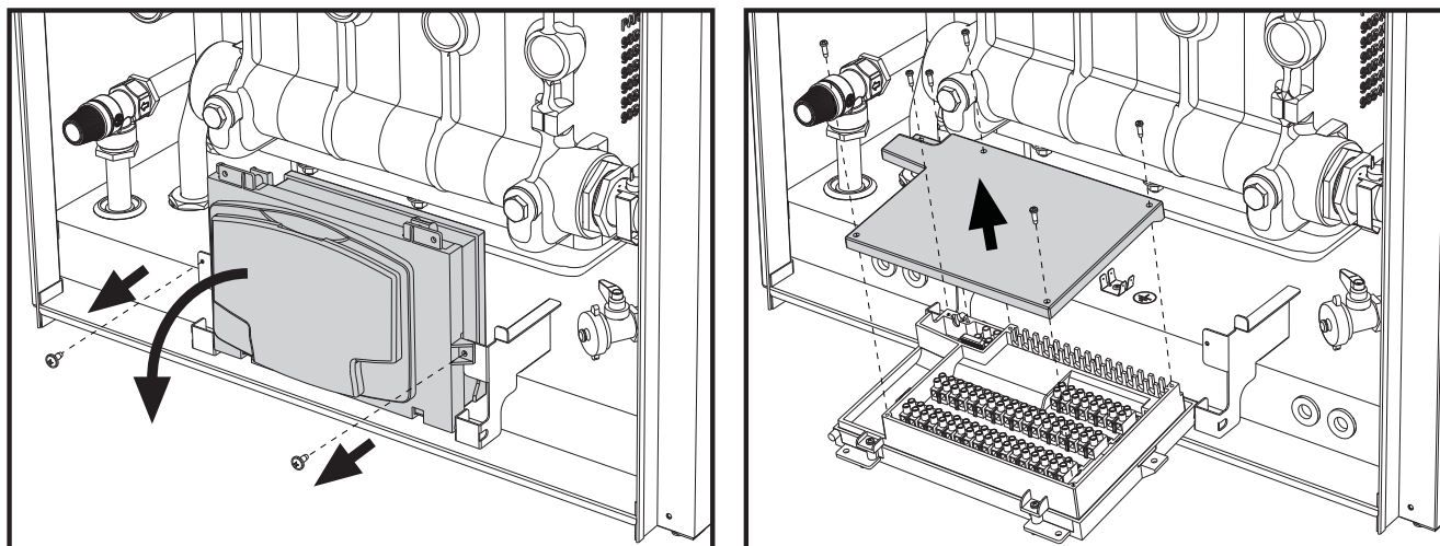
fig. 52- Panoul de borne electric
