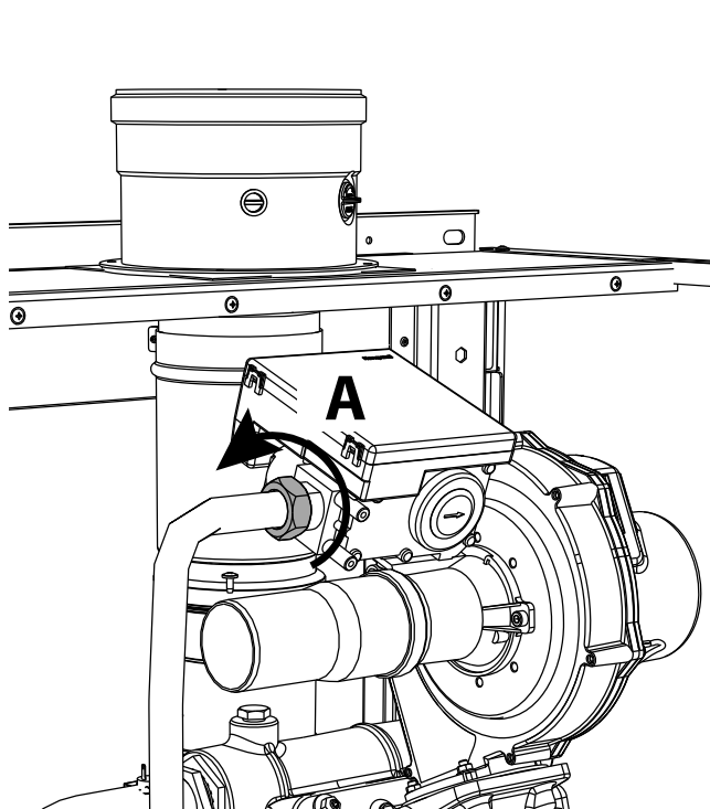
wygląd 61- Modele W 60 i W 80
