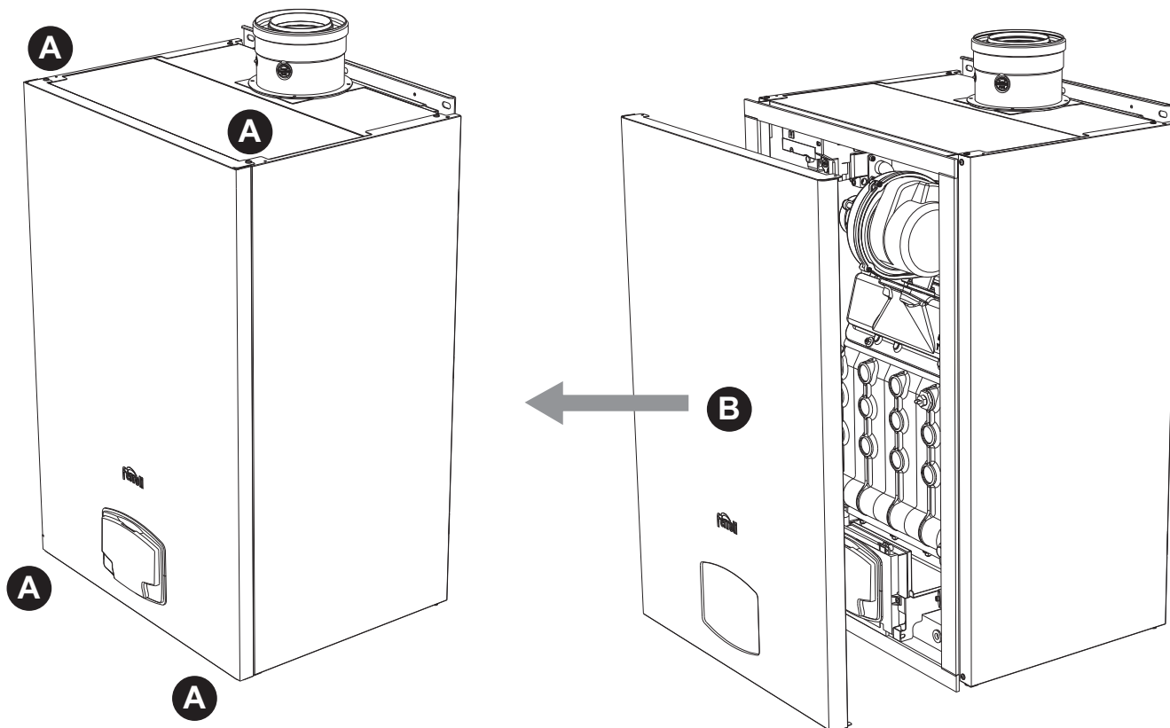
fig. 75 - Apertura pannello frontale
