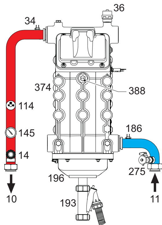
fig. 83- Circuitul hidraulic
