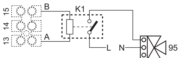
fig. 86 - Collegamento della valvola a 3 vie con 2 fili
