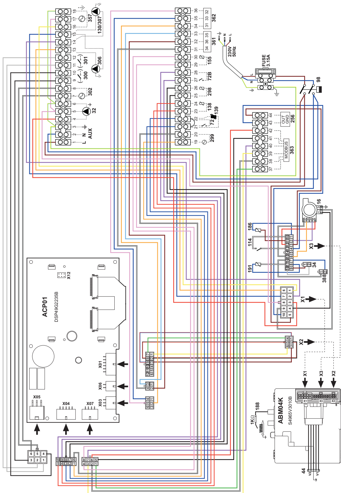
fig. 89- Schemă electrică modelele FORCE W 60 și FORCE W 80
