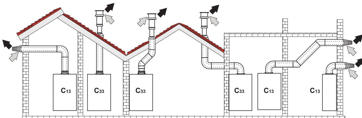
fig. 59- Exemples de raccordement avec tubes coaxiaux (⇐ = Air / ⇨ = Fumées)
