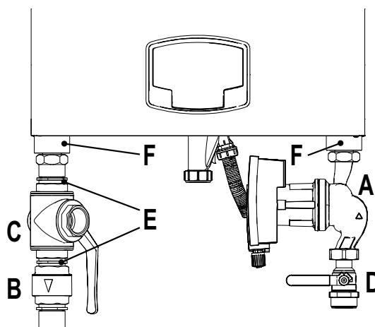
fig. 34 - Caldaia con i kit installati
