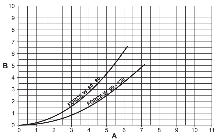
рис. 84- Диаграмма потери нагрузки для моделей FORCE W 60 - FORCE W 80 - FORCE W 99 - FORCE W 120
