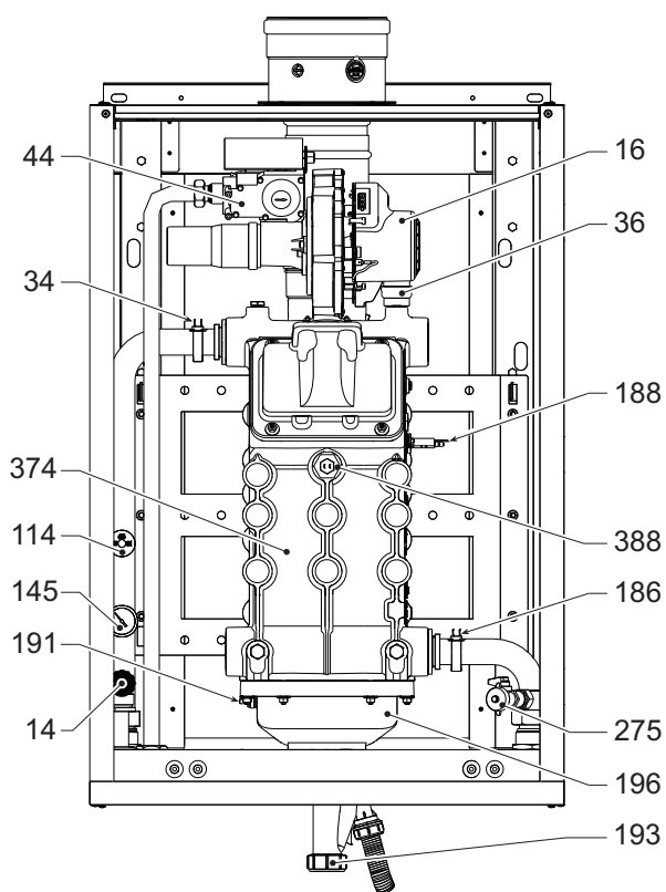
рис. 80- Общий вид, мод. FORCE W 60 и FORCE W 80
