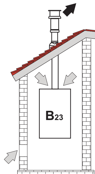
fig. 58- Exemples de raccordement (⇐ = Air / ➡ = Fumées)
