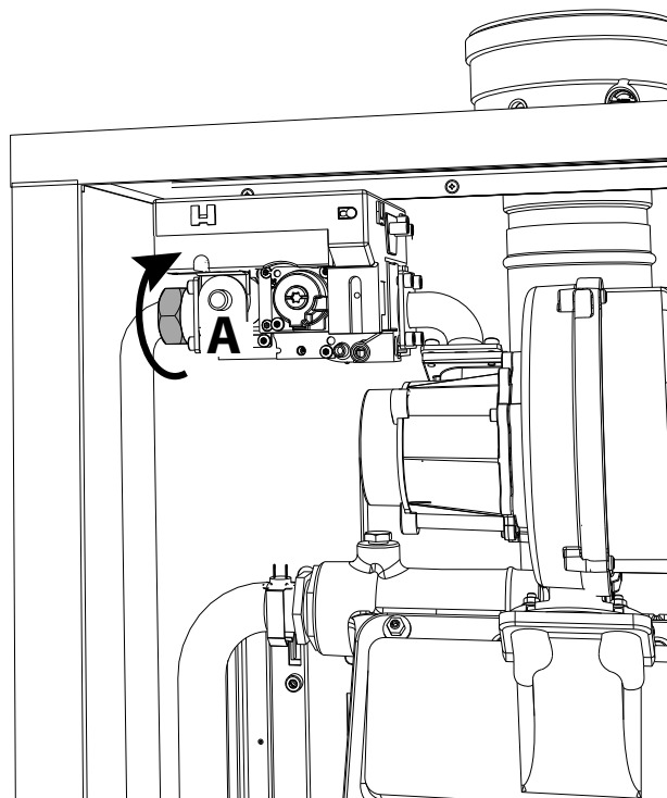
fig. 62- Modelos W 99, W 120 y W 150
