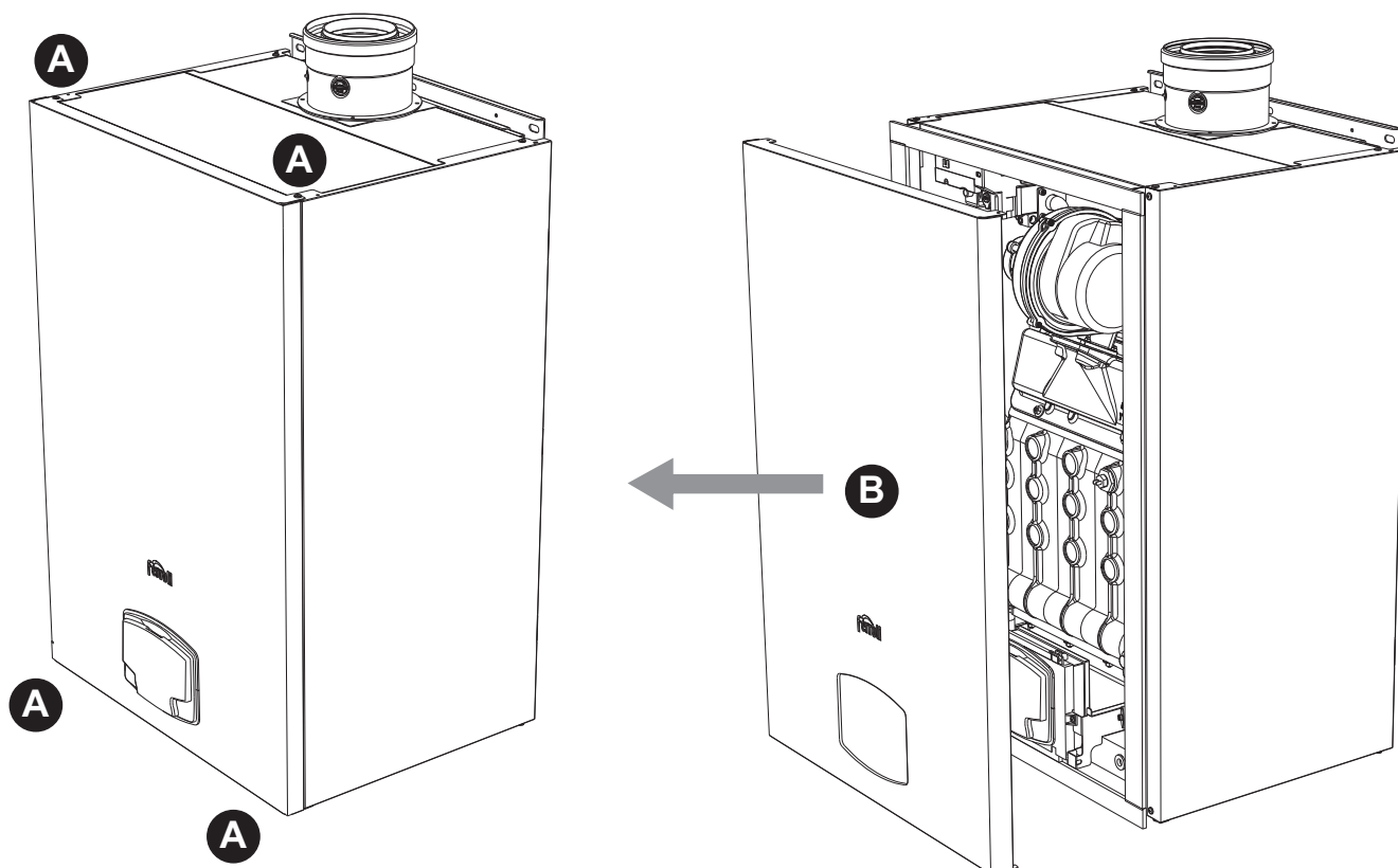
fig. 75- Apertura del panel frontal
