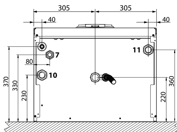
fig. 79- Vue de dessous
