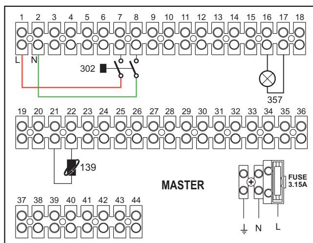
рис. 56- MASTER (ВЕДУЩИЙ)
