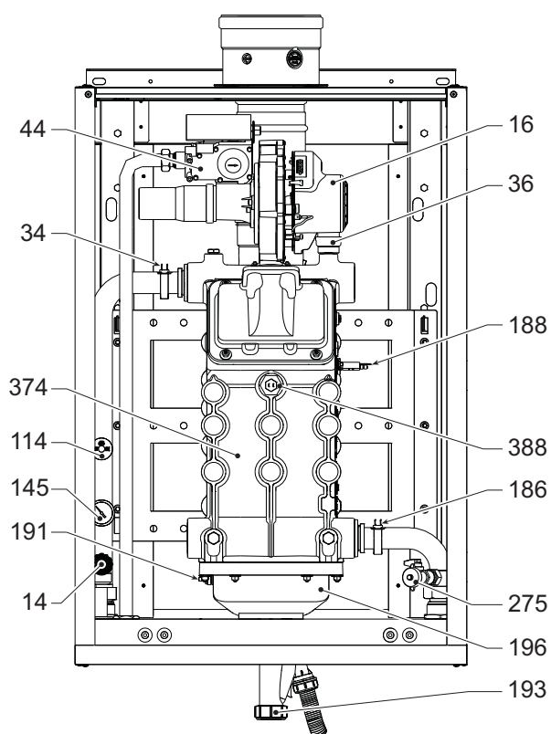
fig. 80- Vue générale mod. FORCE W 60 et FORCE W 80
