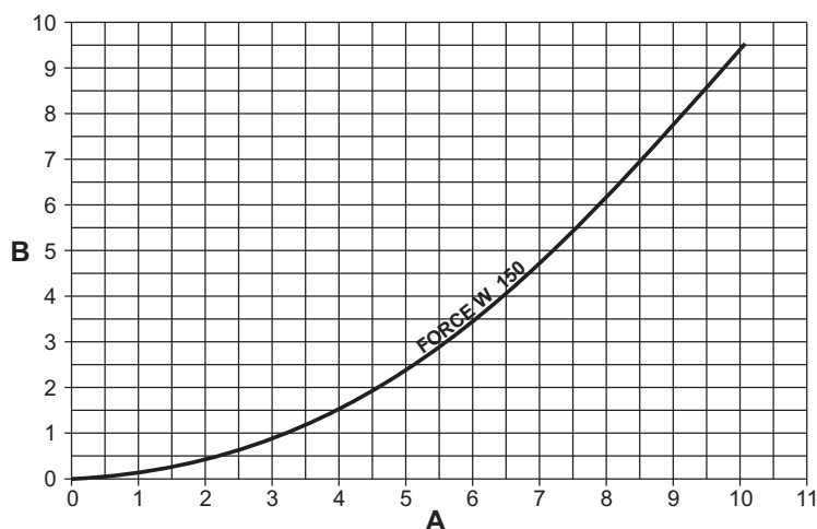
fig. 85- Diagramme perte de charge modèles FORCE W 150
