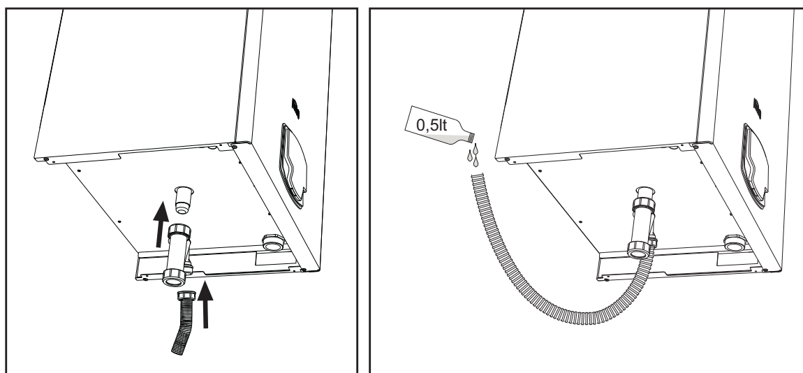
fig. 60 - Collegamento scarico condensa
