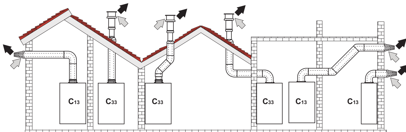
fig. 59- Ejemplos de conexión con tubos coaxiales (⇨ = aire / ⇨ = humos)
