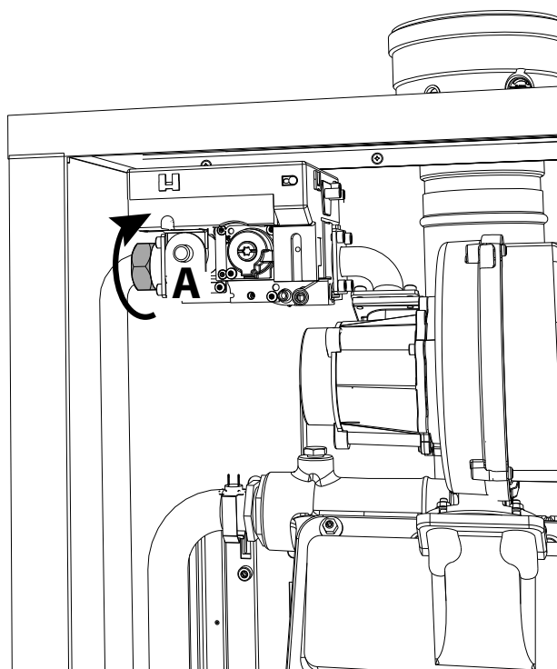
fig. 62- Modèles W 99, W 120 et W 150
