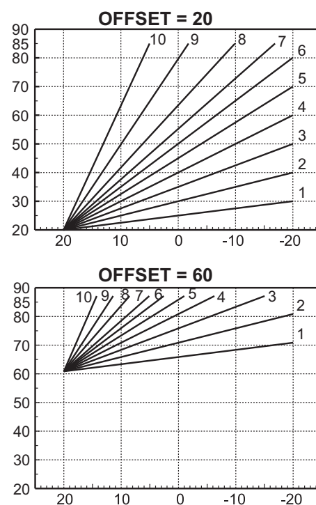
fig. 31- Exemplu de deplasare paralelă a curbelor de compensare
