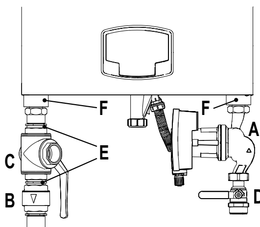
fig. 34- Centrală cu kiturile instalate
