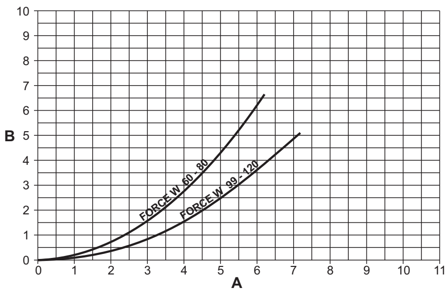
fig. 84 - Diagramma perdita di carico modelli FORCE W 60 - FORCE W 80 - FORCE W 99 - FORCE W 120
