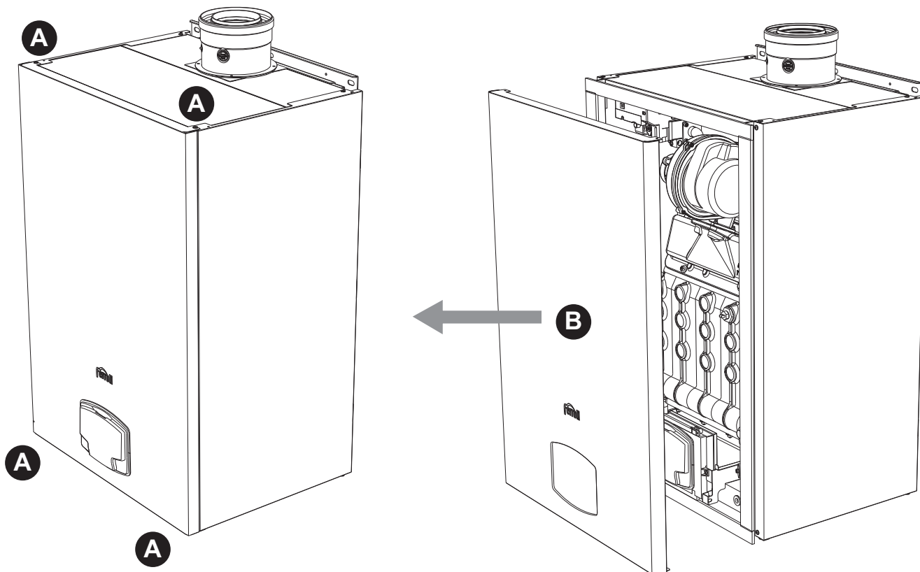
fig. 75- Ouverture du panneau avant
