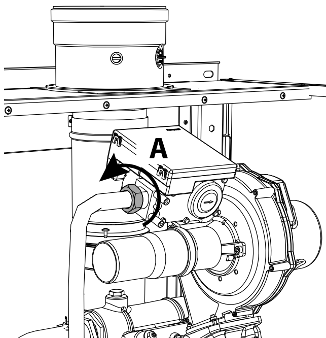
fig. 61- Modelele W 60 și W 80
