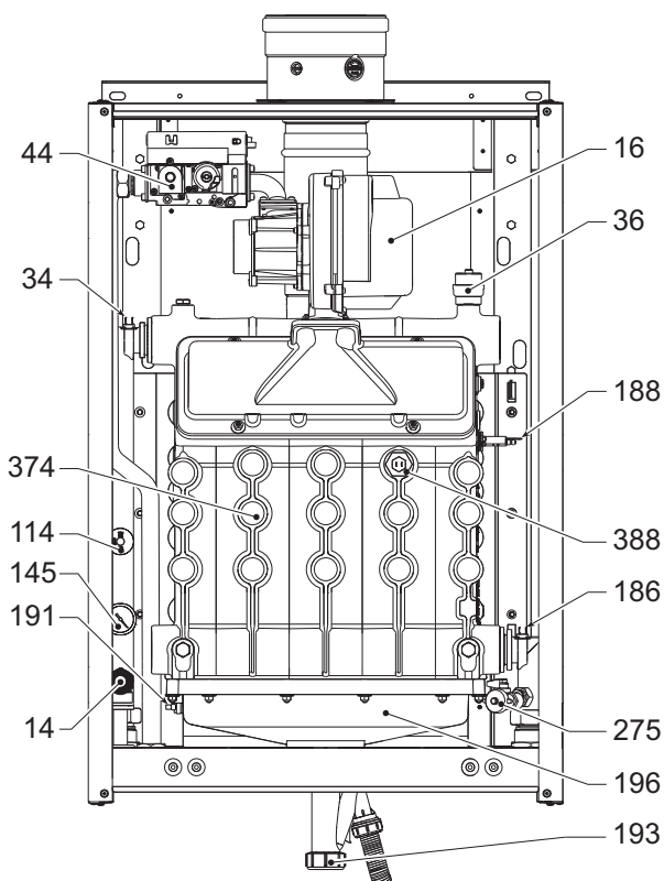
fig. 82- Vedere generală mod. FORCE W 150
