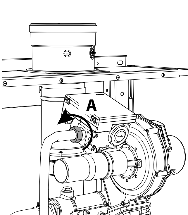
рис. 61- Модели W 60 и W 80
