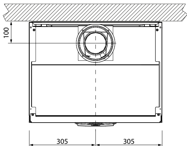
fig. 78- Vedere de sus
