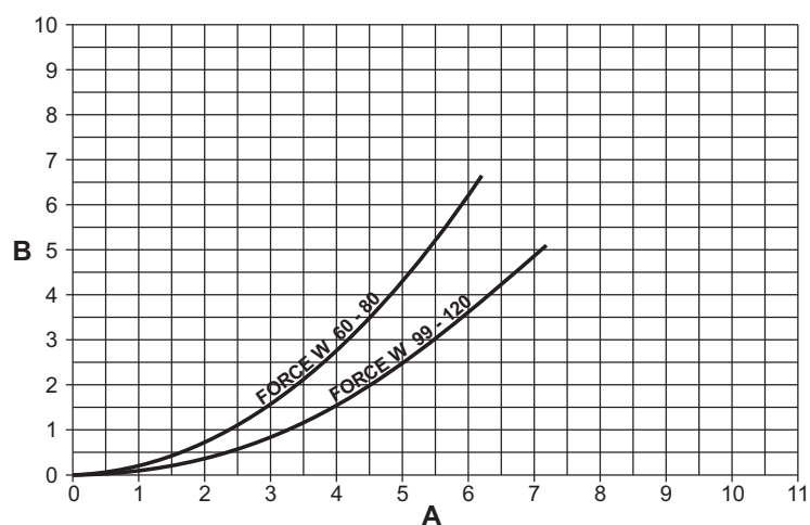
fig. 84- Diagramă pierderi de sarcină modelele FORCE W 60 - FORCE W 80 - FORCE W 99 - FORCE W 120
