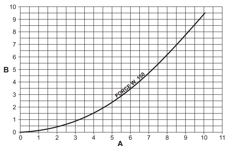
fig. 85- Diagramă pierderi de sarcină modelele FORCE W 150
