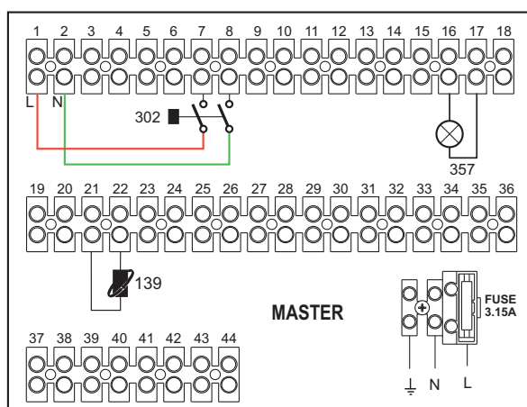
fig. 56- MAESTRA
