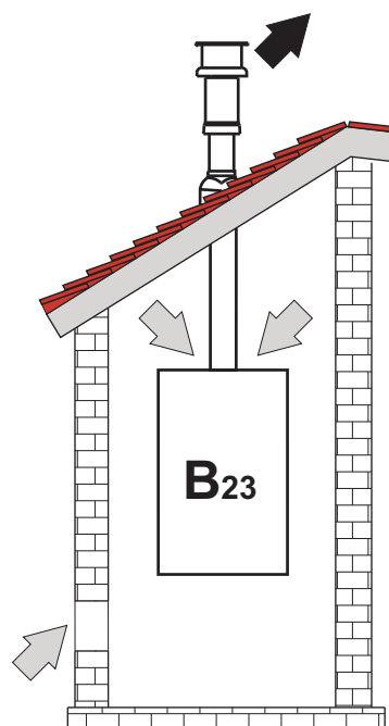
fig. 58- Exemple de conectare (⇨ = Aer / ⇨ = Gaze arse)
