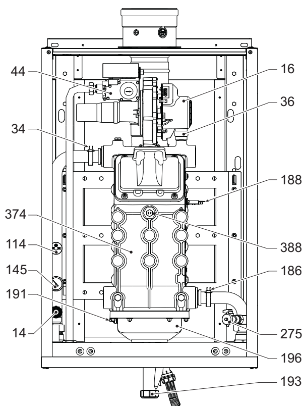
fig. 80- Vedere generală mod. FORCE W 60 și FORCE W 80
