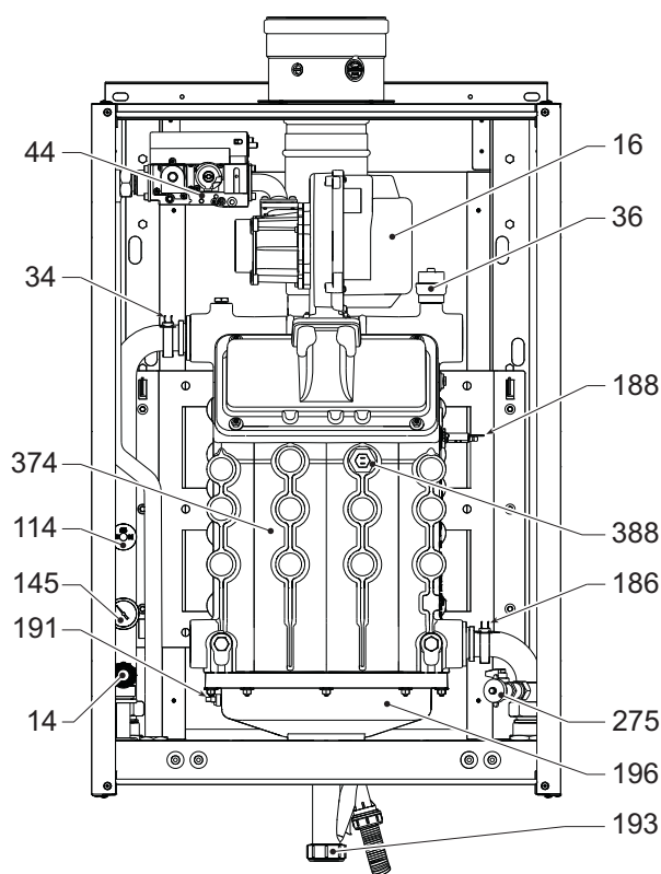
рис. 81- Общий вид, мод. FORCE W 99 и FORCE W 120
