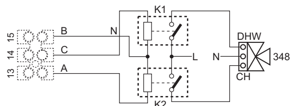
fig. 87 - Collegamento della valvola a 3 vie con 3 fili
