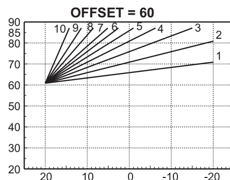
wygląd 31- Przykład przesunięcia równoległego krzywych kompensacji
