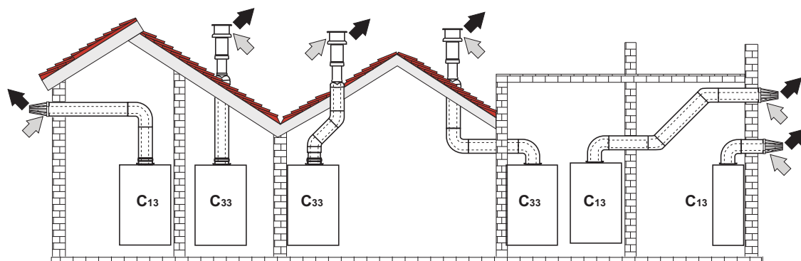
fig. 59 - Esempi di collegamento con tubi coassiali (→ = Aria / → = Fumi)
