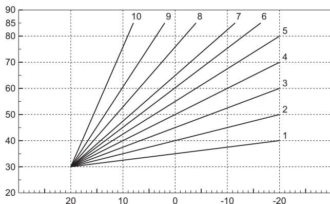
рис. 30- Компенсационные кривые
