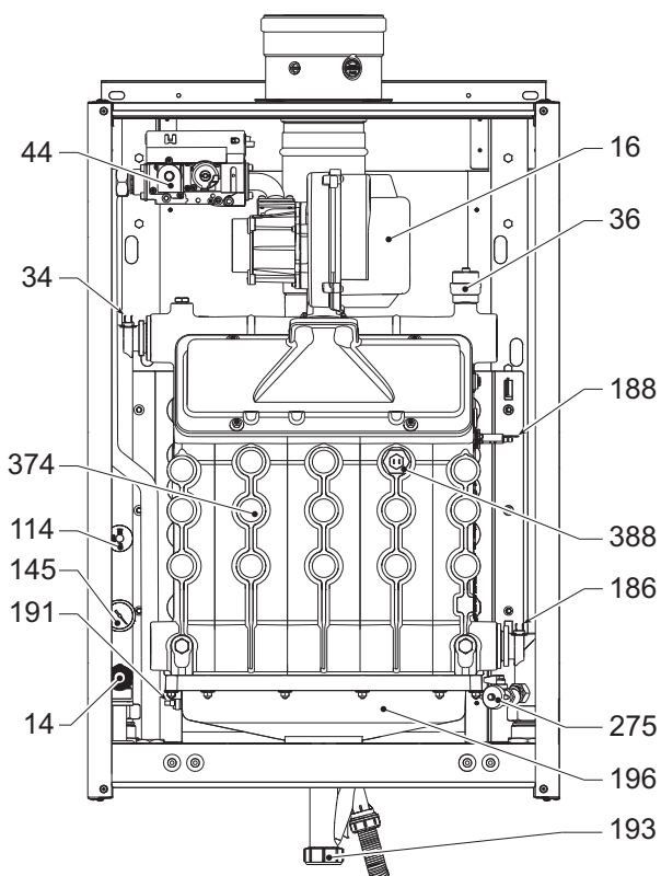
fig. 82 - Vista generale mod. FORCE W 150
