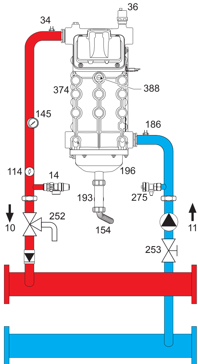
Circuito de agua
