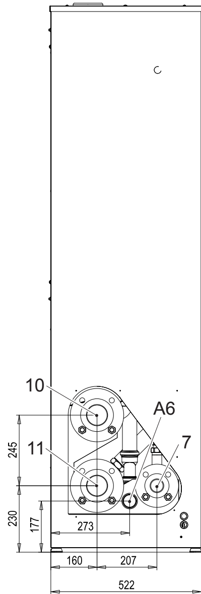
Vista lateral
