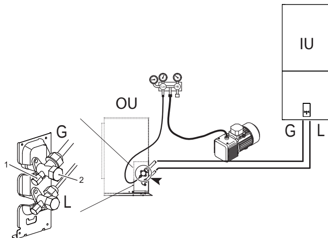
fig. 15 - Purga de aire con bomba de vacío
