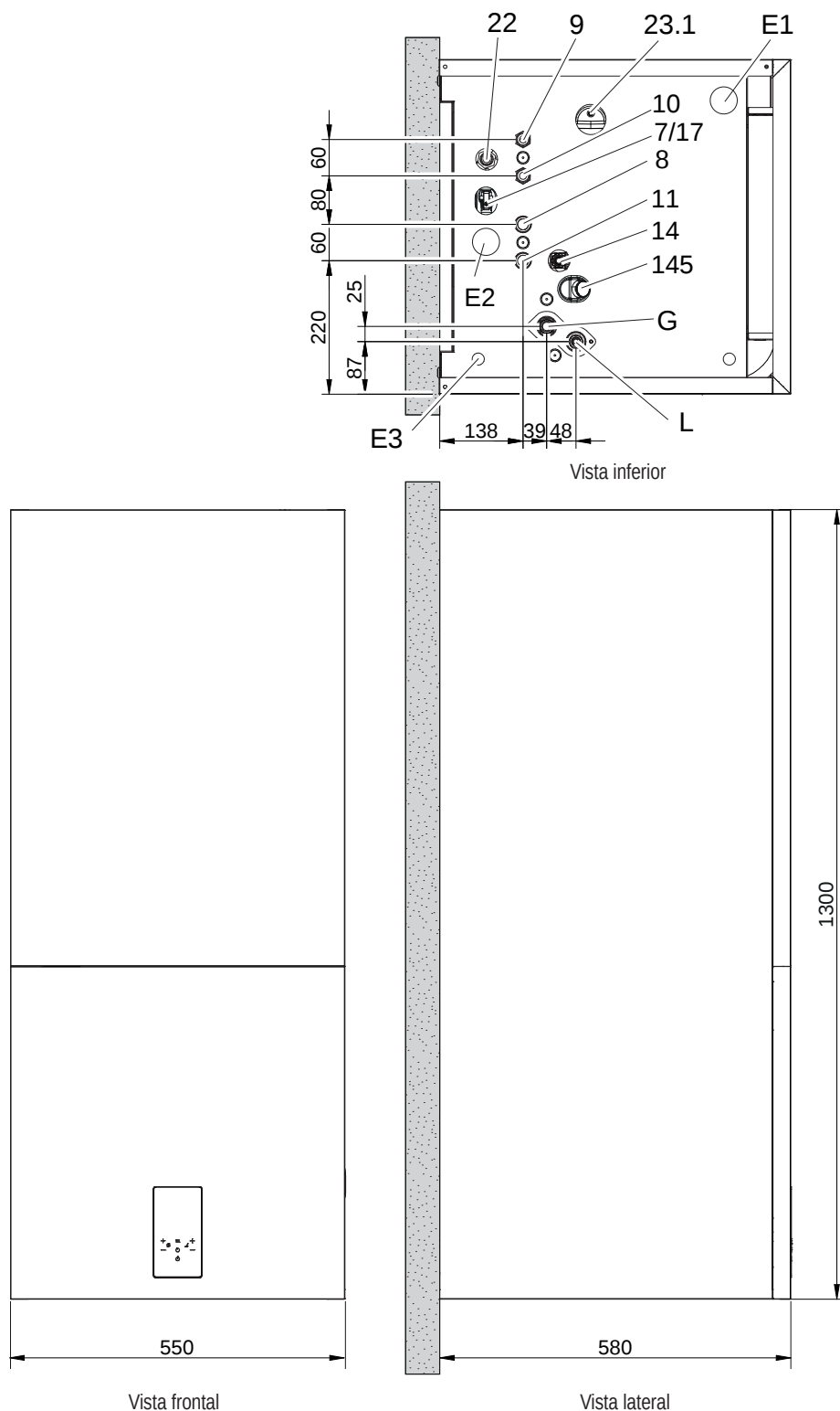
fig. 3 - datos dimensionales y conexiones
