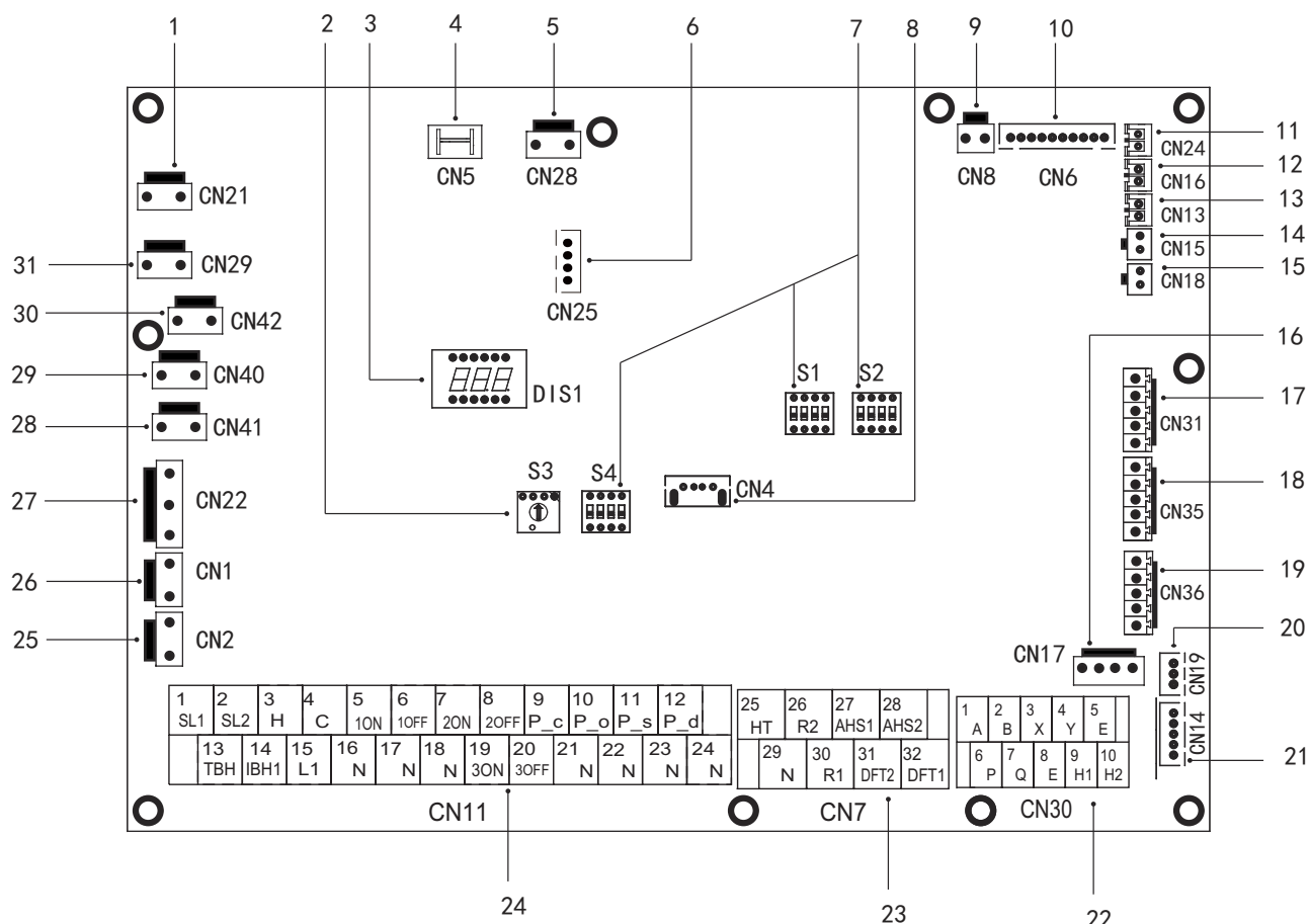
fig. 23 - Tarjeta hidráulica
