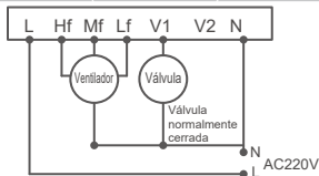
Refrigeración / refrigeración y calefacción de dos tubos (en red / sin red)
